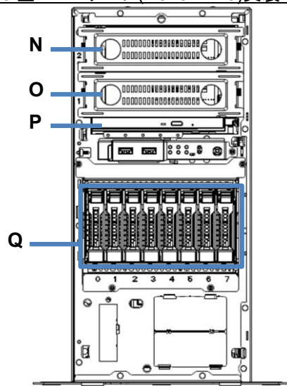
2.5 型 HDD ケージ(N8154-170)実装時
