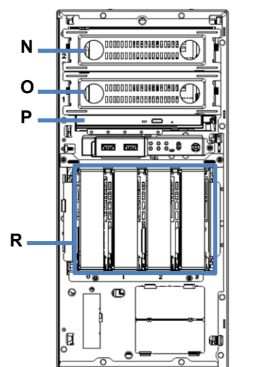
3.5 型 Fixed HDD ケージ(N8154-143)実装時
