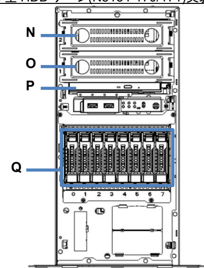
2.5 型 HDD ケージ(N8154-170/171)実装時
