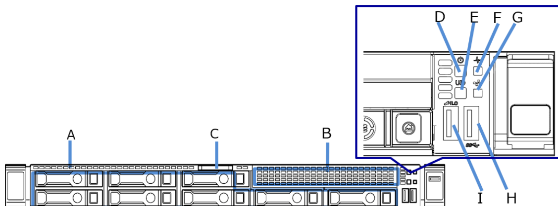
8x 2.5 型ドライブモデル正面図
