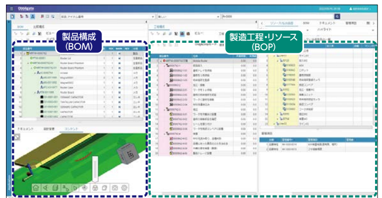
工程構成管理画面
