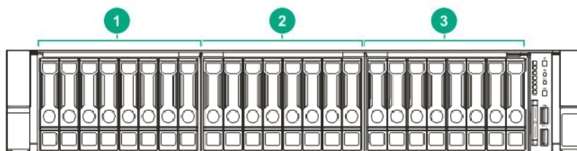
24x2.5 型ドライブモデル
