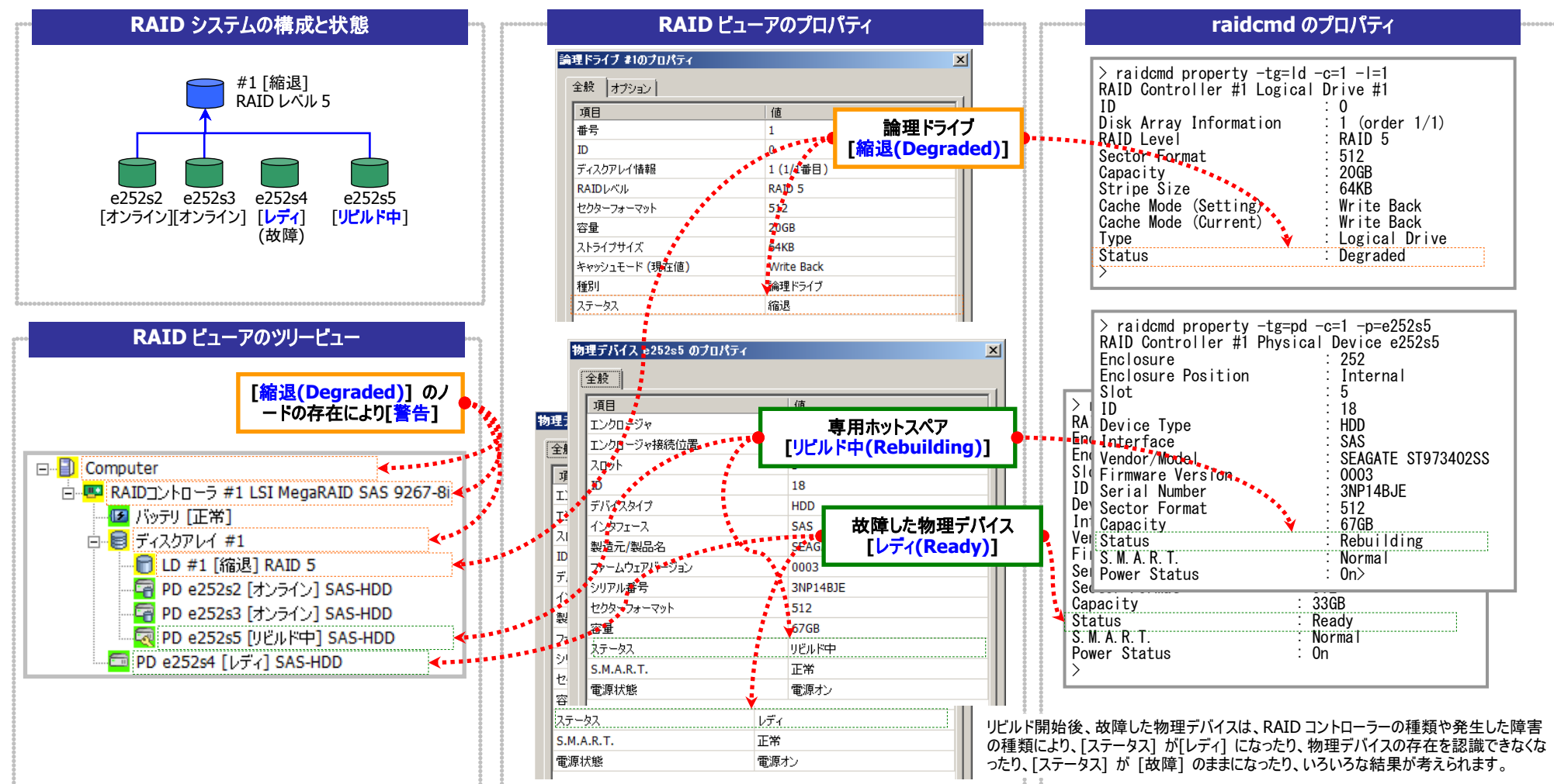
図 26 RAID ビューア/raidcmd の表示(物理デバイスのリビルド)
