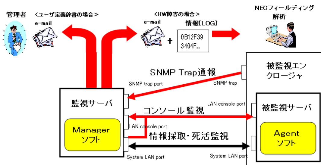
図1 サーバ監視の動作概念図 (NEC フィールドインテグレーション宛の通報は https にて送信可能)
