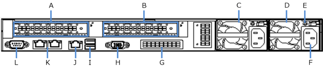
背面図
