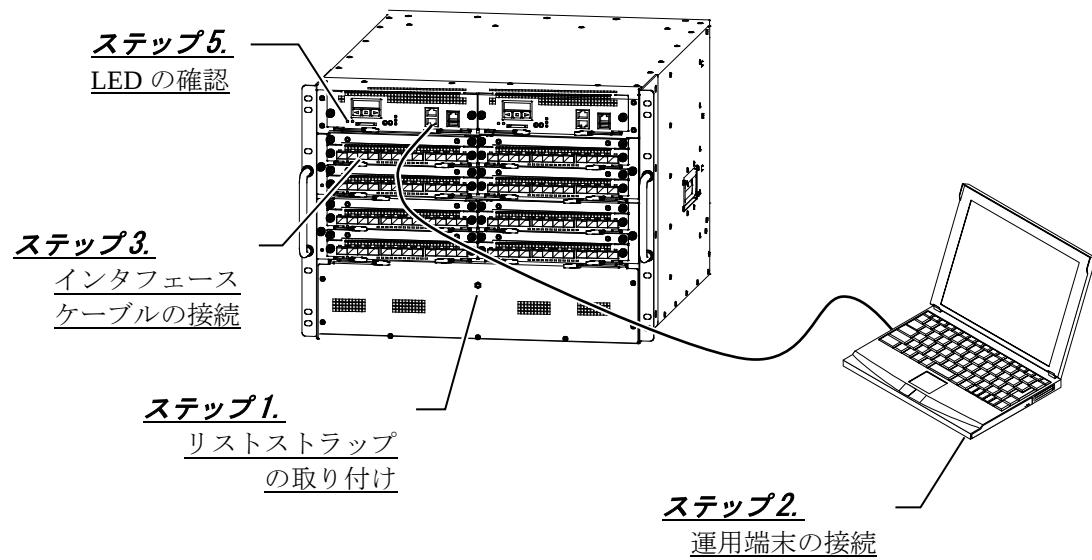
図2-4 IP8800/S8308（背面）概略図
