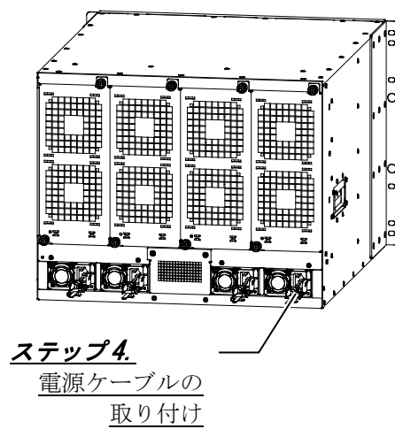
図2-4 IP8800/S8308（背面）概略図
