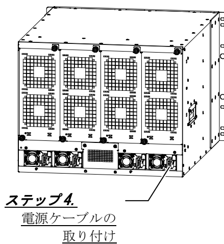
図2-6 IP8800/S8308（背面）概略図
