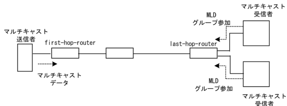
図 3-17 IPv6 PIM-SSM ネットワーク例
