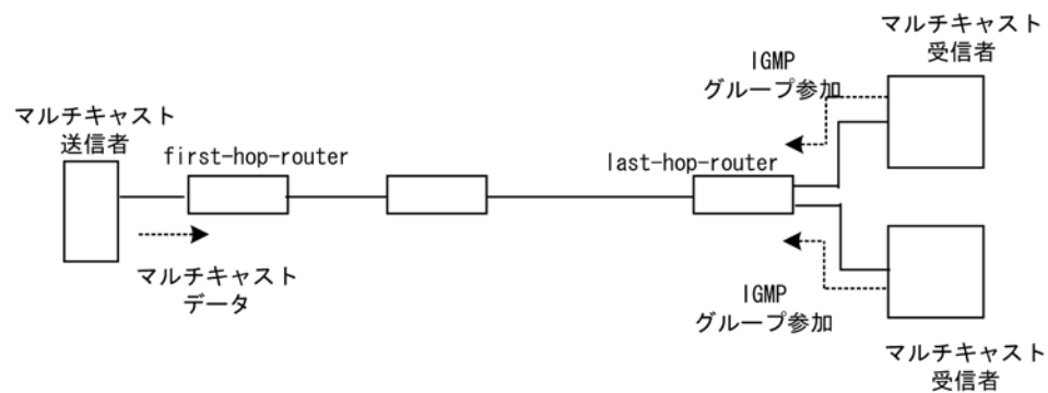
図 3-11 IPv4 PIM-SSM ネットワーク例
