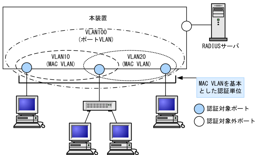
図 6-6 VLAN 単位認証（動的）の構成例
