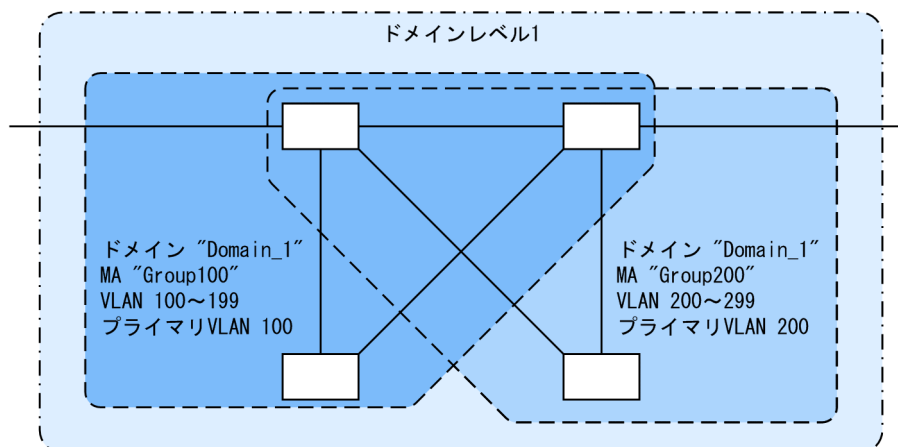
図 24-3 MA の管理範囲の例
