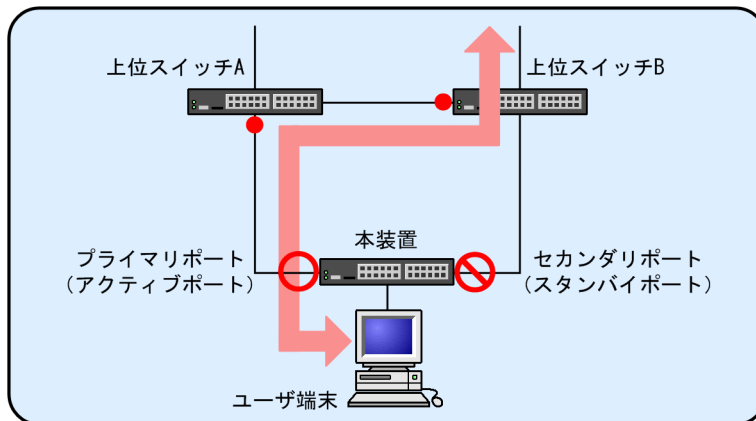
図 17-5 MAC アドレスアップデートフレームの使用による切り替え動作の違い
