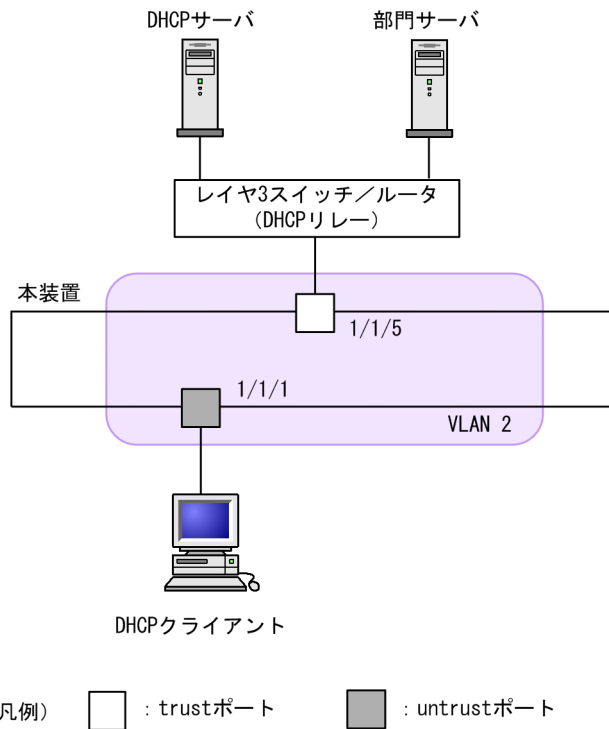
図 12-10 DHCP snooping の基本的な構成例
