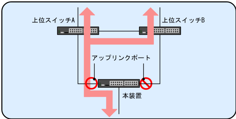
図 17-1 アップリンク・リダンダントの基本構成
