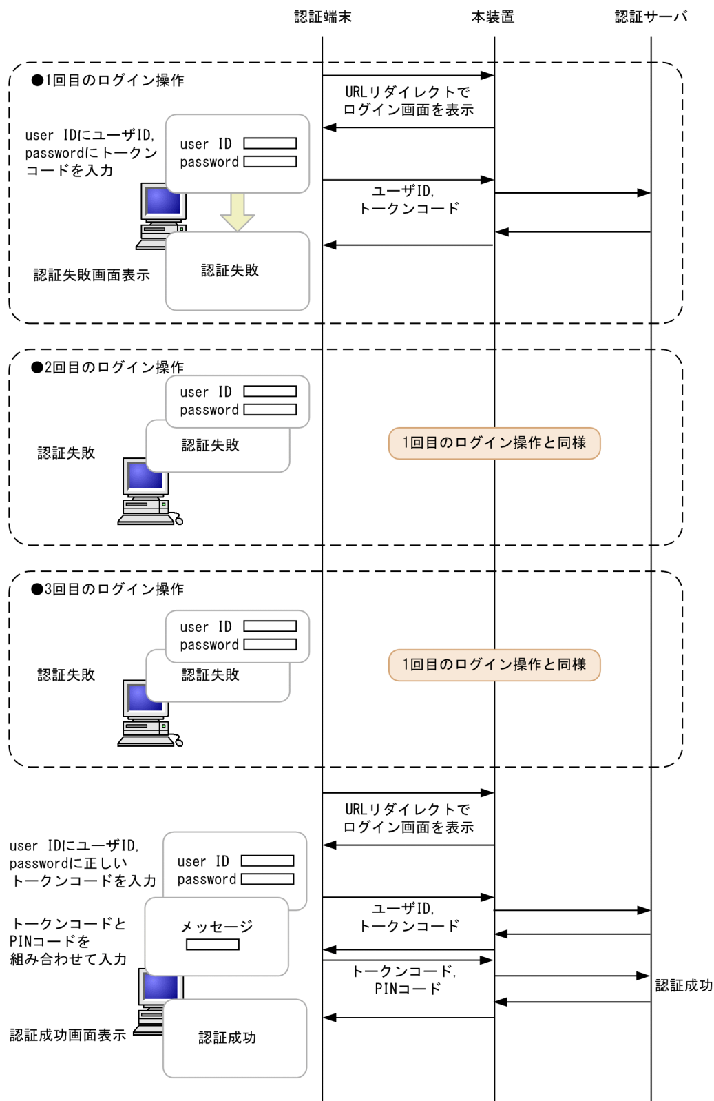
図 8-15 Next Token モードでの動作概要
