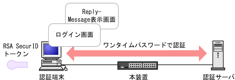
図 8-13 ワンタイムパスワード認証の構成
