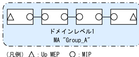
図 24-4 Up MEP の設定例
