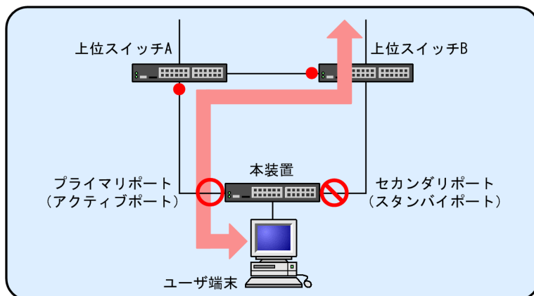
図 17-4 フラッシュ制御フレームの使用による切り替え動作の違い
