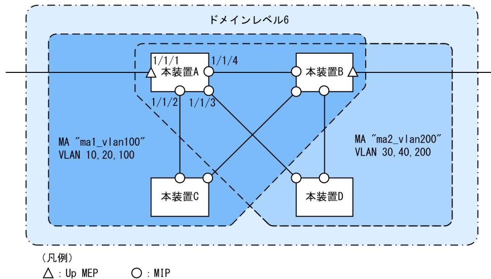
図 24-32 CFM の設定例 (同一ドメイン, 複数 MA)
