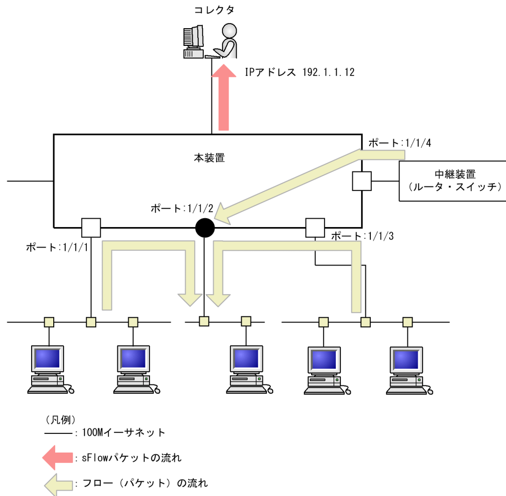
図 22-8 ポート 1/1/2 の送信パケットをモニタする設定例
