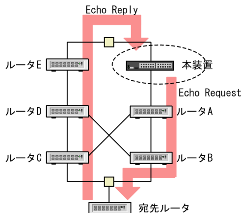
図 16-12 自装置配下ではないネットワーク上のインタフェース不一致
