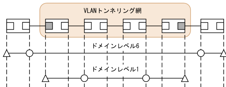
図 24-27 VLAN トネリング網内と VLAN トネリング網外で CFM を使用する例
