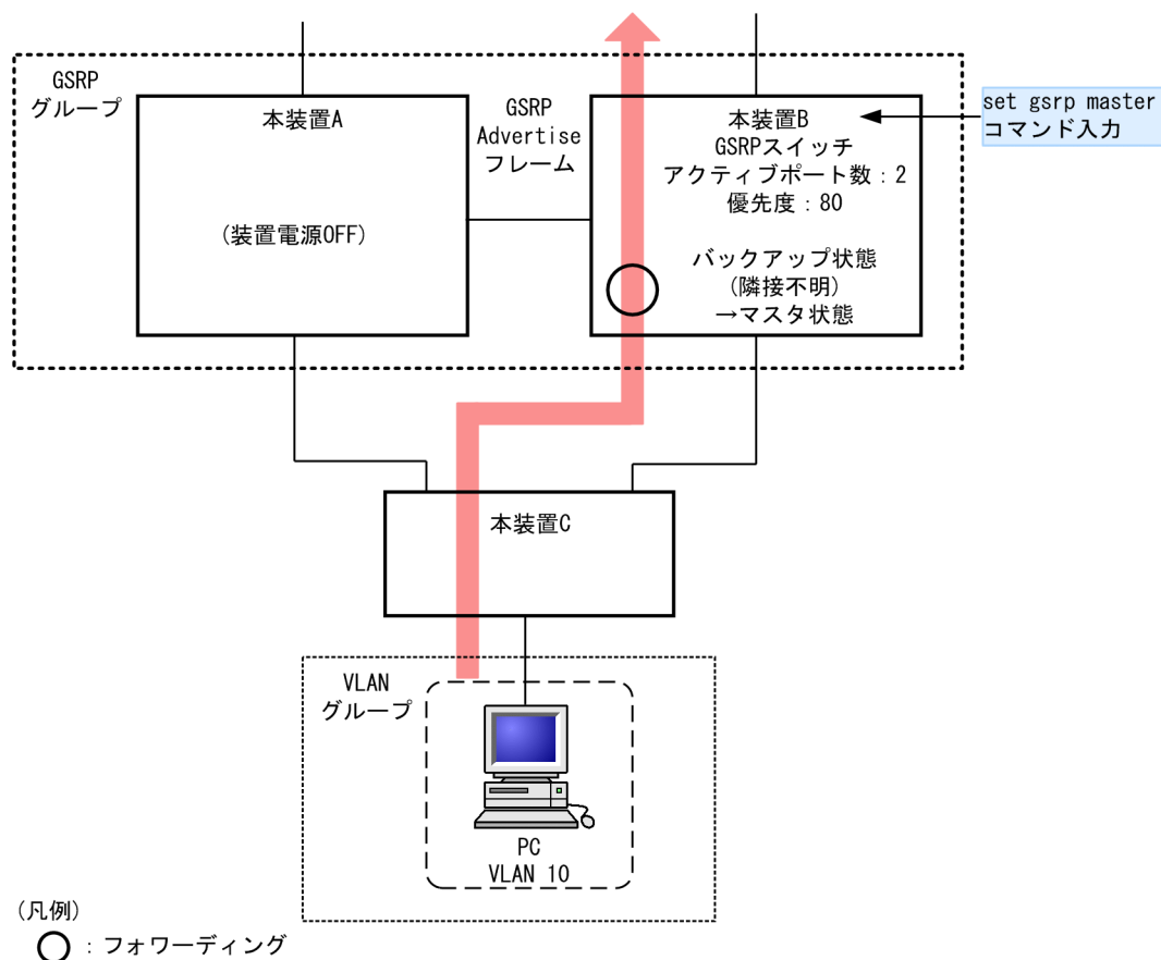
図 14-6 運用コマンド set gsrp master 入力後の動作
