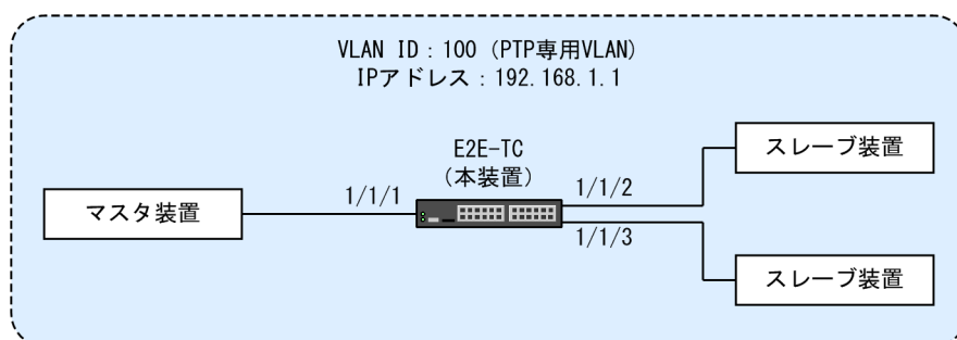
図 27-3 E2E-TC の設定例
