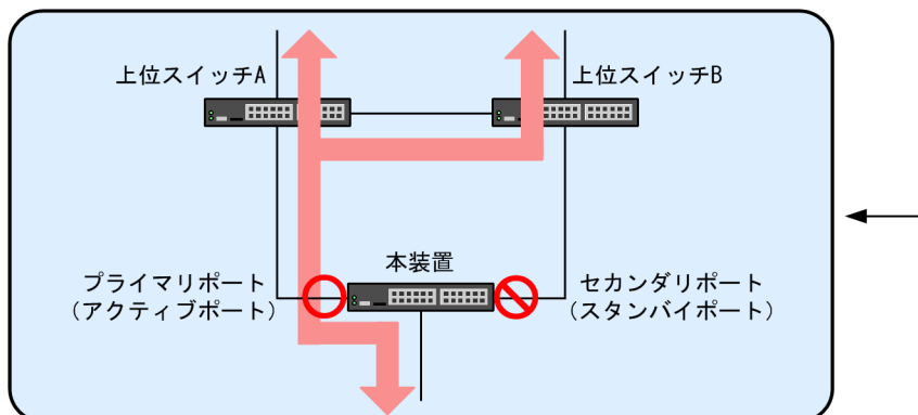
図 17-2 アップリンク・リダンダントの動作概要
