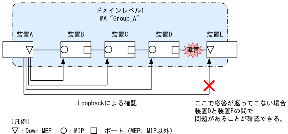
図 24-11 ドメイン内に MIP を設定した構成の例
