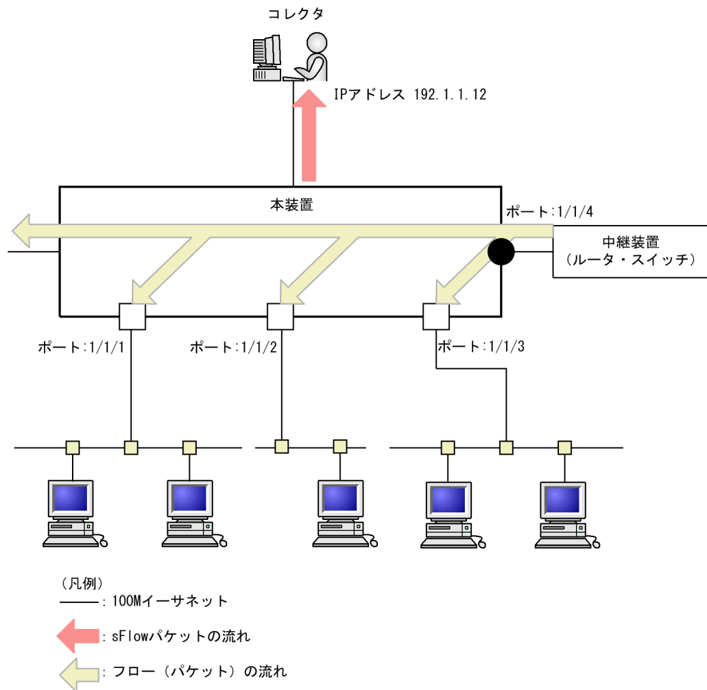
図 22-7 ポート 1/1/4 の受信パケットをモニタする設定例
