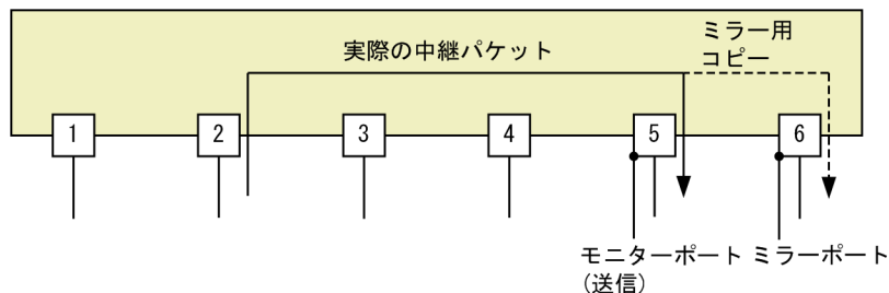
図 20-2 送信フレームのミラーリング
