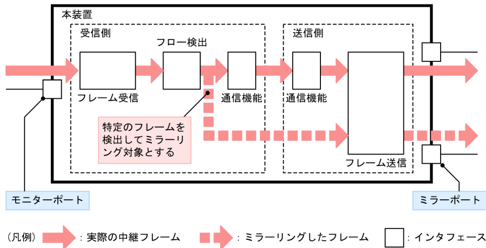
図 21-1 受信フレームのミラーリング
