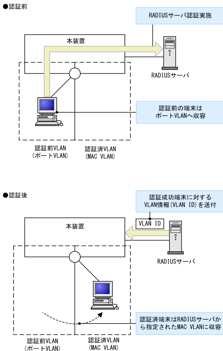
図 6-7 VLAN 単位認証（動的）の動作イメージ
