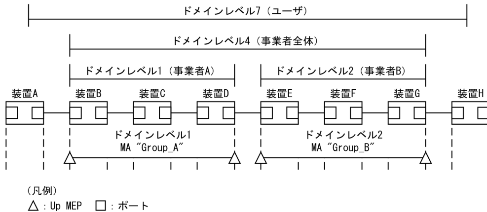
図 24-13 ドメインレベル 1, 2 の設定
