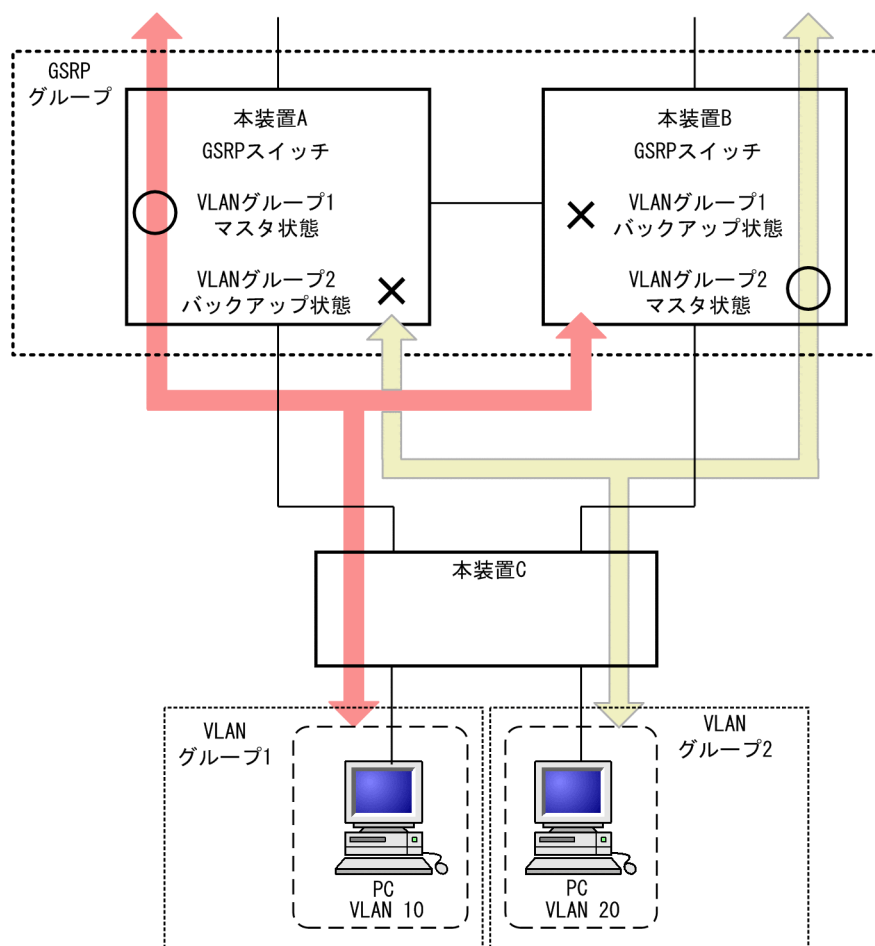
図 14-10 ロードバランス構成
