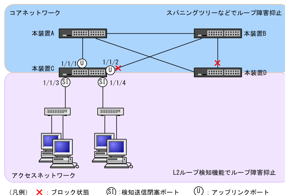
図 18-6 L2 ループ検知の設定例
