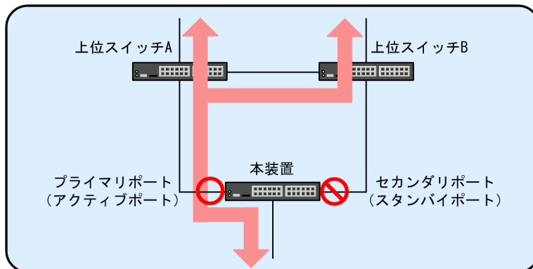
図 17-3 切り替え動作
