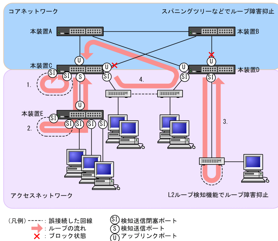
図 18-3 L2 ループ検知機能を適用したネットワーク構成
