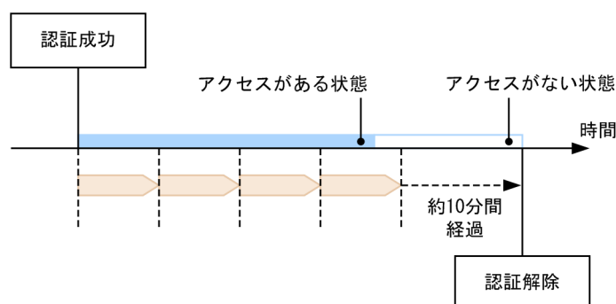
図 8-16 認証済み端末の MAC アドレステーブルエージングによるログアウト
