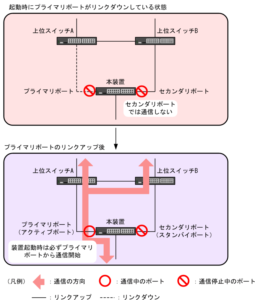
図 17-6 装置起動時のアクティブポート固定機能有効時の動作
