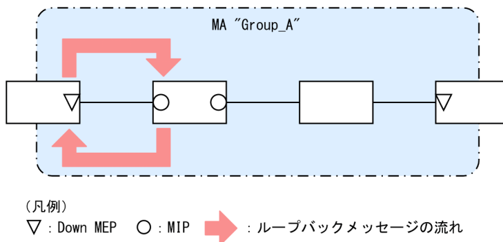
図 24-21 MIP に対して Loopback を実行
