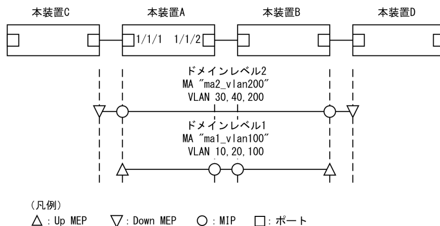
図 24-31 CFM の設定例（複数ドメイン）
