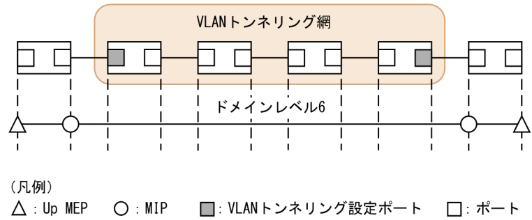
図 24-29 VLAN トンネリング網外だけで CFM を使用する例
