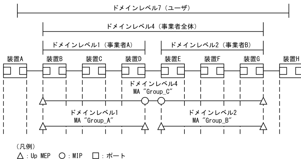
図 24-14 ドメインレベル 4 の設定
