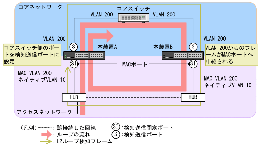
図 18-5 ループ検知可能な構成
