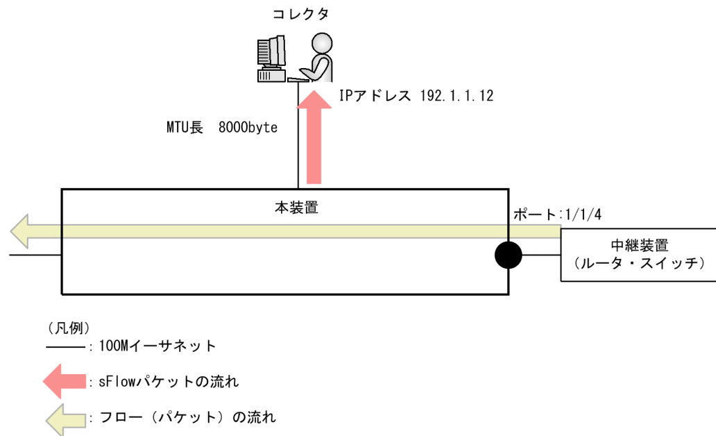
図 22-9 コレクタへの送信を MTU=8000byte に設定する例
