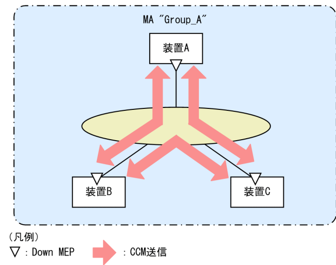
図 24-18 CC での常時接続性の監視
