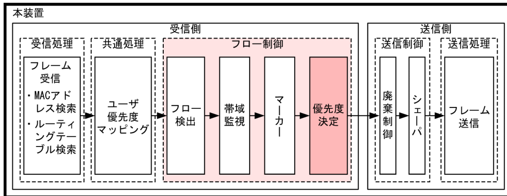
図 3-16 優先度決定の位置づけ
