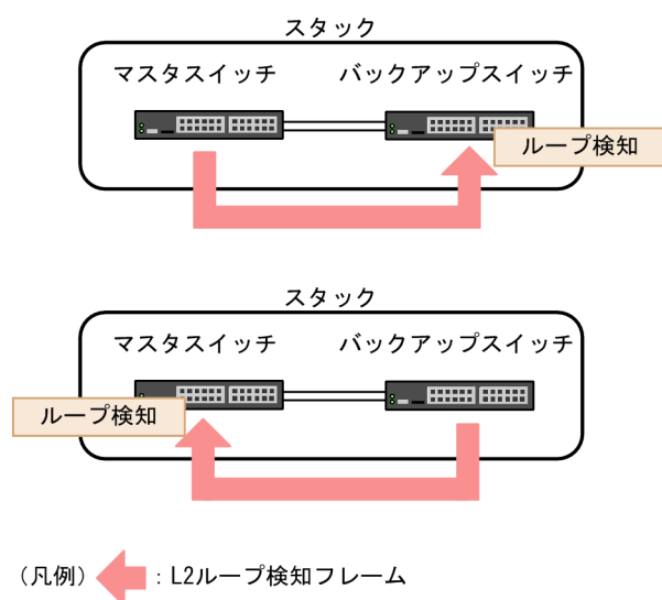
図 18-2 スタック構成時の L2 ループ検知フレームの受信によるループ検知
