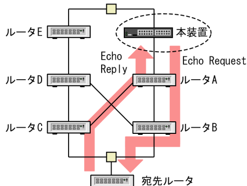
図 16-12 自装置配下ではないネットワーク上のインタフェース不一致
