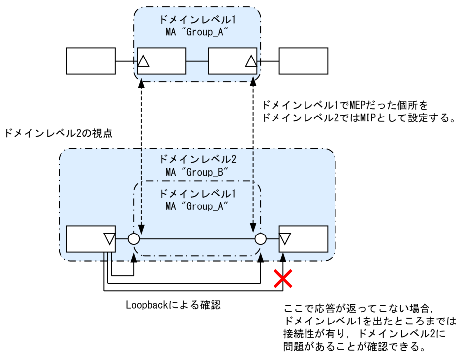
図 24-9 ドメインレベル 1 とドメインレベル 2 の階層構造の例
