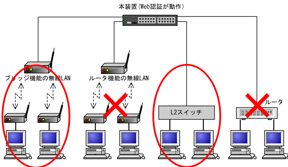
図 8-26 本装置と端末間の接続
