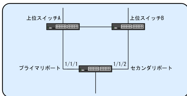
図 17-7 アップリンク・リダンダントの設定例
