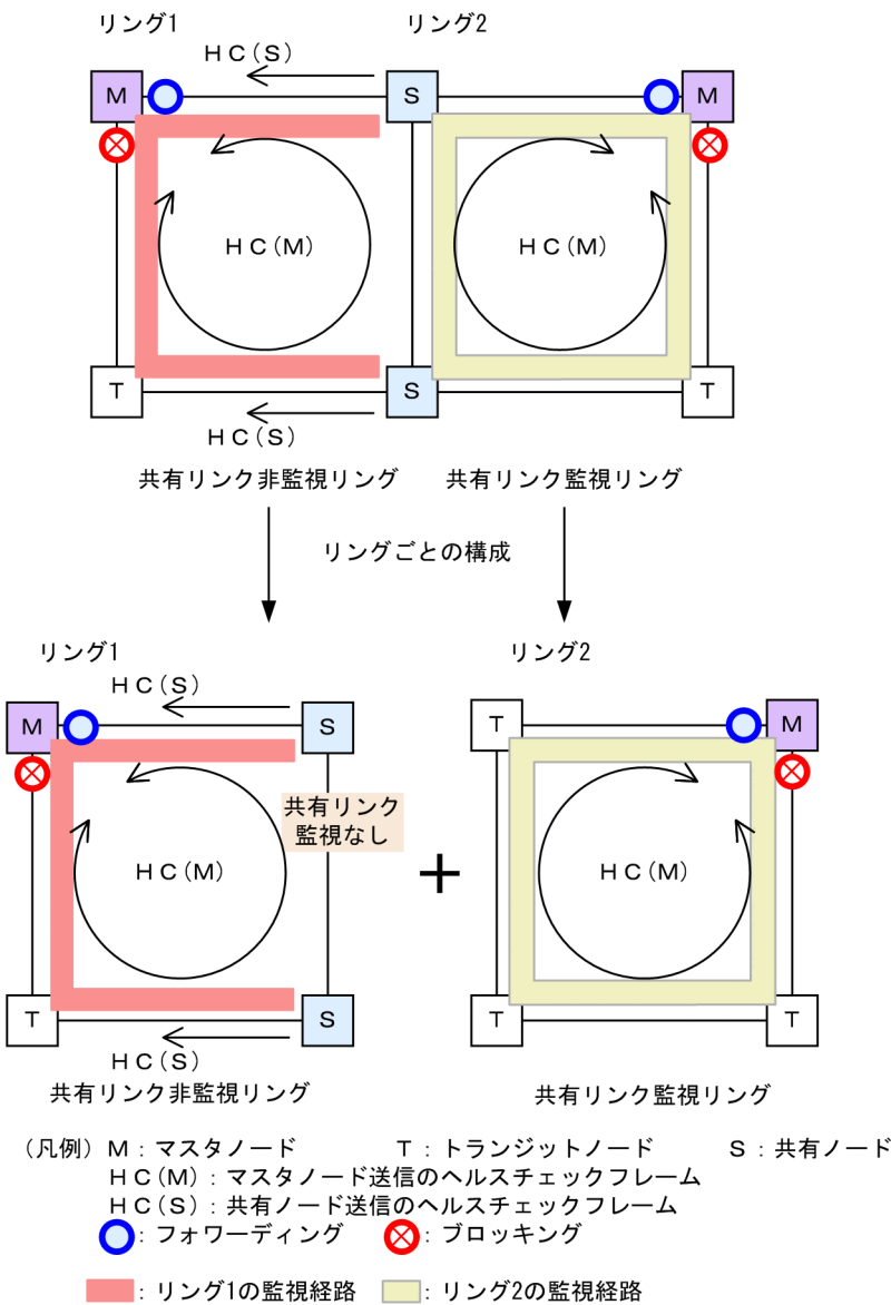
図 28-13 リング正常時の状態
