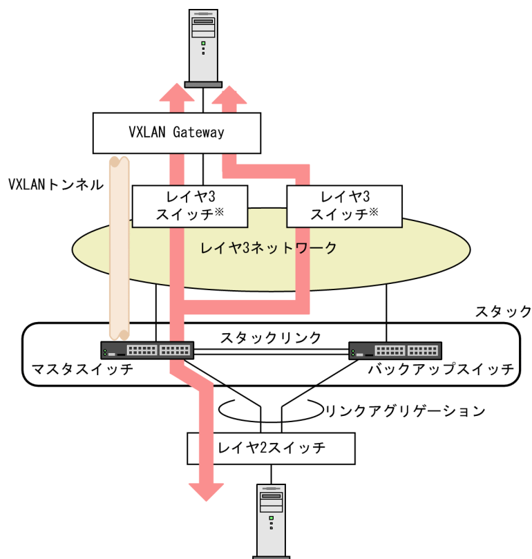
図 26-7 スタック構成での VXLAN 使用例
