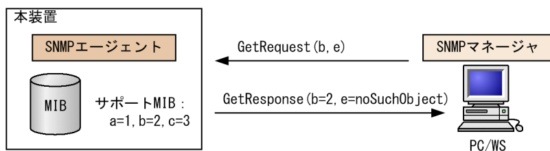
図 19-8 GetRequest オペレーション (SNMPv2C)
