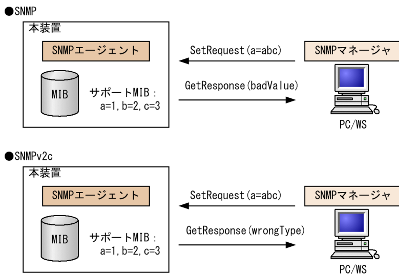
図 19-14 設定値のタイプが正しくない場合の SetRequest オペレーション例
