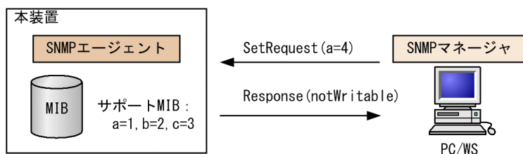
図 19-21 MIB 変数が読み出し専用の場合の SetRequest オペレーション
