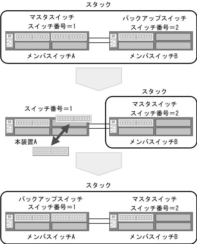
図 8-12 マスタスイッチ（メンバスイッチ A）の NIF を異なる NIF 種別に交換
