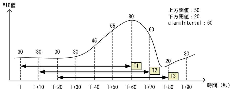
図 19-29 delta 方式による MIB 監視例
