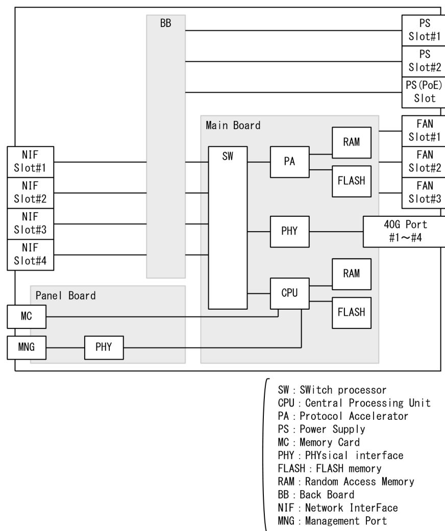
図 2-2 ハードウェアの構成
