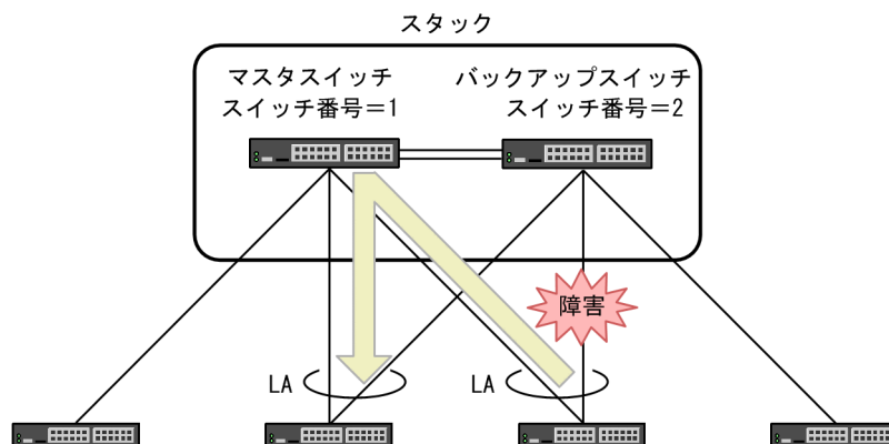
図 7-13 転送元のポート障害時の転送動作（リンクアグリゲーション）
