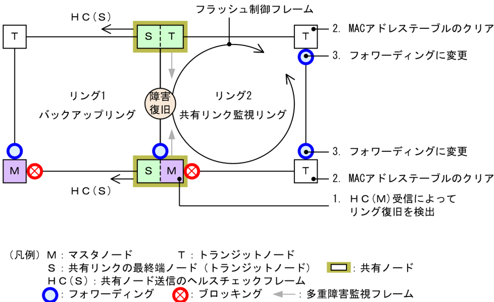
図 28-38 共有リンク障害復旧時の動作
