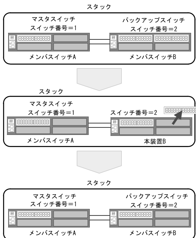
図 8-9 バックアップスイッチ (メンバスイッチ B) の NIF を抜去
