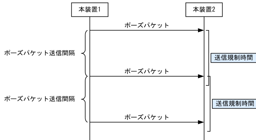
図 20-4 デフォルトでの動作シーケンス
