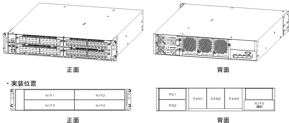
図 2-1 IP8800/S4630-4M モデル
