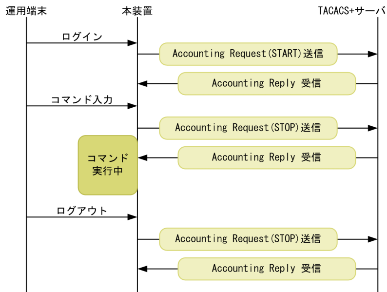
図 10-31 TACACS+アカウントティングのシーケンス (ログインアカウントティング START-STOP, コマンドアカウントティング STOP-ONLY 送信モード時)
