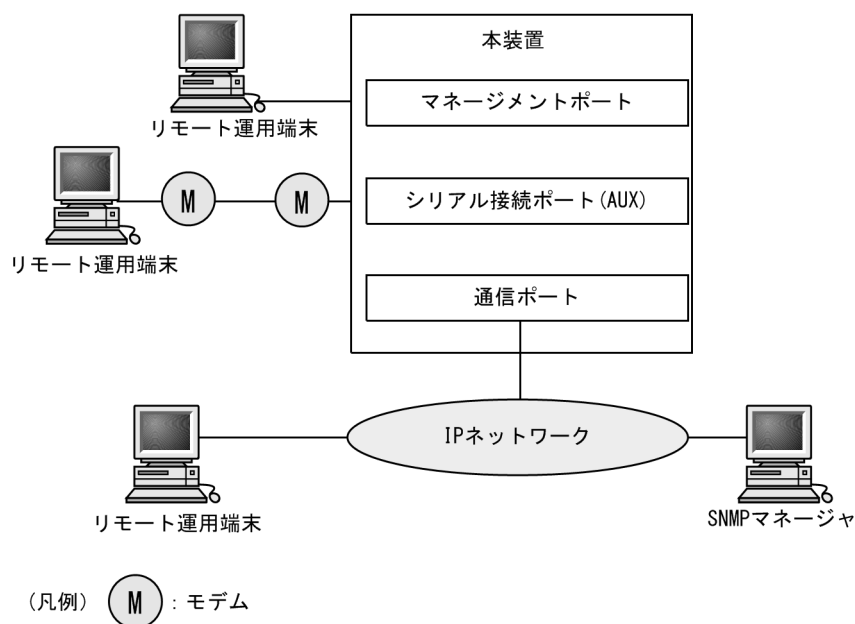
図 4-2 リモート運用端末の接続形態
