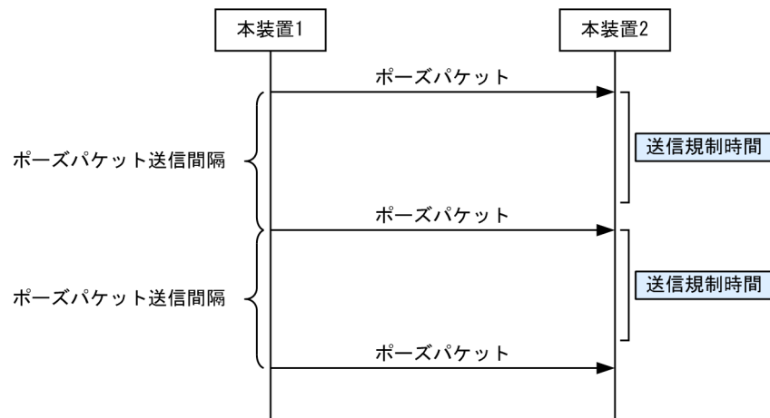
図 20-5 ルーズモードでの動作シーケンス
