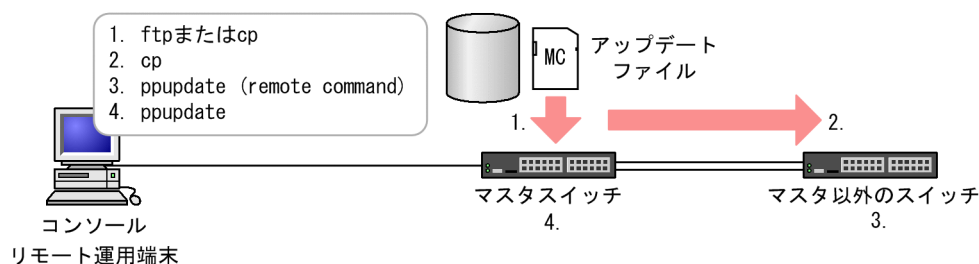
図 16-3 スタック構成でアップデートする流れ
