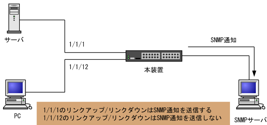
図 19-31 リンクトラップの構成図
