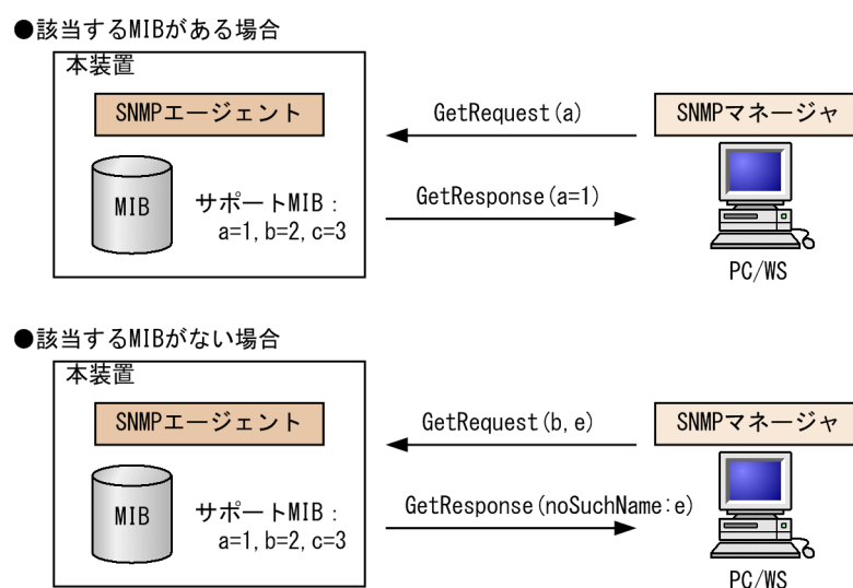
図 19-7 GetRequest オペレーション
