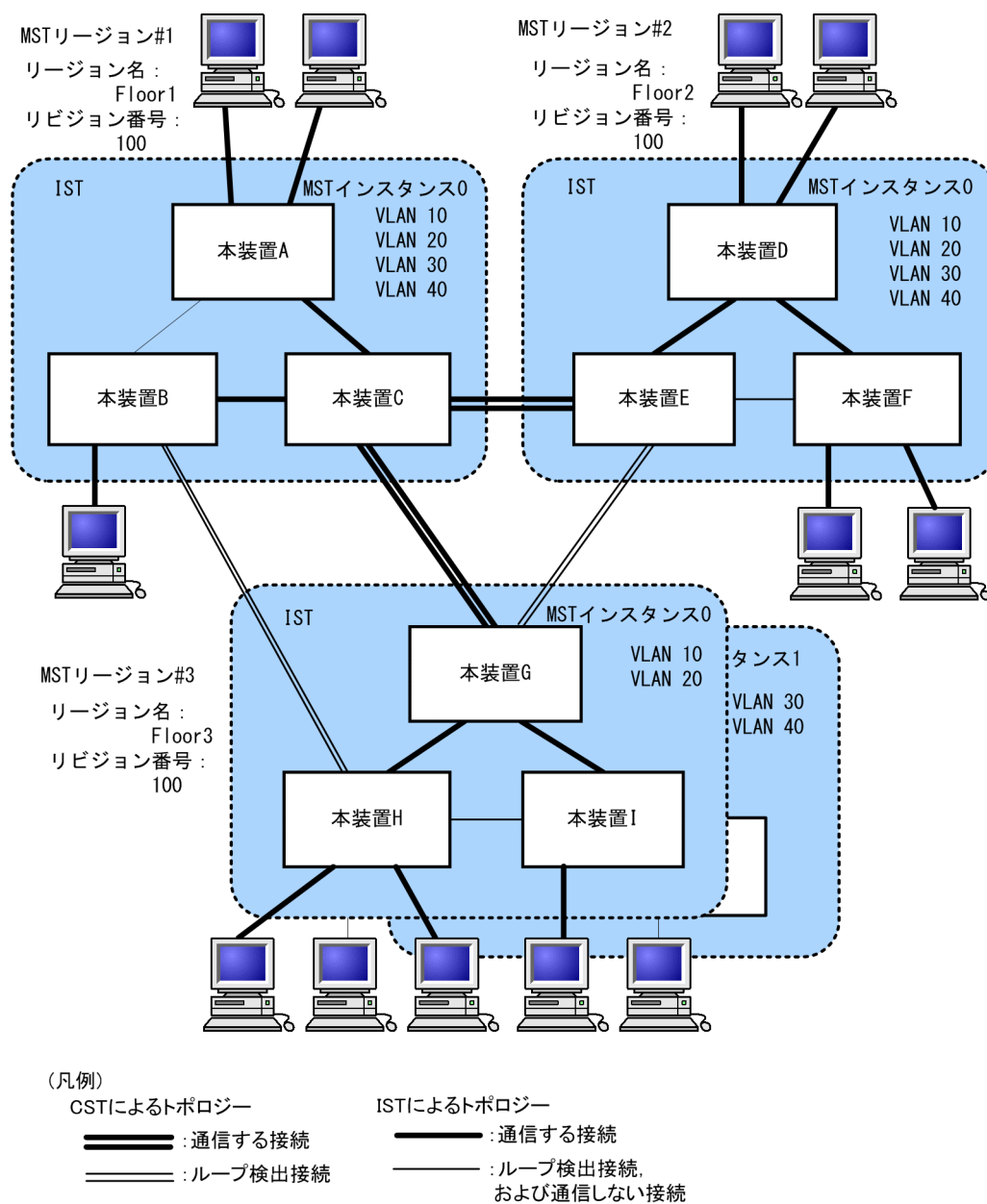
図 27-12 マルチプルスパニングツリー概要
