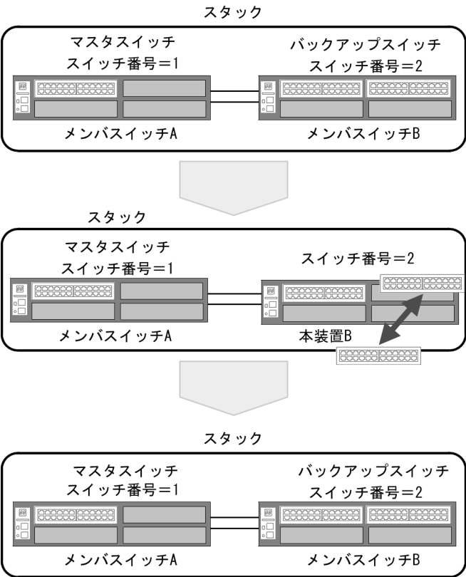
図 8-11 バックアップスイッチ（メンバスイッチ B）の NIF を交換
