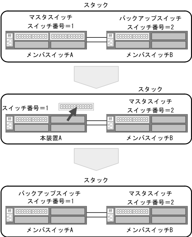
図 8-8 マスタスイッチ（メンバスイッチ A）の NIF を抜去
