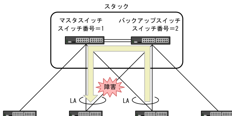
図 7-14 転送先のポート障害時の転送動作（リンクアグリゲーション）
