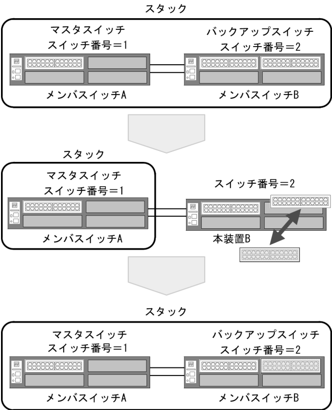
図 8-13 バックアップスイッチ（メンバスイッチ B）の NIF を異なる NIF 種別に交換
