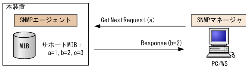
図 19-18 GetNextRequest オペレーション
