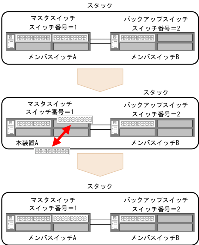
図 8-10 マスタスイッチ（メンバスイッチ A）の NIF を交換
