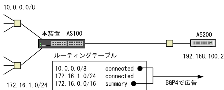
図 7-18 集約経路を BGP4 で広告する構成
