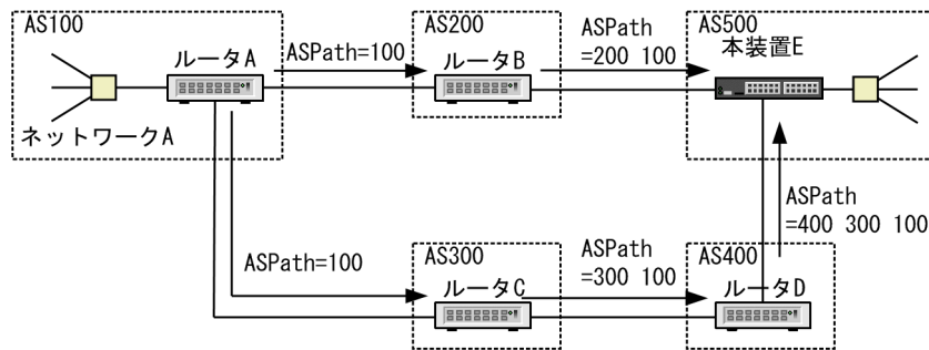
図 28-3 AS_PATH 属性による経路選択
