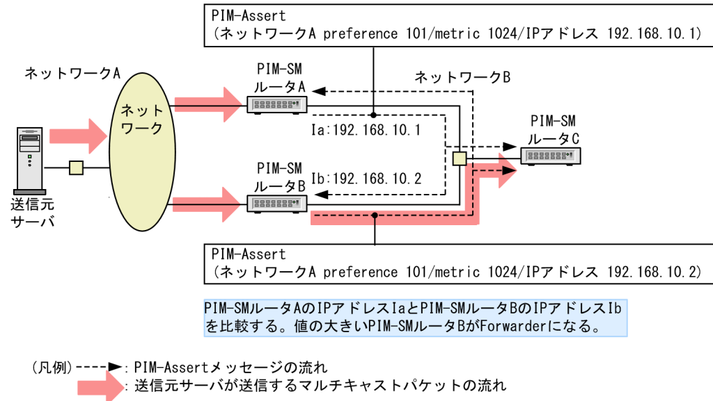
図 14-14 Forwarder の決定
