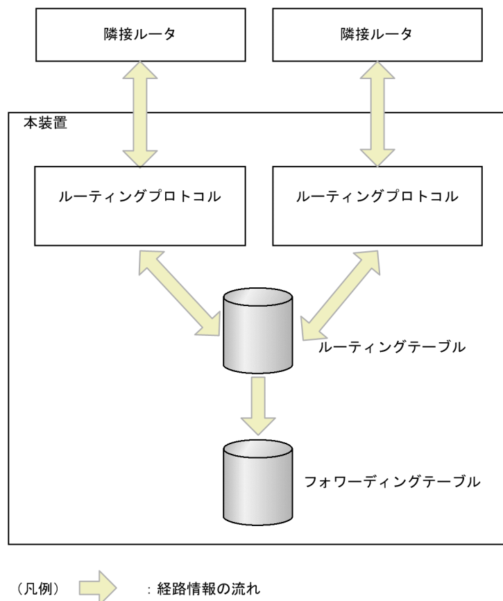
図 23-1 ルーティングの概要
