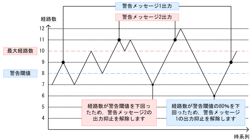
図 7-22 経路数と警告メッセージ出力の関係
