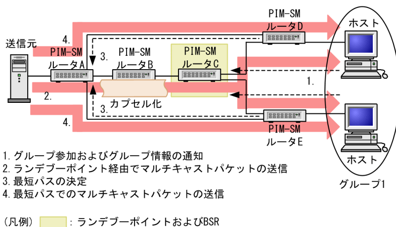
図 14-7 PIM-SM の動作概要
