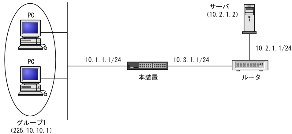
図 15-1 PIM-SM 構成例
