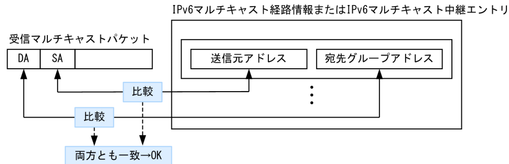
図 30-5 IPv6 マルチキャスト経路情報または IPv6 マルチキャスト中継エントリの検索方法
