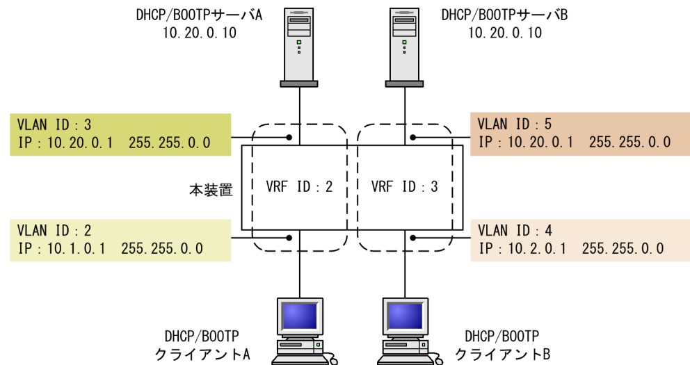
図 5-3 VRF 構成
