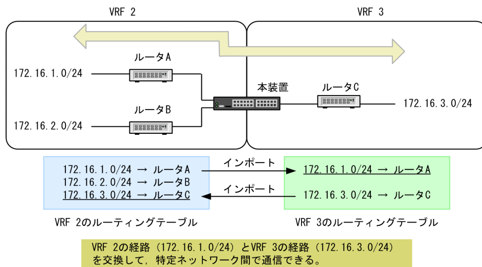
図 7-23 VRF 間の経路交換
