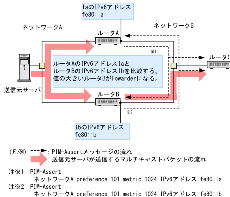
図 30-14 Forwarder の決定
