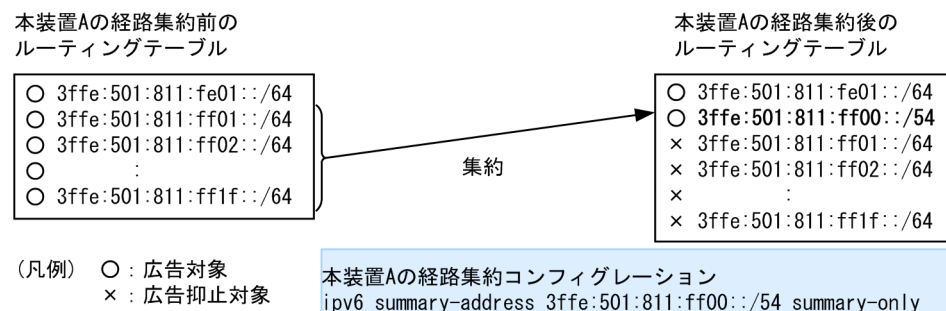
図 23-7 経路集約のコンフィグレーション例と経路集約前後の経路
