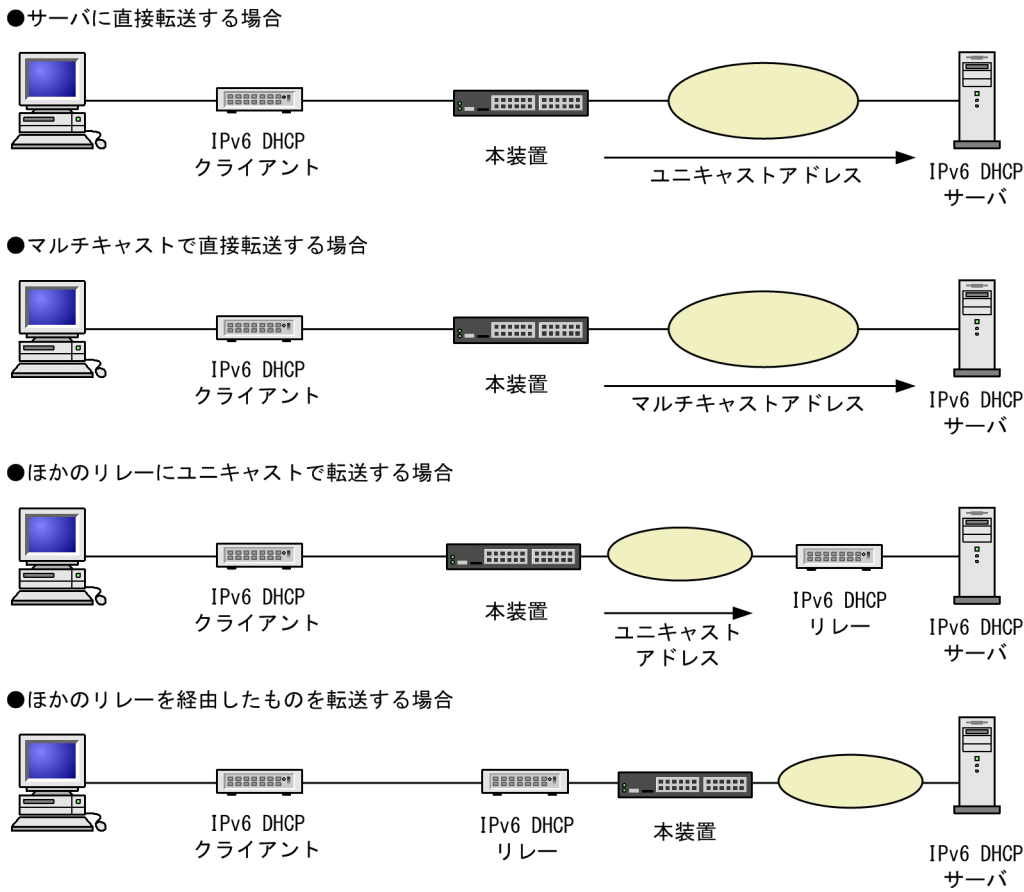
図 21-1 IPv6 DHCP リレーの接続構成
