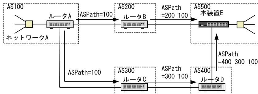
図 12-3 AS_PATH 属性による経路選択
