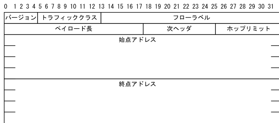
図 17-19 IPv6 ヘッダ形式
