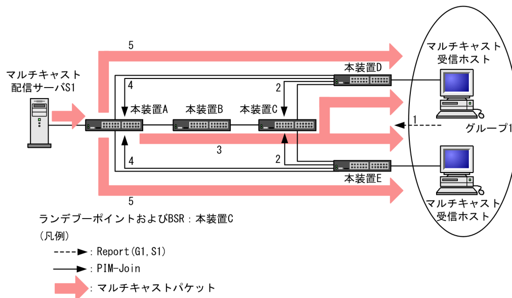
図 14-20 IGMPv3 使用時の IPv4 PIM-SM 動作概要
