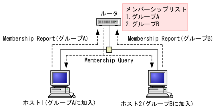
図 14-3 IGMPv2 グループの参加・離脱
