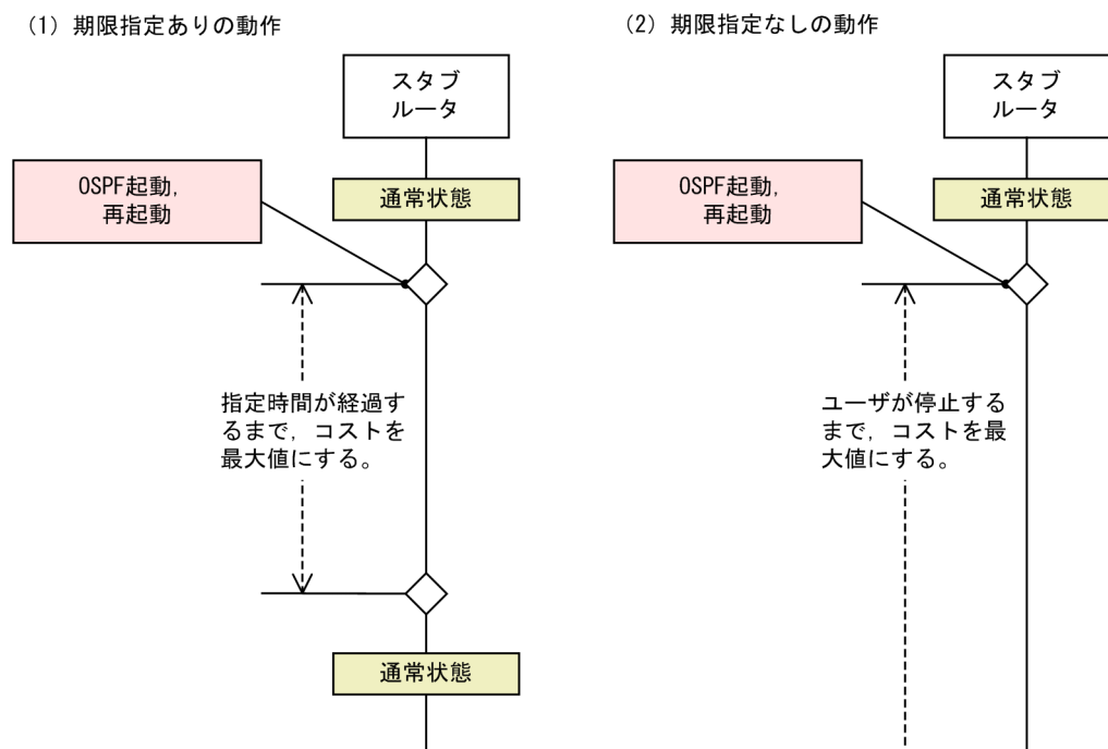
図 11-7 スタブルータの動作
