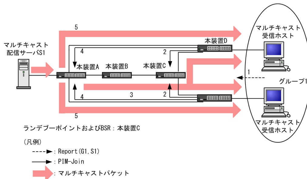
図 30-16 MLDv2 使用時の IPv6 PIM-SM 動作概要
