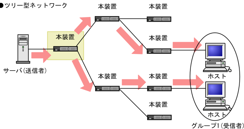
図 30-32 IPv6 PIM-SM 推奨ネットワーク構成
