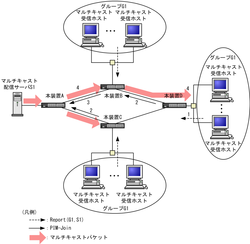
図 30-19 IPv6 PIM-SSM 動作概要（ホストが MLDv2（INCLUDE モード）の場合）
