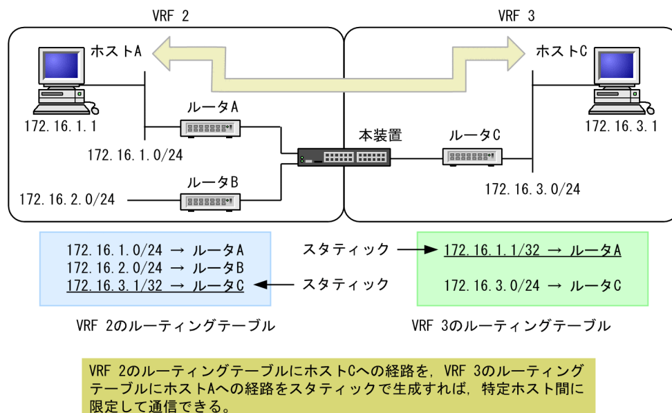
図 7-24 VRF 間にわたるスタティックルーティング
