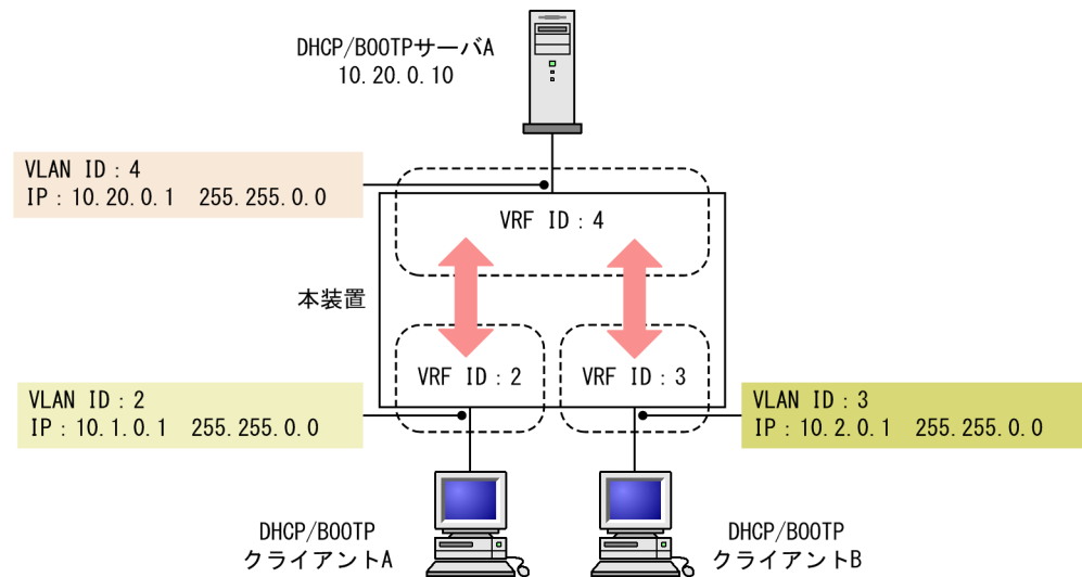
図 5-4 エクストラネット構成
