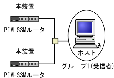
図 30-34 注意が必要な構成（複数ルータとホストの接続）
