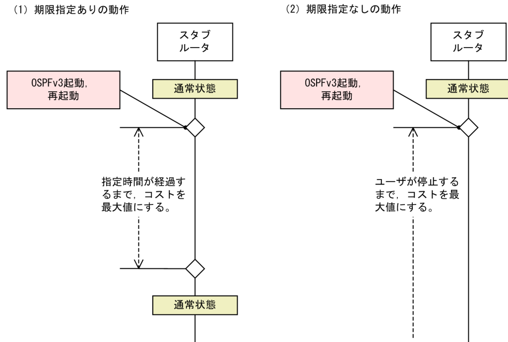
図 27-5 スタブルータの動作
