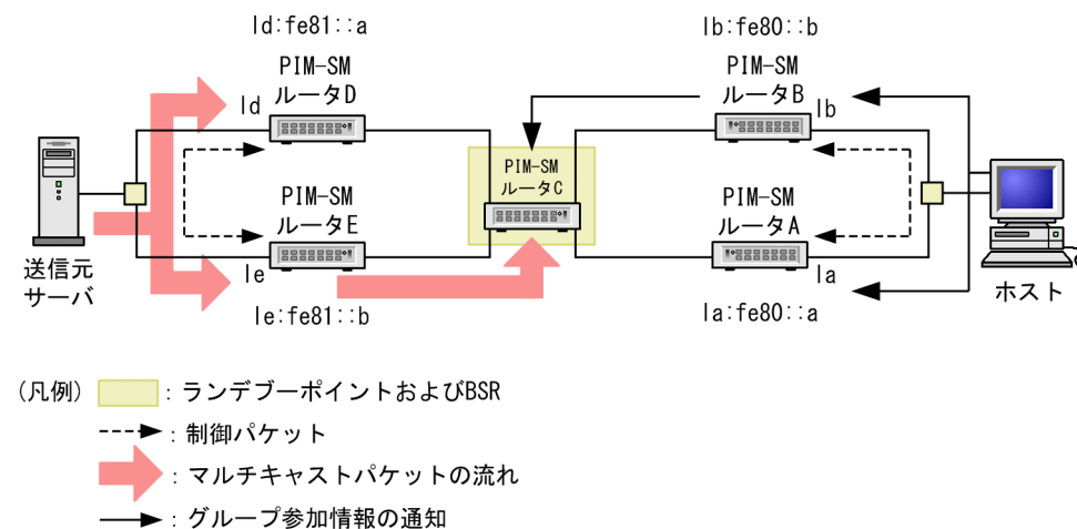
図 30-15 DR の動作
