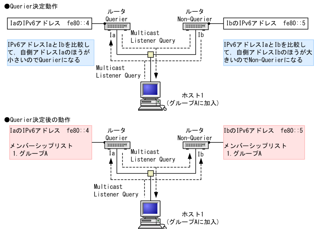
図 30-4 Querier と Non-Querier の決定
