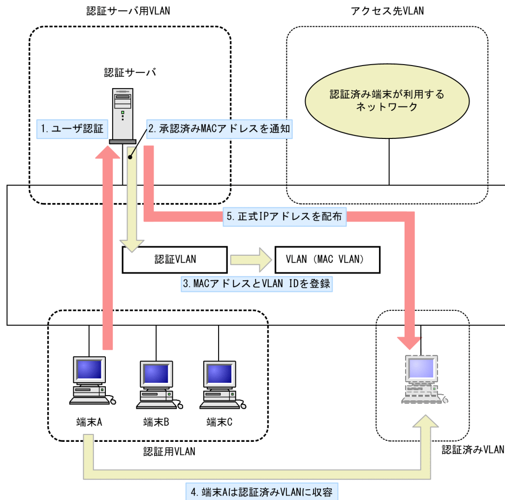
図 12-1 認証 VLAN 基本構成
