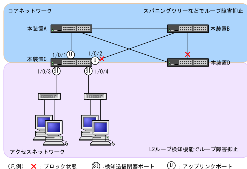
図 18-6 L2 ループ検知の設定例
