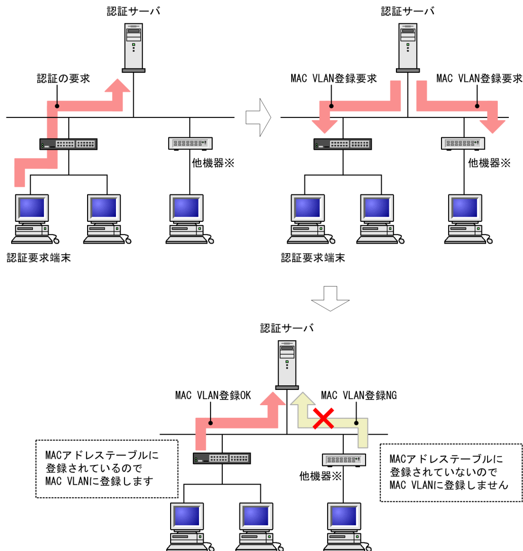
図 12-5 認証対象端末だけの登録
