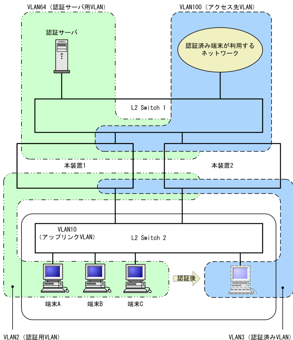
図 12-3 認証 VLAN 冗長構成
