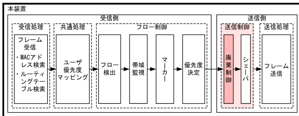
図 4-8 廃棄制御の位置づけ
