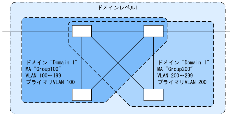
図 23-3 MA の管理範囲の例
