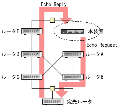
図 16-12 自装置配下ではないネットワーク上のインタフェース不一致
