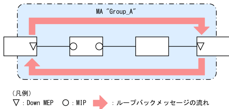
図 23-22 MEP に対して Loopback を実行
