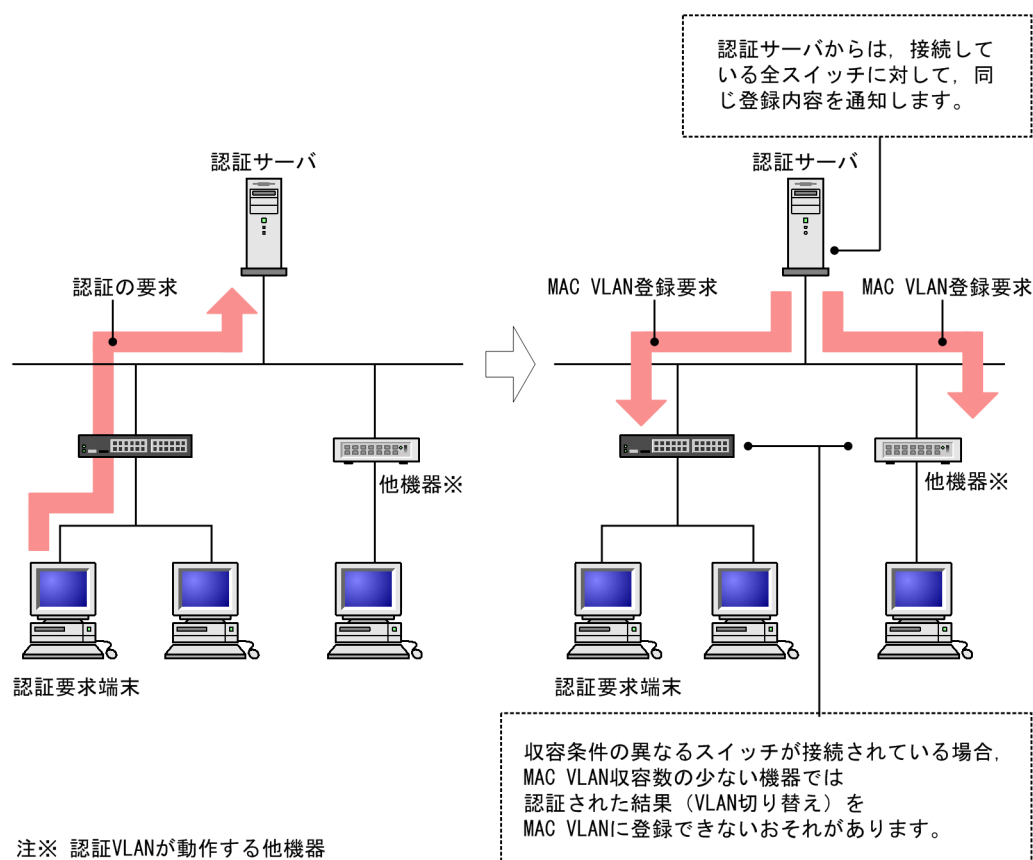
図 12-4 通常モードでの動作
