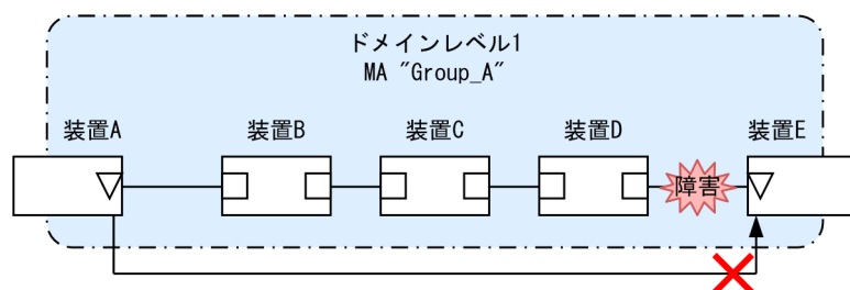
図 23-10 ドメイン内に MIP が設定されていない構成の例
