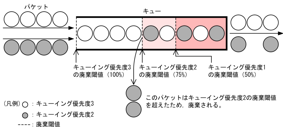
図 4-9 テールドロップの概念
