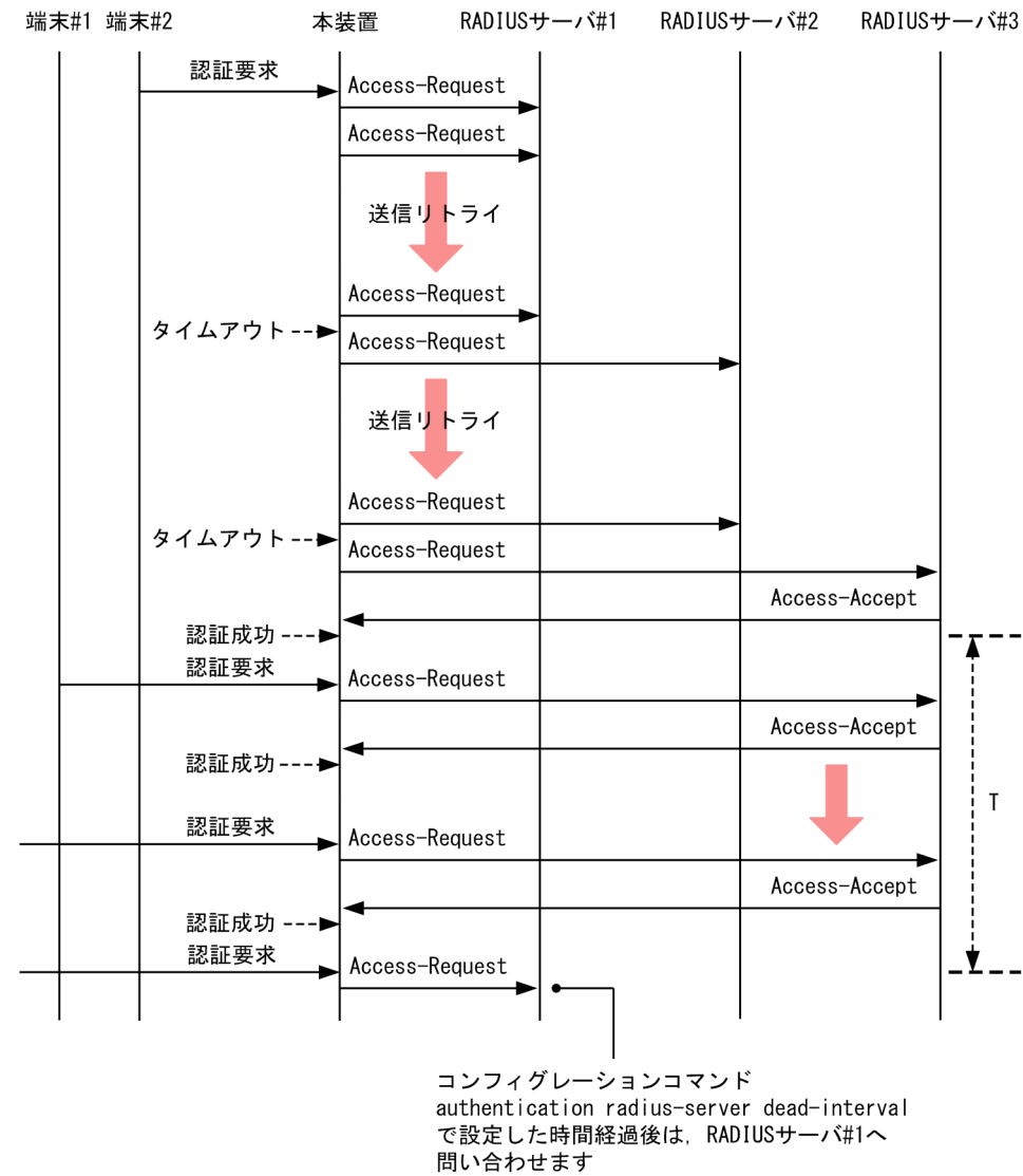
図 5-7 RADIUS サーバ通信の dead interval 機能
