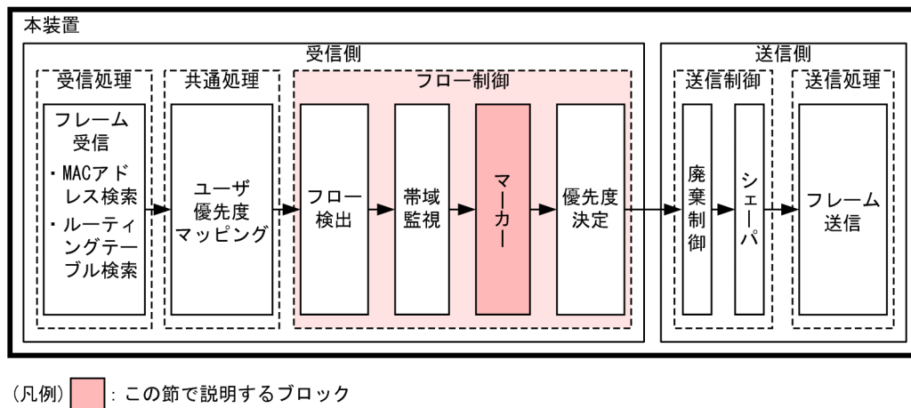
図 3-8 マーカーの位置づけ
