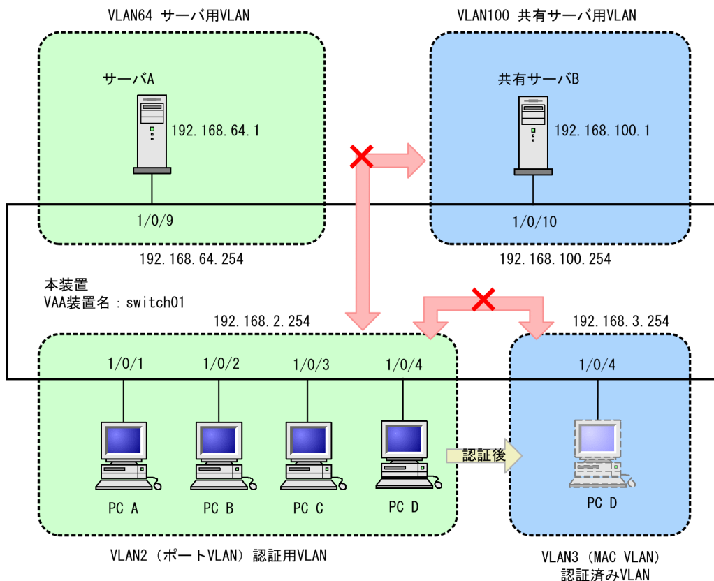
図 12-6 認証 VLAN 基本構成
