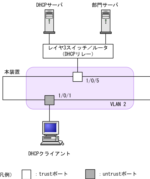
図 13-10 DHCP snooping の基本的な構成例
