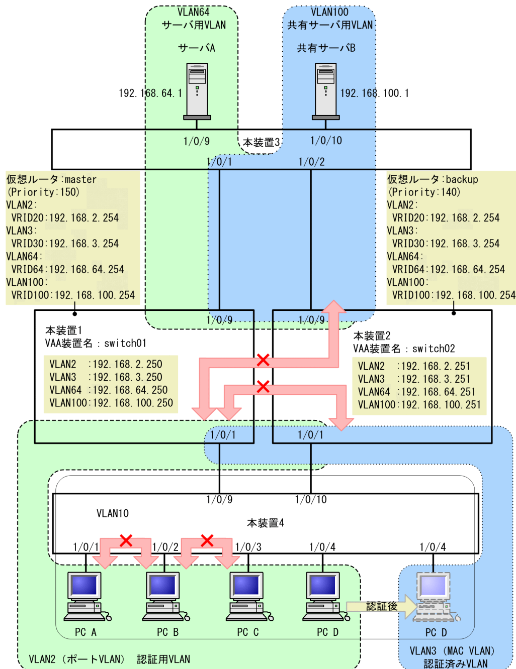
図 12-7 認証 VLAN 冗長構成
