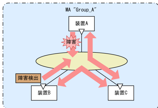
図 23-19 CC で障害を検出
