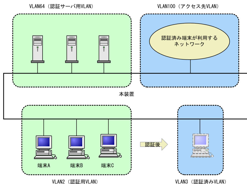
図 12-2 認証サーバ複数台構成
