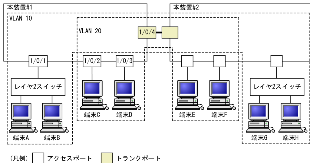
図 23-4 ポート VLAN の設定例
