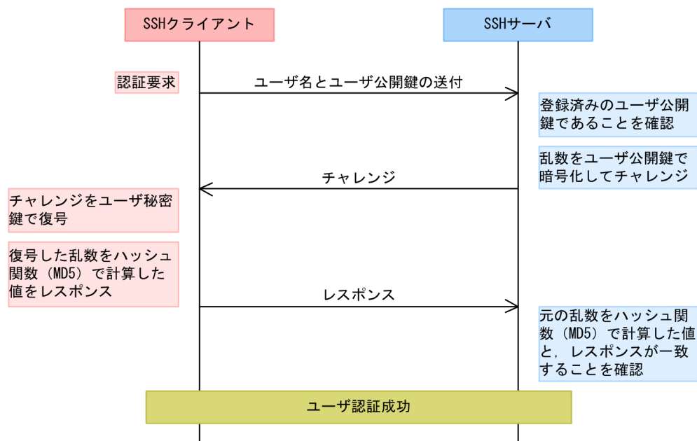
図 11-10 公開鍵暗号方式によるユーザ認証の流れ (SSHv1)
