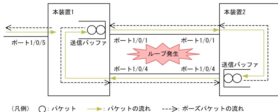
図 19-2 相互に送信規制する例
