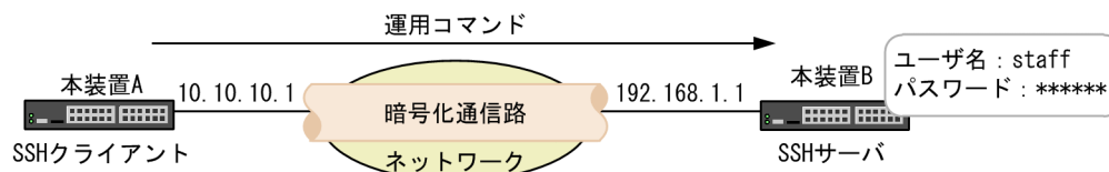
図 11-21 SSH クライアントから SSH サーバでコマンドを実行する構成例
