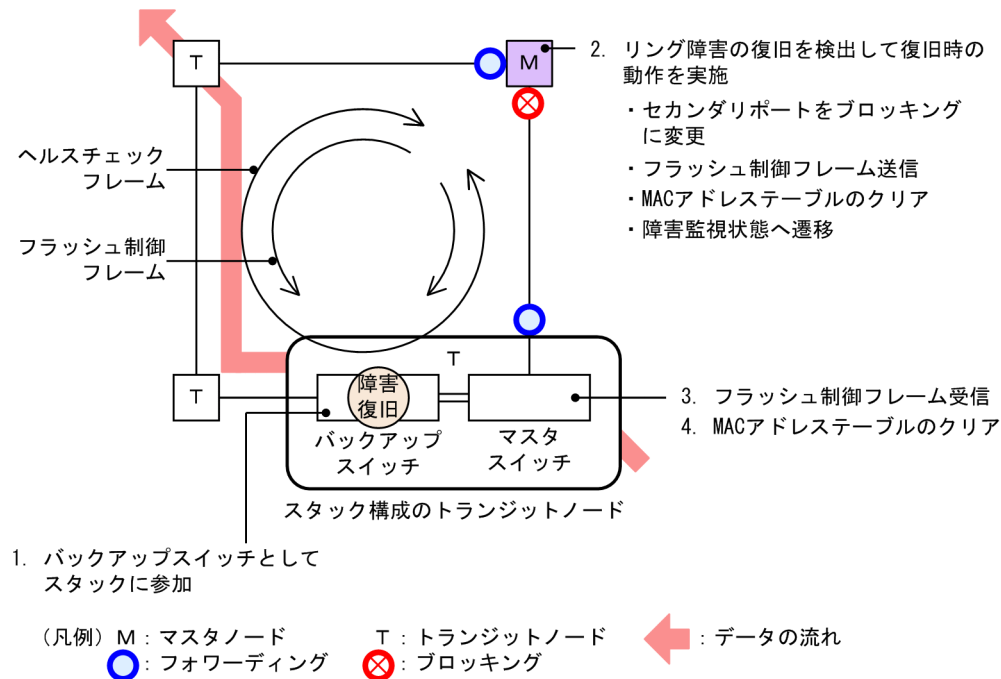
図 26-29 トランジットノードでのメンバスイッチ障害復旧時の動作
