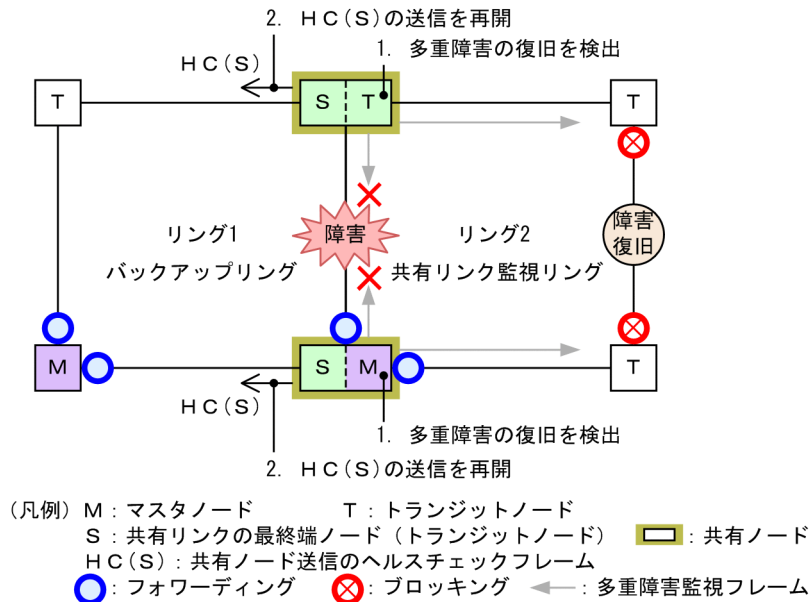
図 26-36 多重障害からの一部復旧時の動作
