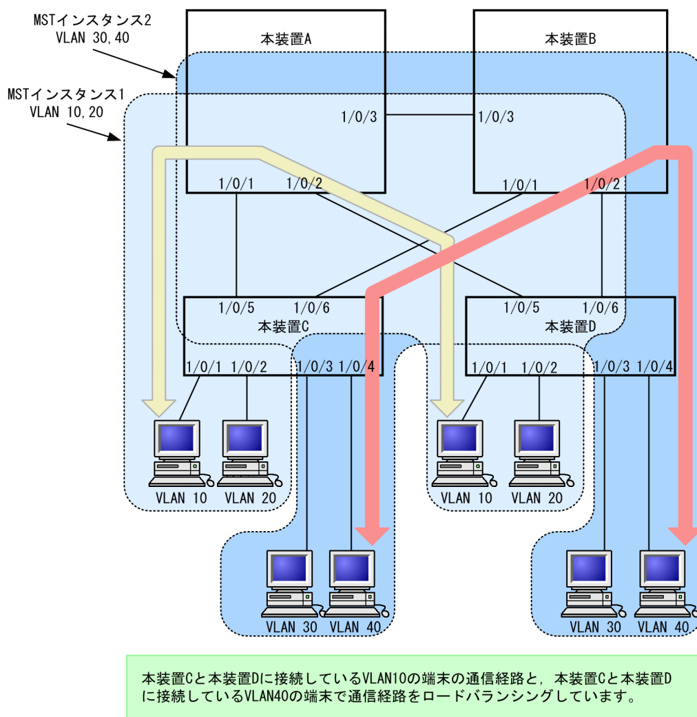
図 25-13 マルチプルスパニングツリーのロードバランシング構成
