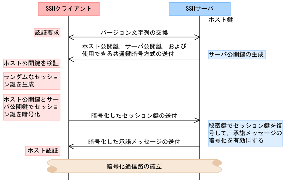
図 11-9 暗号化通信路の確立までの流れ (SSHv1)
