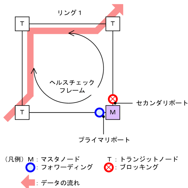
図 26-9 リング正常時の動作
