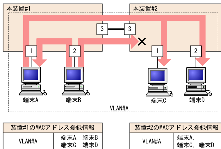
図 23-9 装置間を MAC ポートで接続した場合
