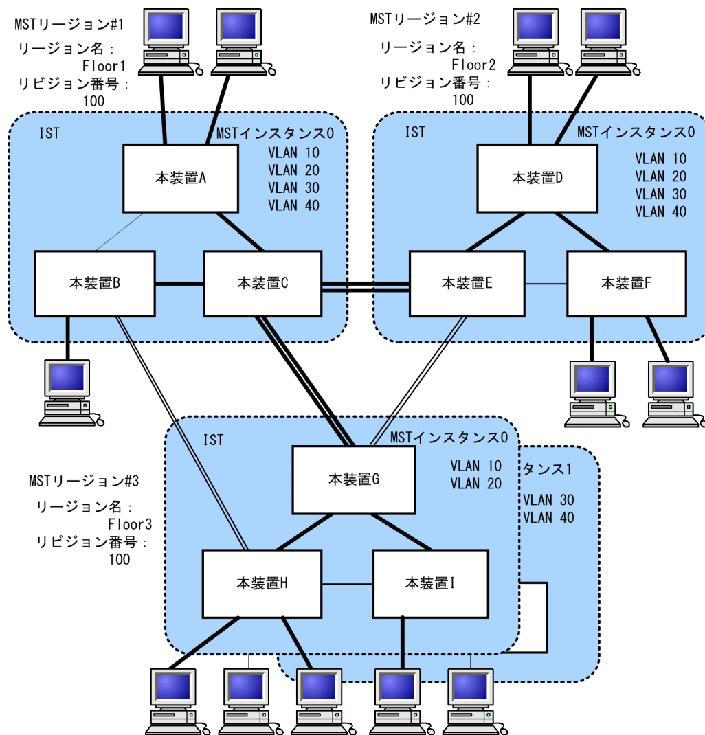
図 25-12 マルチプルスパニングツリー概要
