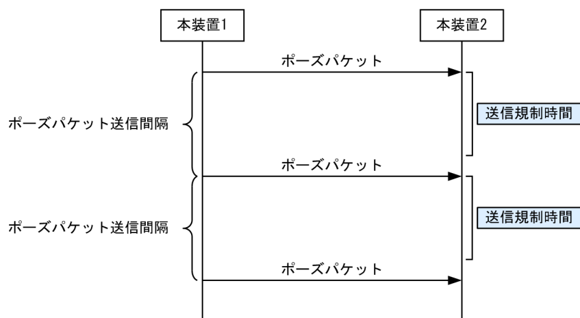
図 19-4 ルーズモードでの動作シーケンス
