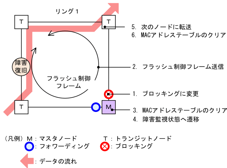
図 26-11 障害復旧時の動作
