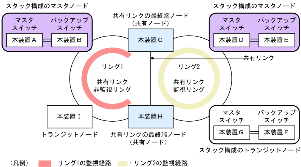
図 26-24 スタック構成のノードを含む共有リンクありのマルチリング構成
