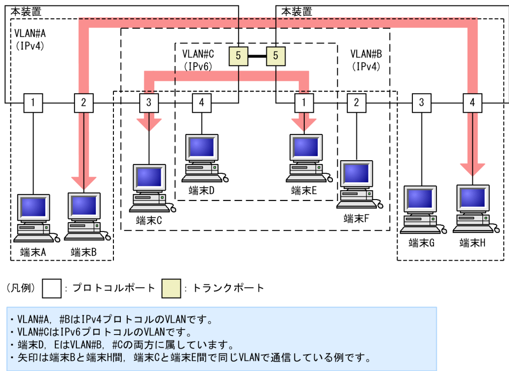
図 23-5 プロトコル VLAN の構成例
