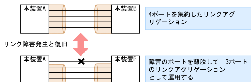
図 20-1 リンクアグリゲーションの構成例
