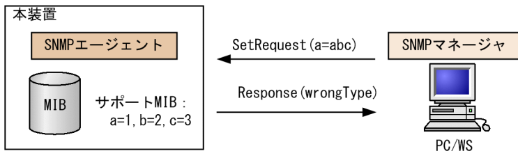
図 18-22 設定値のタイプが正しくない場合の SetRequest オペレーション例
