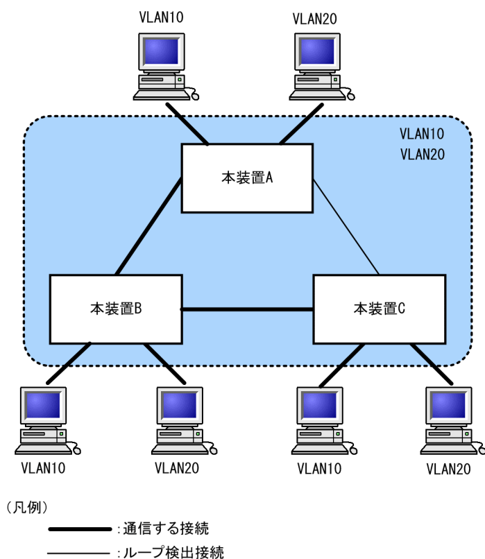
図 25-9 シングルスパニングツリーによるネットワーク構成
