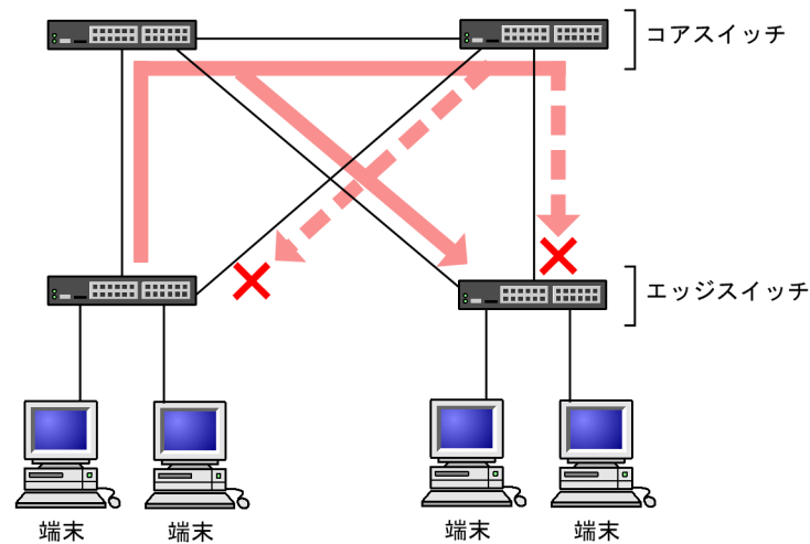
図 25-1 スパニングツリーを適用したネットワークの概要
