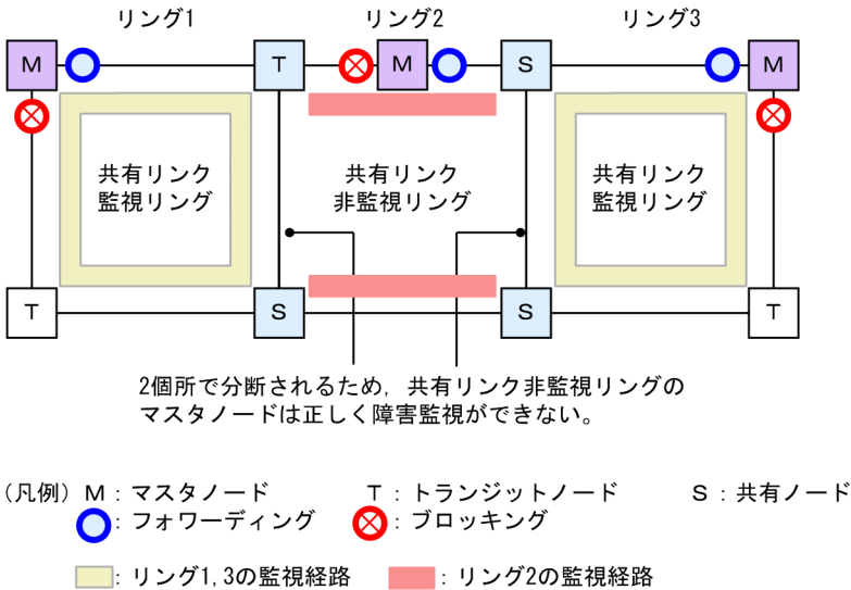
図 26-43 共有リンク監視リングが複数ある構成
