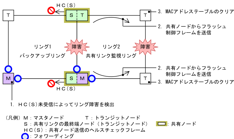
図 26-35 バックアップリングへの切り替え動作
