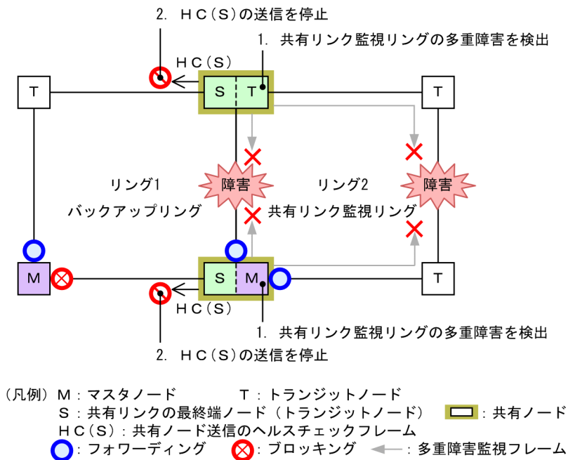
図 26-34 多重障害発生時の動作
