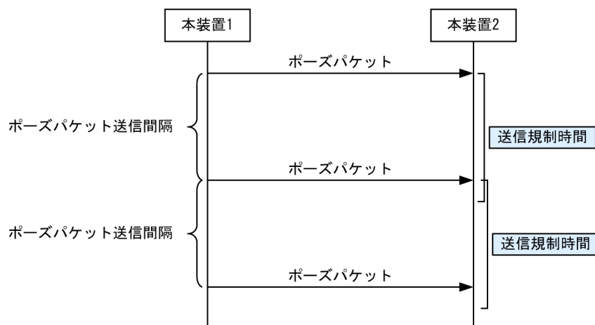
図 19-3 デフォルトでの動作シーケンス
