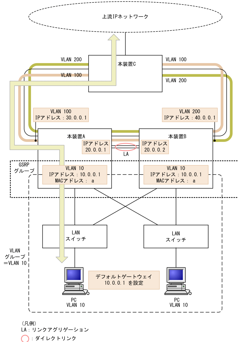
図 28-12 レイヤ 3 冗長切替機能（通常運用時）
