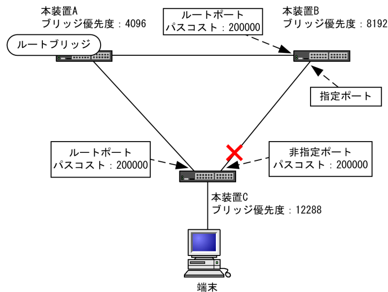
図 25-4 スパニングツリーのトポロジー設計
