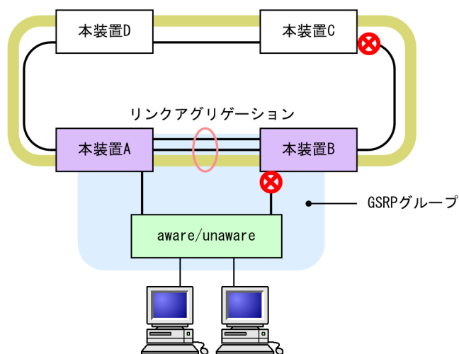
図 28-9 Ring Protocol と GSRP の併用例（ダイレクトリンクをリングネットワークで使用する場合）
