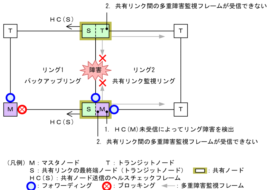
図 26-33 共有リンク障害時の動作
