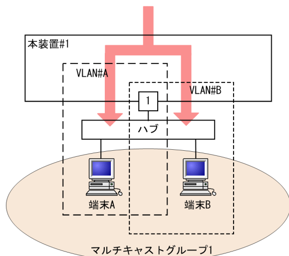
図 23-10 VLAN 混在時のマルチキャスト
