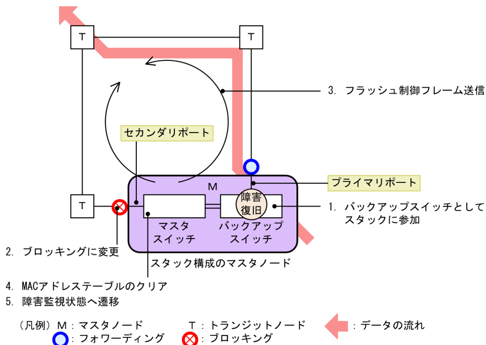
図 26-27 マスタノードでのメンバスイッチ障害復旧時の動作
