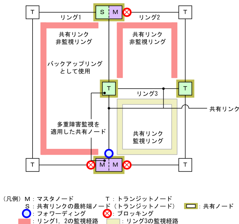
図 26-47 共有リンク内の共有ノードで多重障害を監視する構成
