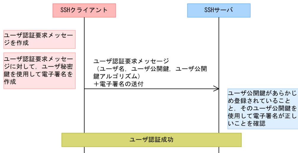
図 11-12 公開鍵暗号方式によるユーザ認証の流れ (SSHv2)
