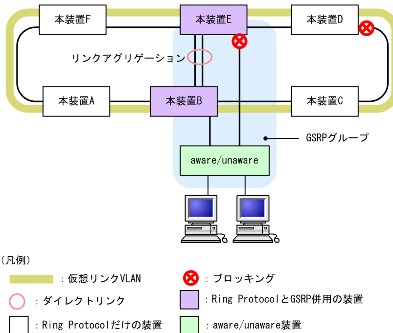
図 28-10 Ring Protocol と GSRP の併用例 (ダイレクトリンクをリングネットワークで使用しない場合)
