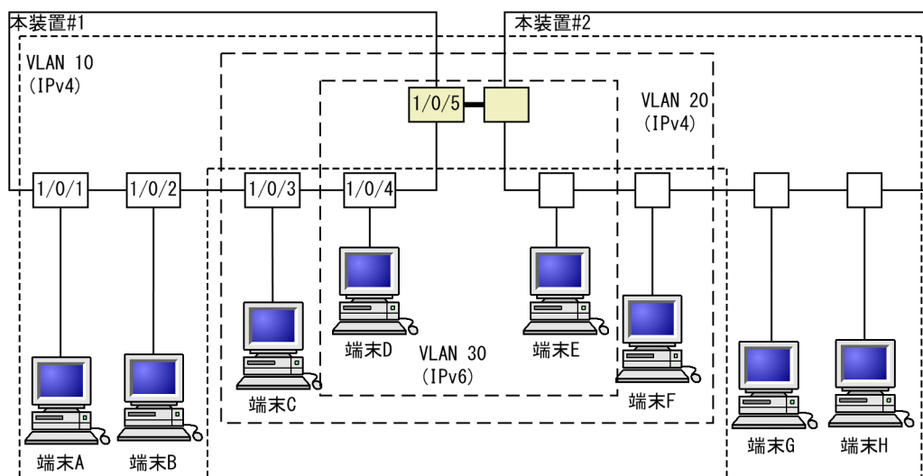
図 23-7 プロトコル VLAN の設定例
