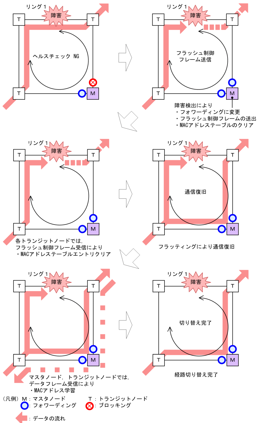
図 26-8 Ring Protocol の経路切り替え動作概要
