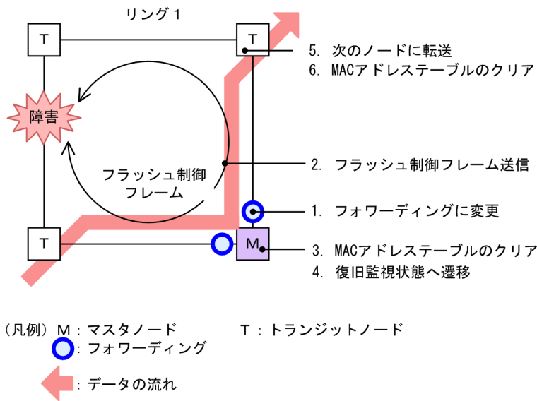
図 26-10 リング障害時の動作
