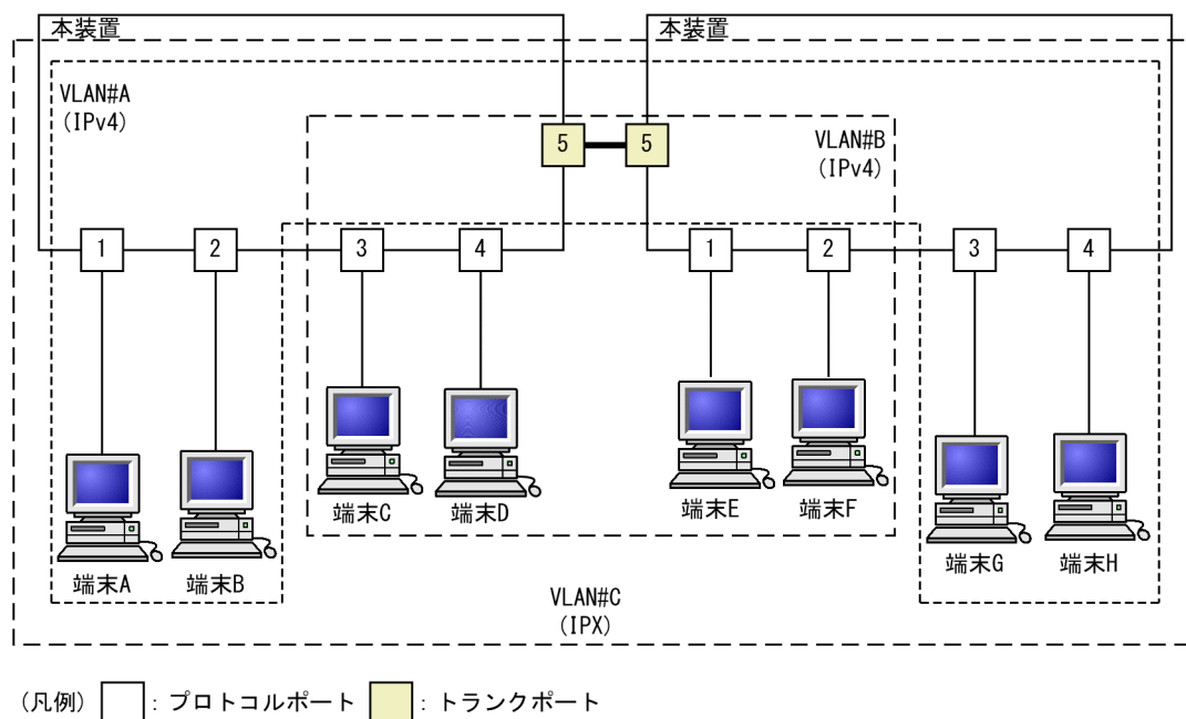
図 23-6 プロトコルポートでネイティブ VLAN を使用する構成例
