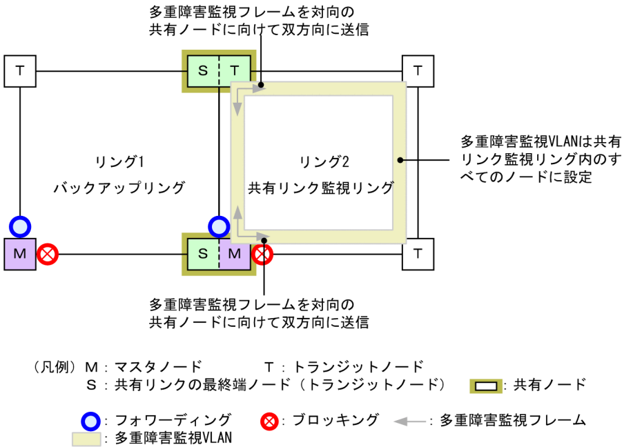
図 26-32 多重障害監視の動作概要
