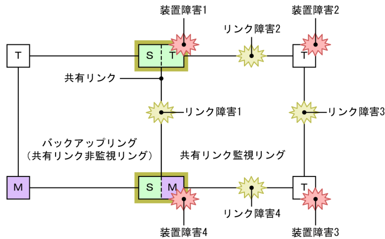
図 26-30 共有リンク監視リングでの障害発生例
