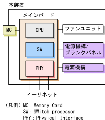
図 2-2 ハードウェアの構成
