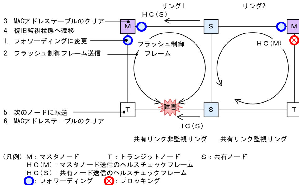
図 26-18 共有リンク非監視リングにおける共有リンク以外のリング障害時の動作
