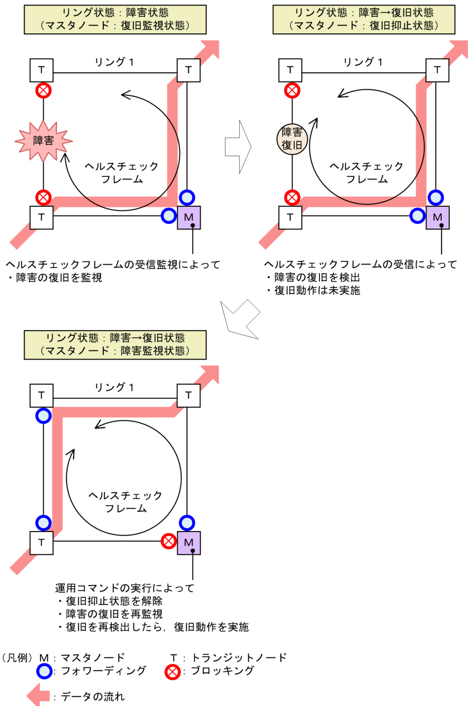
図 26-12 運用コマンドの実行によって経路切り戻し抑止を解除した場合の動作
