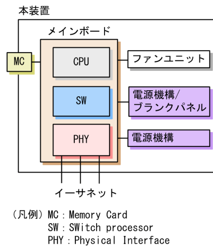
図 2-1 ハードウェアの構成
