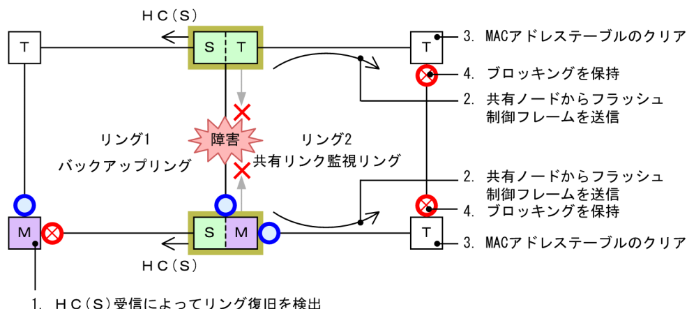
図 26-37 バックアップリングからの切り戻し動作
