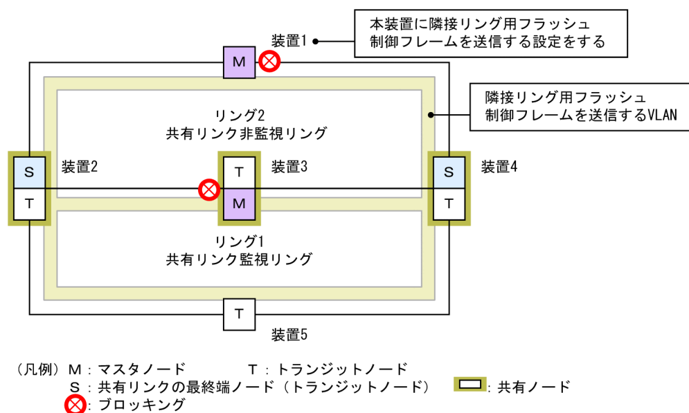
図 27-5 マスタノードの両リングポートが共有リンクとなる構成
