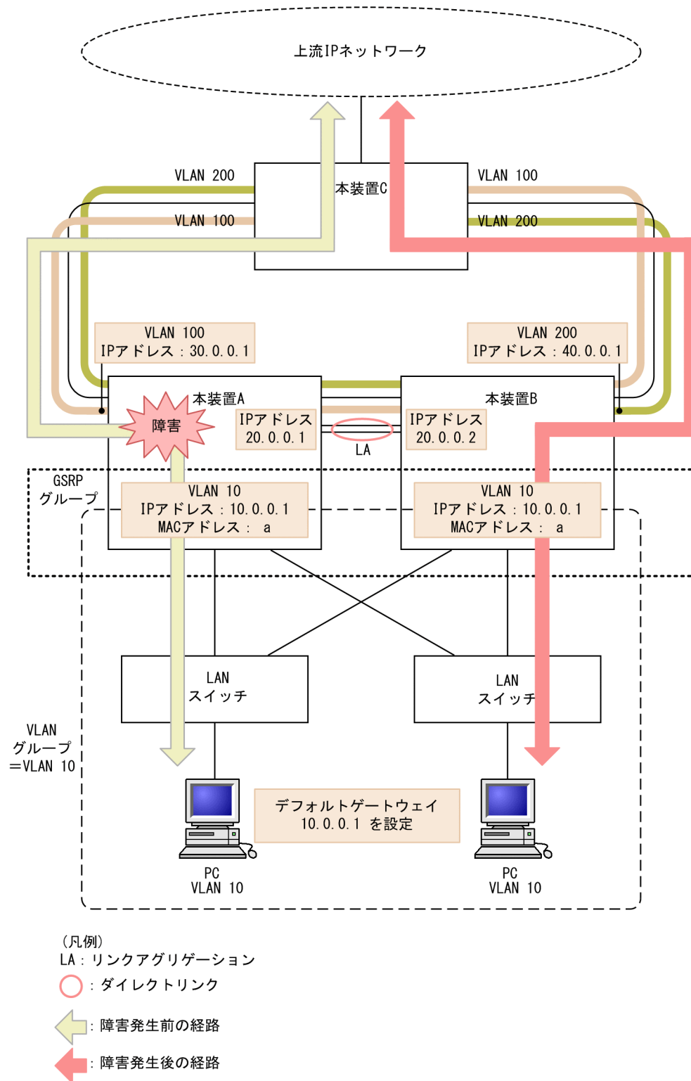
図 28-13 レイヤ 3 冗長切替機能（障害発生時）
