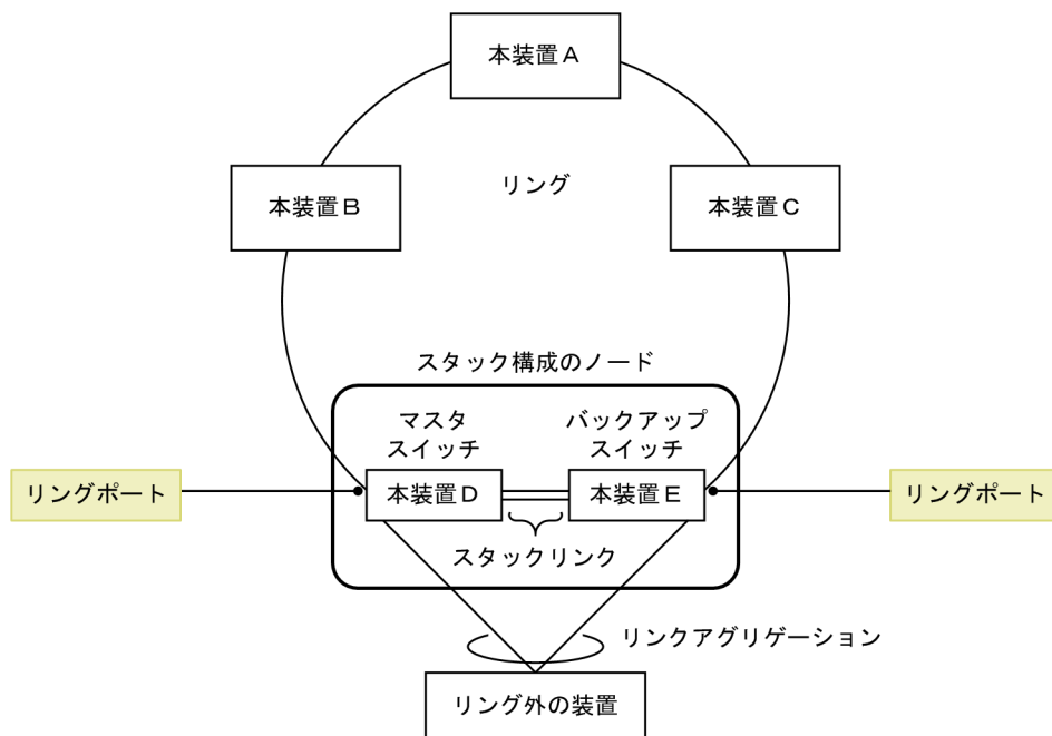
図 26-7 スタック構成のノードを含むリング構成
