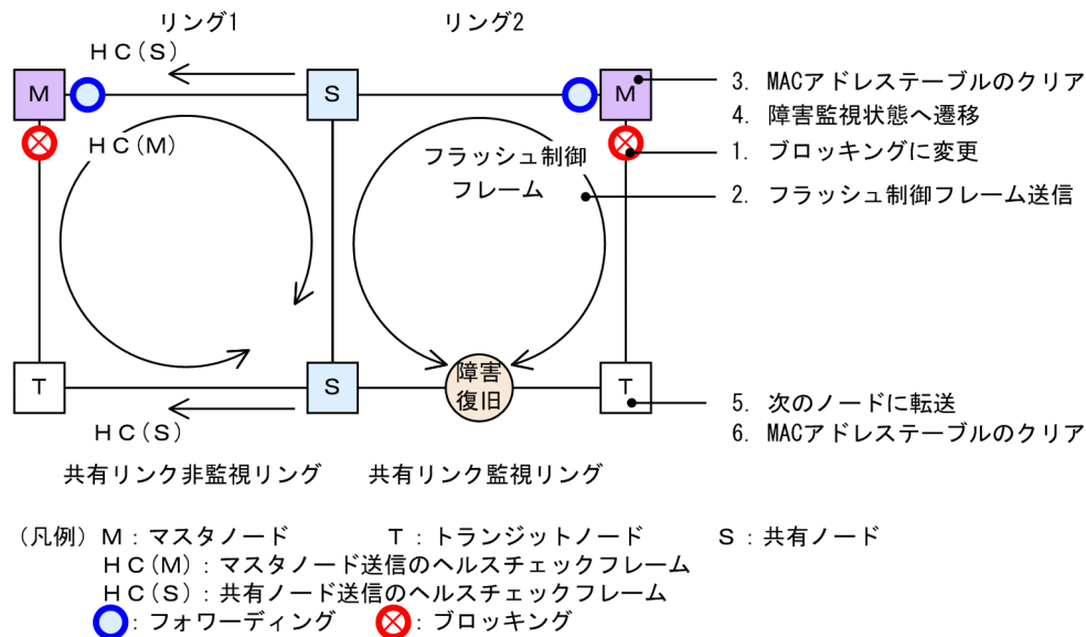
図 26-21 共有リンク監視リングでの共有リンク以外のリング障害復旧時の動作
