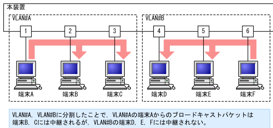
図 21-1 VLAN の概要
