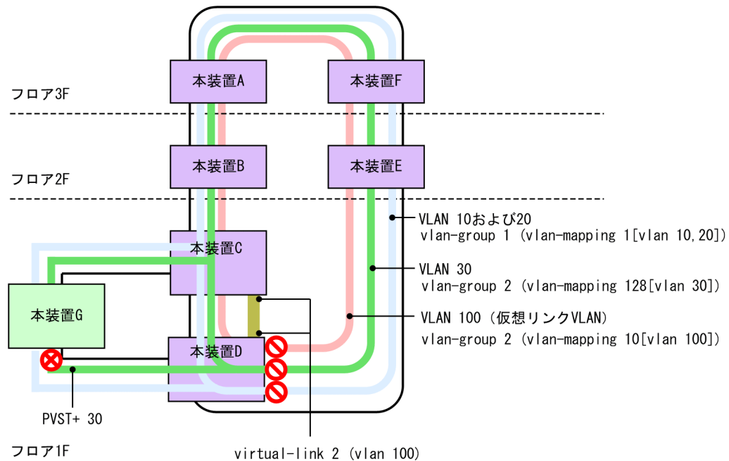
図 28-4 PVST+と Ring Protocol の共存構成
