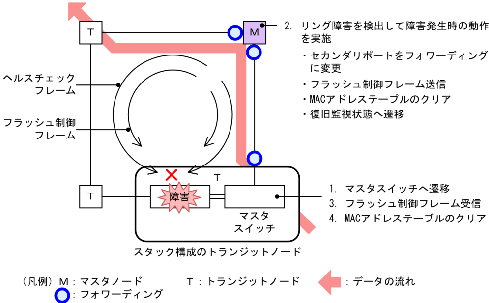
図 26-28 トランジットノードでのメンバスイッチ障害発生時の動作
