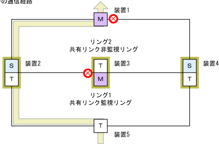
図 26-48 マスタノードの両リングポートが共有リンクとなる構成例
