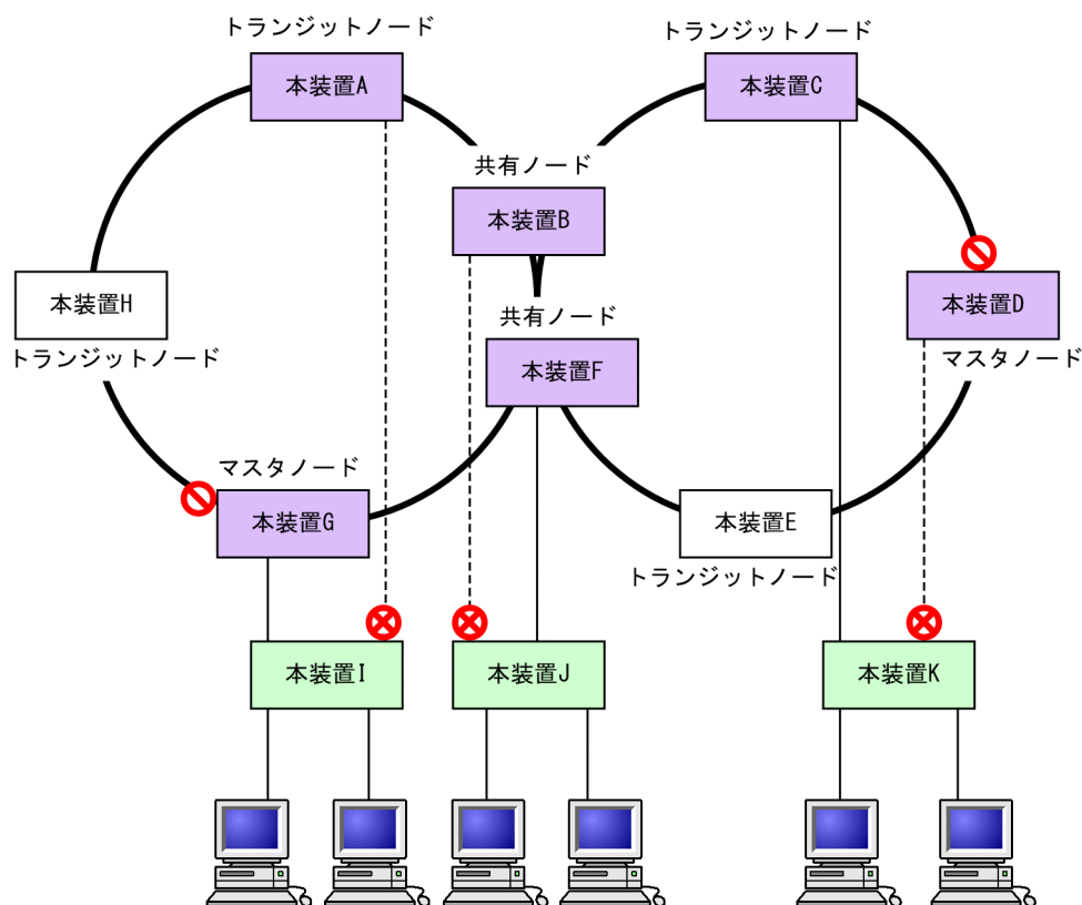
図 28-2 Ring Protocol とスパニングツリーの併用例 (マルチリング構成)
