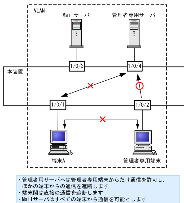
図 24-6 ポート間中継遮断機能の設定例
