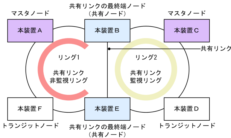
図 26-6 共有リンクありのマルチリング構成
