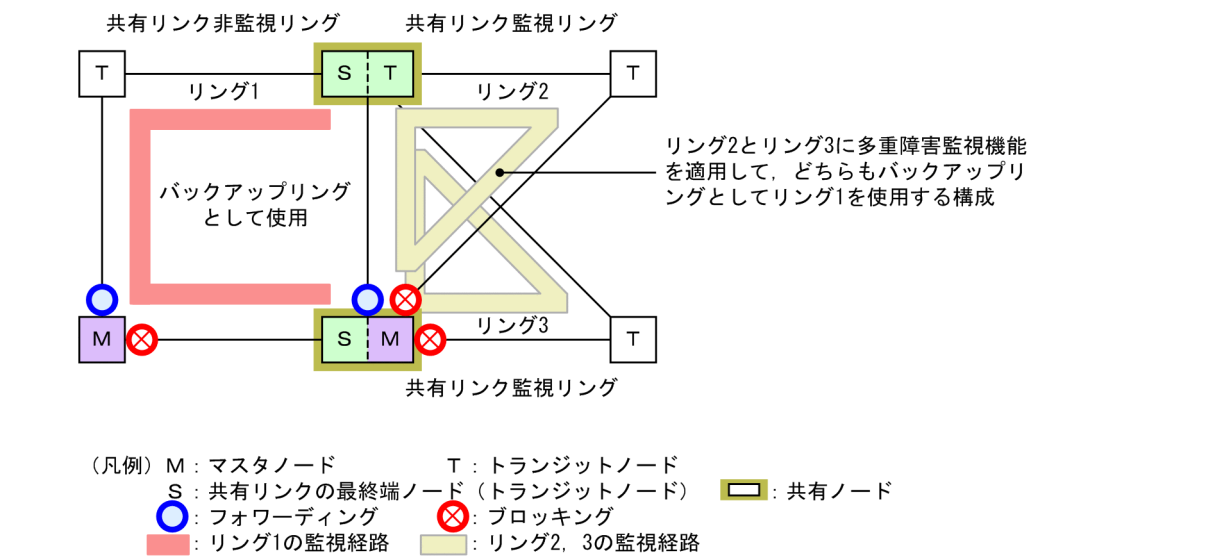
図 26-46 複数の共有リンク監視リングが同じバックアップリングを使用する構成
