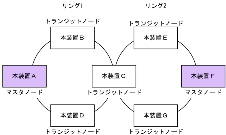
図 26-5 マルチリング構成
