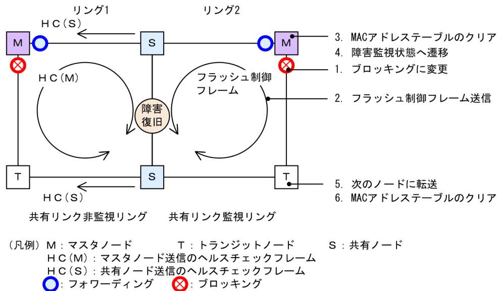
図 26-17 共有リンク復旧時の動作
