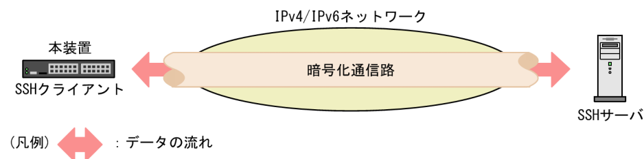
図 11-7 本装置の SSH クライアントからリモートにある SSH サーバへ接続する例
