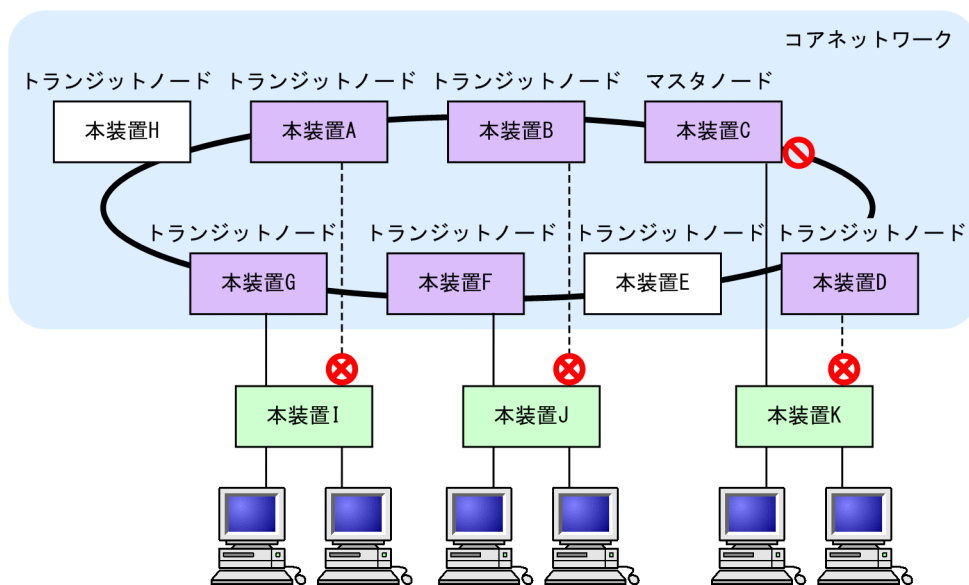
図 28-1 Ring Protocol とスパニングツリーの併用例（シングルリング構成）
