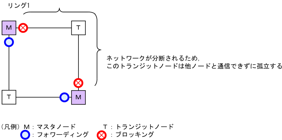
図 26-42 同一リング内に複数のマスタノードを設定
