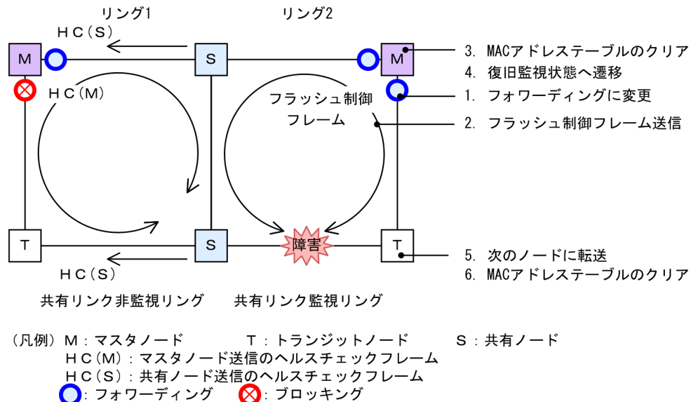
図 26-20 共有リンク監視リングでの共有リンク以外のリング障害時の動作
