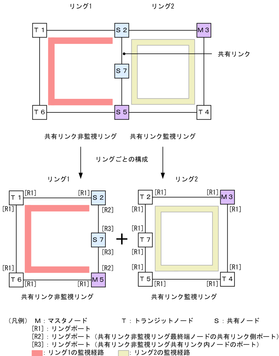
図 27-4 共有リンクありのマルチリング構成（拡張構成）
