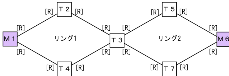
図 27-2 共有リンクなしマルチリング構成
