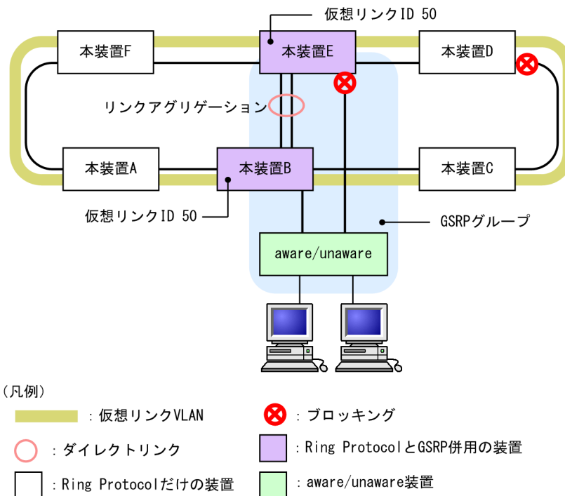
図 28-11 仮想リンク ID の設定
