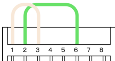
図 10-3 10BASE-T/100BASE-TX 用ループコネクタの配線仕様
