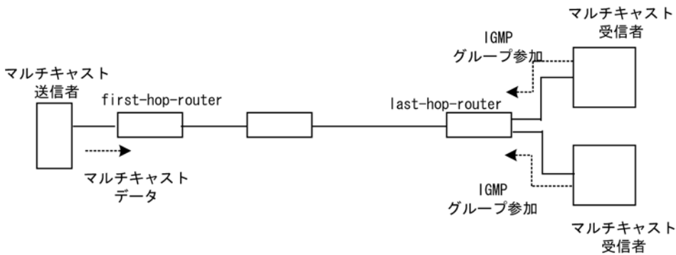
図 7-6 IPv4 PIM-SSM ネットワーク例
