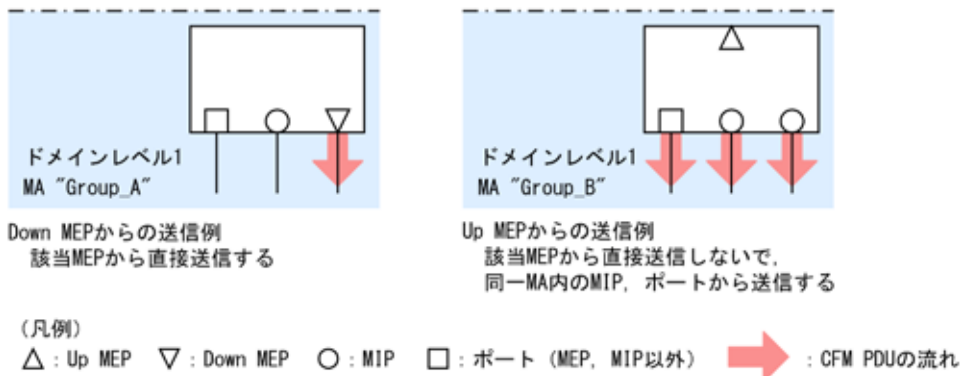
図 22-6 Down MEP, Up MEP からの送信
