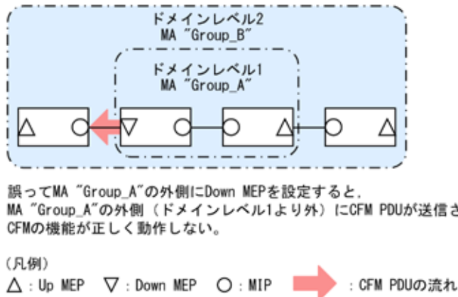
図 22-8 誤って Down MEP を設定した例
