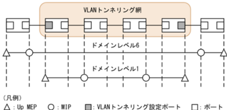
図 22-27 VLAN トネリング網内と VLAN トネリング網外で CFM を使用する例
