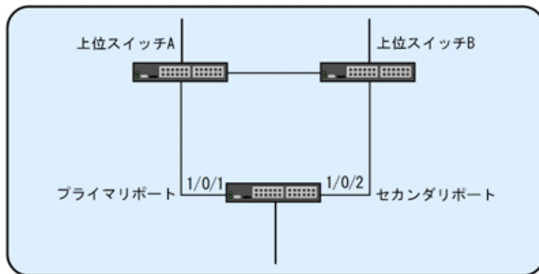
図 15-8 アップリンク・リダンダントの設定例
