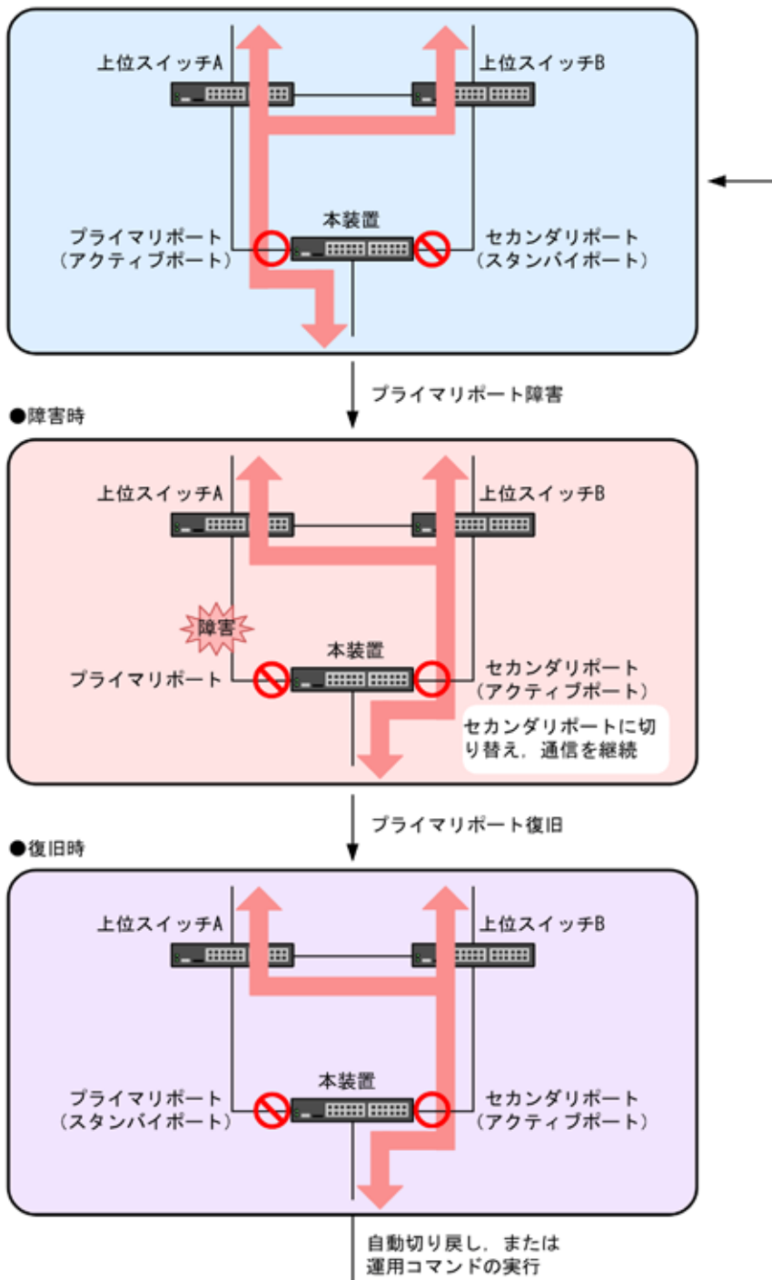
図 15-2 アップリンク・リダンダントの動作概要
