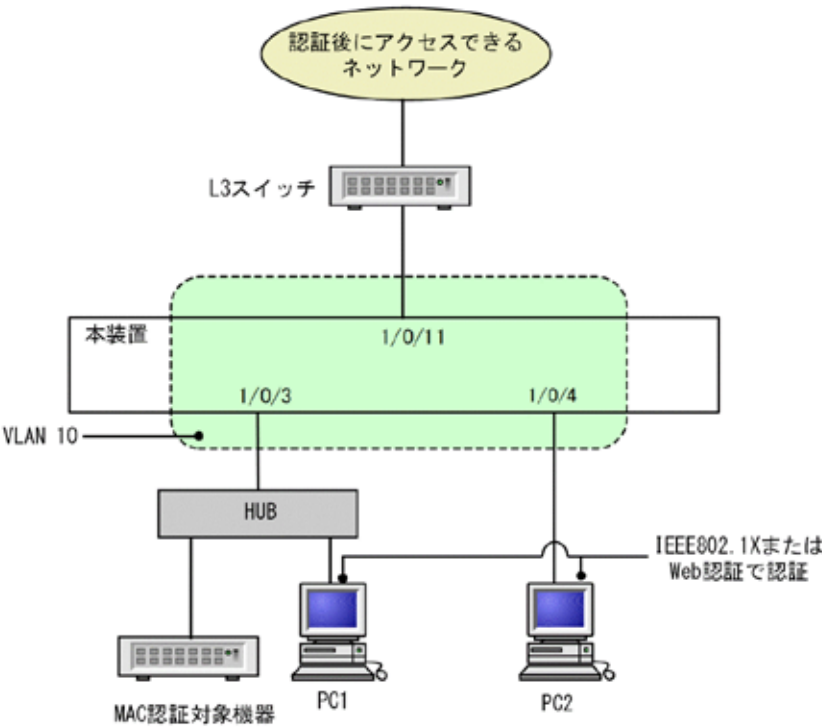
図 11-1 固定 VLAN モードのローカル認証方式の基本構成
