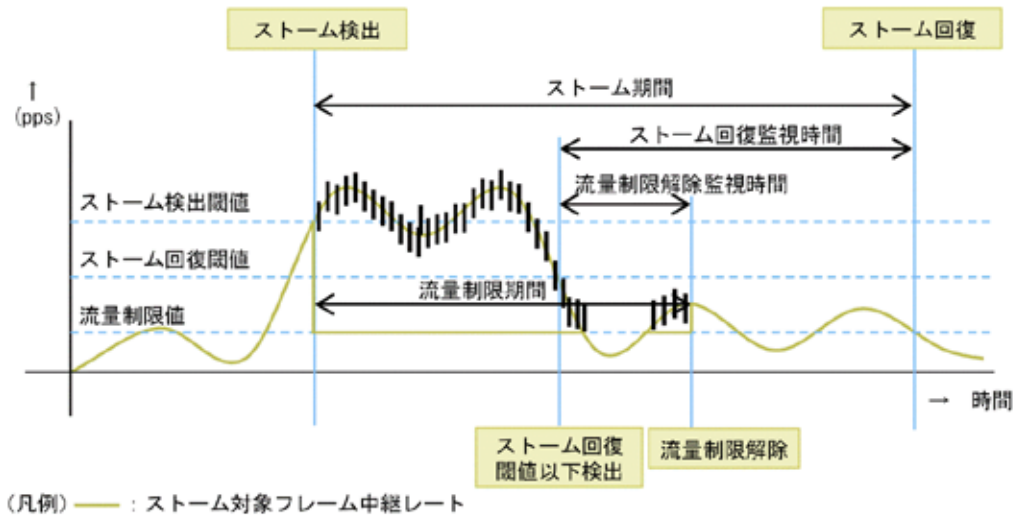
図 17-1 流量制限の動作
