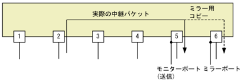
図 18-2 送信フレームのミラーリング
