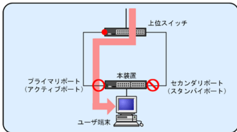
図 15-6 ポトリセット機能の有効／無効による切り替え動作の違い
