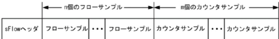
図 20-4 sFlow パケットフォーマット
