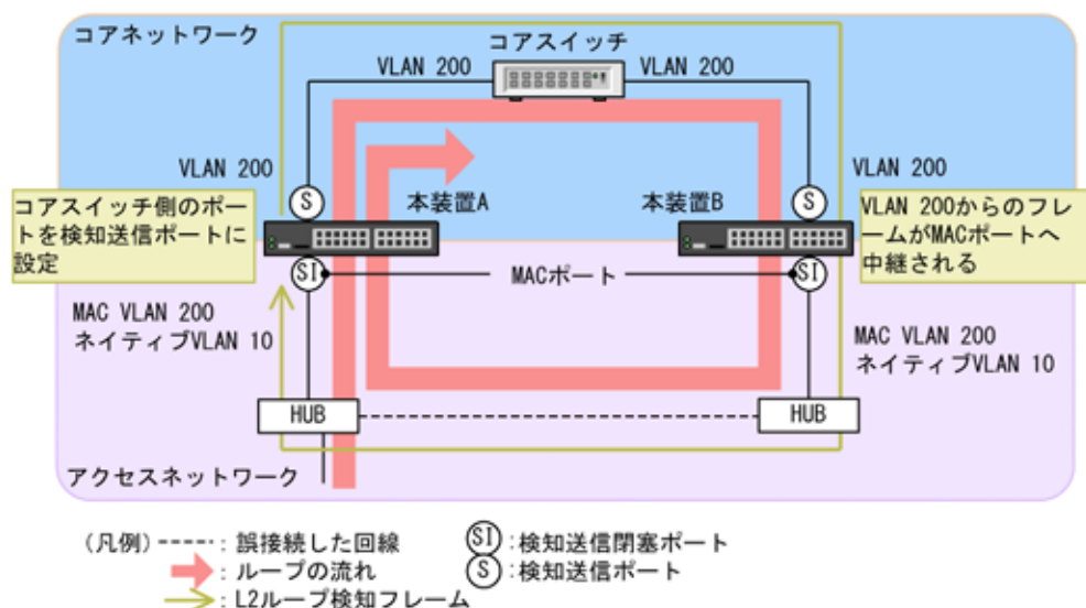
図 16-5 ループ検知可能な構成
