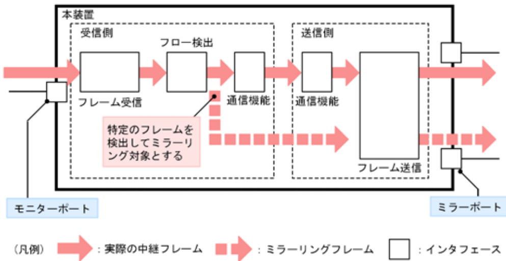
図 19-1 受信フレームのミラーリング
