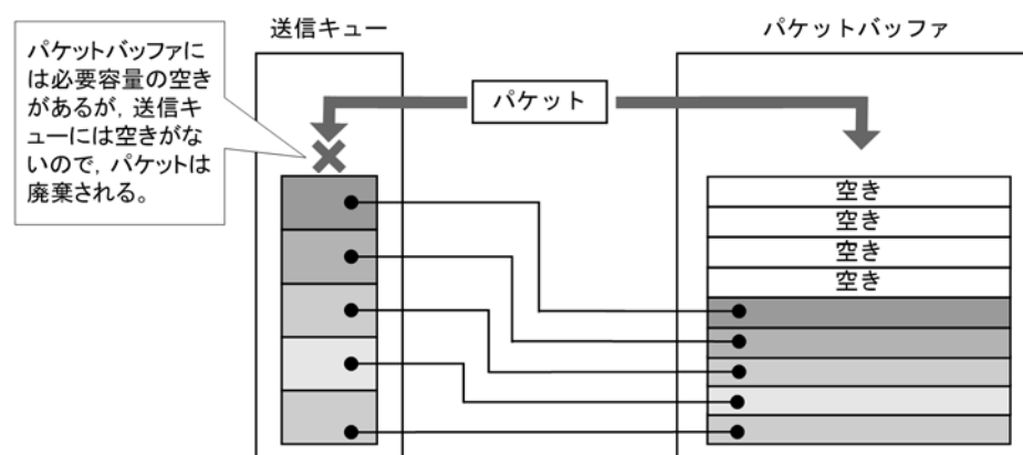
図 26-12 送信キューに空きがないためパケットが廃棄される場合
