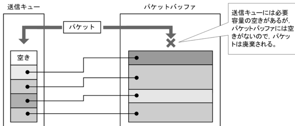
図 26-13 パケットバッファに空きがないためパケットが廃棄される場合
