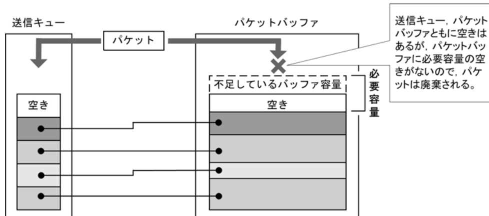
図 26-14 パケットバッファに受信パケットを格納する空きがないためパケットが廃棄される場合
