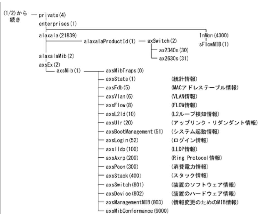
図 1-2 MIB 体系図(2/2)
