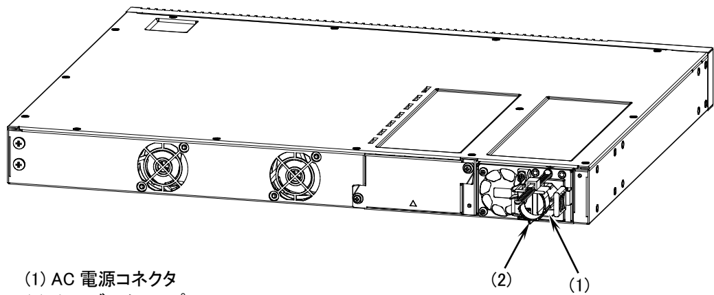
図1-14 背面外観
