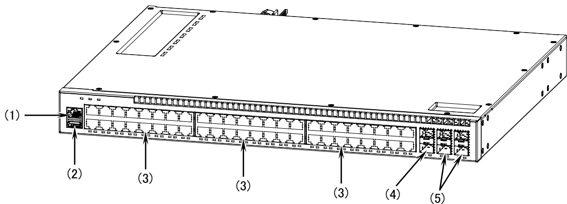
図1-9 正面外観
