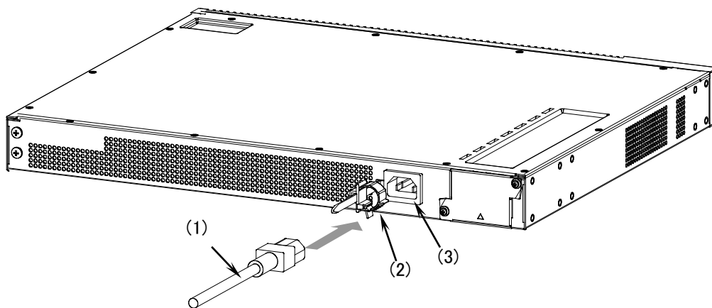
図4-16 電源の投入
