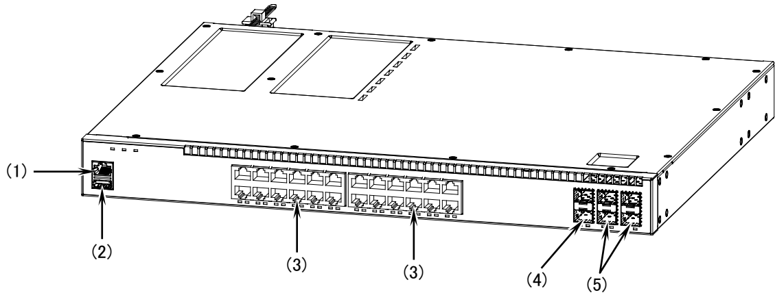
図1-13 正面外観
