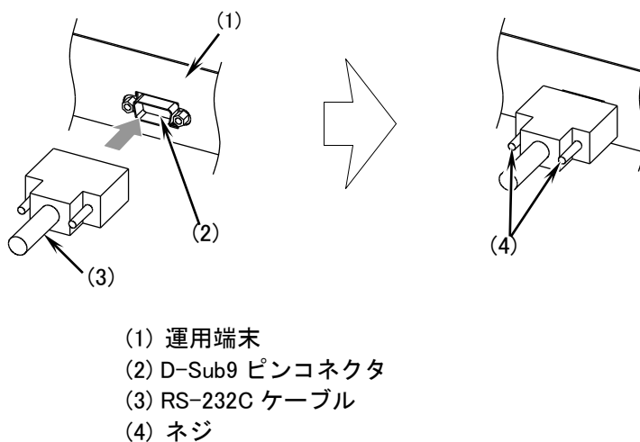
図4-12 RS-232C ケーブルの取り付け
