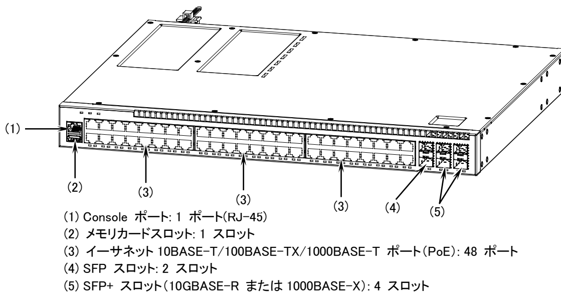
図1-17 正面外観
