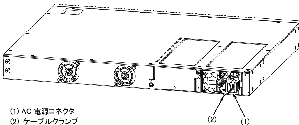
図1-22 背面外観
