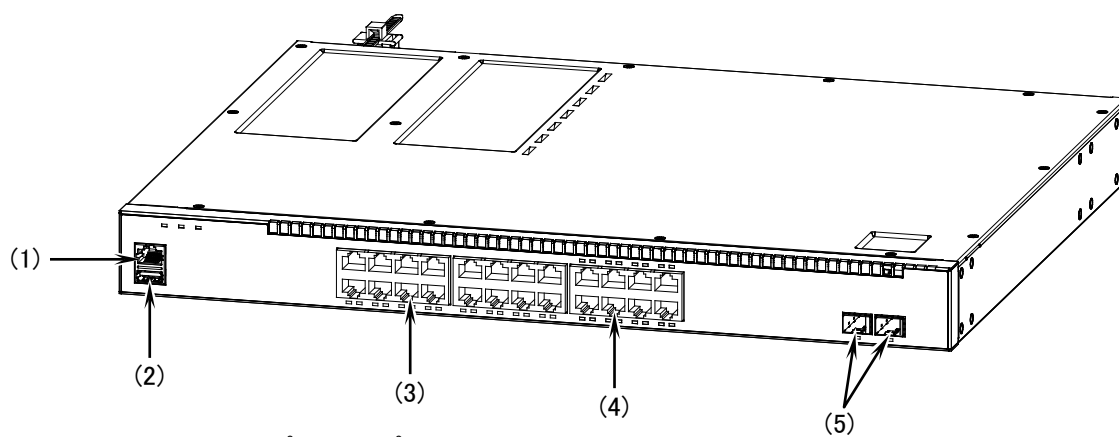
図1-21 正面外観
