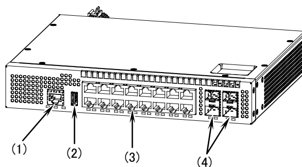
図1-1 正面外観
