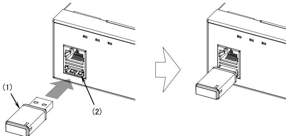
図4-9 メモリカードの取り付け
