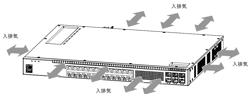
図2-6 IP8800/S2340-16T4X , IP8800/S2340-24T4X , IP8800/S2340-24TH4X , IP8800/S2340-24PH4X のエアフロー
