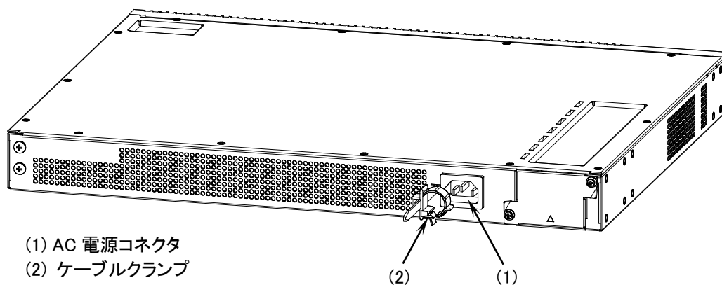
図1-6 背面外観
