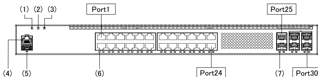
図1-7 正面パネルレイアウト
