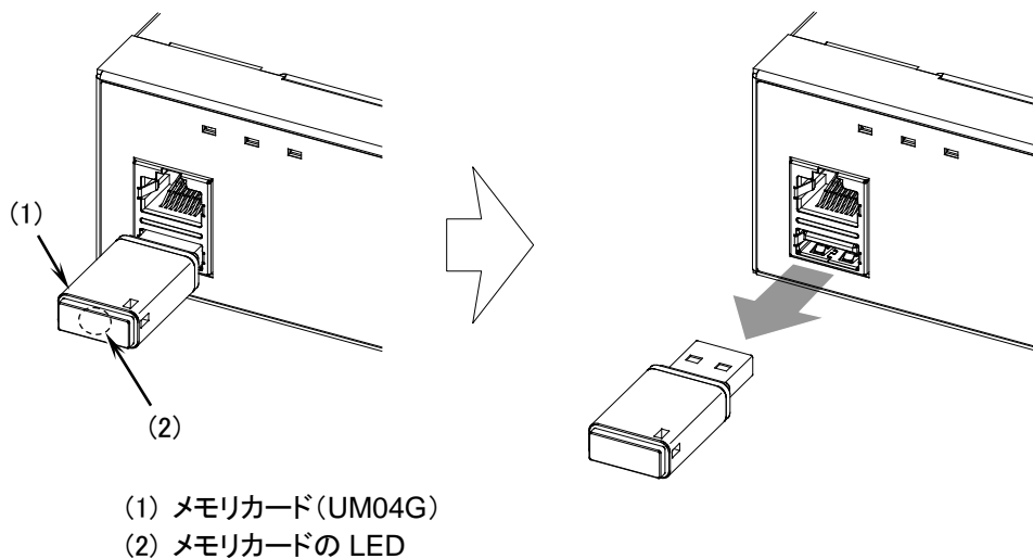
図4-10 UM04G の取り外し
