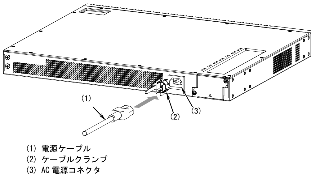
図4-7 電源ケーブルの取り付け
