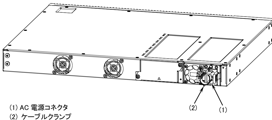
図1-18 背面外観
