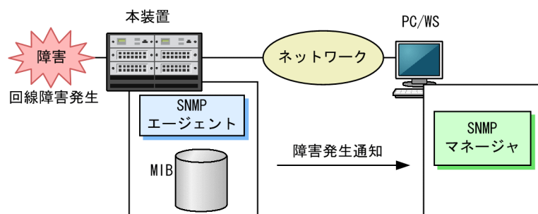
図 16-24 トラップの例
