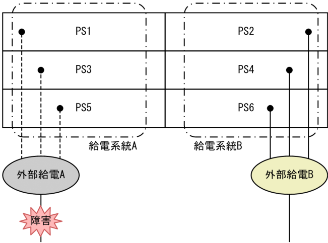
図 14-7 給電系統冗長の構成例
