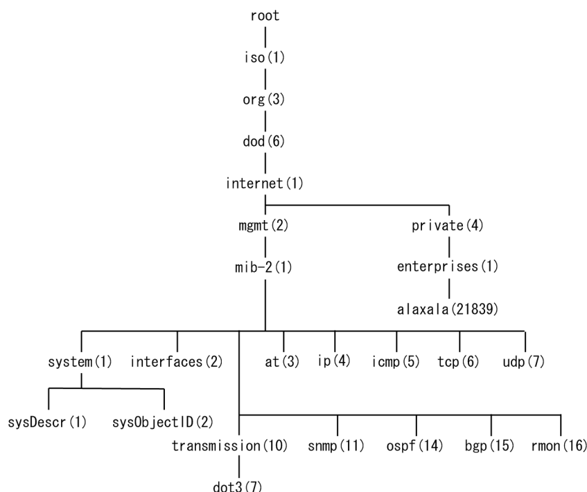
図 16-6 MIB ツリーの構造例
