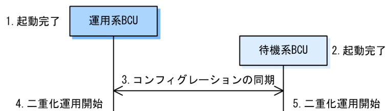
図 14-1 二重化構成での運用開始時の動作
