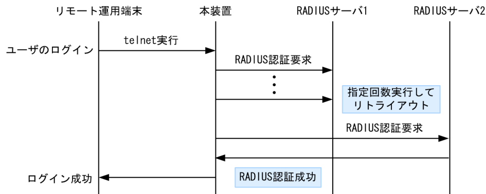
図 8-20 RADIUS サーバ選択のシーケンス
