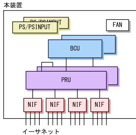
図 2-5 IP8800/R8616 および IP8800/R8632 のハードウェアの構成
