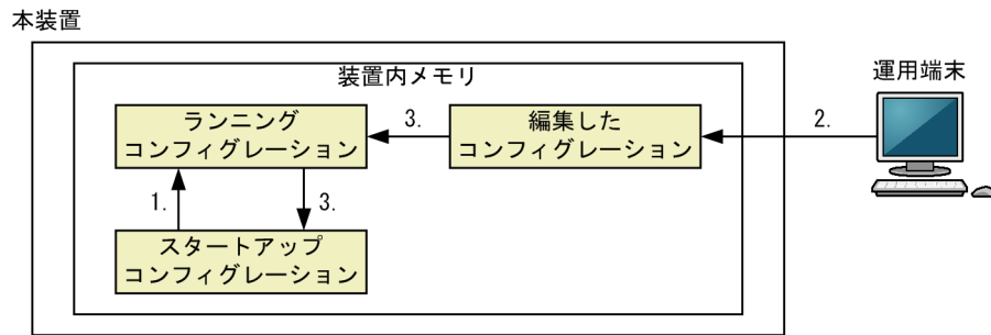
図 6-2 起動時および運用中のコンフィグレーションの概要（手動コミットモード）
