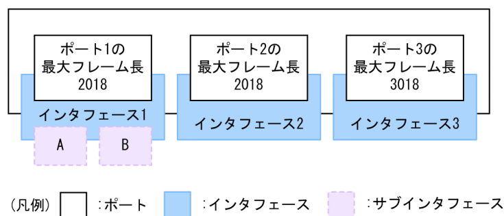
図 20-2 インタフェースとポートが 1 対 1 に対応する場合の IP MTU 値の例
