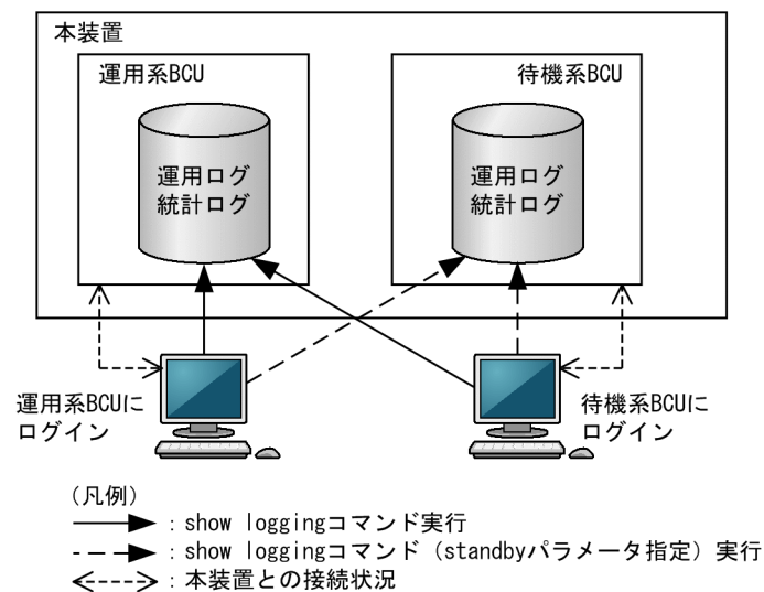
図 15-4 BCU 二重化時のログの参照
