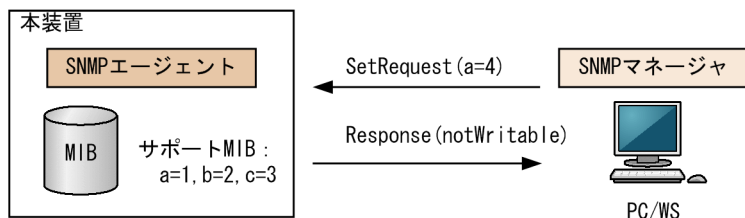
図 16-21 MIB 変数が読み出し専用の場合の SetRequest オペレーション
