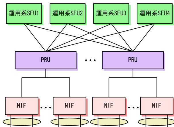
図 14-3 障害発生前の動作
