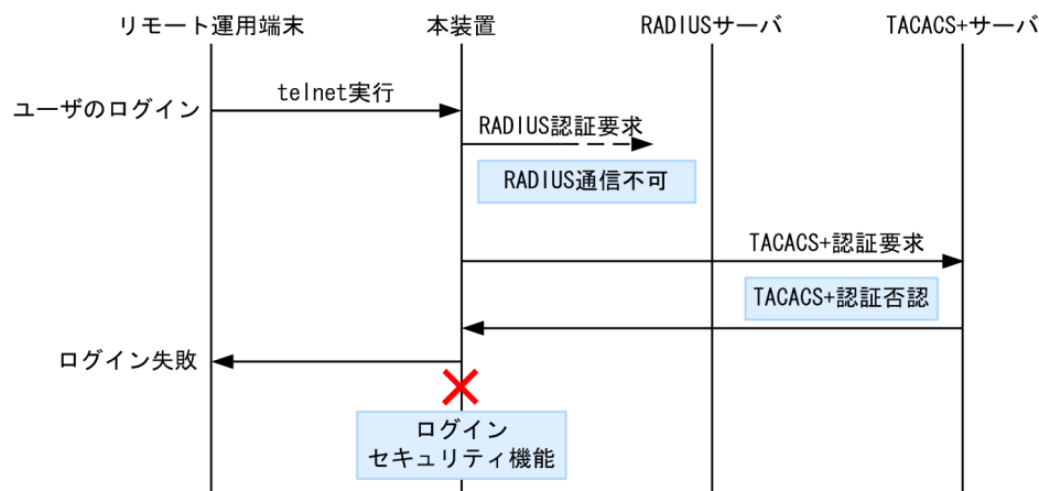
図 8-19 認証方式シーケンス (end-by-reject 設定時)
