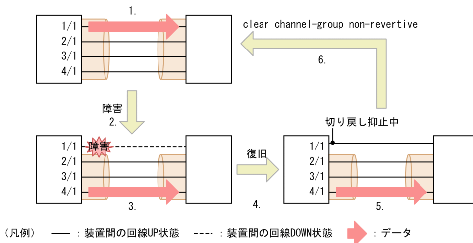
図 19-5 切り戻し抑止機能の概要
