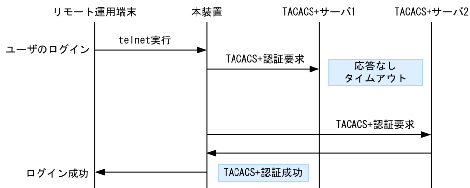
図 8-21 TACACS+サーバ選択のシーケンス
