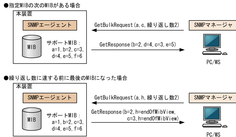
図 16-11 GetBulkRequest オペレーション
