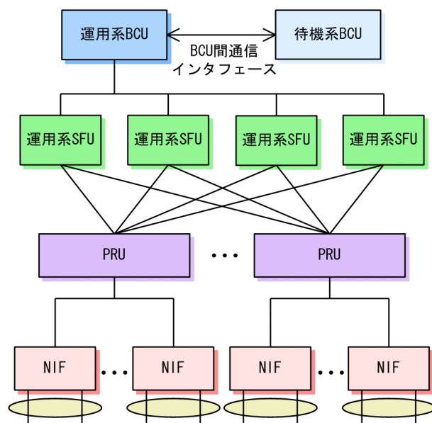
図 14-2 BCU-SFU-PRU-NIF 間の冗長構成でのインタフェース
