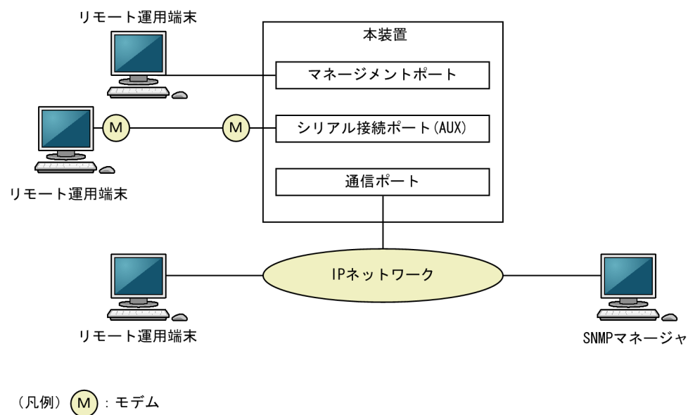
図 4-2 リモート運用端末の接続形態
