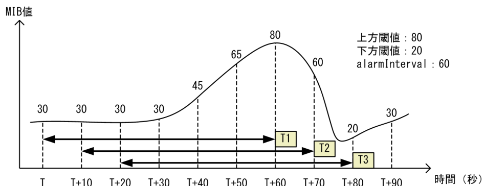
図 16-30 absolute 方式による MIB 監視例
