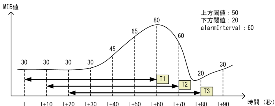
図 16-29 delta 方式による MIB 監視例
