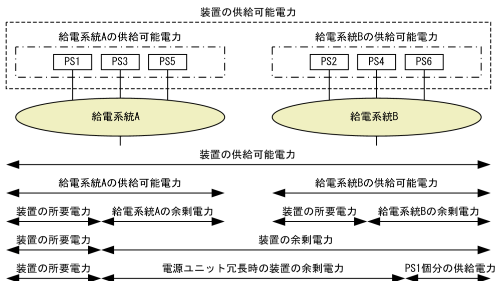
図 14-8 供給電力の管理（PS を 6 個搭載した例）
