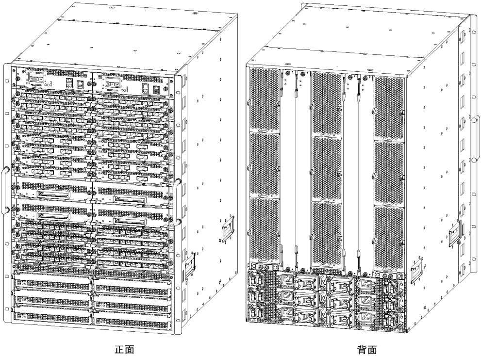
図 2-3 IP8800/R8632 モデル
