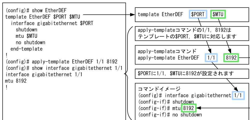
図 6-46 テンプレートパラメータの指定例
