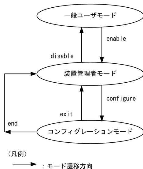
図 5-1 モード遷移の概要
