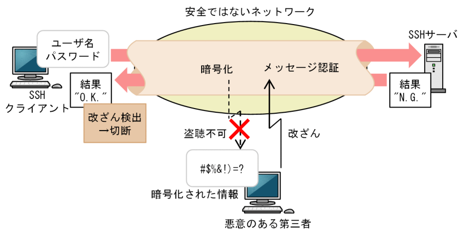
図 9-2 SSH 接続によるセキュアな運用管理
