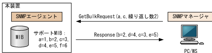
図 16-19 GetBulkRequest オペレーション
