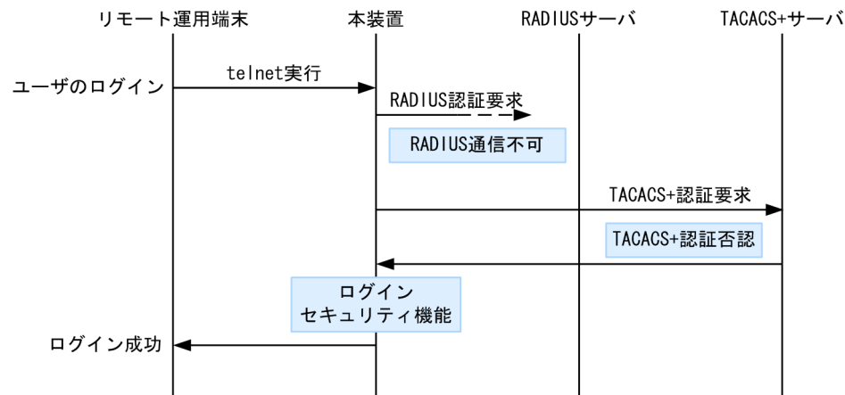
図 8-18 認証方式シーケンス（end-by-reject 未設定時）
