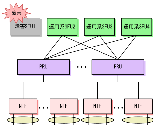
図 14-4 障害発生後の動作
