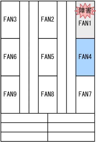
図 12-45 ファンユニット故障時の動作例（IP8800/R8632 で FAN1 のファンユニットが故障した場合）
