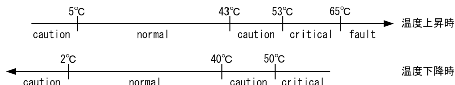
図 12-44 運用環境レベルと温度値
