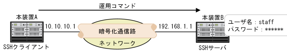
図 9-18 本装置 A から本装置 B 上でコマンドを実行する構成例
