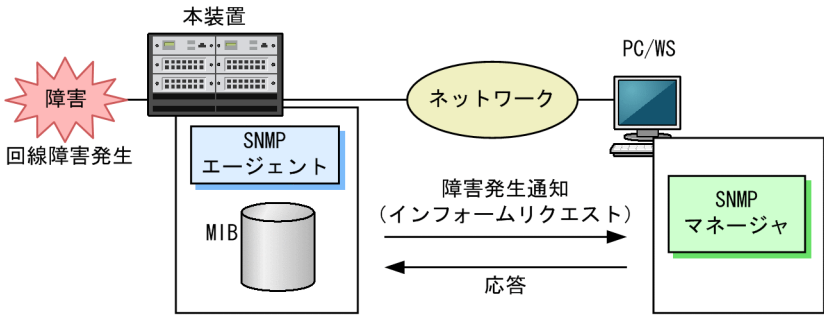
図 16-27 インフォームの例
