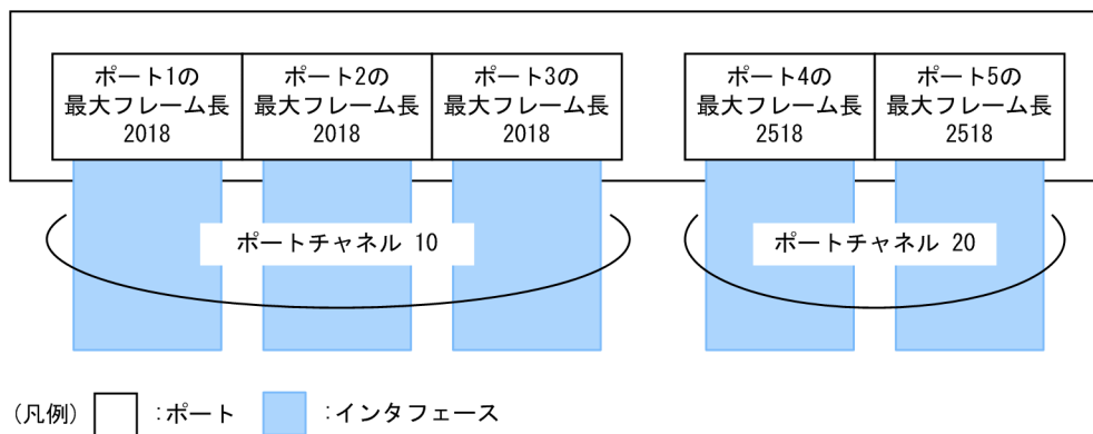
図 20-3 ポートチャネルインタフェースの IP MTU 値の例
