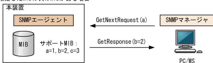
図 16-9 GetNextRequest オペレーション
