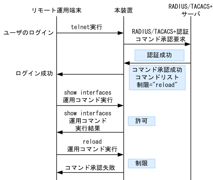
図 8-23 RADIUS/TACACS+サーバによるコマンド承認例
