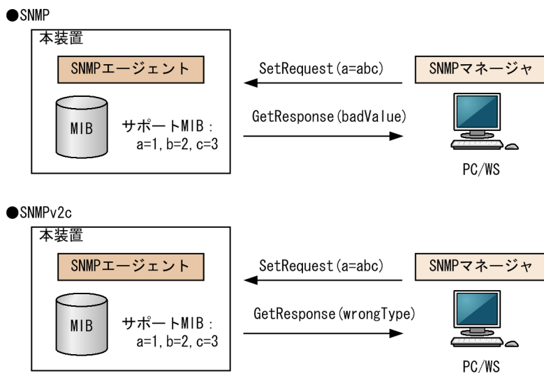
図 16-14 設定値のタイプが正しくない場合の SetRequest オペレーション例
