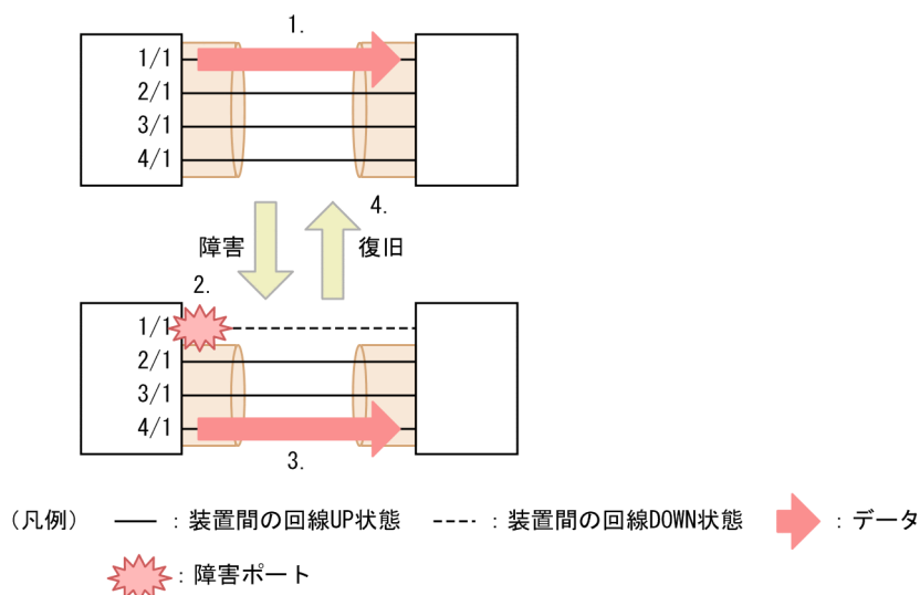
図 19-1 リンクアグリゲーションの構成例
