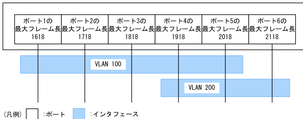
図 20-4 VLAN インタフェースの IP MTU 値の例
