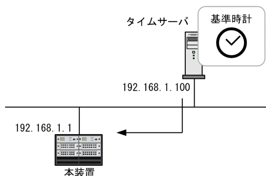
図 10-3 NTP 構成図（タイムサーバへの時刻の同期）
