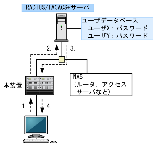
図 8-17 RADIUS/TACACS+認証の流れ
