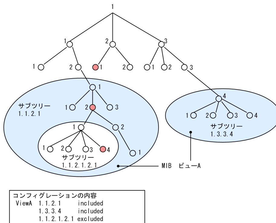
図 16-5 MIB ビューの例
