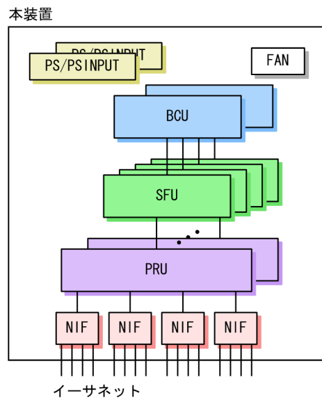
図 2-5 IP8800/R8616 および IP8800/R8632 のハードウェアの構成
