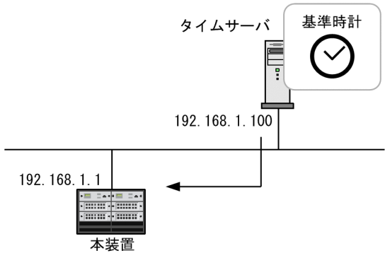
図 10-5 SNTP 構成図（タイムサーバへの時刻の同期）
