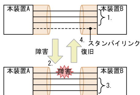
図 19-4 スタンバイリンク機能の構成例
