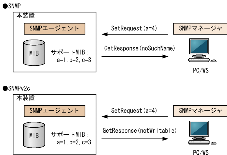
図 16-13 MIB 変数が読み出し専用の場合の SetRequest オペレーション
