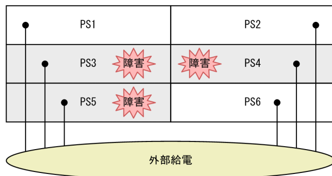
図 14-6 電源ユニット冗長の構成例
