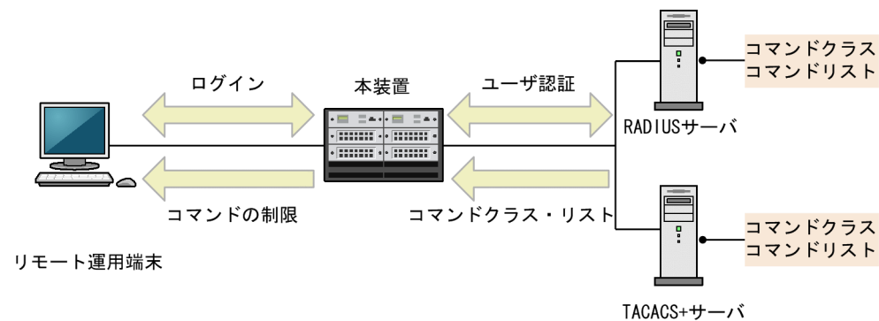
図 8-22 RADIUS/TACACS+サーバによるログイン認証、コマンド承認
