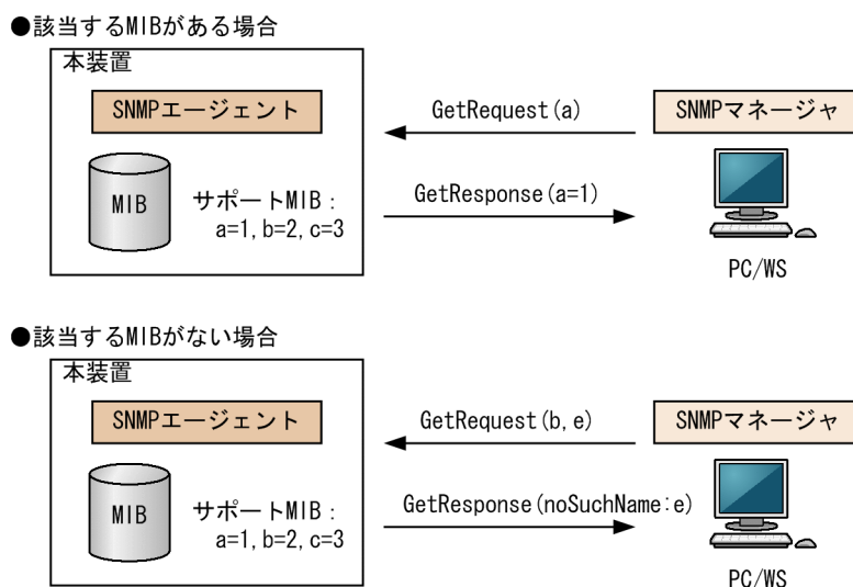
図 16-7 GetRequest オペレーション
