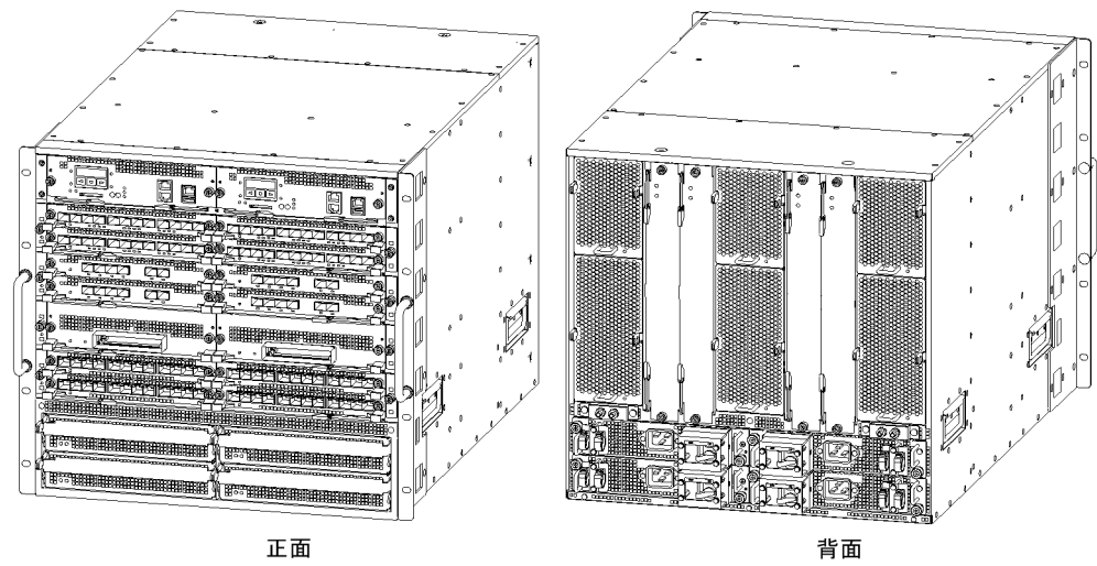
図 2-2 IP8800/R8616 モデル
