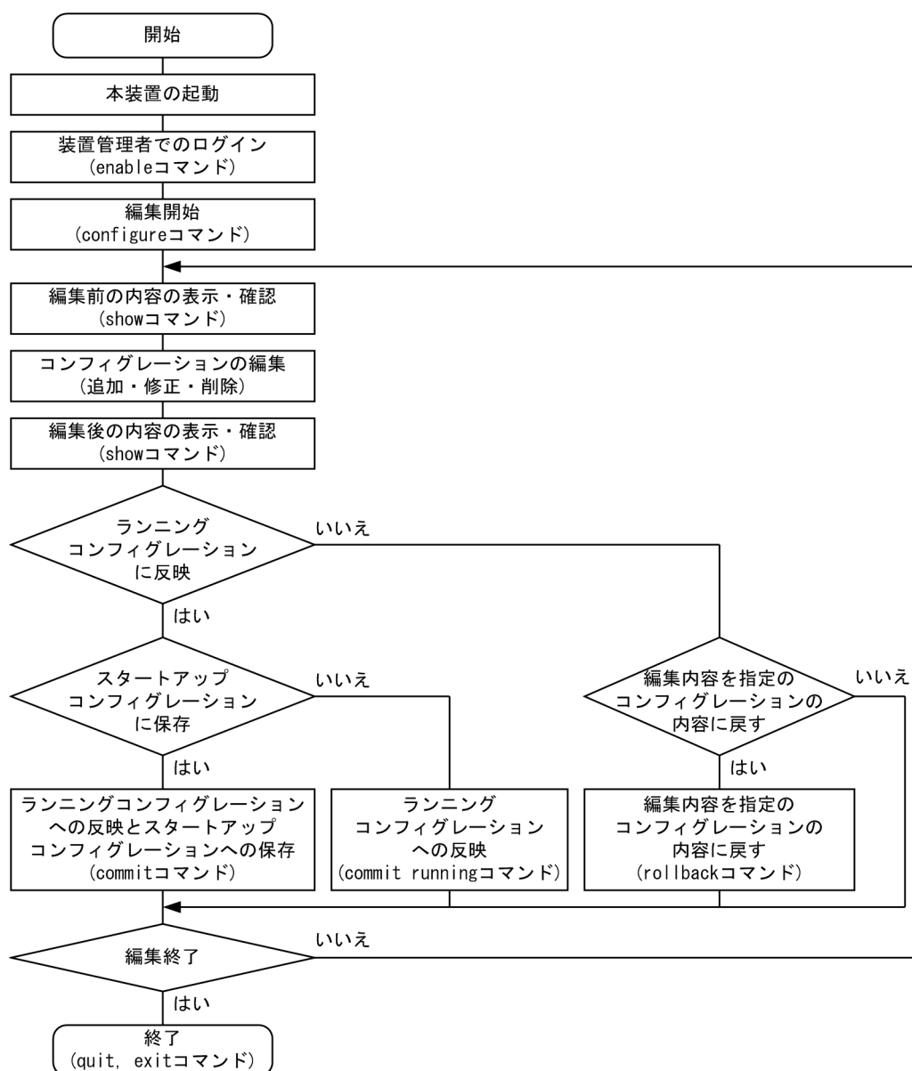
図 6-4 ランニングコンフィグレーションの編集の流れ (手動コミットモード)
