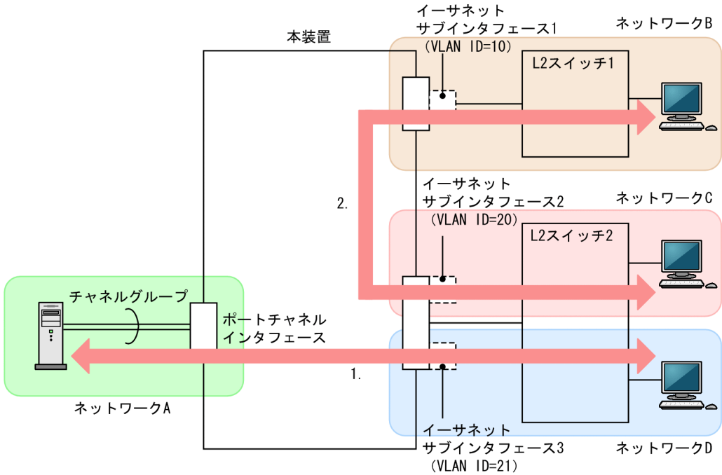
図 20-1 IP インタフェースを使用するネットワーク構成例
