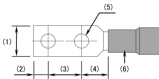
図2-8 DC 電源ケーブルの端子
