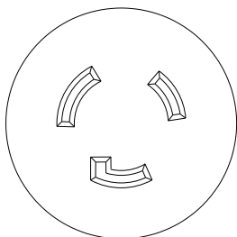
図2-6 接地形 2 極差し込みコンセント (20A 250V)
