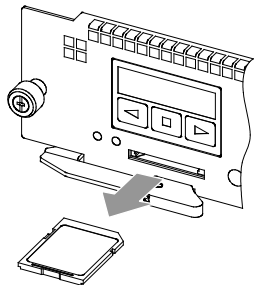
図4-43 メモ리카ードの取り出し
