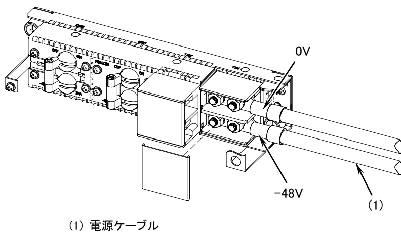
図4-36 電源ケーブルの取り付け（奥側）
