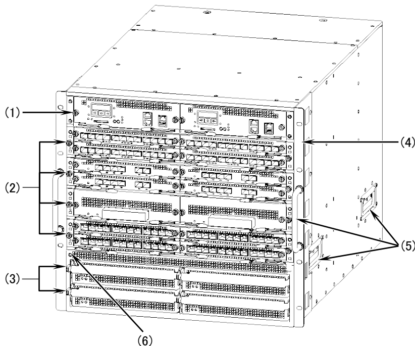
図1-5 正面外観
