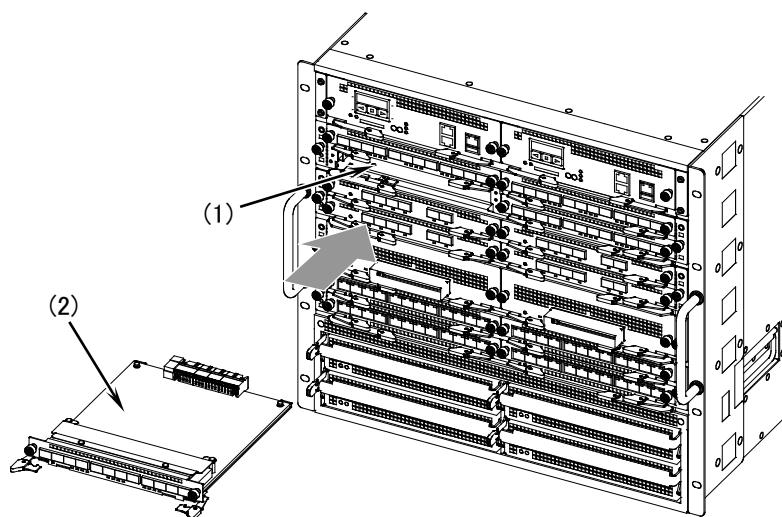
図5-60 ネットワークインタフェース機構の取り付け -1
