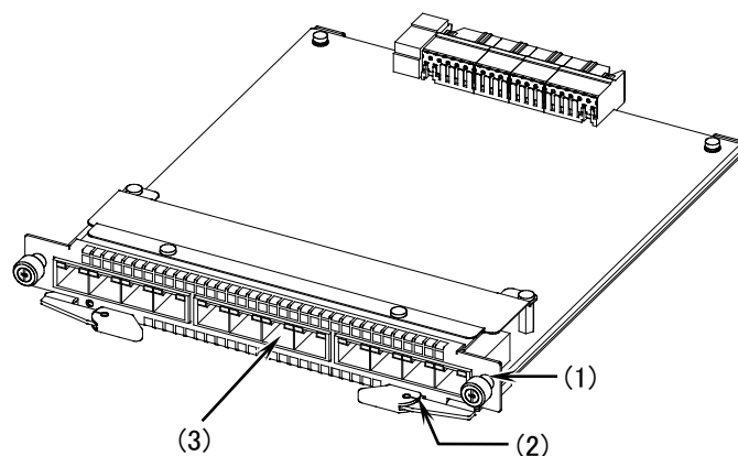
図1-30 外観
