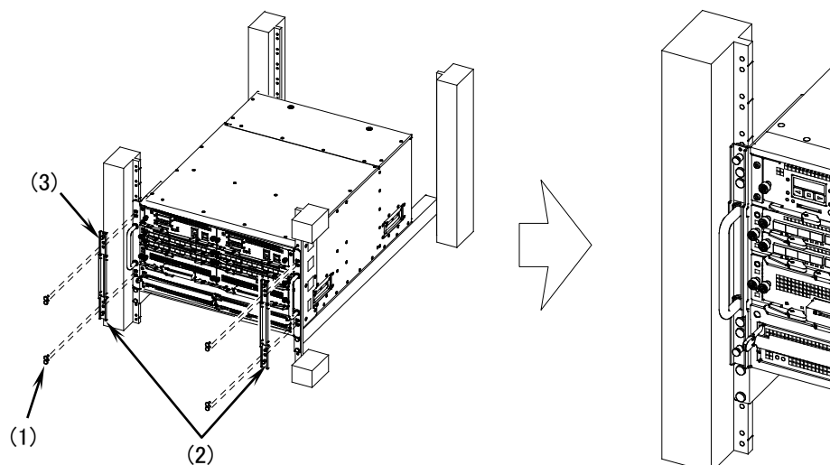
図4-10 ラックへの固定とアダプタ金具の取り付け
