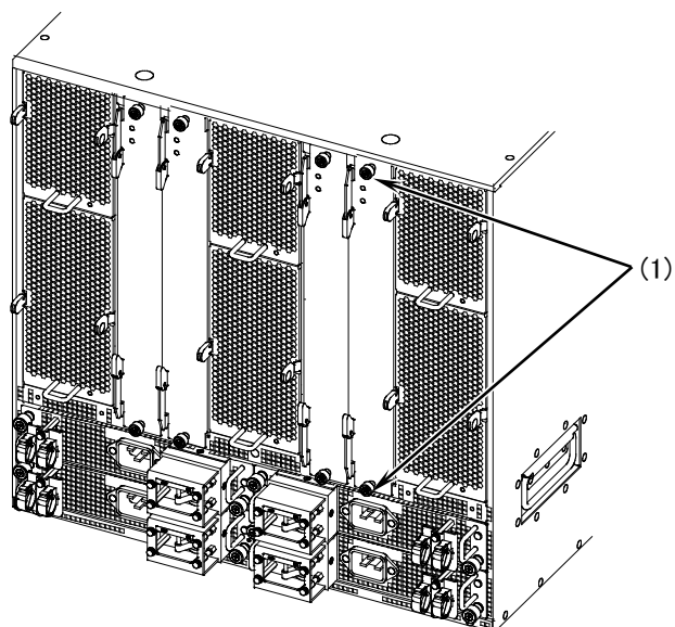
図5-36 スwitchファブリック機構の取り外し -1
