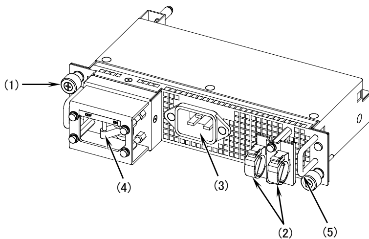
図1-15 外観
