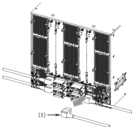
図5-6 電源ケーブルの取り外し
