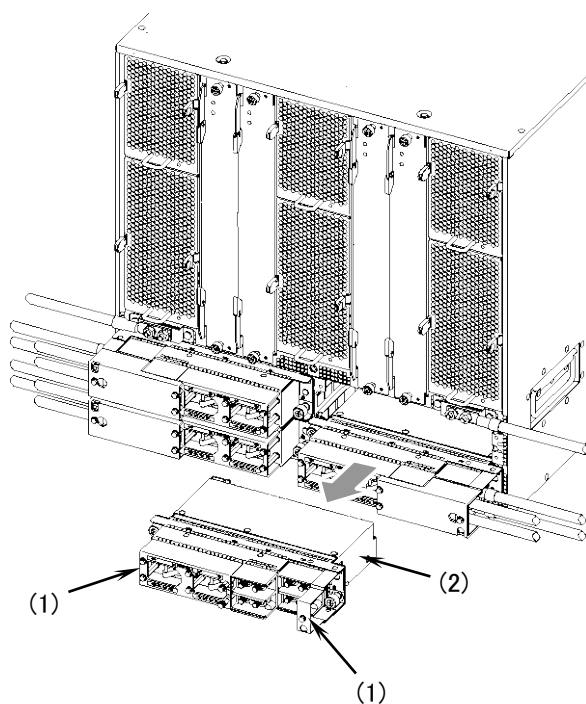
図5-14 電源入力機構の取り外し -2
