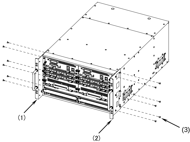
図4-2 ラック取り付け金具の取り付け
