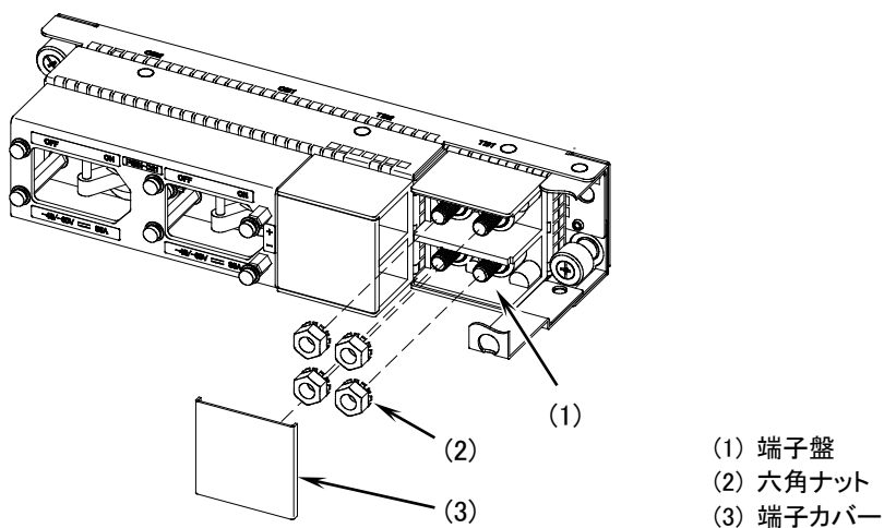
図4-30 端子カバー，六角ナットの取り外し（奥側）
