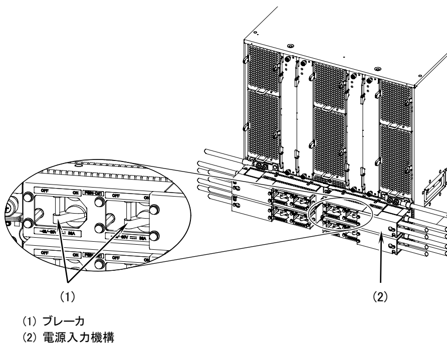
図5-11 電源の切断
