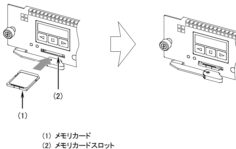
図4-40 メモリカードの取り付け
