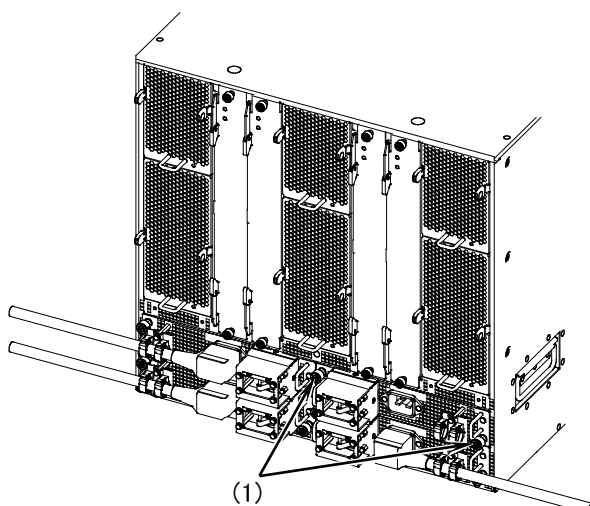
図5-10 電源入力機構の取り付け -2
