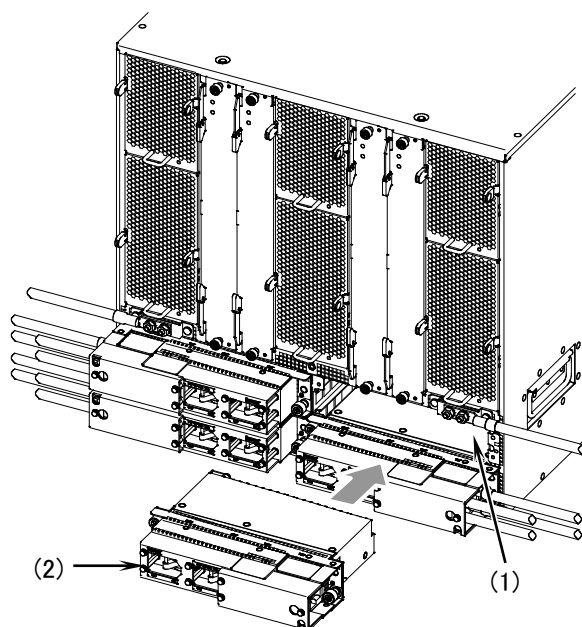
図5-15 電源入力機構の取り付け -1
