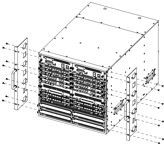
図4-3 ラック取り付け金具の取り外し
