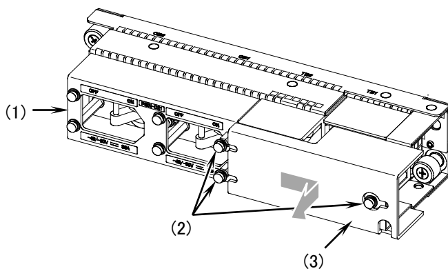
図4-29 端子盤のカバーの取り外し
