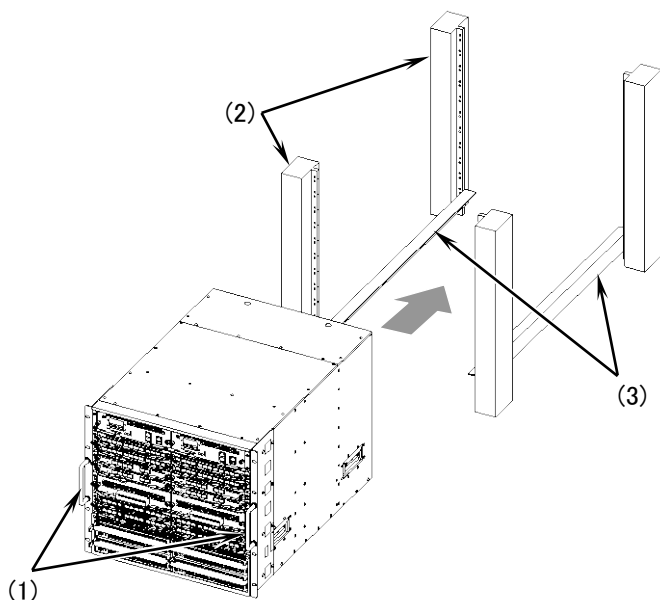
図4-15 ラックへの搭載
