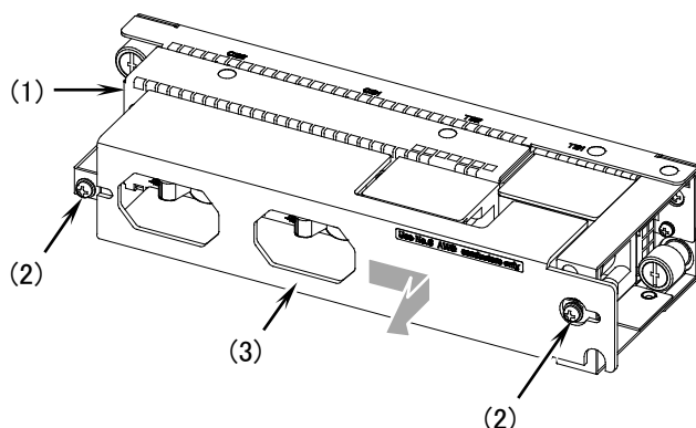
図4-34 端子盤のカバーの取り外し
