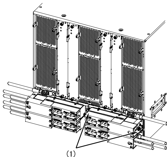
図5-16 電源入力機構の取り付け -2
