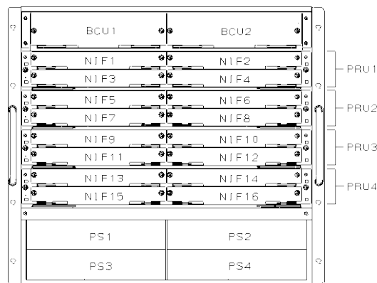
図1-7 装置正面側
