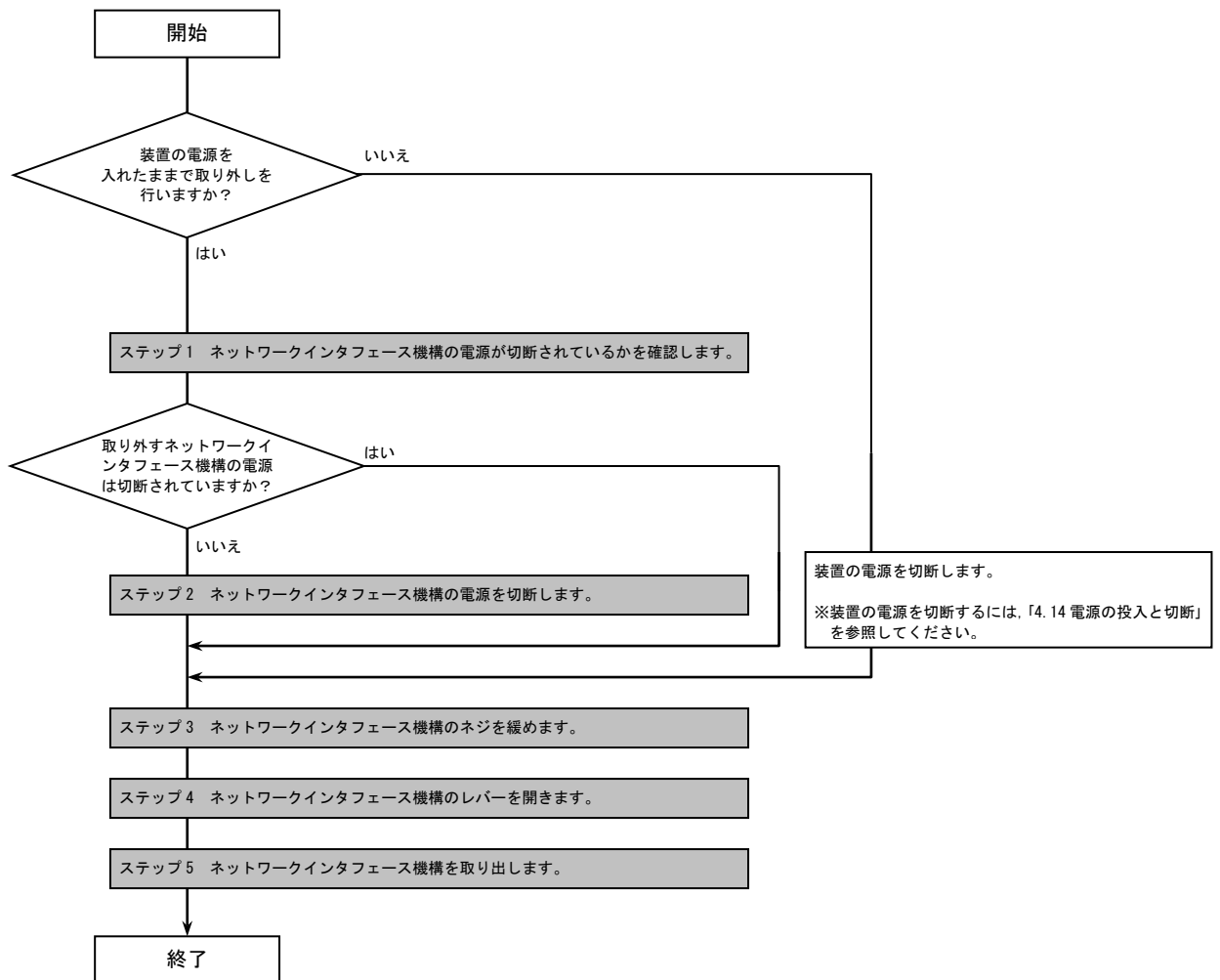
図5-54 取り外しの操作の流れ
