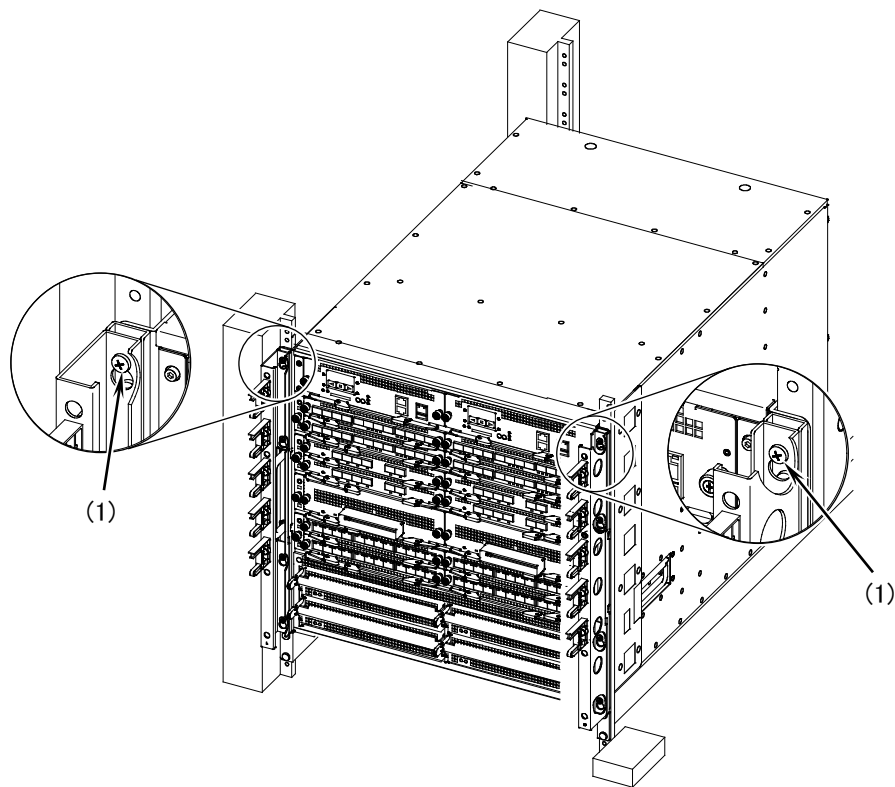
図4-18 ケーブルガイドの固定
