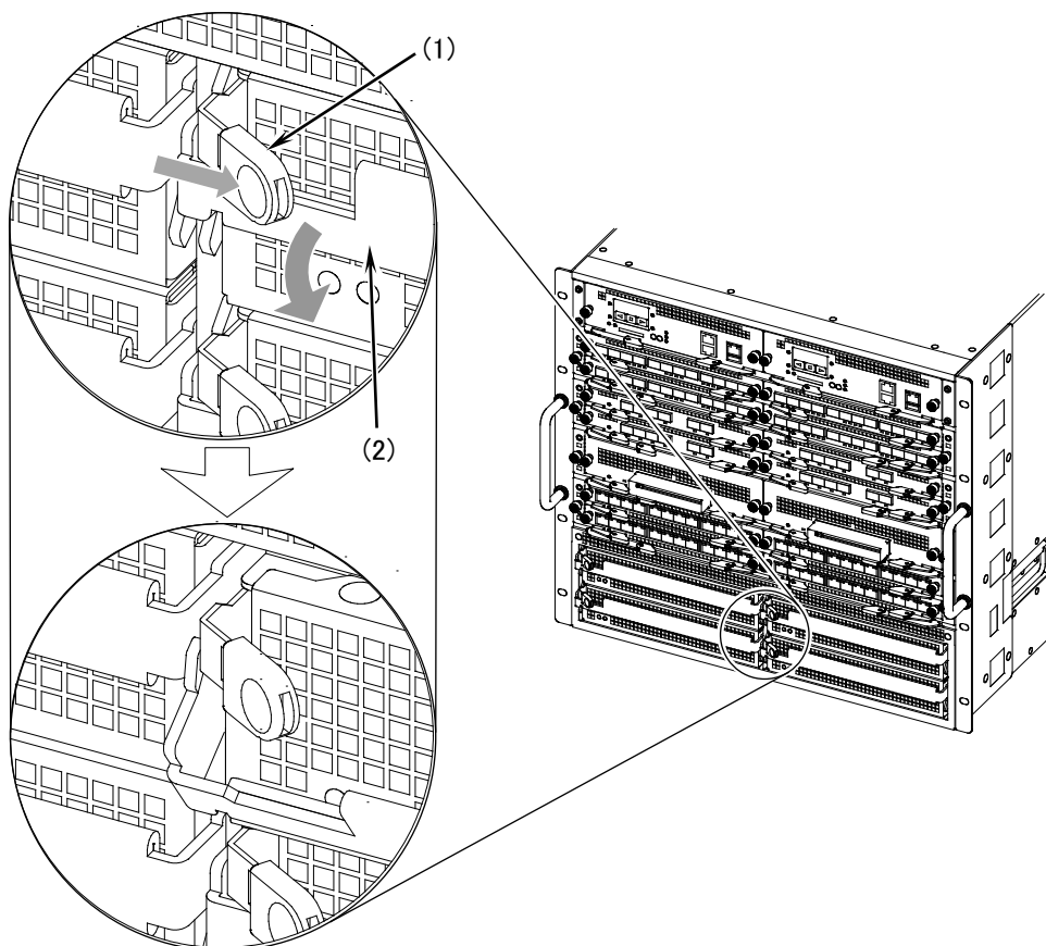
図5-18 電源機構のレバーロックの解除
