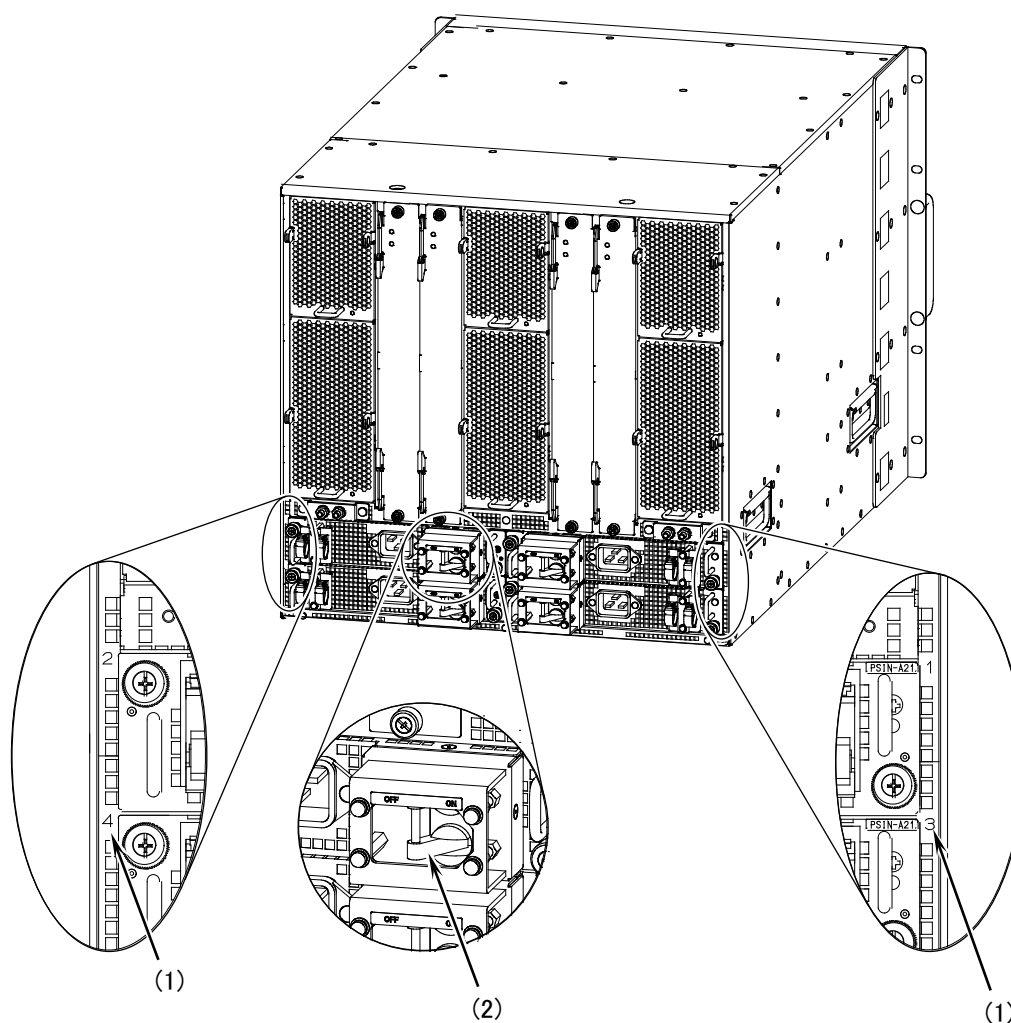
図4-60 電源の投入（PSIN-A21, PSIN-A22 の場合）
