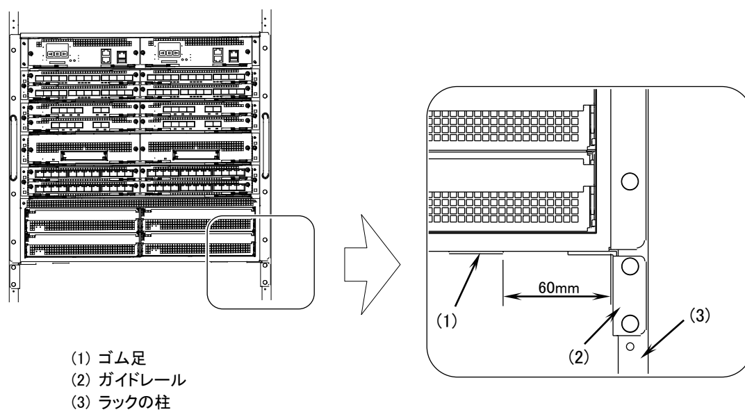
図2-10 ガイドレールの詳細
