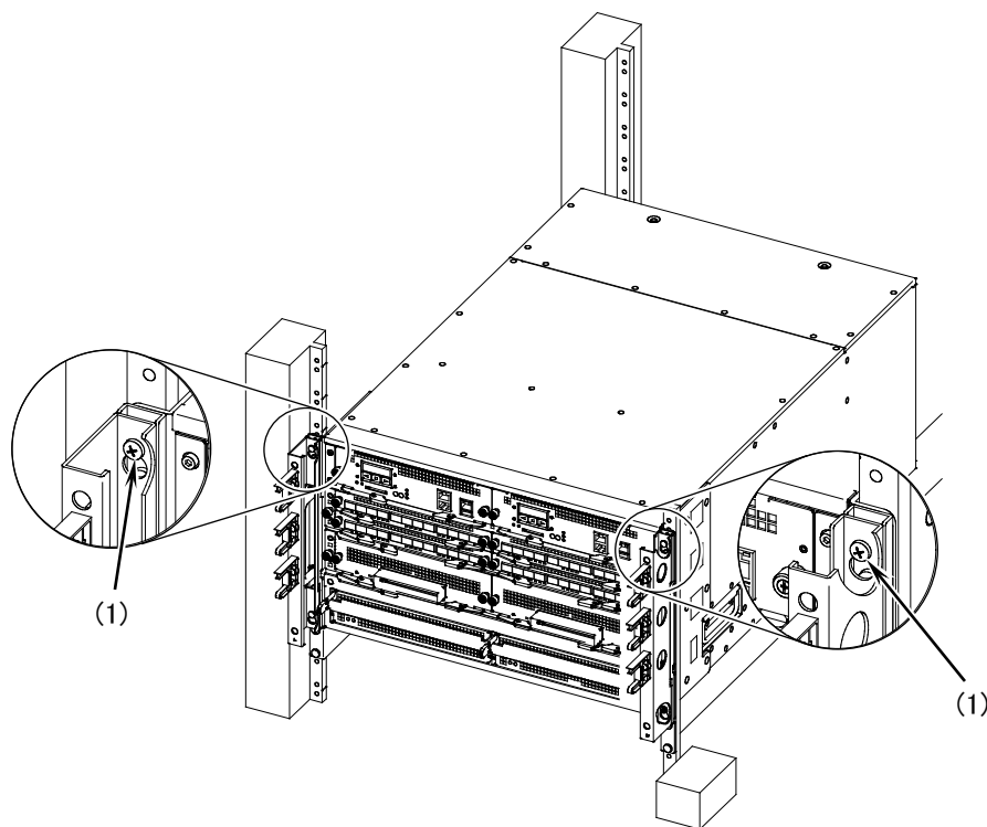
図4-12 ケーブルガイドの固定
