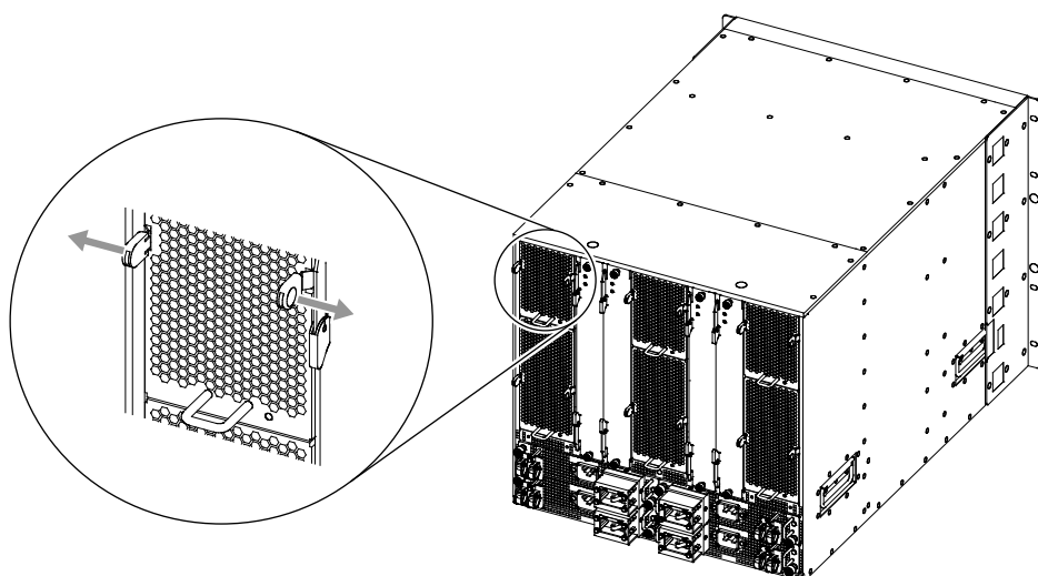
図5-4 ファンユニットのロックの確認
