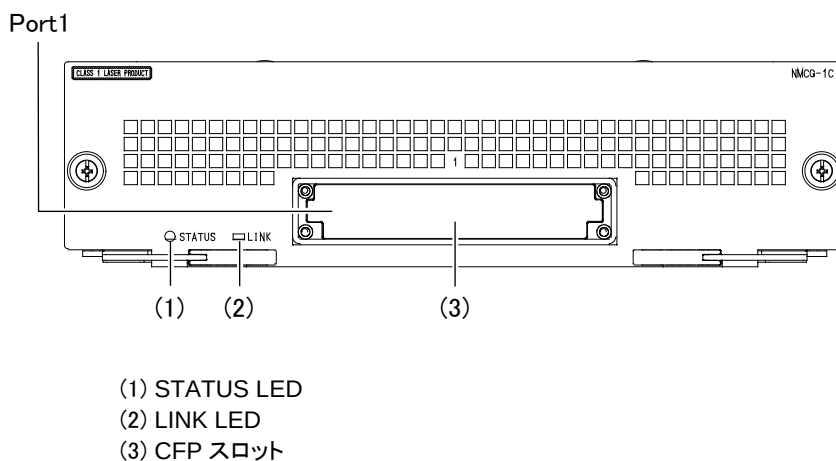
図1-44 正面外観
