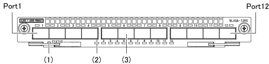
図1-38 正面外観
