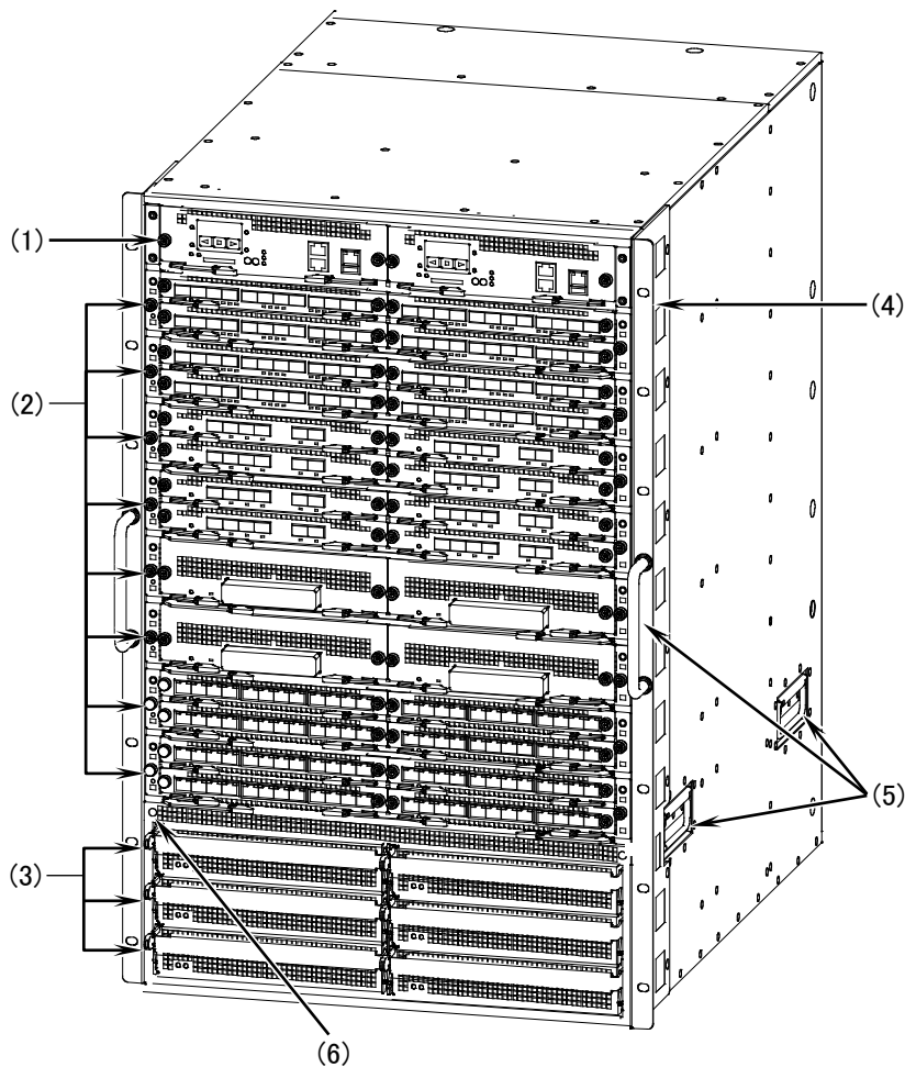
図1-9 正面外観
