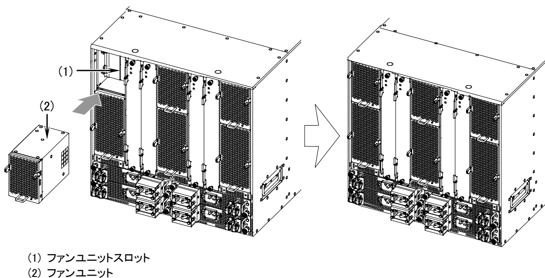
図5-3 ファンユニットの取り付け
