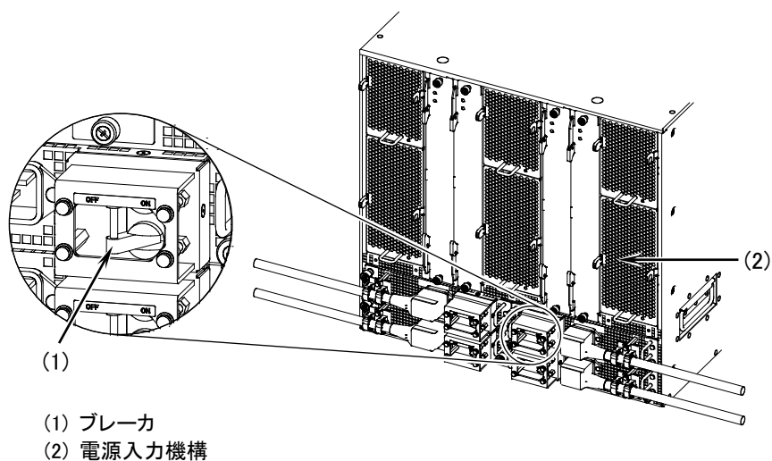
図5-5 電源の切断
