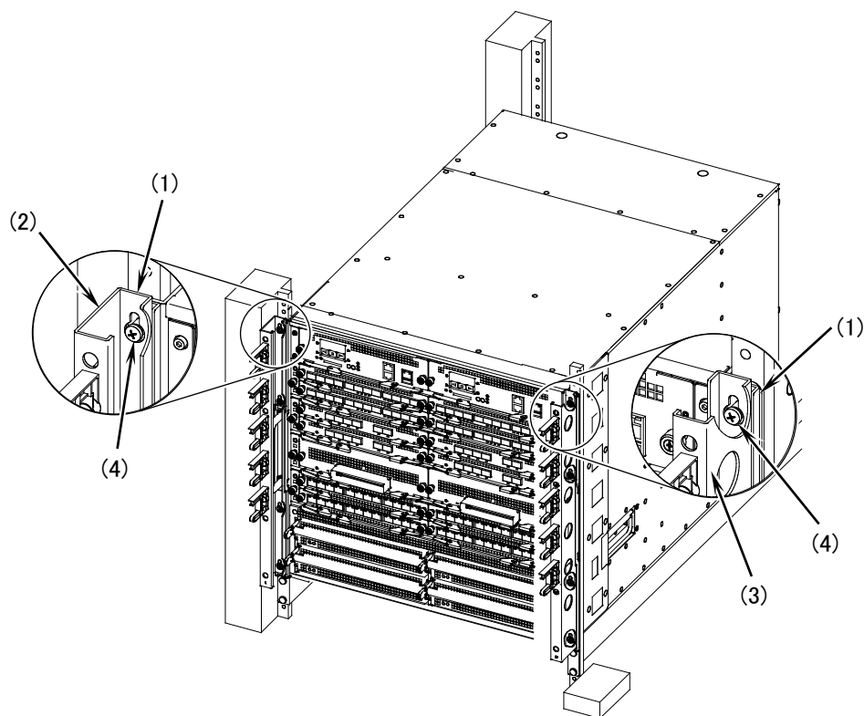
図4-17 ケーブルガイドの取り付け
