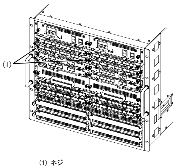
図5-56 ネットワークインタフェース機構の取り外し-1
