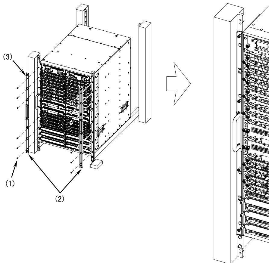
図4-22 ラックへの固定とアダプタ金具の取り付け
