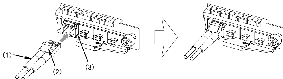
図4-56 光ファイバケーブル（LC2 芯コネクタ）の取り付け
