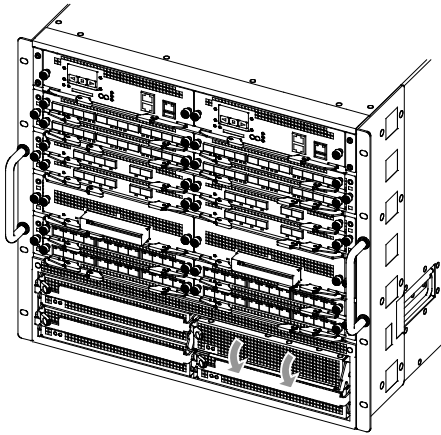
図5-19 電源機構の取り外し -1
