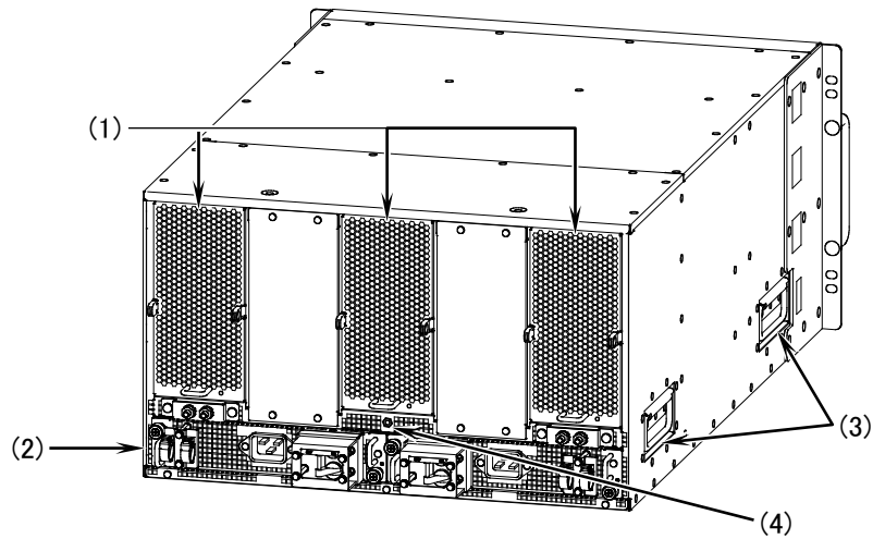
図1-2 背面外観
