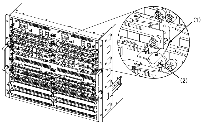
図5-61 ネットワークインタフェース機構の取り付け -2
