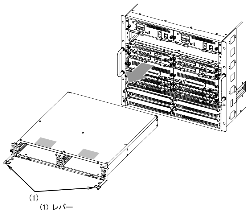
図5-48 パケットルーティング機構の取り外し -3
