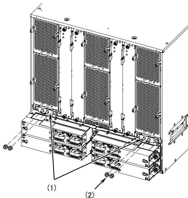
図4-27 六角ナットを取り外し
