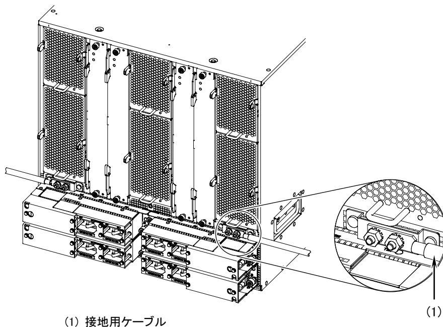
図4-28 接地用ケーブルの固定
