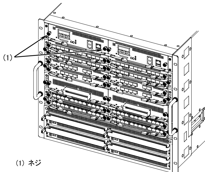
図5-26 基本制御機構の取り外し -1
