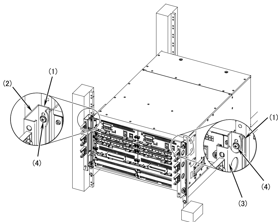
図4-11 ケーブルガイドの取り付け
