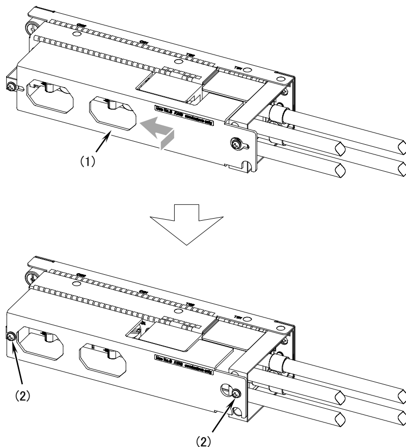
図4-38 端子盤のカバーの取り付け
