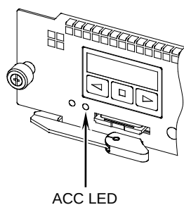
図4-41 ACC LED の確認
