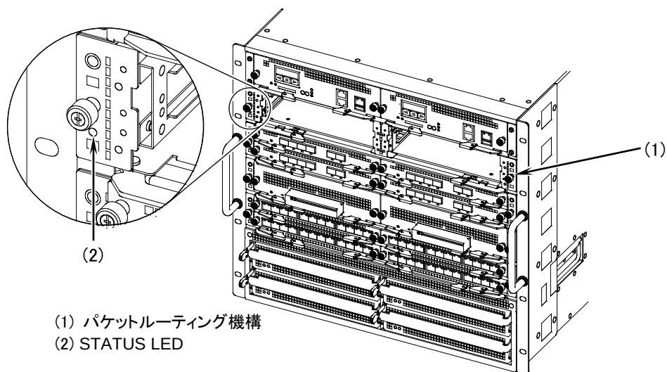
図5-45 STATUS LED の確認
