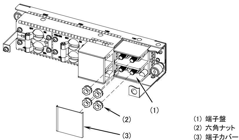
図4-35 端子カバー，六角ナットの取り外し（奥側）
