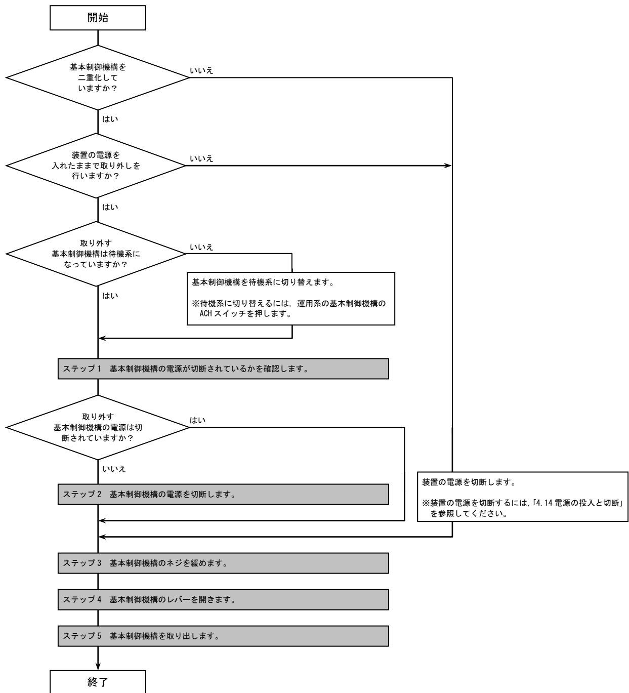
図5-24 取り外しの操作の流れ
