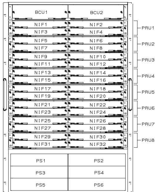
図1-11 装置正面側
