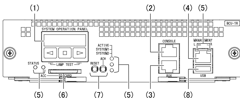
図1-22 正面外観
