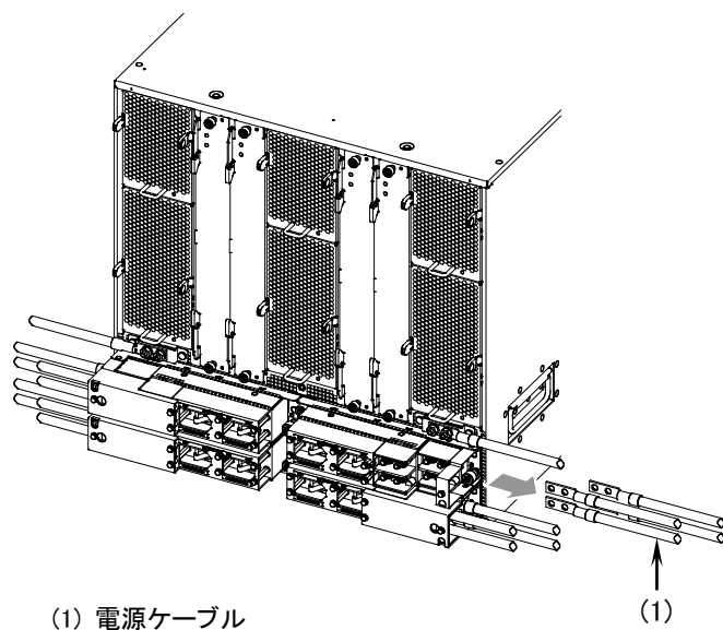
図5-12 電源ケーブルの取り外し
