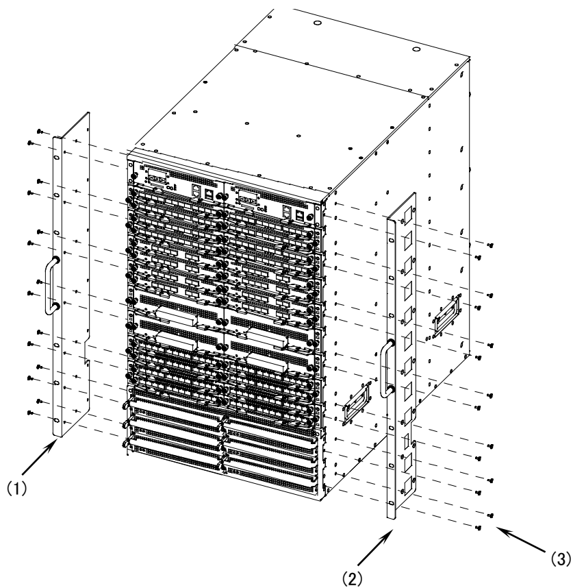
図4-5 ラック取り付け金具の取り外し
