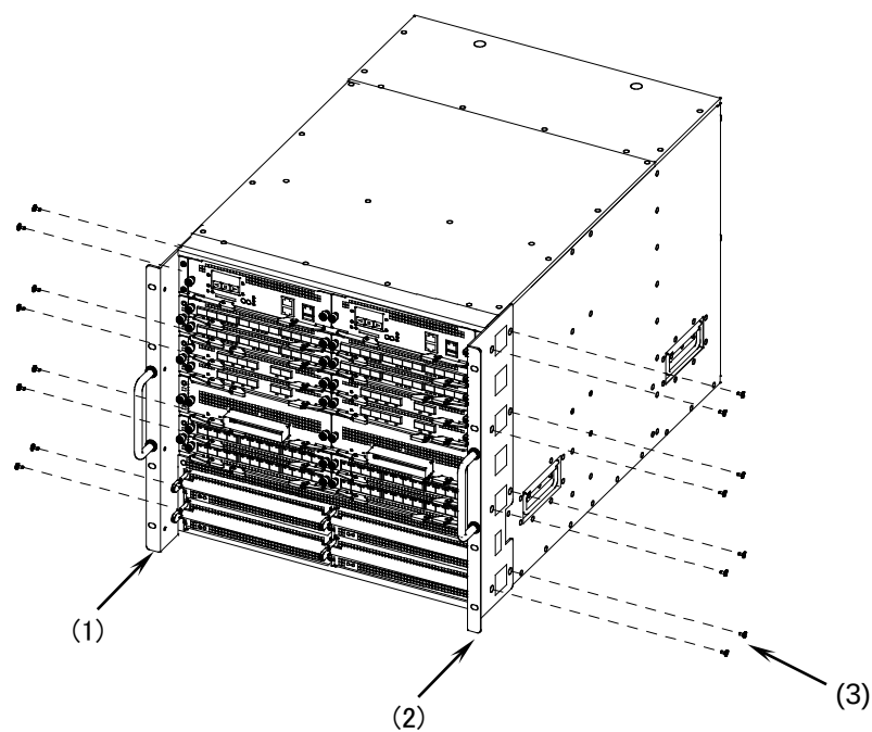
図4-4 ラック取り付け金具の取り付け
