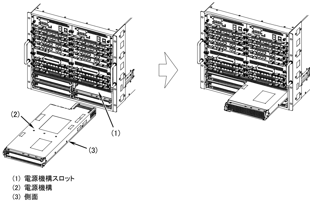
図5-21 電源機構の取り付け -1
