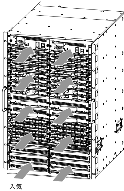
図2-14 IP8800/R8632 のエアフロー
