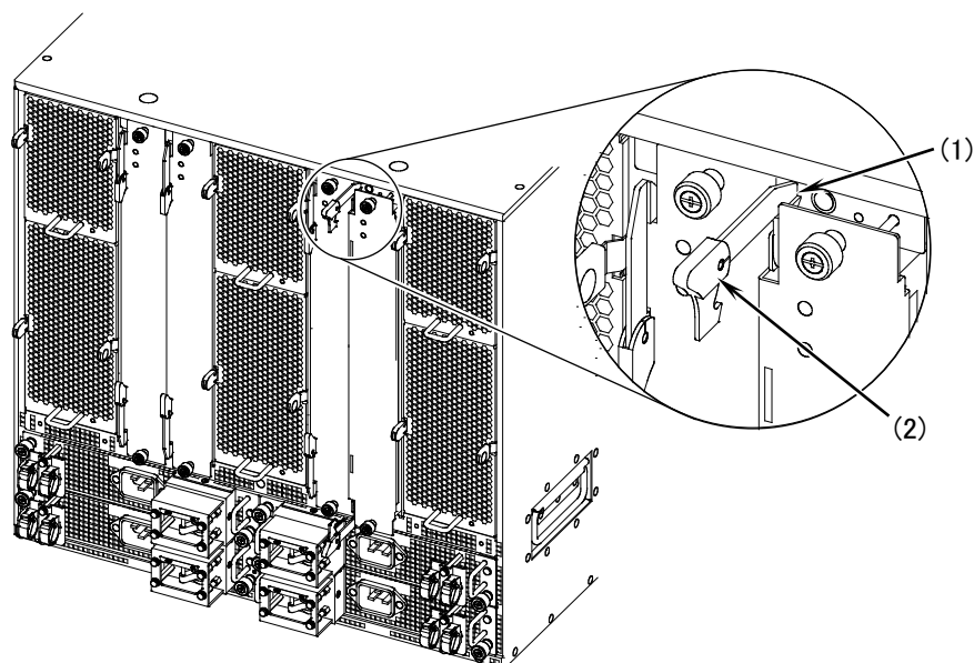
図5-41 スイッチファブリック機構の取り付け -2
