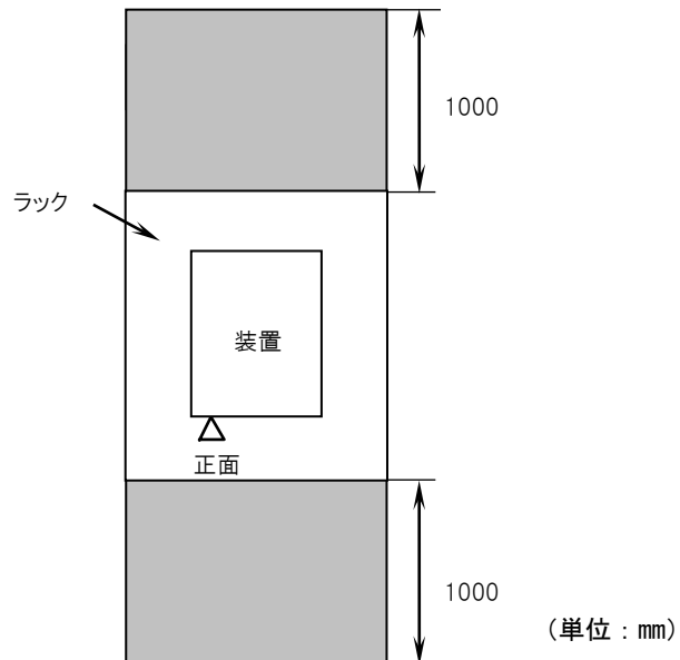
図2-11 ラック搭載時の保守エリア
