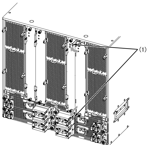
図5-37 スwitchファブリック機構の取り外し -2
