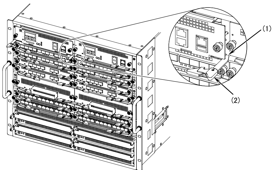
図5-31 基本制御機構の取り付け -2
