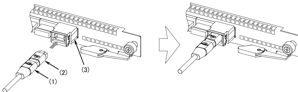
図4-58 光ファイバケーブル（MPO コネクタ）の取り付け
