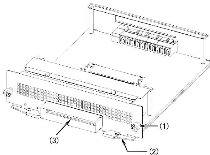
図1-43 外観
