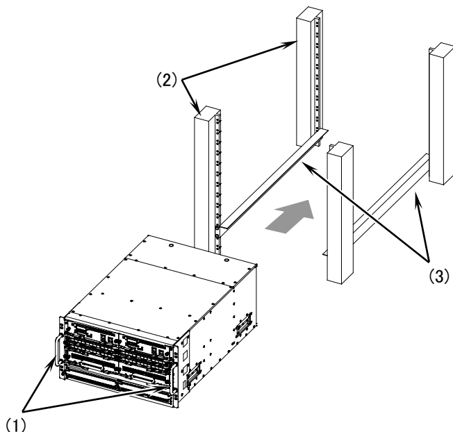
図4-9 ラックへの搭載
