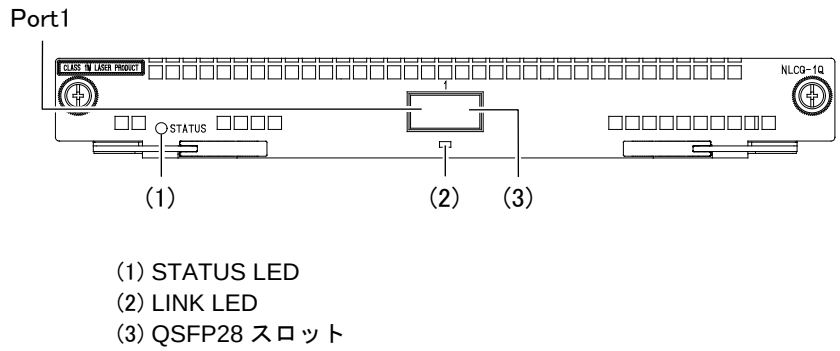
図1-42 正面外観
