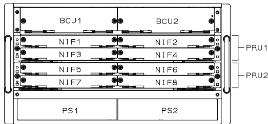
図1-3 装置正面側
