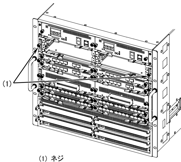
図5-53 パケットルーティング機構の取り付け -4
