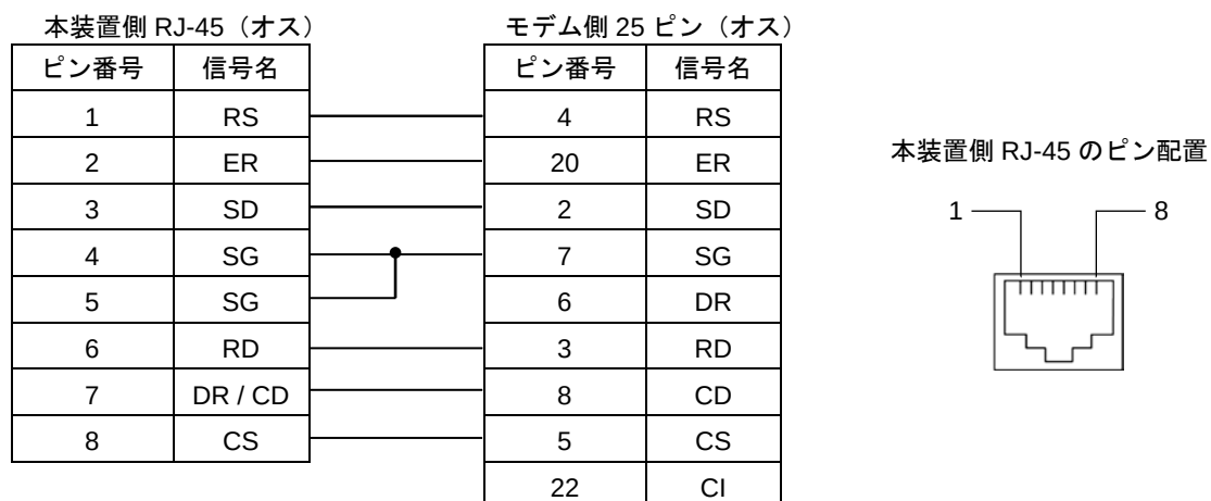
図3-2 モデム接続ケーブル
