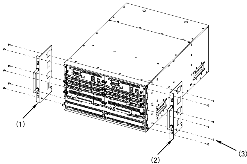
図4-1 ラック取り付け金具の取り外し
