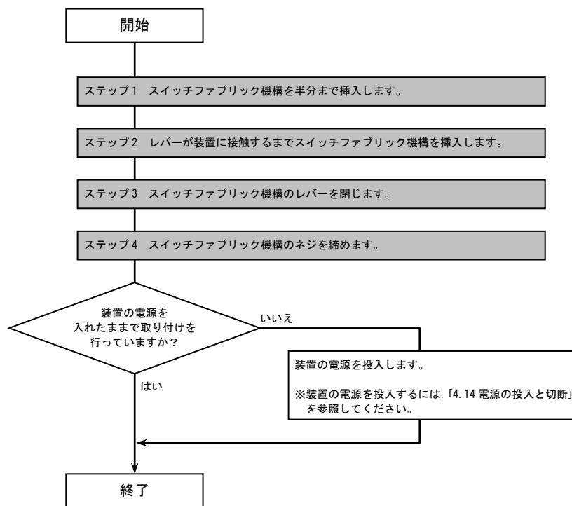
図5-39 取り付けの操作の流れ
