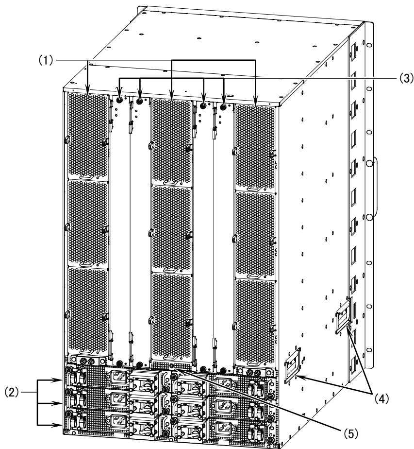
図1-10 背面外観
