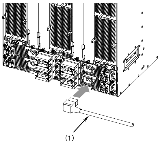
図4-25 電源ケーブルの取り付け
