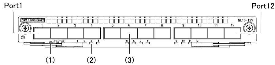
図1-32 正面外観
