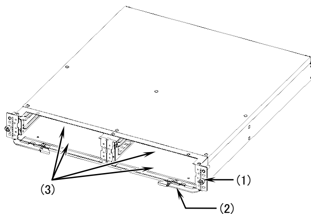
図1-27 外観
