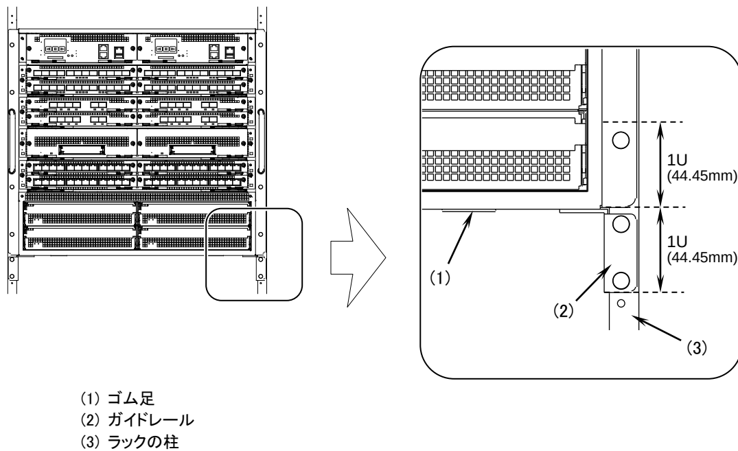
図4-14 ガイドレールの取り付け位置
