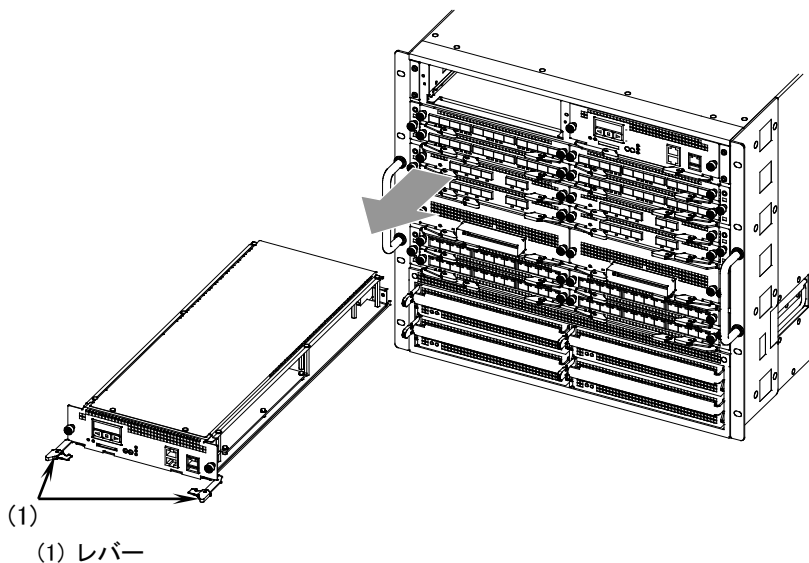
図5-28 基本制御機構の取り外し -3
