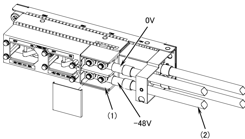
図4-32 電源ケーブルの取り付け（手前側）
