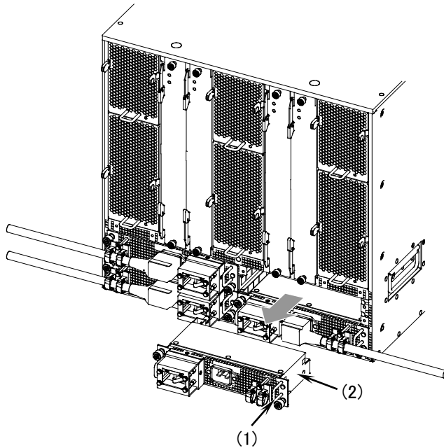
図5-8 電源入力機構の取り外し -2
