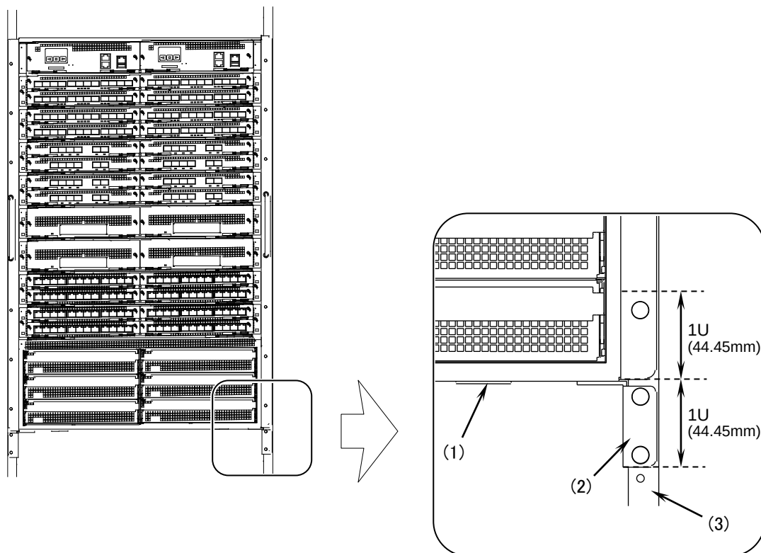
図4-20 ガイドレールの取り付け位置
