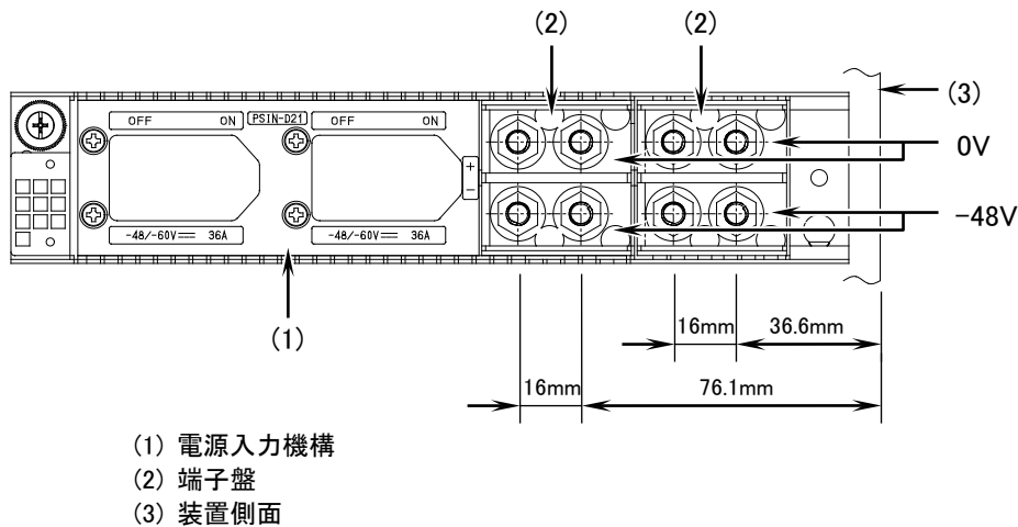
図2-9 電源入力機構の端子盤
