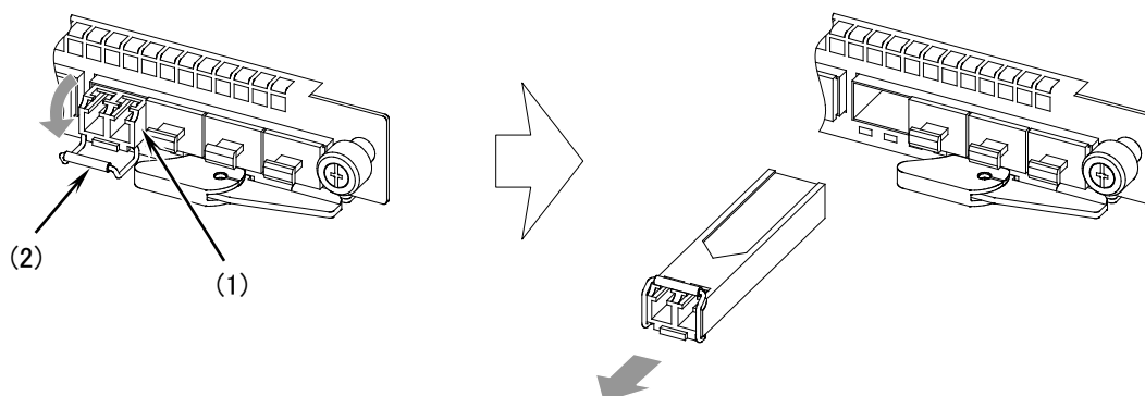
図4-45 SFP の取り外し
