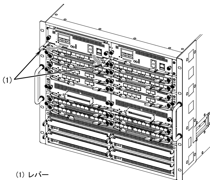
図5-27 基本制御機構の取り外し -2
