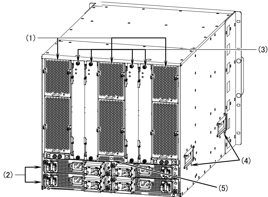
図1-6 背面外観
