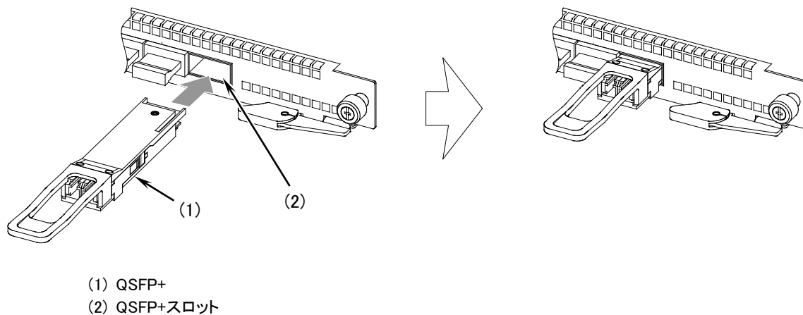
図4-47 QSFP+ の取り付け（プルタブタイプの場合）
