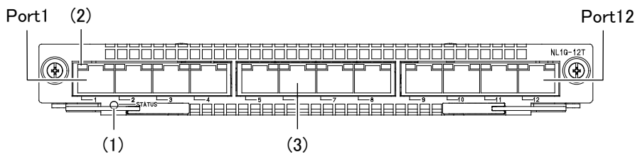
図1-31 正面外観
