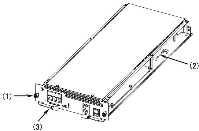
図1-21 外観
