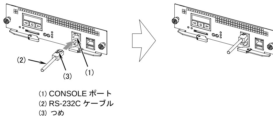
図4-53 RS-232C ケーブルの取り付け
