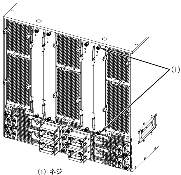
図5-43 スwitchファブリック機構の取り付け -4
