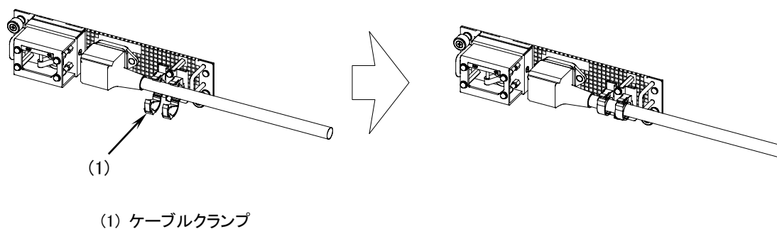
図4-26 電源ケーブルのクランプ
