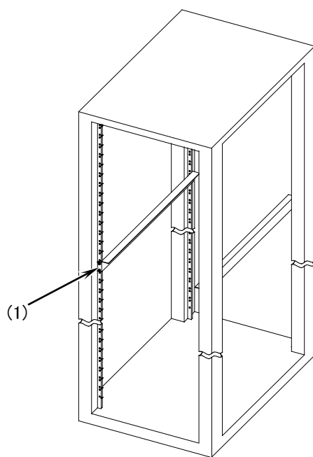
図4-13 ガイドレールの取り付け
