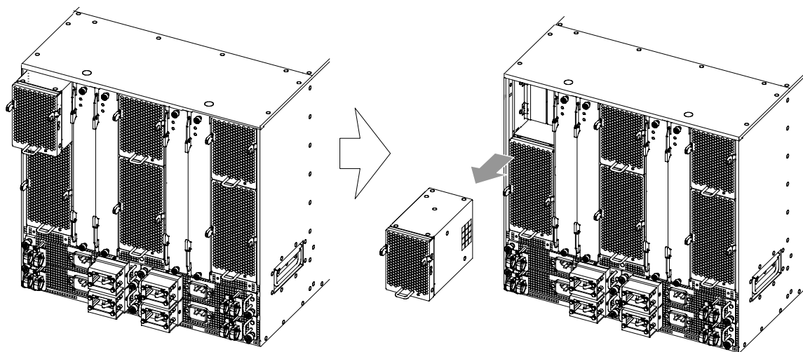
図5-2 ファンユニットの取り外し
