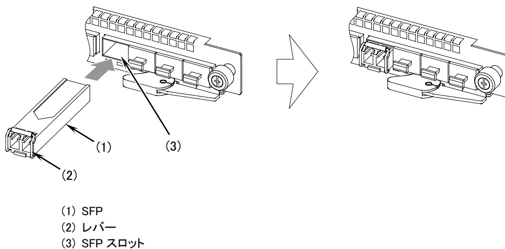
図4-44 SFP の取り付け
