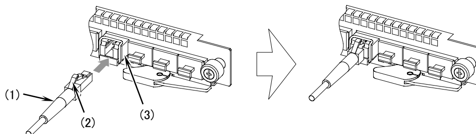
図4-57 光ファイバケーブル（LC1 芯コネクタ）の取り付け
