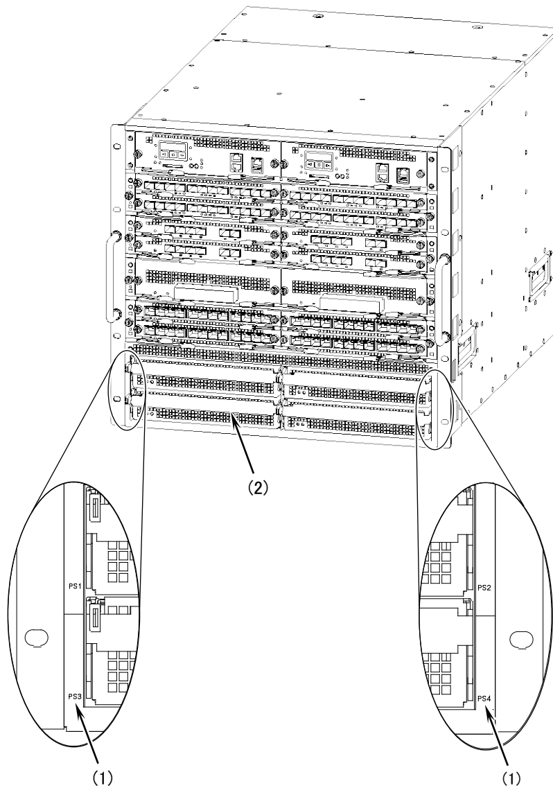
図4-59 電源機構搭載位置の確認
