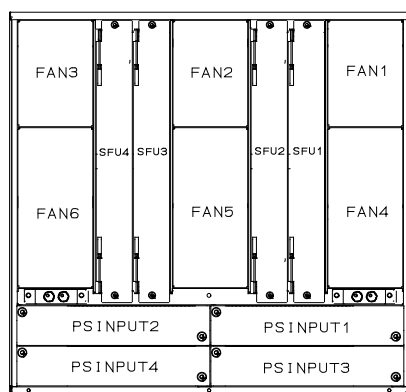
図1-8 装置背面側
