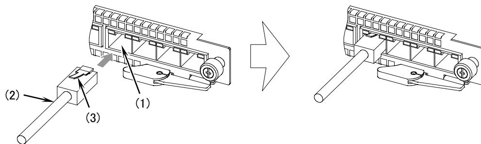
図4-55 UTP ケーブルの取り付け
