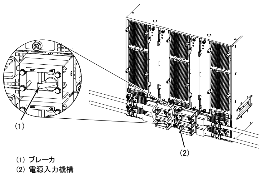
図5-17 電源の切断（PSIN-A21, PSIN-A22 の場合）
