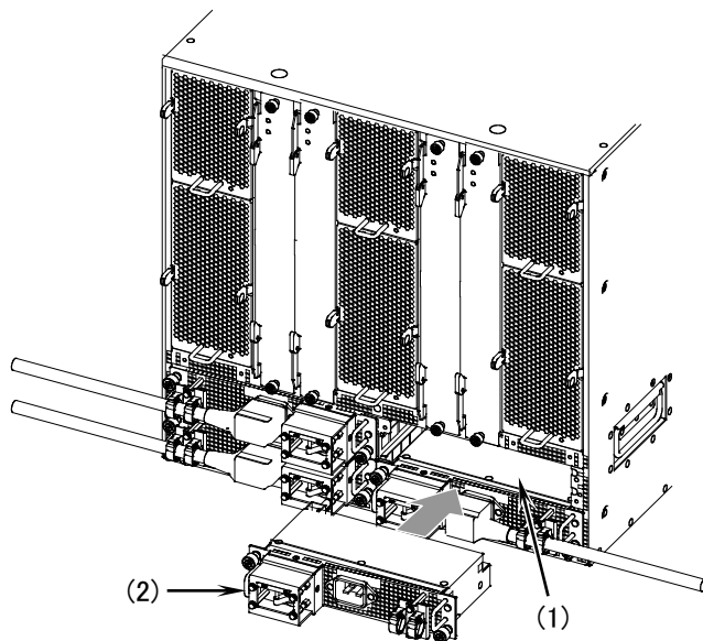
図5-9 電源入力機構の取り付け -1
