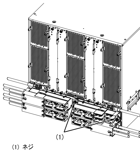
図5-13 電源入力機構の取り外し -1
