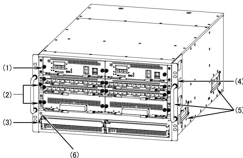
図1-1 正面外観
