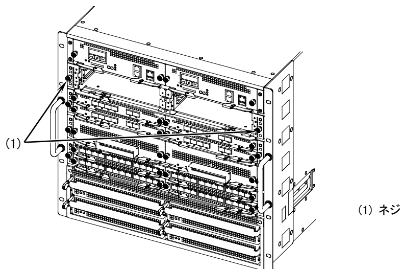
図5-46 パケットルーティング機構の取り外し -1
