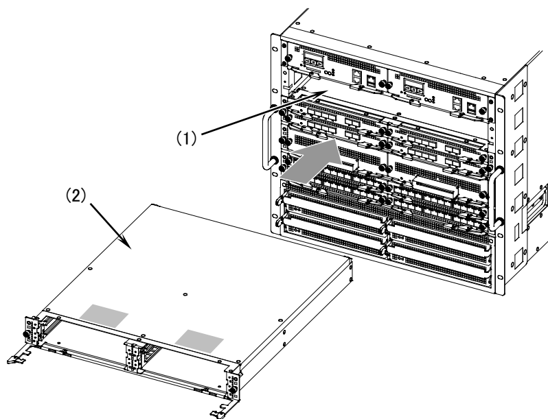
図5-50 パケットルーティング機構の取り付け -1
