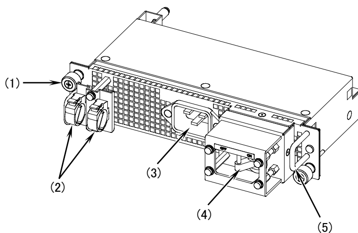
図1-16 外観
