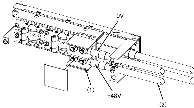
図4-37 電源ケーブルの取り付け（手前側）
