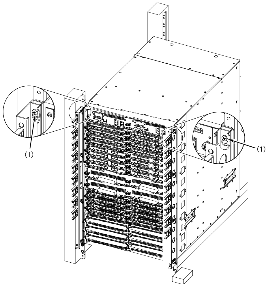
図4-24 ケーブルガイドの固定
