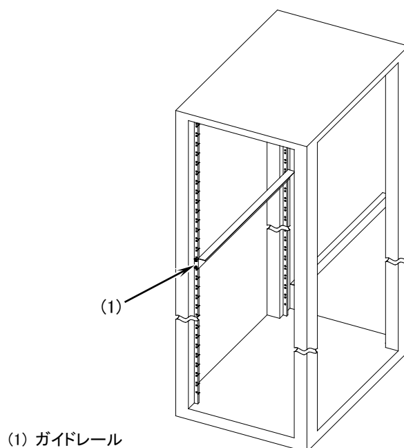
図4-7 ガイドレールの取り付け
