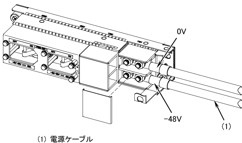
図4-31 電源ケーブルの取り付け（奥側）
