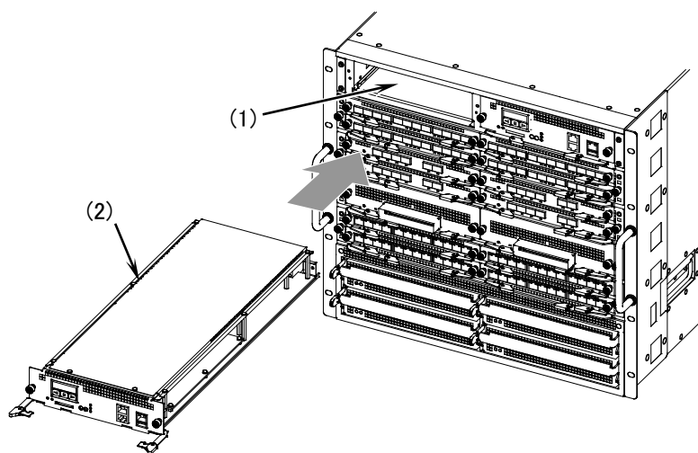
図5-30 基本制御機構の取り付け -1
