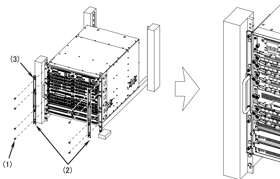
図4-16 ラックへの固定とアダプタ金具の取り付け
