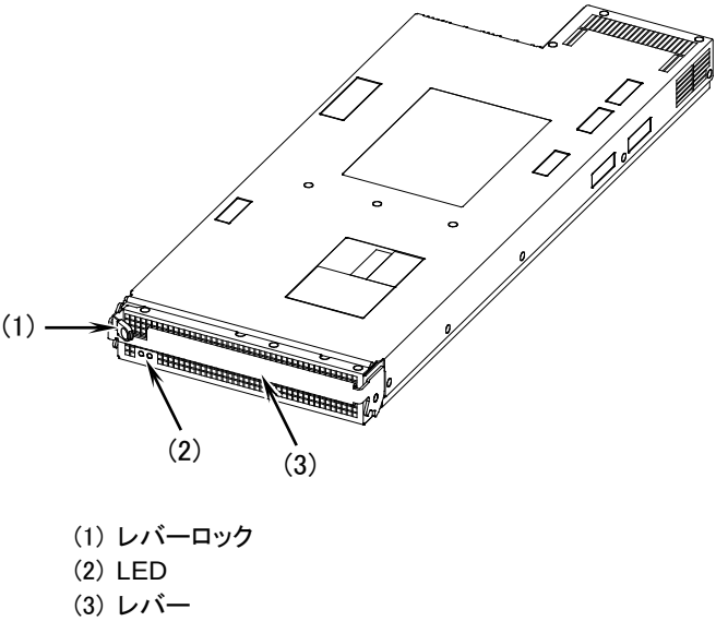
図1-19 外観
