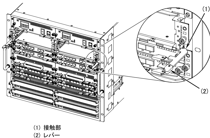
図5-51 パケットルーティング機構の取り付け -2
