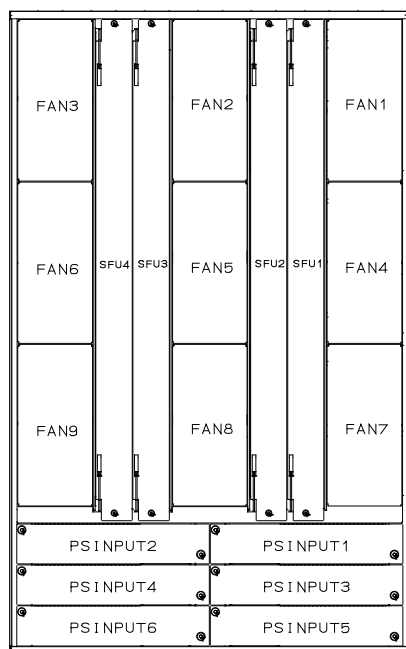
図1-12 装置背面側
