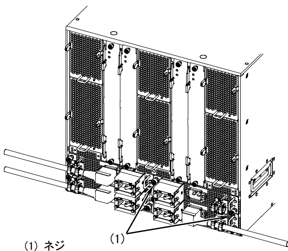
図5-7 電源入力機構の取り外し -1
