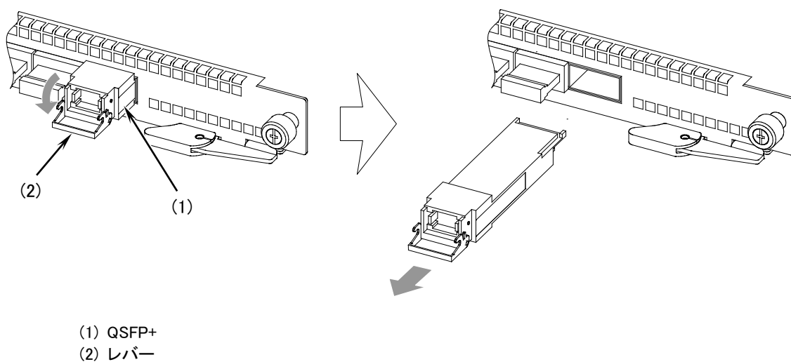
図4-48 QSFP+ の取り外し（レバータイプの場合）
