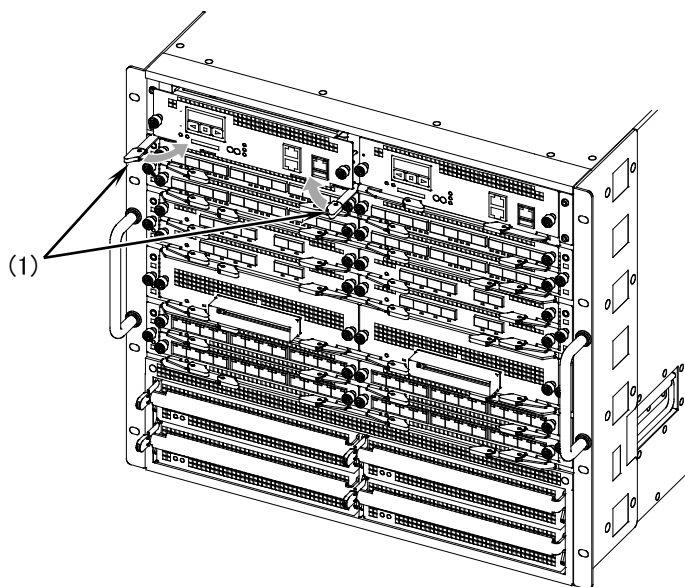
図5-32 基本制御機構の取り付け -3
