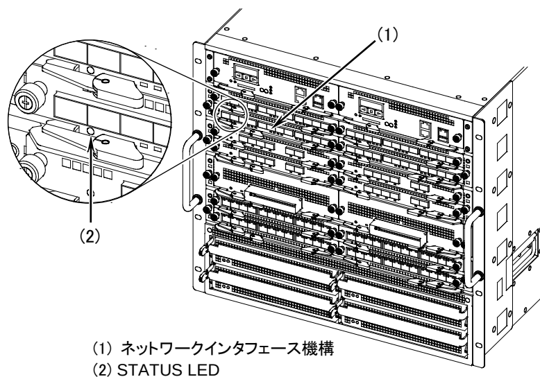
図5-55 STATUS LED の確認
