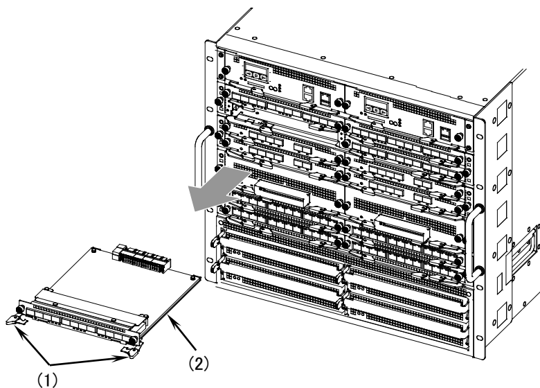
図5-58 ネットワークインタフェース機構の取り外し-3
