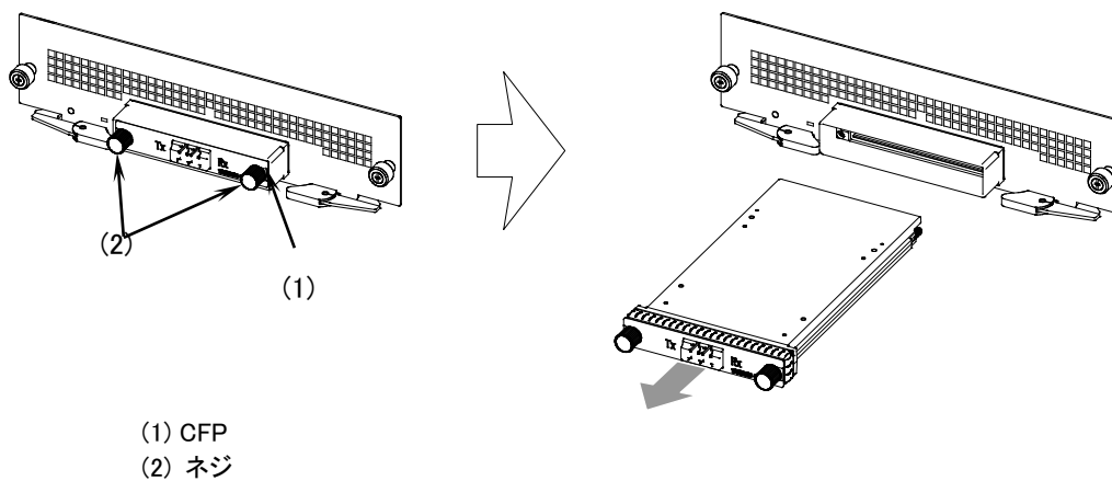
図4-51 CFP の取り外し
