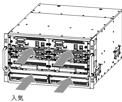
図2-12 IP8800/R8608 のエアフロー
