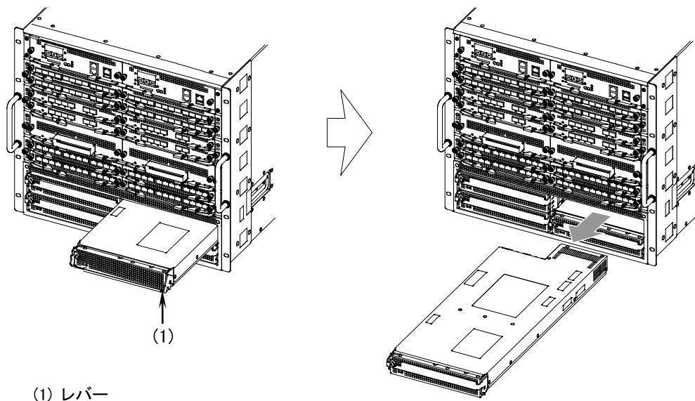
図5-20 電源機構の取り外し -2
