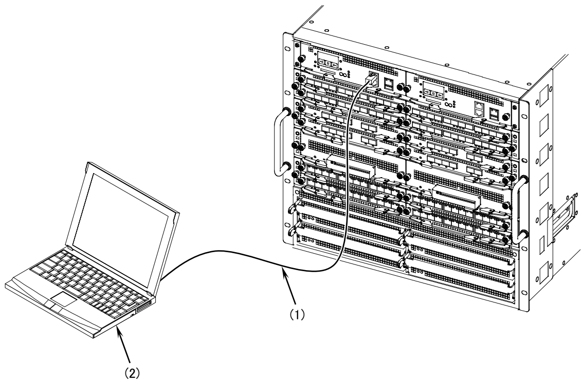
図4-52 運用端末の接続
