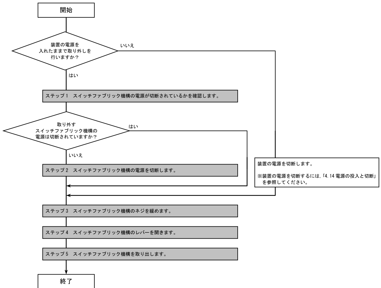
図5-34 取り外しの操作の流れ
