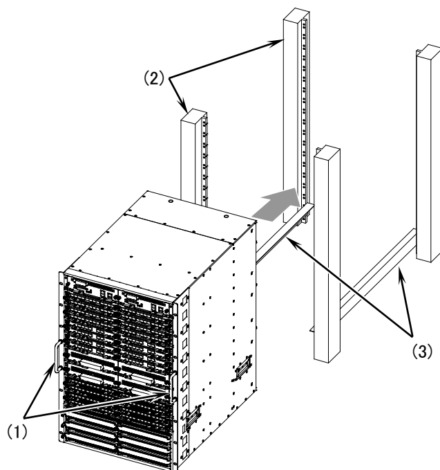
図4-21 ラックへの搭載
