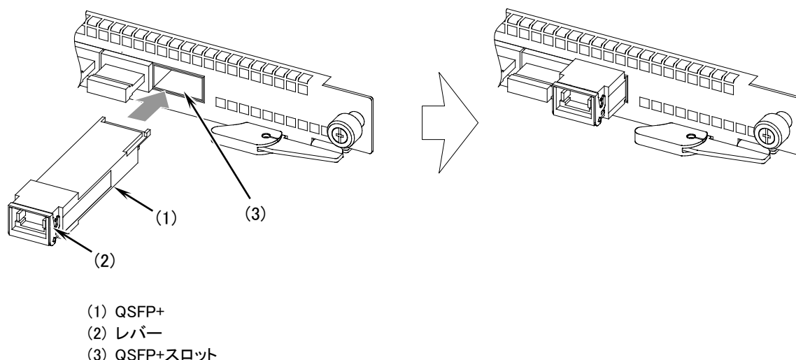
図4-46 QSFP+ の取り付け（レバータイプの場合）
