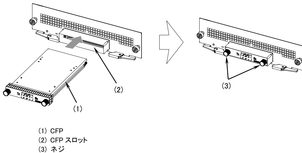
図4-50 CFP の取り付け
