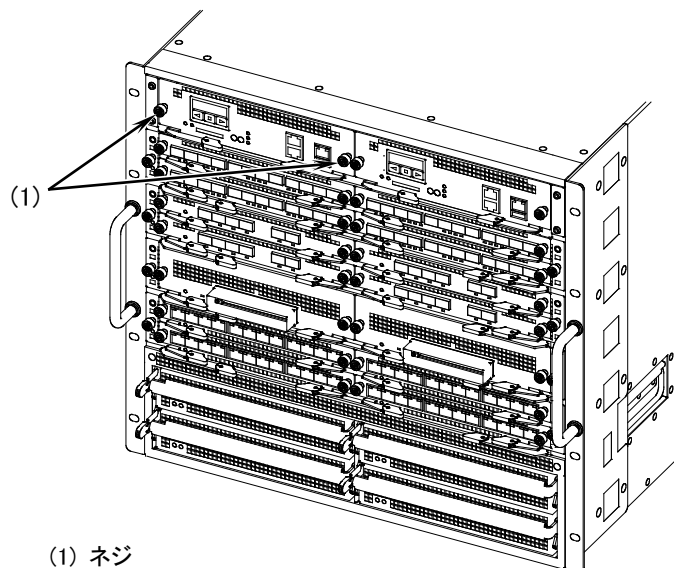
図5-33 基本制御機構の取り付け -4
