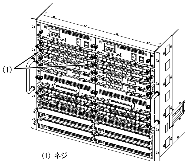
図5-63 ネットワークインタフェース機構の取り付け -4
