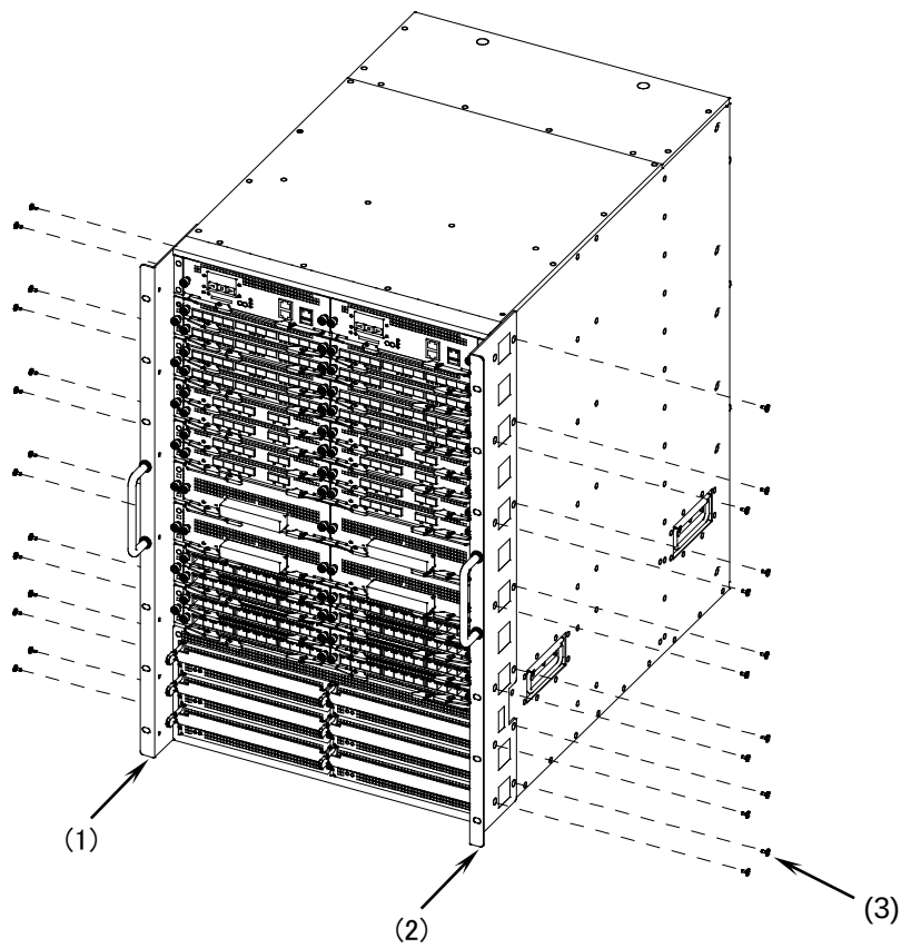
図4-6 ラック取り付け金具の取り付け
