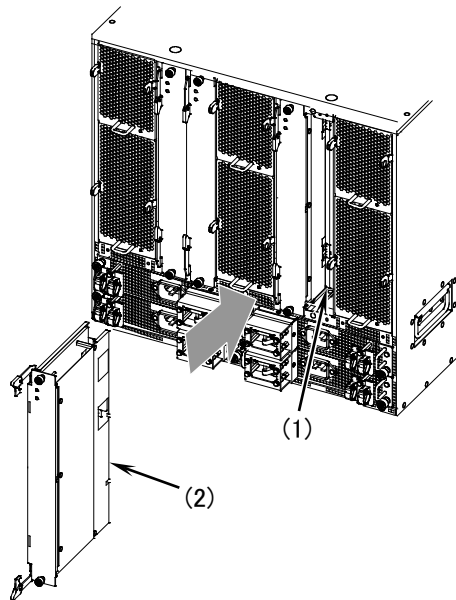
図5-40 スwitchファブリック機構の取り付け -1
