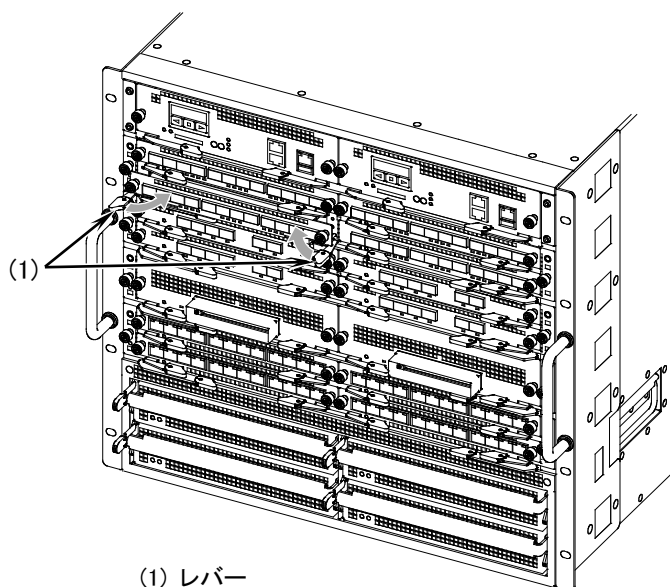
図5-62 ネットワークインタフェース機構の取り付け -3
