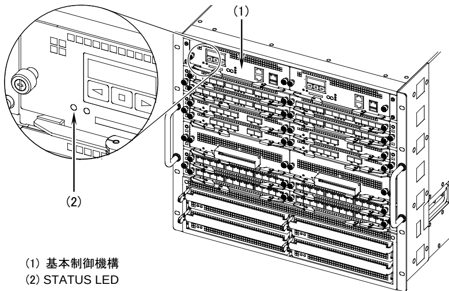
図5-25 STATUS LED の確認
