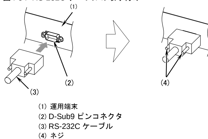
図4-54 RS-232C ケーブルの取り付け
