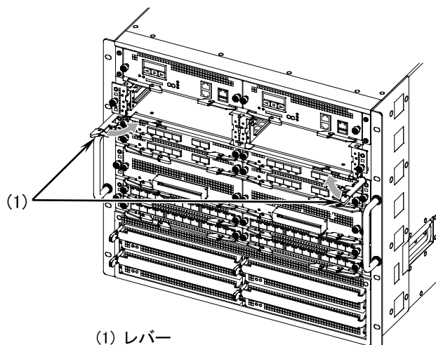
図5-52 パケットルーティング機構の取り付け -3
