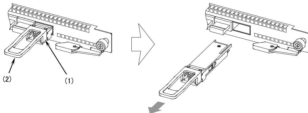
図4-49 QSFP+ の取り外し（プルタブタイプの場合）
