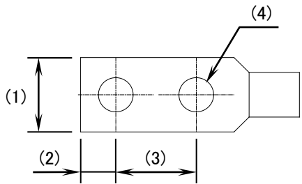
図2-7 接地用ケーブルの端子
