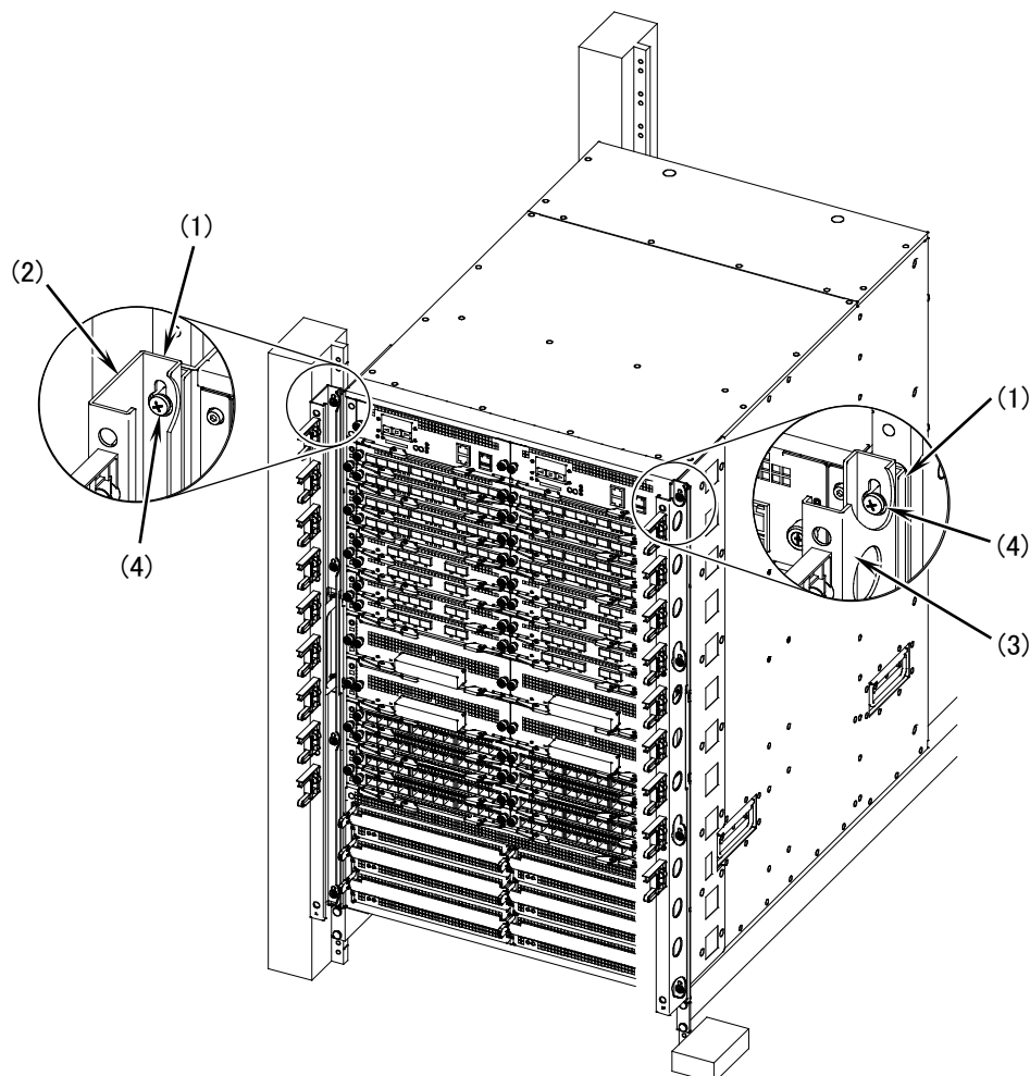
図4-23 ケーブルガイドの取り付け
