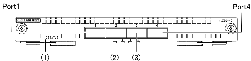
図1-40 正面外観
