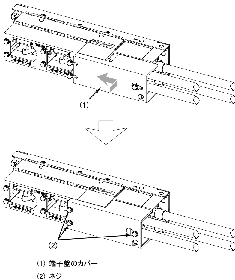
図4-33 端子盤のカバーの取り付け
