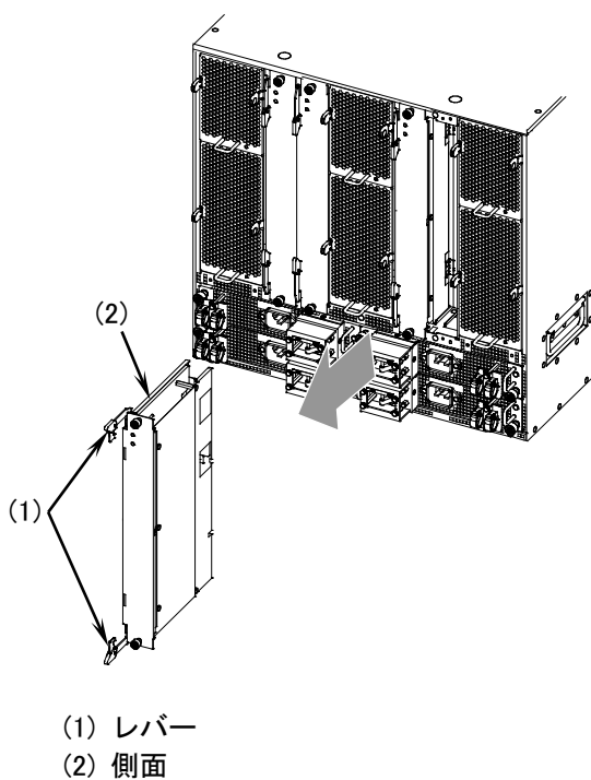
図5-38 スwitchファブリック機構の取り外し -3
