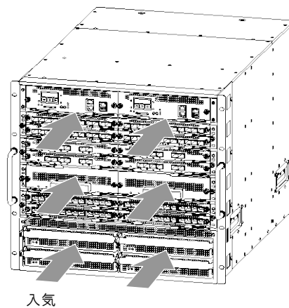
図2-13 IP8800/R8616 のエアフロー
