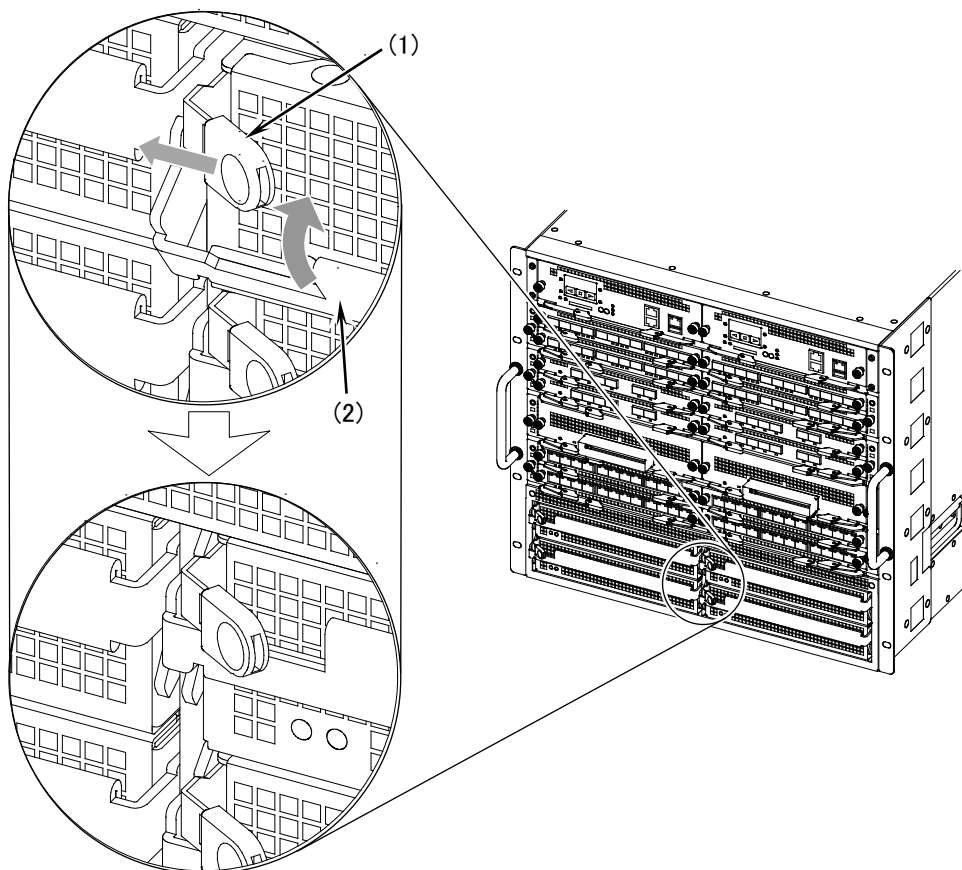
図5-23 電源機構のレバーロックの確認
