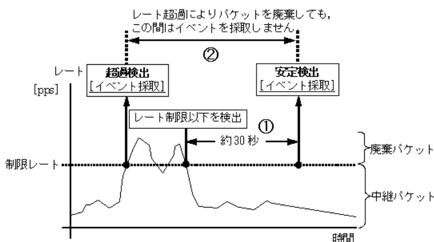
図 13-12 DHCP パケット受信レートの運用ログ情報採取契機
