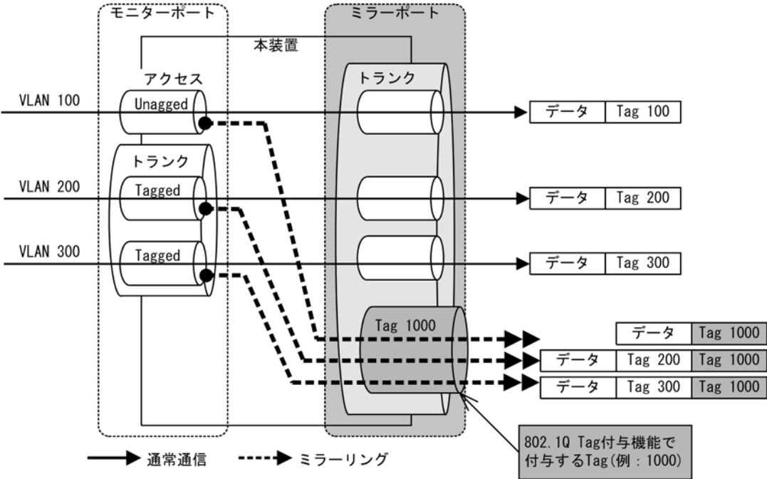
図 26-6 802.1Q Tag 付与機能の概要
