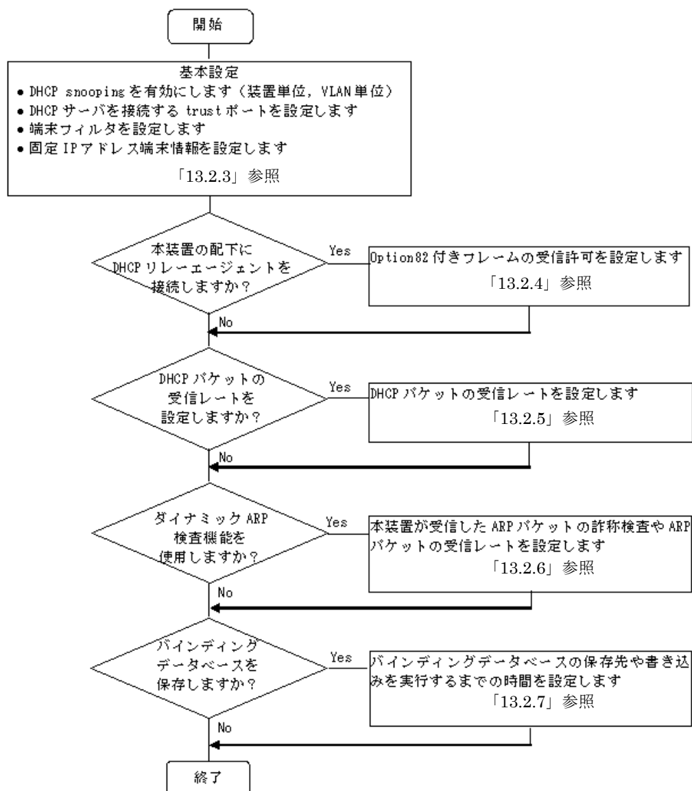
図 13-16 DHCP snooping の設定手順
