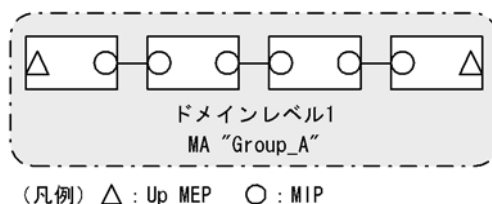
図 21-4 Up MEP の設定例
