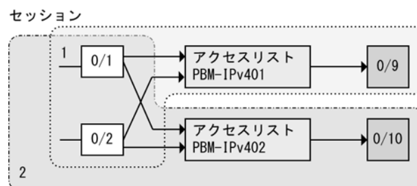
図 27-5 複数モニターポート対複数ミラーポートの設定例
