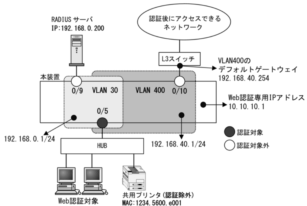
図 9-8 ダイナミック VLAN モードの認証除外の構成例
