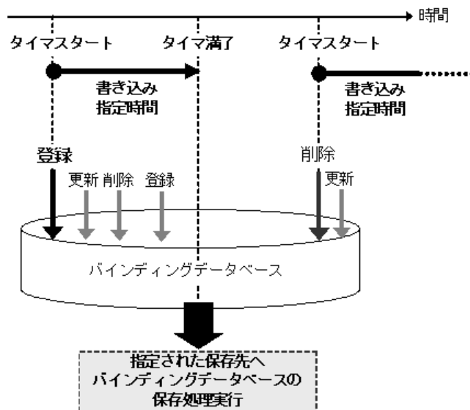
図 13-15 保存契機と書き込み指定時間の動作概要（バインディングデータベース登録を契機とした例）
