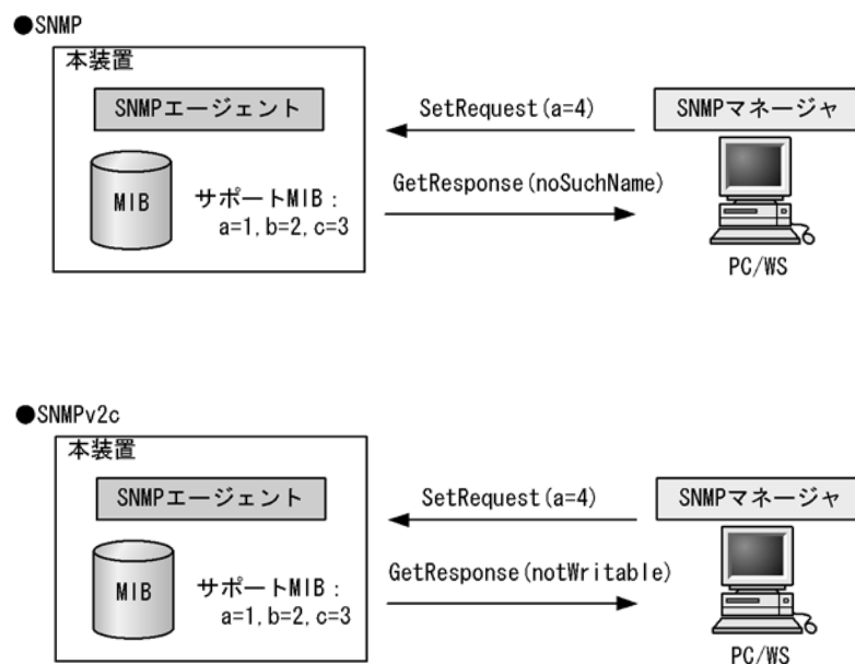
図 22-12 MIB 変数が読み出し専用の場合の SetRequest オペレーション
