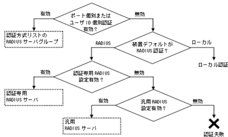
図 5-9 RADIUS サーバ情報併用設定時の運用
