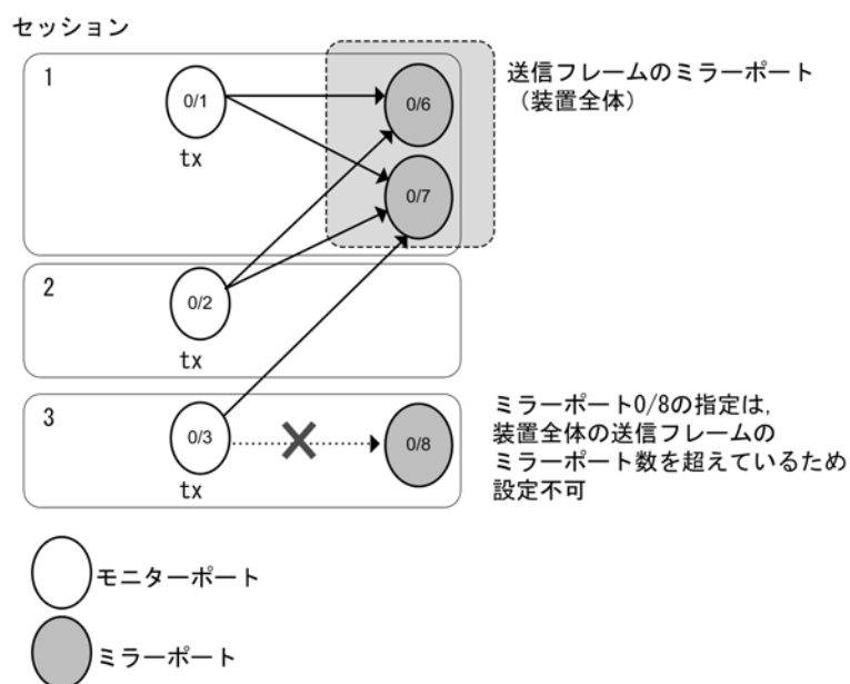
図 26-9 送信フレームのミラーポート数
