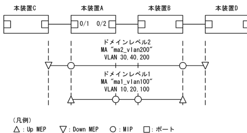
図 21-31 CFM の設定例（複数ドメイン）
