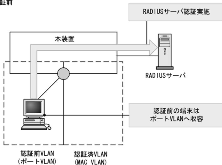
図 6-15 ポート単位認証（動的）の動作イメージ
