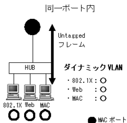
図 5-27 同一ポート内ダイナミック VLAN モードの共存例
