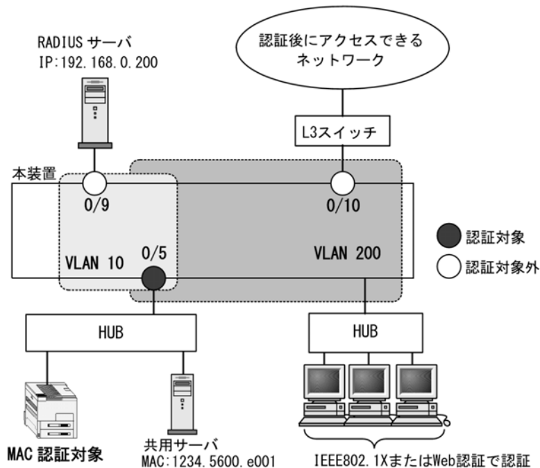
図 11-7 ダイナミック VLAN モードの構成例
