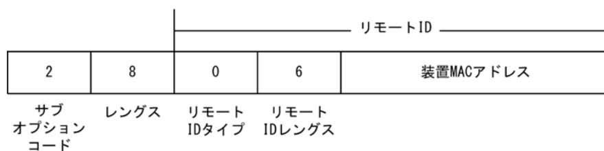
図 13-10 リモート ID タイプ 0 の形式
