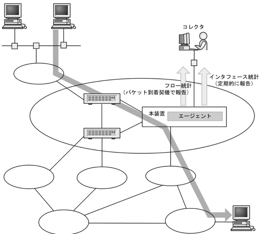
図 24-1 sFlow 統計のネットワーク構成例
