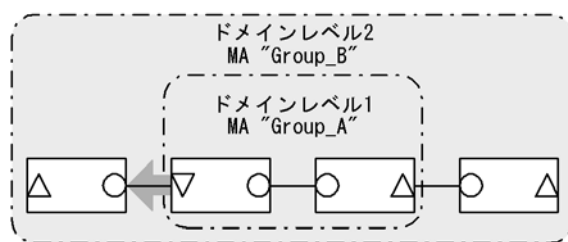
図 21-8 誤って Down MEP を設定した例
