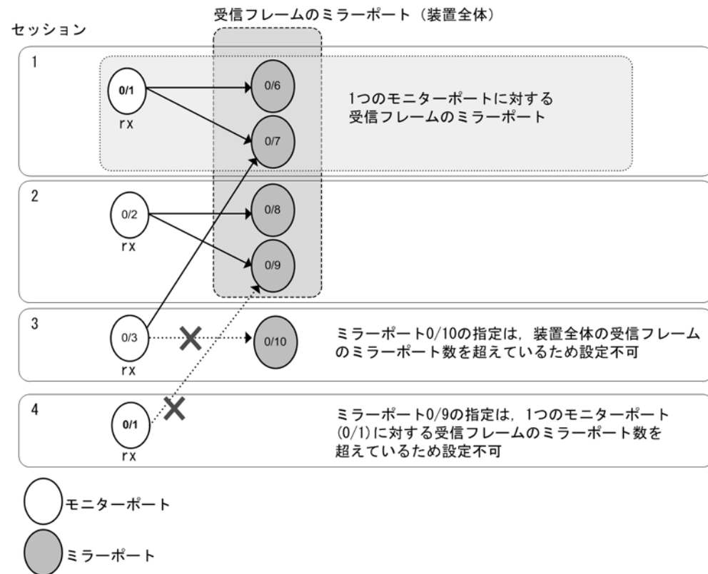
図 26-7 受信フレームのミラーポート数（ホワイトリスト機能、ICMP 限定ミラーリング機能のミラー設定無）
