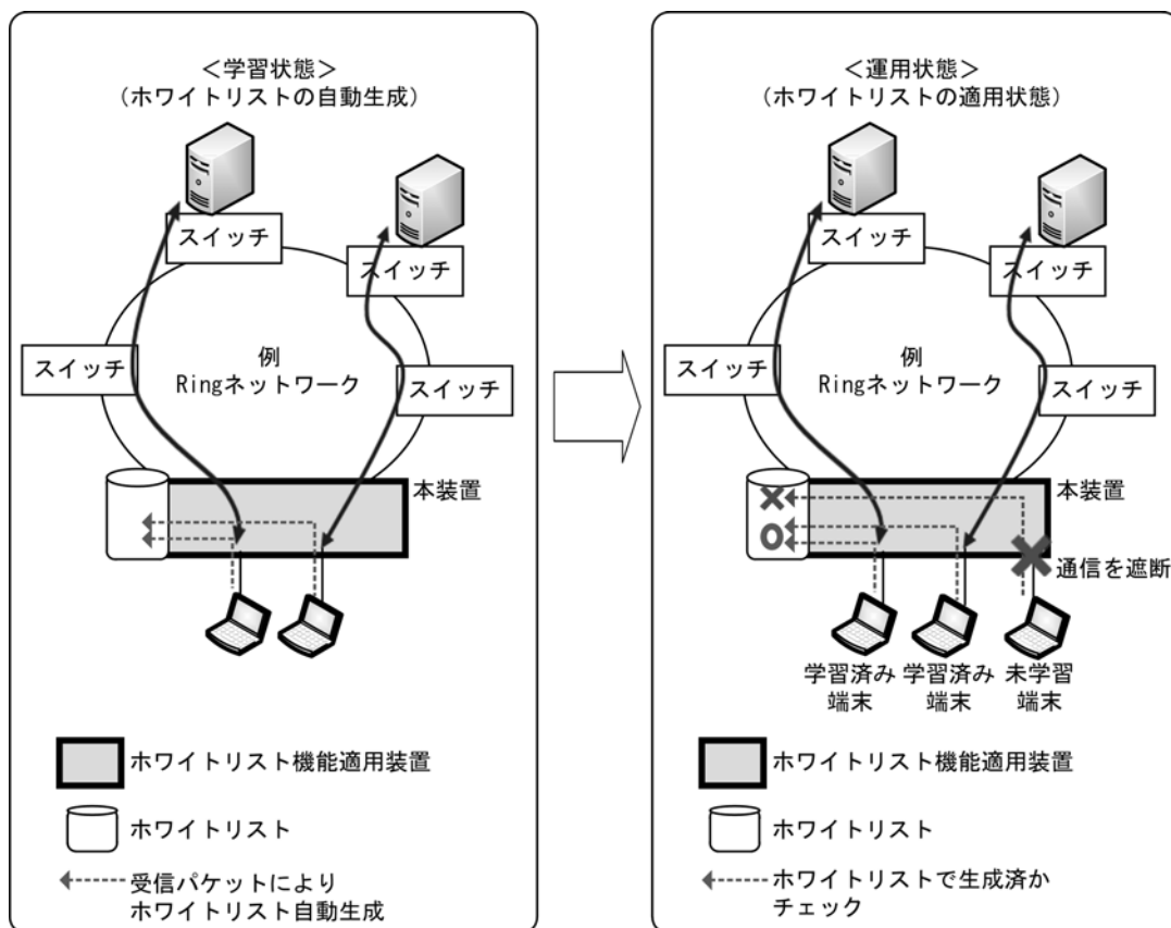
図 14-1 ホワイトリスト機能の概要
