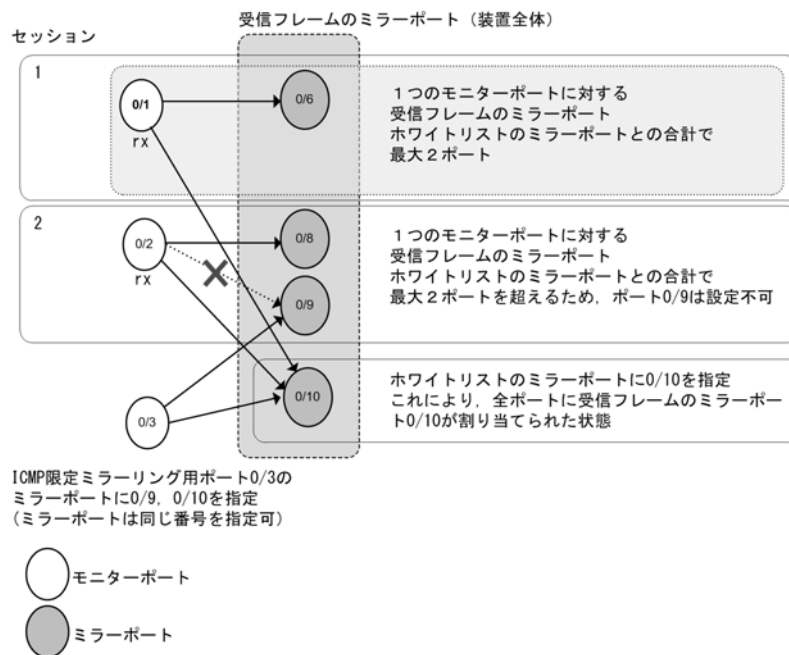
図 26-8 (ホワイトリスト機能, ICMP 限定ミラーリング機能のミラー設定有)
