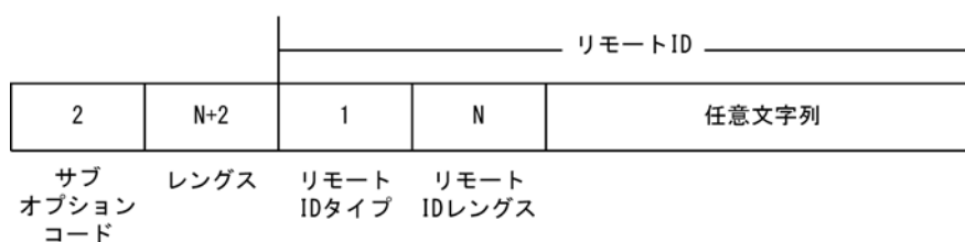
図 13-11 リモート ID タイプ 1 の形式
