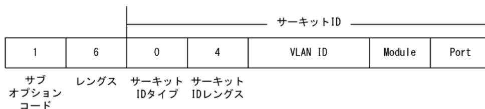
図 13-7 サーキット ID タイプ 0 の形式
