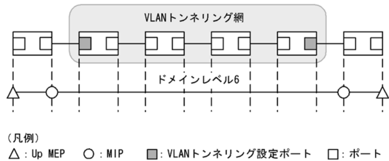
図 21-29 VLAN トンネリング網外だけで CFM を使用する例
