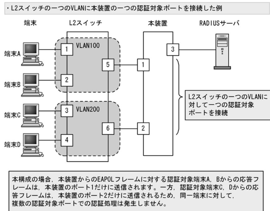
図 6-19 正しい構成例
