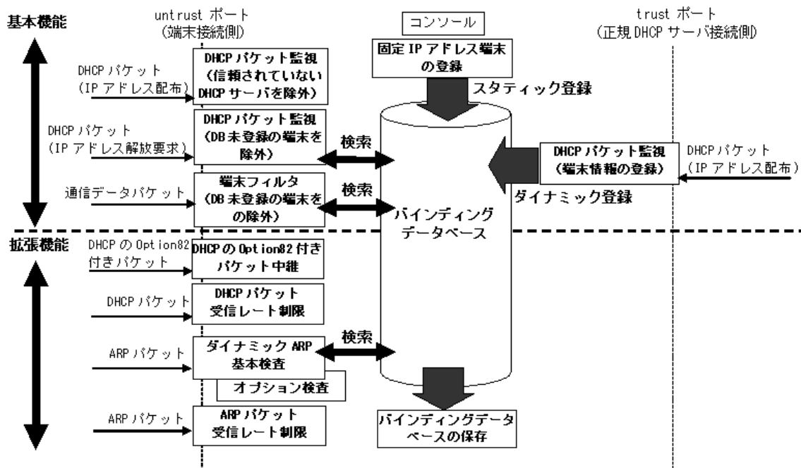
図 13-2 各機能とバインディングデータベースの動作関係図
