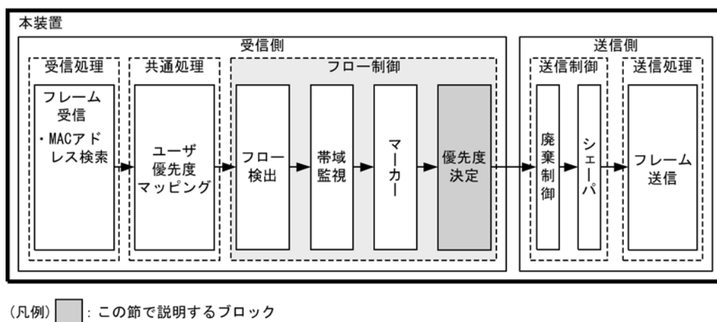
図 3-16 優先度決定の位置づけ
