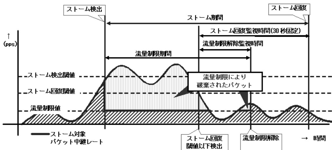
図 18-1 流量制限動作
