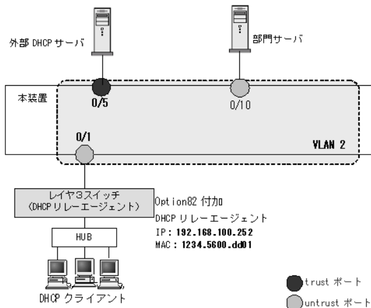
図 13-19 本装置の配下に DHCP リレーエージェントを接続した場合の構成例
