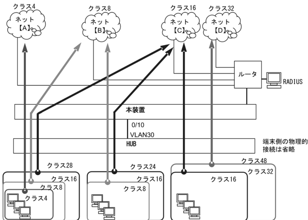
図 5-24 端末が複数クラスに所属する場合の構成例
