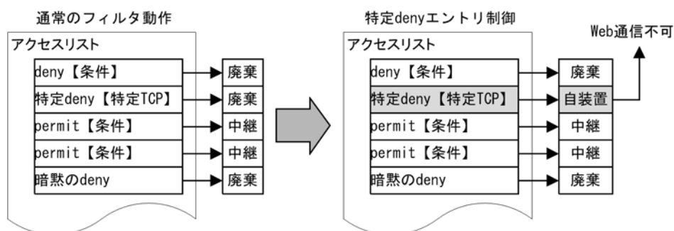
図 15-2 特定 deny エントリ制御
