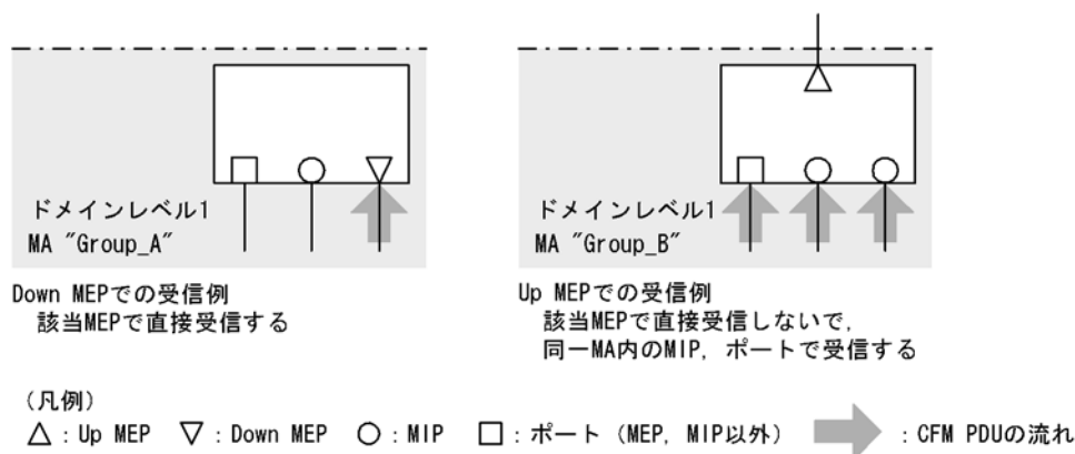
図 21-7 Down MEP, Up MEP での受信
