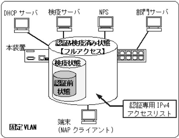
図 6-13 ポート単位認証（静的）での NAP 検疫システム連携概要図
