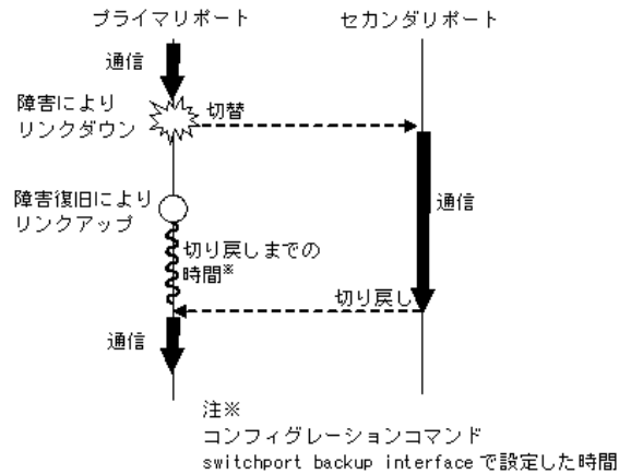
図 17-4 タイマ切り戻し概要
