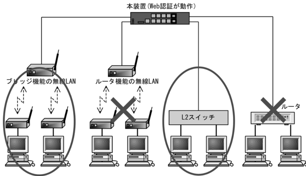
図 8-17 本装置と端末間の接続
