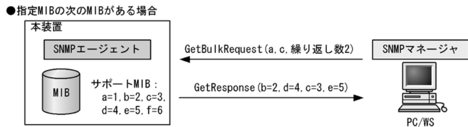
図 22-10 GetBulkRequest オペレーション
