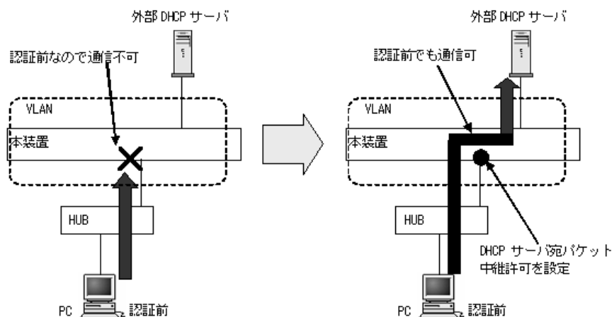
図 5-16 認証専用 IPv4 アクセスリストの使用前と使用後
