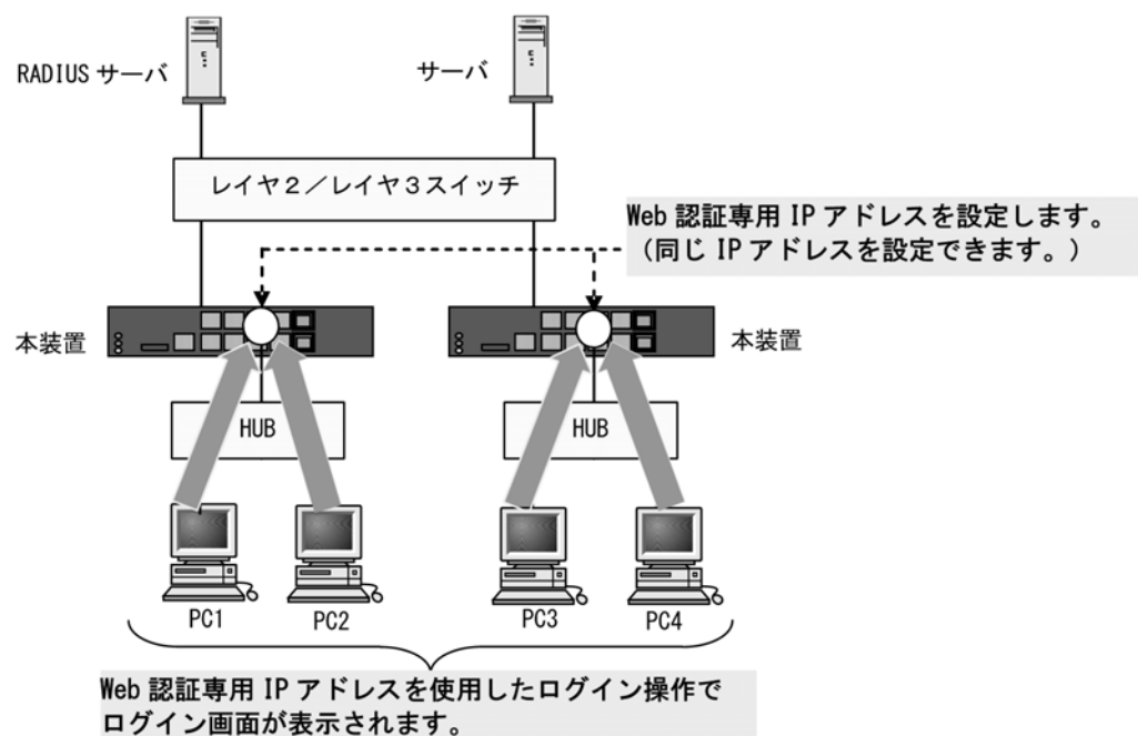
図 8-3 Web 認証専用 IP アドレスによるログイン操作
