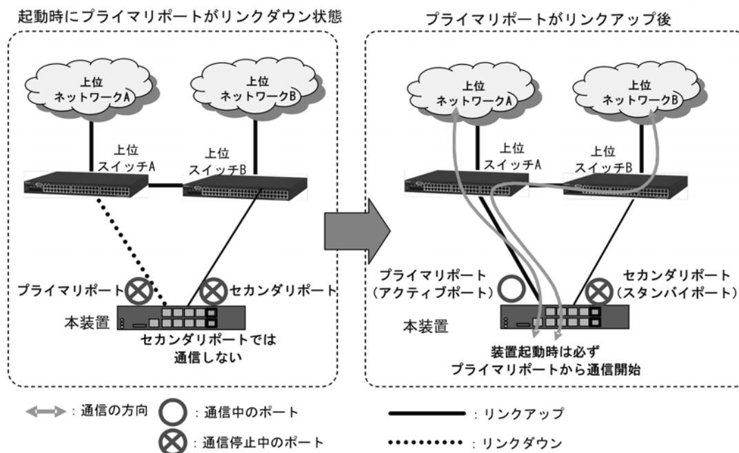
図 17-7 装置起動時のアクティブポート固定機能有効時の動作
