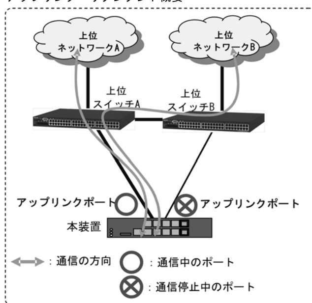
図 17-1 アップリンク・リダンダント概要
