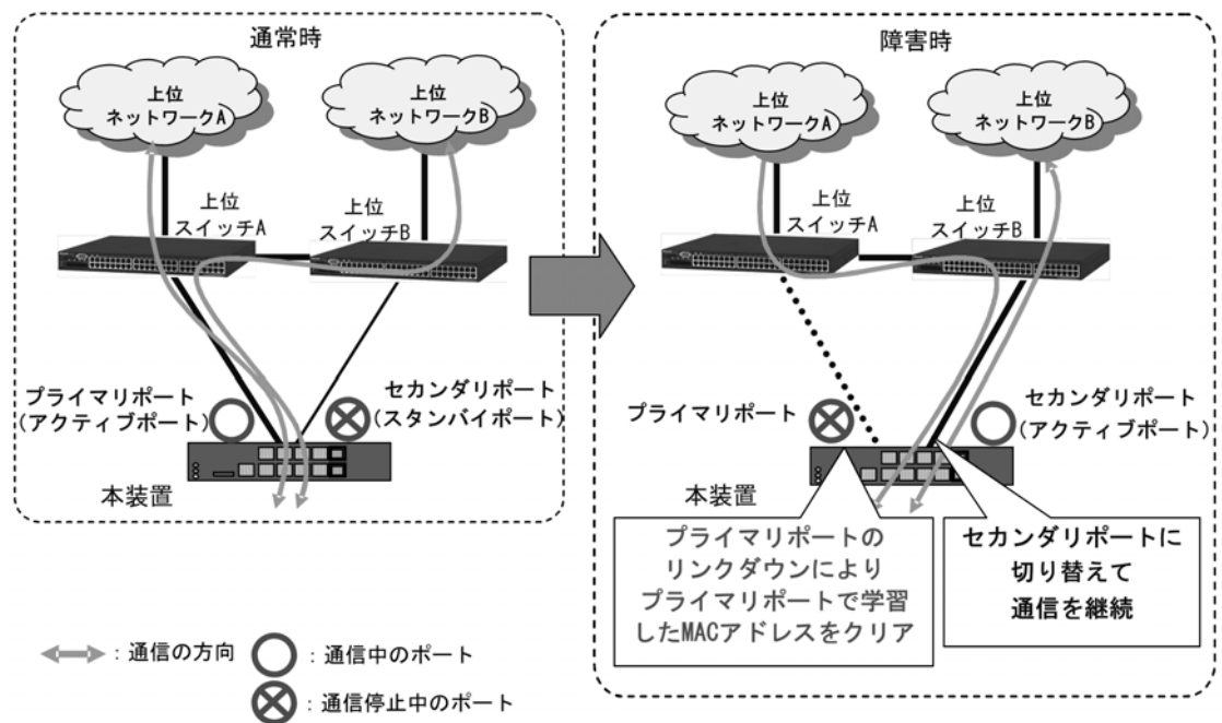
図 17-3 プライマリ・セカンダリ切り替え概要
