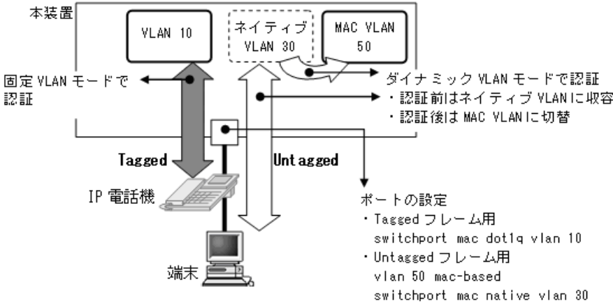
図 5-17 MAC ポートに dot1q vlan を設定したときの動作
