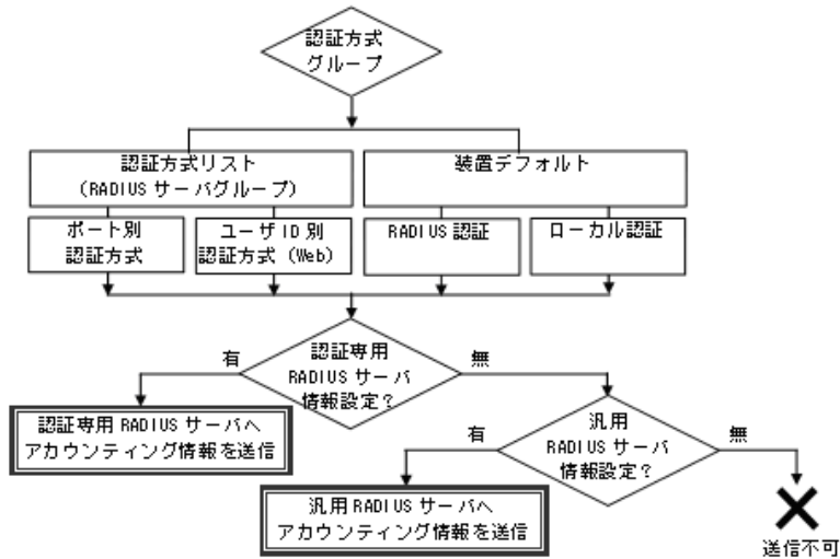
図 5-15 アカウンティング情報の送信先 RADIUS サーバの選択
