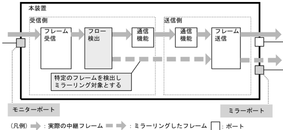
図 27-1 受信フレームに対するポリシーベースミラーリングの動作
