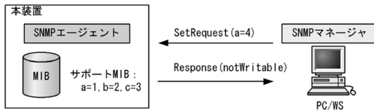
図 22-20 MIB 変数が読み出し専用の場合の SetRequest オペレーション
