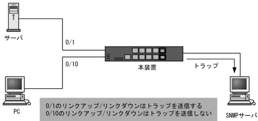
図 22-25 リンクトラップの構成図
