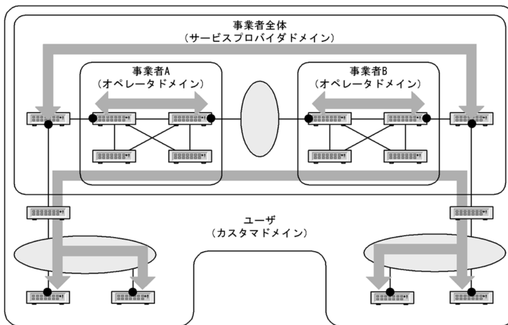
図 21-1 CFM の構成例
