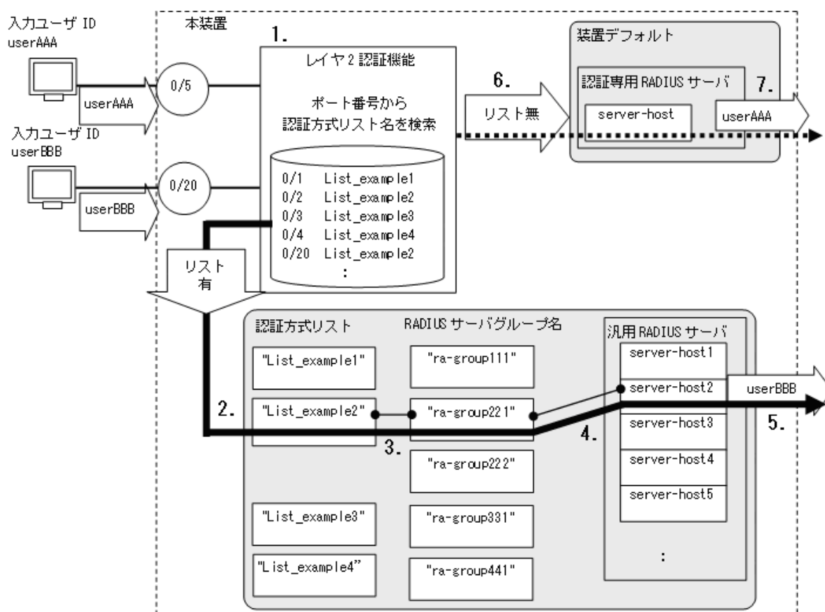
図 5-5 ポート別認証方式の動作概要
