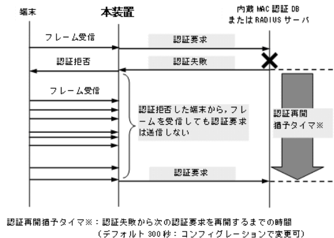
図 10-3 認証再開猶予タイマ概要
