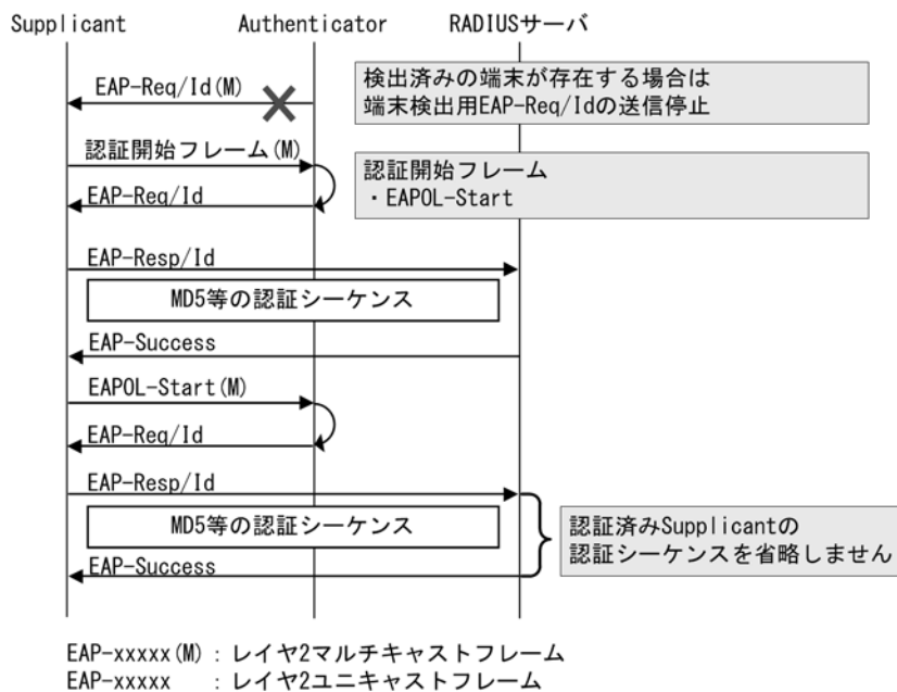
図 6-9 disable の EAP-Request/Identity のシーケンス
