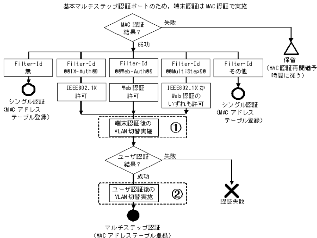
図 12-2 基本マルチステップ認証ポートの認証動作
