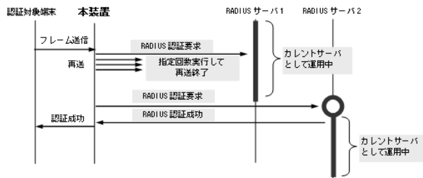
図 5-10 RADIUS サーバ選択のシーケンス
