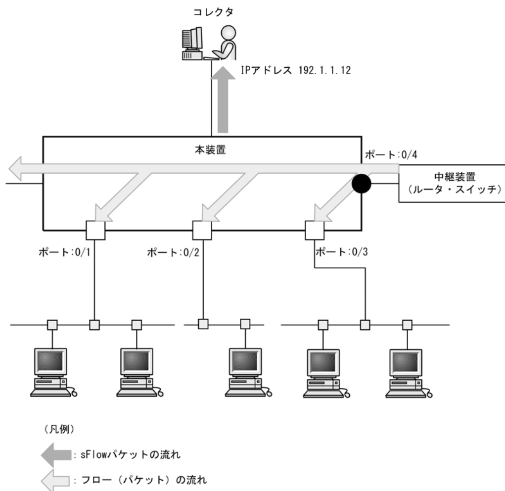
図 24-7 ポート 0/4 の受信パケットをモニタする設定例
