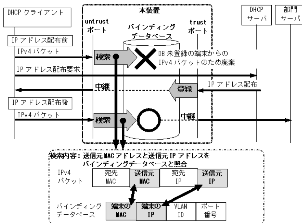
図 13-5 端末フィルタの動作概要（送信元 IP アドレスと送信元 MAC アドレスの端末フィルタ例）
