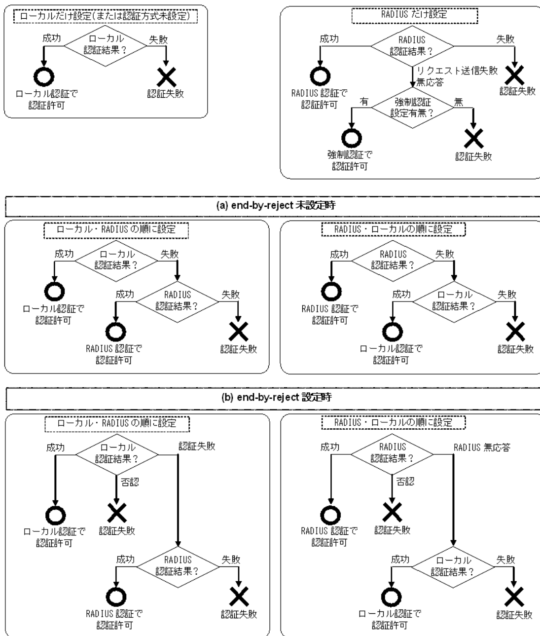
図 5-14 認証方式の設定種別と認証結果の関連
