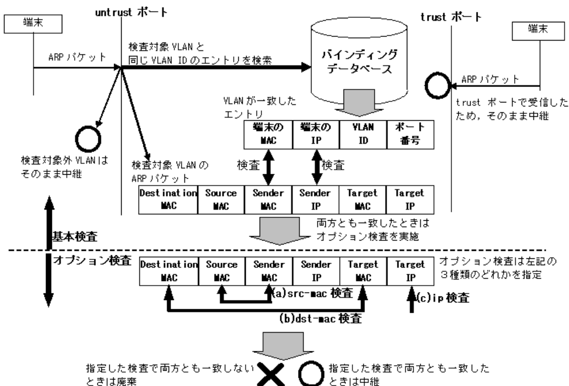
図 13-14 ダイナミック ARP 検査の基本検査とオプション検査の関係
