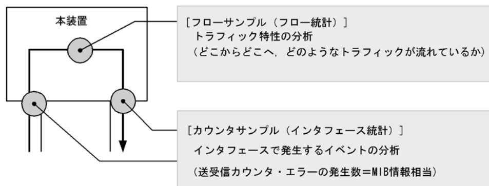
図 24-3 フローサンプルとカウンタサンプル
