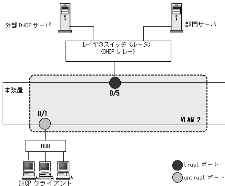
図 13-17 レイヤ3スイッチ経由の構成例
