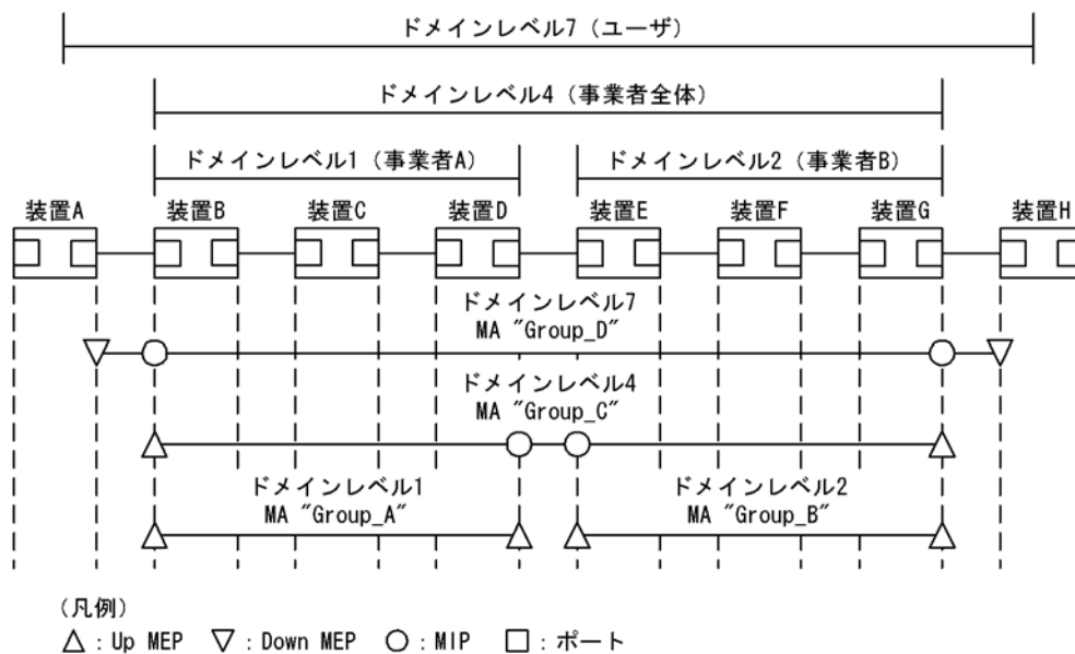
図 21-15 ドメインレベル7の設定
