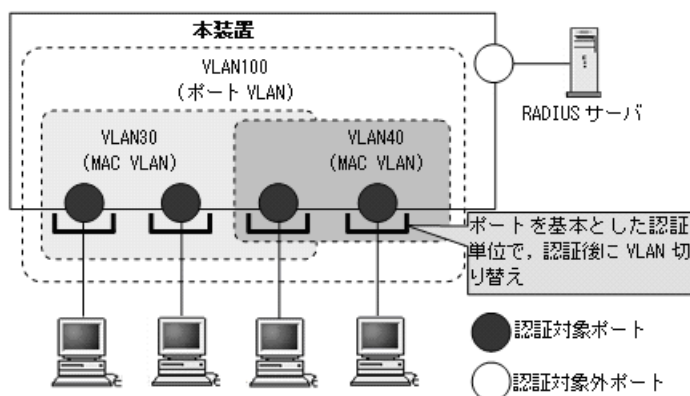
図 6-14 ポート単位認証（動的）の構成例
