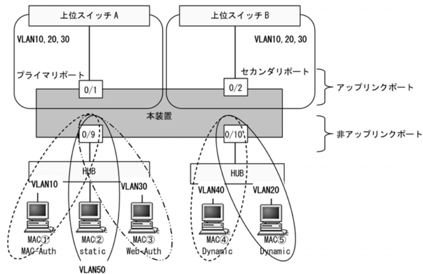
図 17-6 MAC アドレス送信対象例
