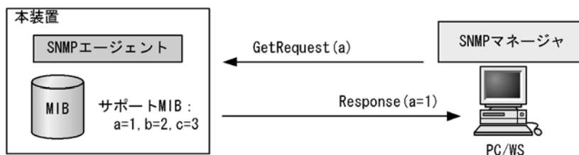
図 22-16 GetRequest オペレーション
