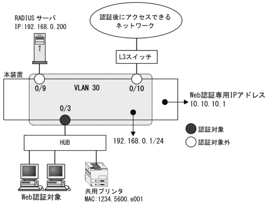
図 9-4 固定 VLAN モードの構成例
