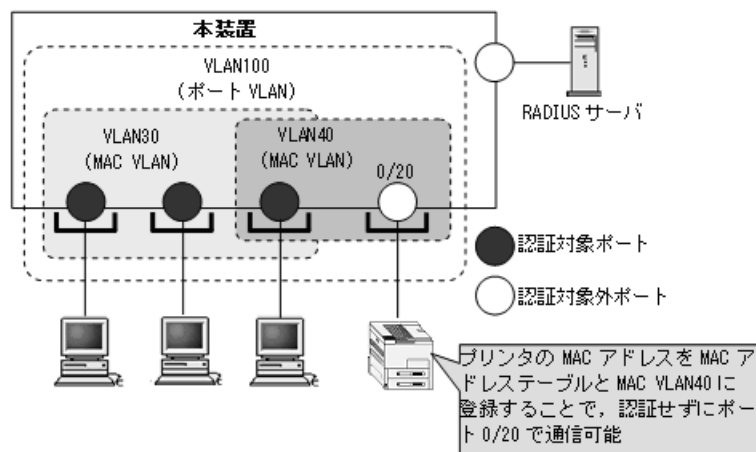
図 6-16 ポート単位認証（動的）での認証除外端末構成例
