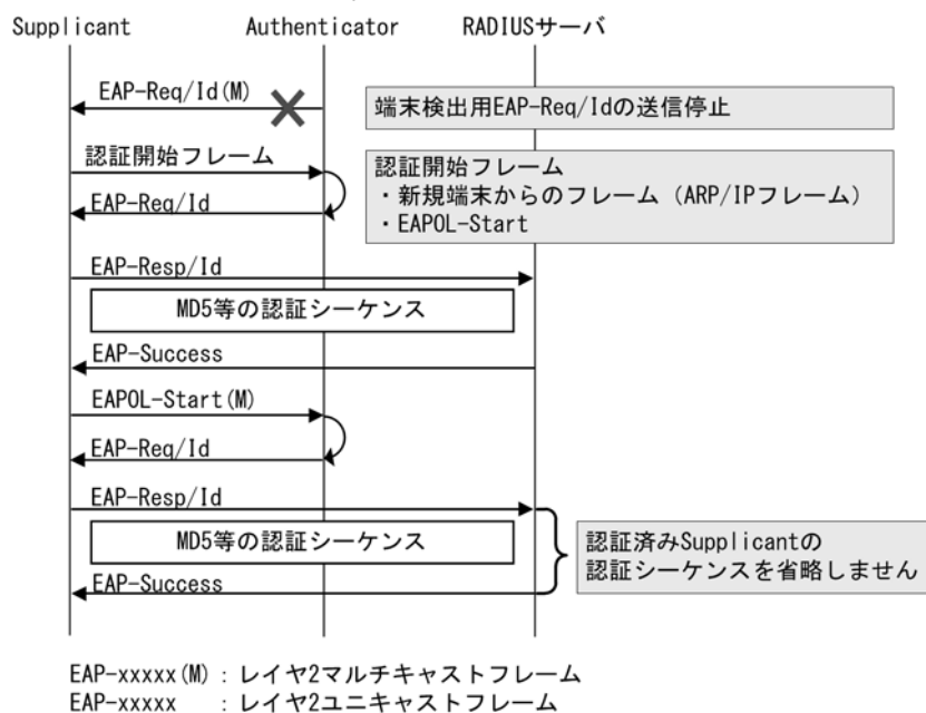
図 6-7 auto の EAP-Request/Identity のシーケンス
