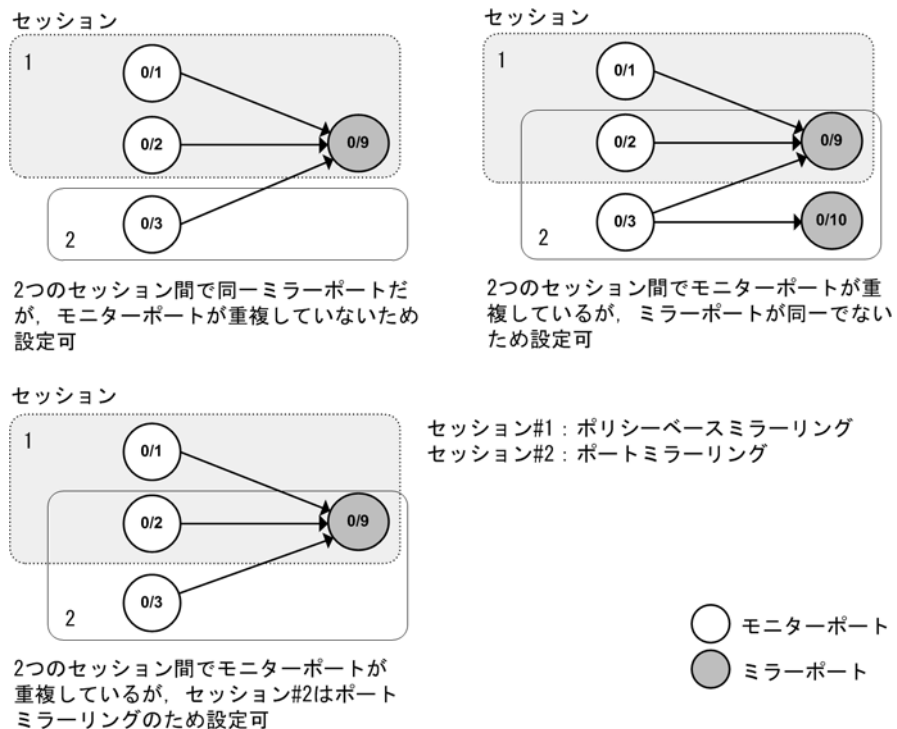
図 27-3 設定可能な組み合わせ
