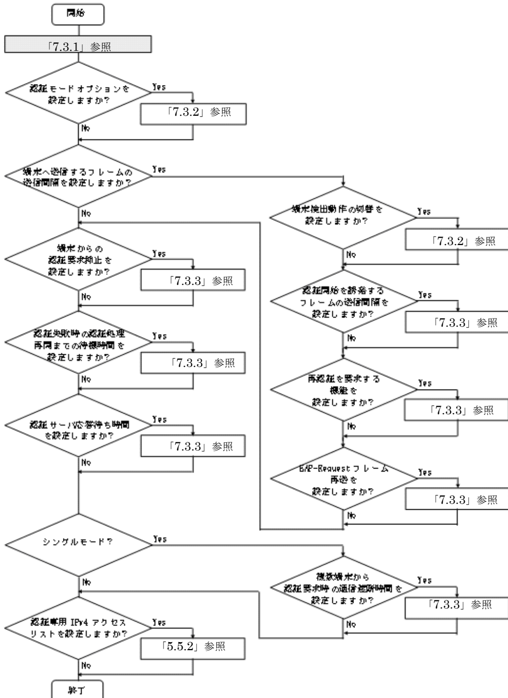
図 7-2 ポート単位認証（静的）の設定手順
