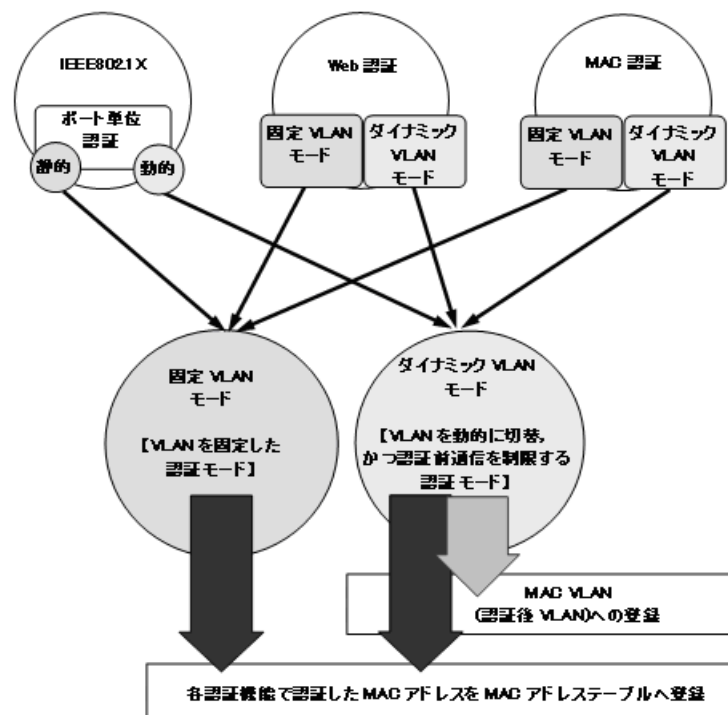
図 5-1 各認証機能と認証モードの対応図
