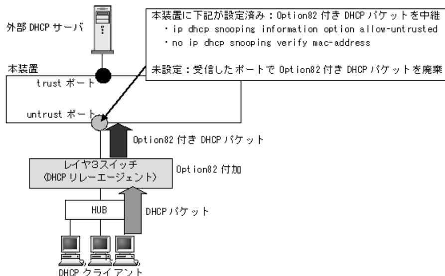
図 13-6 Option82 付きパケットが付加される構成例
