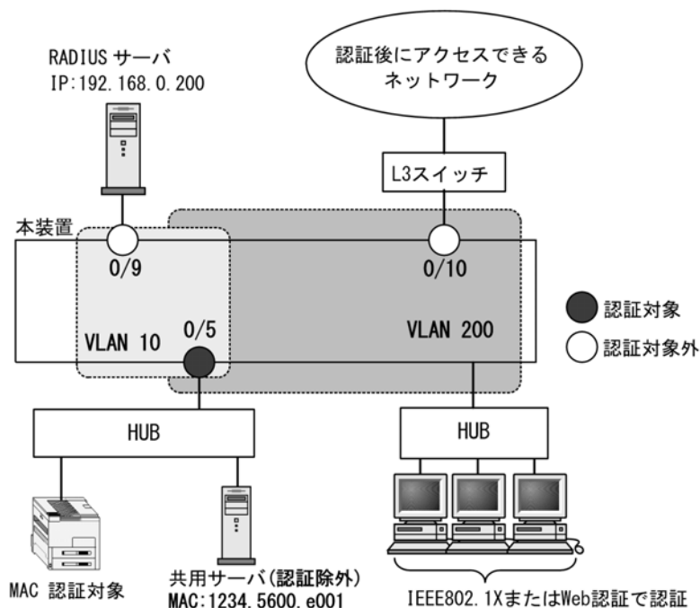
図 11-8 ダイナミック VLAN モードの認証除外の構成例
