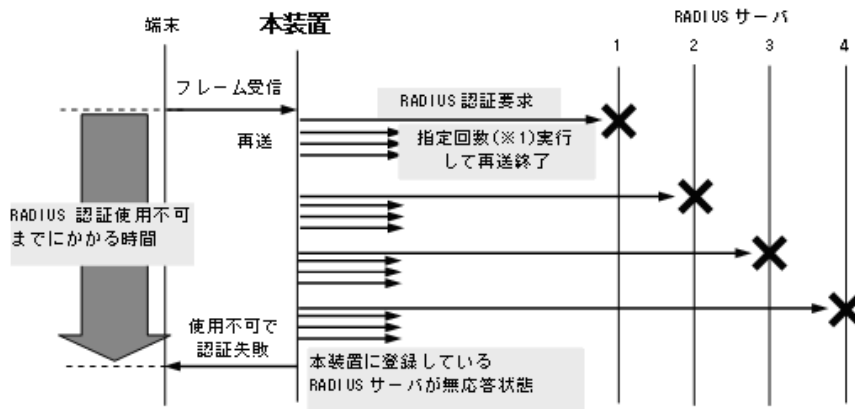
図 5-11 RADIUS 認証使用不可までのシーケンス（RADIUS サーバ最大数設定時）
