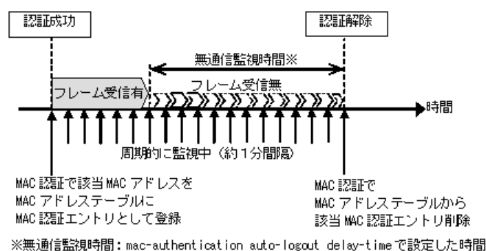
図 10-5 認証済み端末の無通信監視概要
