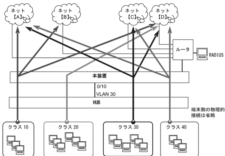
図 5-23 端末が 1 クラスに所属する場合の構成例
