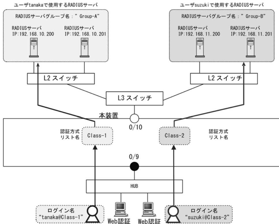
図 5-8 ユーザ ID 別認証方式構成図例
