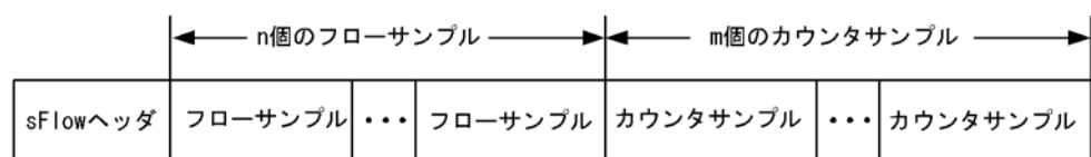
図 24-4 sFlow パケットフォーマット
