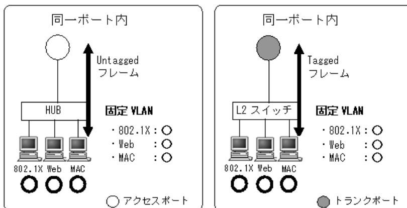
図 5-26 同一ポート内固定 VLAN モードの共存例
