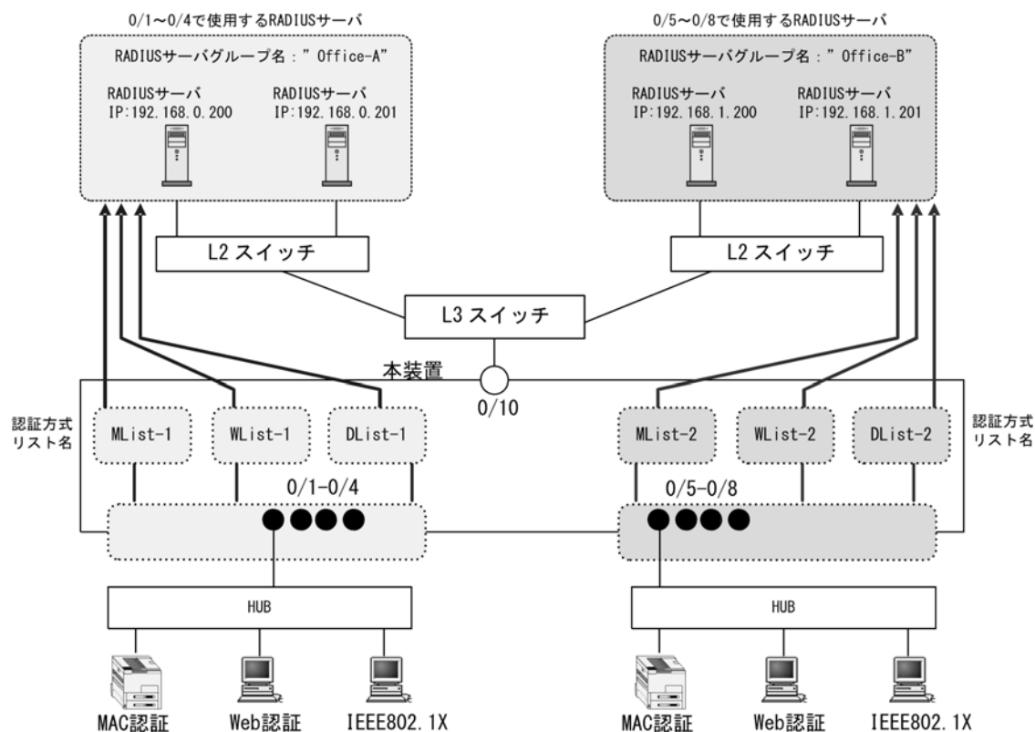
図 5-7 ポート別認証方式構成図例
