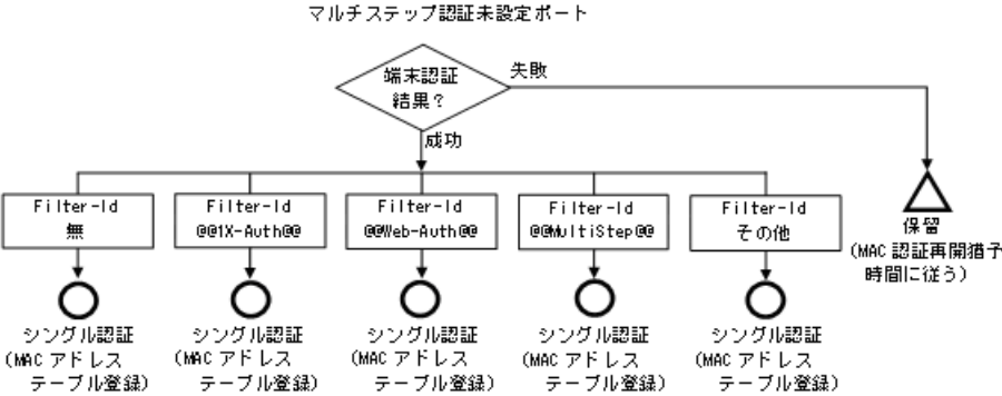
図 12-5 マルチステップ認証未設定ポートの認証動作
