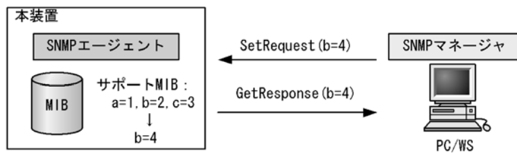
図 22-11 SetRequest オペレーション
