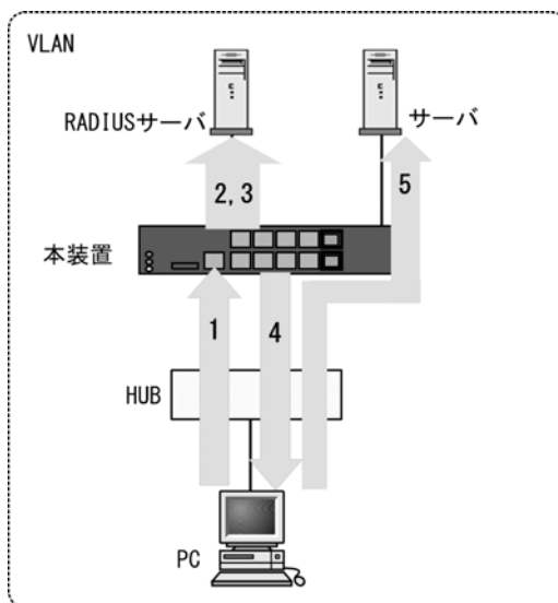
図 8-2 固定 VLAN モード概要図（RADIUS 認証方式）
