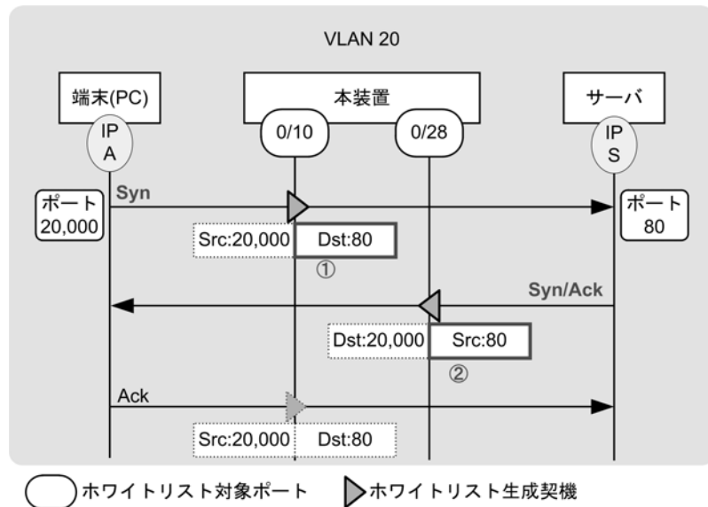
図 14-7 サーバ側ポート番号指定時の例
