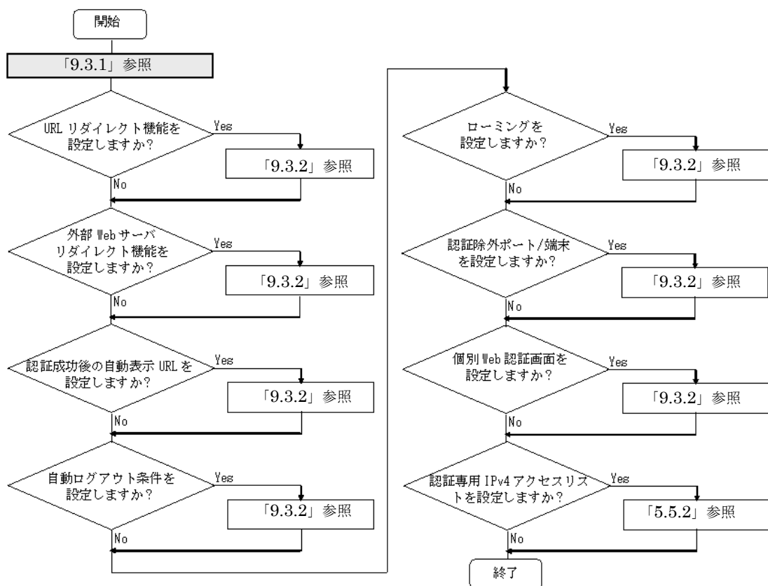
図 9-3 固定 VLAN モードの設定手順
