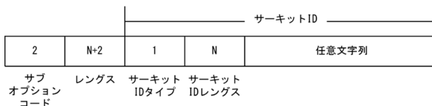
図 13-8 サーキット ID タイプ 1 の形式 (任意文字列)
