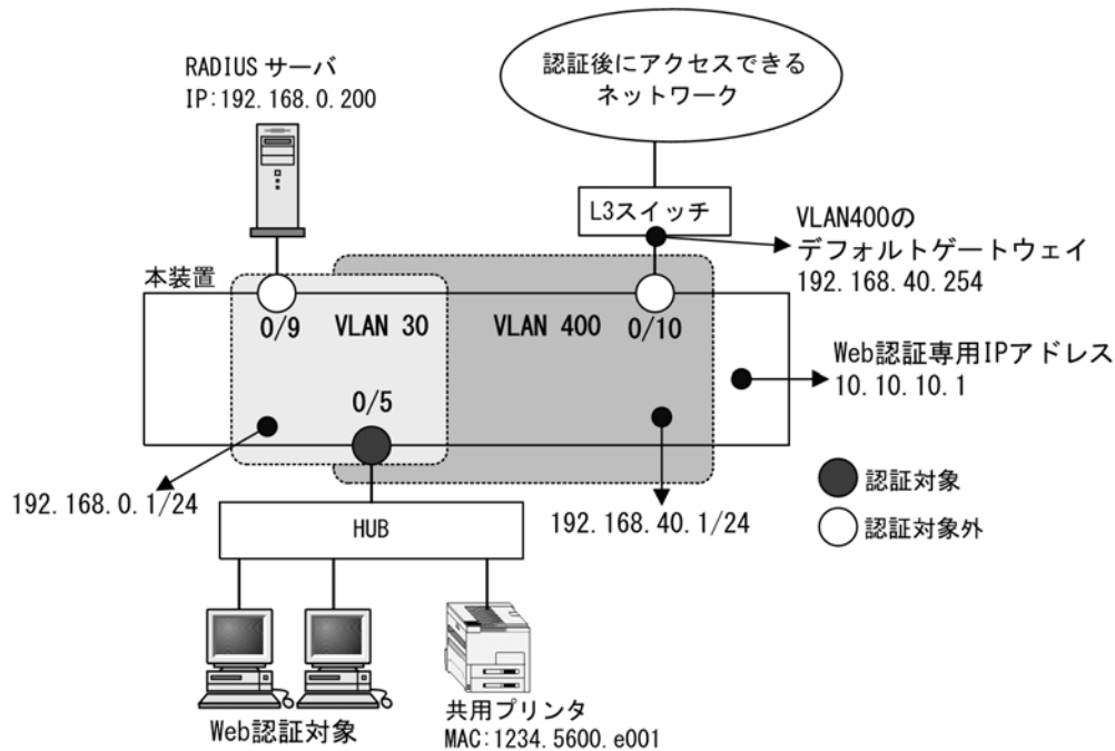
図 9-7 ダイナミック VLAN モードの構成例
