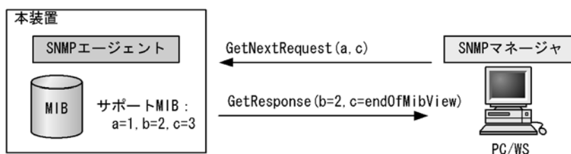
図 22-9 GetNextRequest オペレーション (SNMPv2C)
