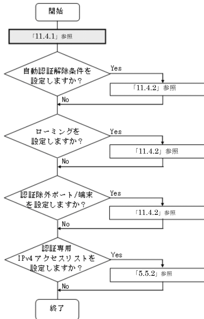
図 11-6 ダイナミック VLAN モードの設定手順
