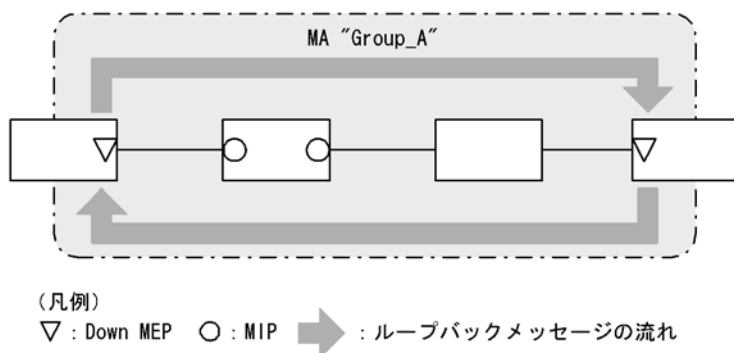
図 21-22 MEP に対して Loopback を実行
