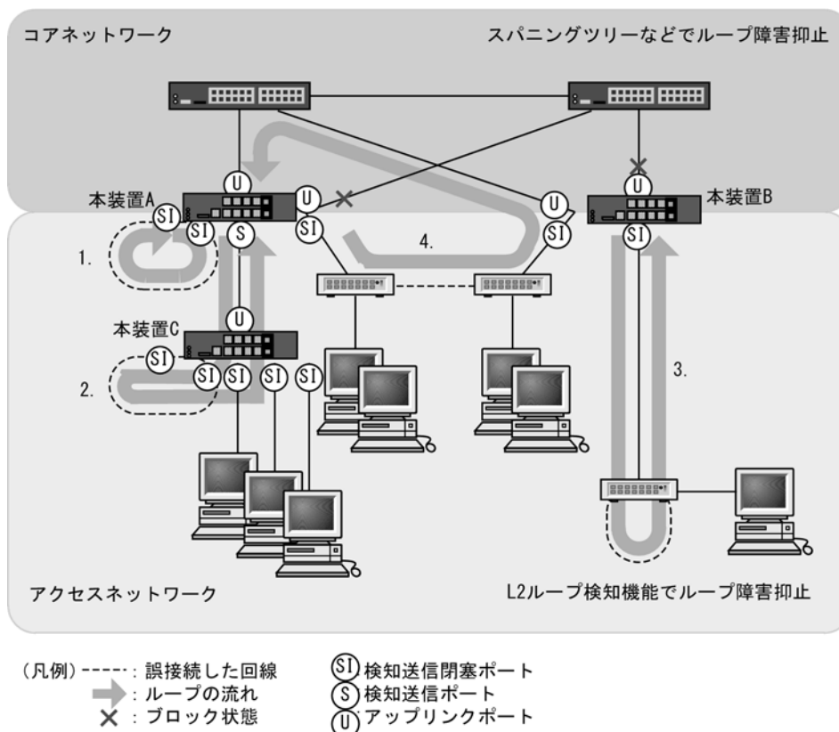
図 20-2 L2 ループ検知機能を適用したネットワーク構成例
