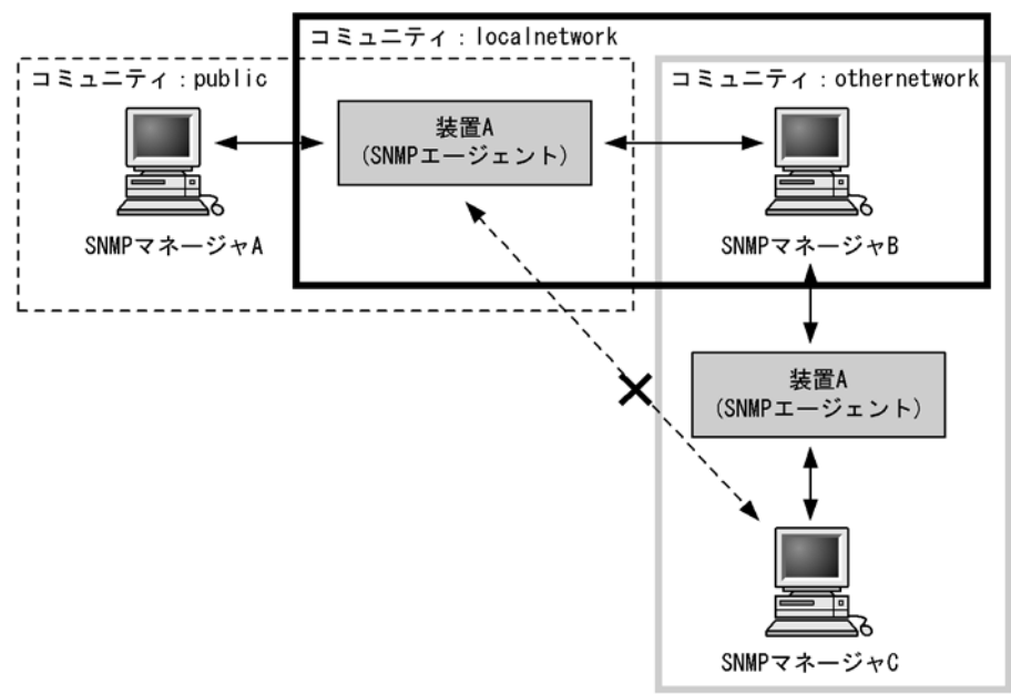
図 22-15 コミュニティによるオペレーション
