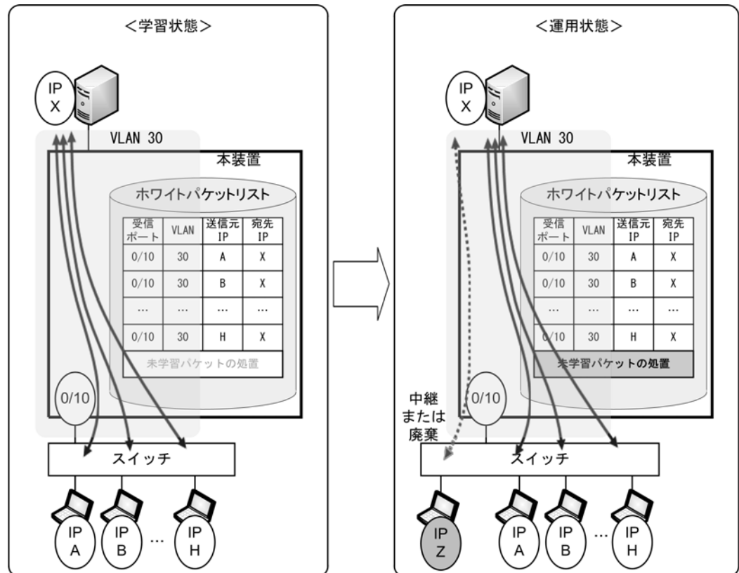
図 14-5 ホワイトパケットリスト機能の概要
