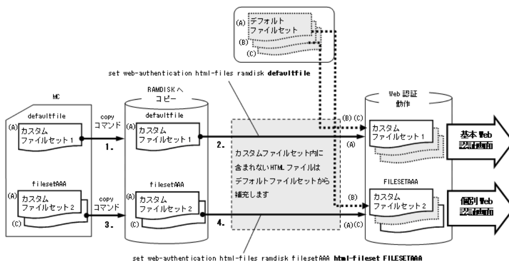
図 8-18 カスタムファイルセット登録手順
