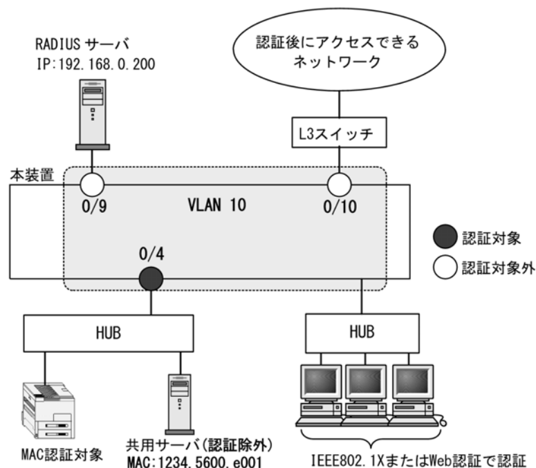
図 11-5 固定 VLAN モードの認証除外の構成例
