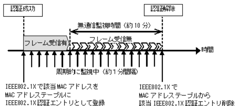
図 6-11 認証済み端末の無通信監視概要
