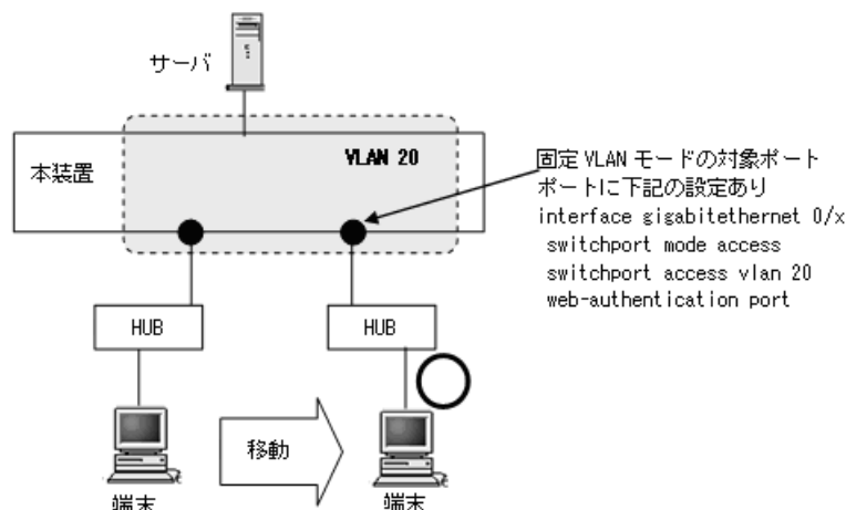
図 8-5 固定 VLAN モード ローミング概要図
