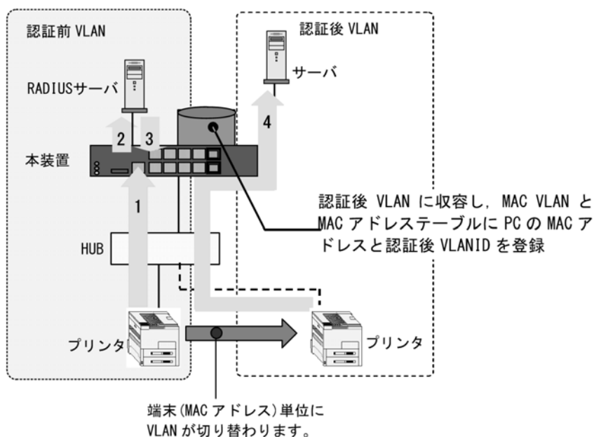
図 10-8 ダイナミック VLAN モード概要図（RADIUS 認証方式）
