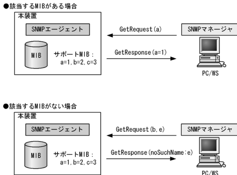
図 22-6 GetRequest オペレーション
