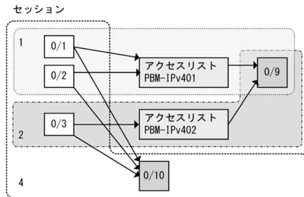
図 27-6 ポートミラーリングと併用
