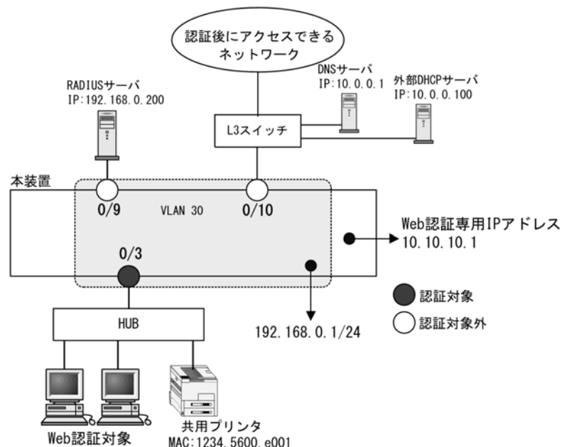
図 5-21 認証専用 IPv4 アクセスリストの使用例
