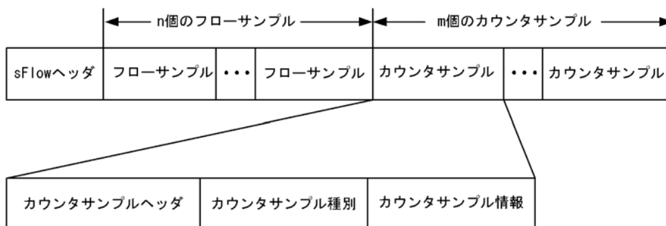
図 24-6 カウンタサンプルのフォーマット
