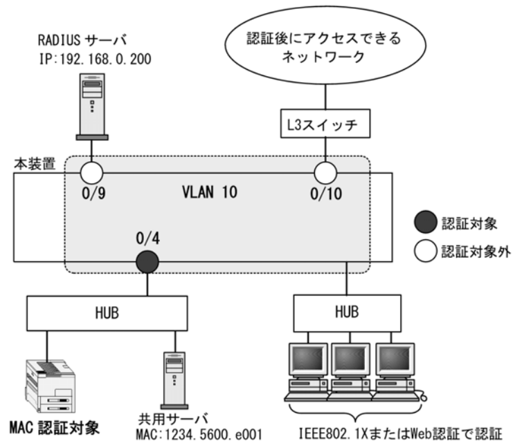
図 11-4 固定 VLAN モードの構成例
