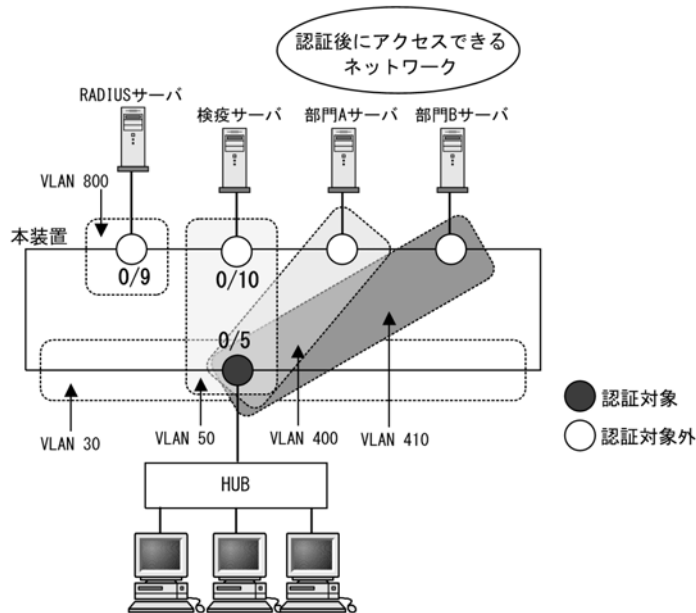
図 5-22 ダイナミック VLAN モードの VLAN 名称指定の使用例
