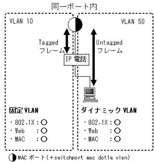
図 5-28 同一ポート内ダイナミック VLAN モードと固定 VLAN モードの共存例
