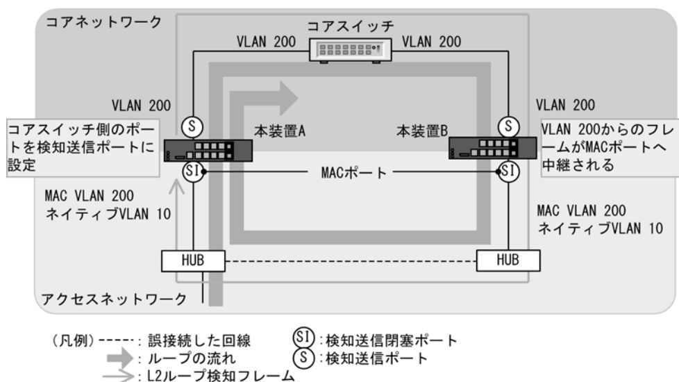
図 20-4 ループ検知可能な構成
