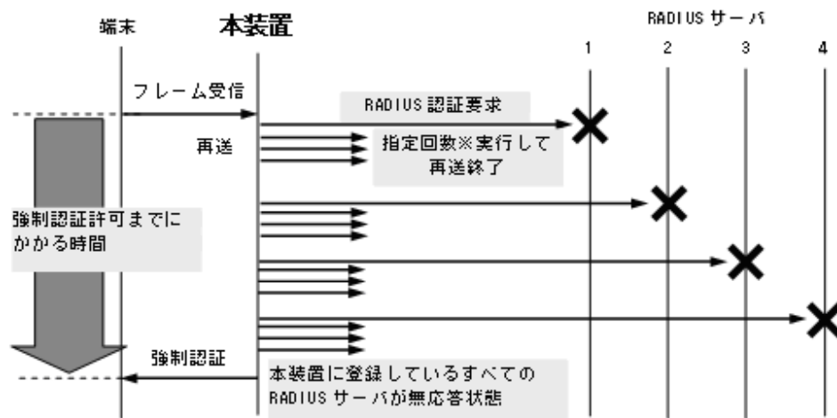
図 5-18 強制認証許可までのシーケンス（RADIUS サーバ最大数設定時）
