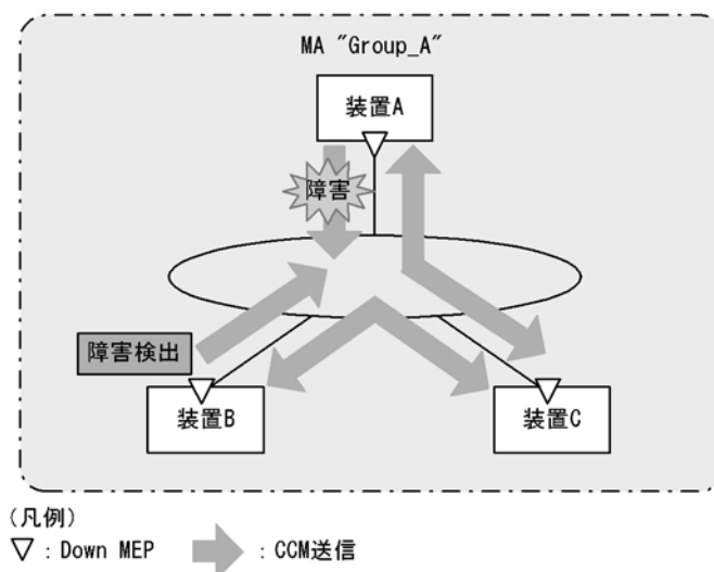
図 21-19 CC で障害を検出
