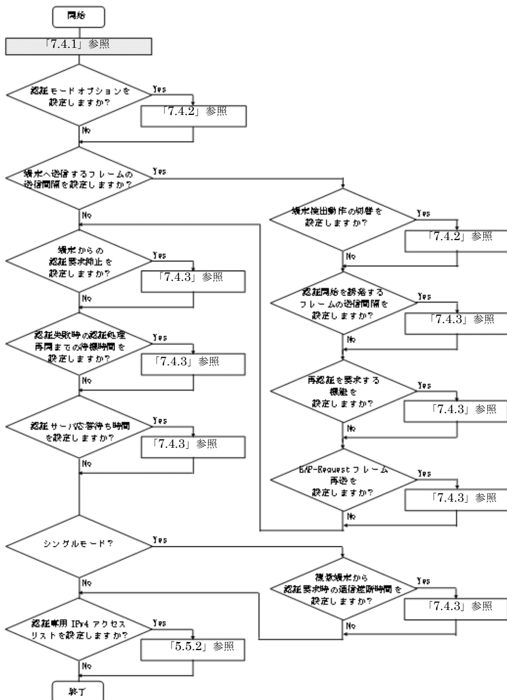
図 7-5 ポート単位認証（動的）の設定手順
