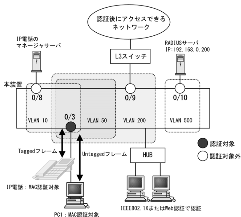
図 5-29 MAC ポートで Tagged フレームを認証する構成例
