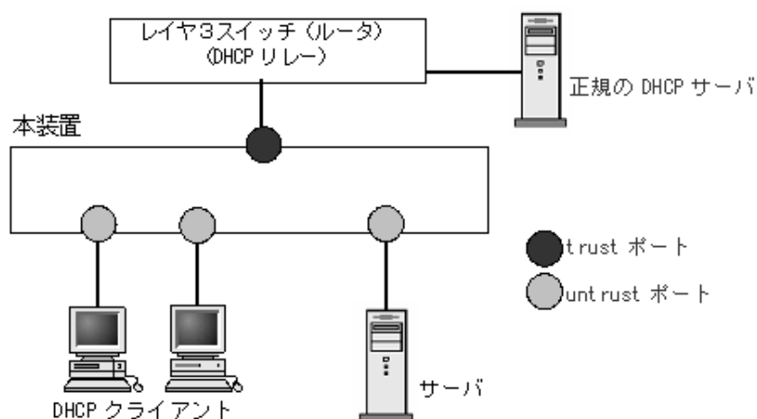
図 13-3 DHCP snooping のポート種別
