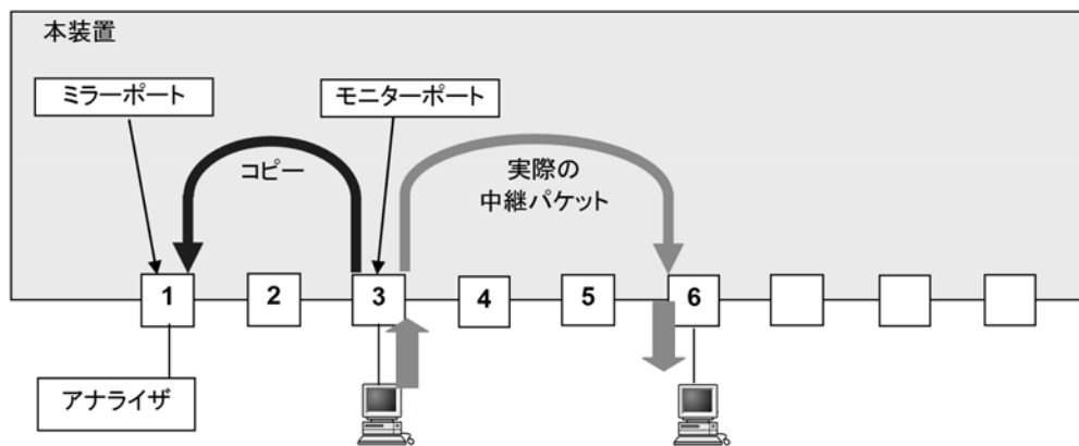
図 26-1 受信フレームのミラーリング
