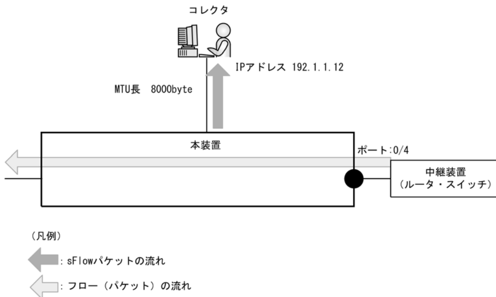
図 24-9 コレクタへの送信を MTU=8000byte に設定する例
