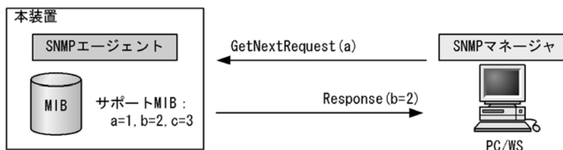
図 22-17 GetNextRequest オペレーション
