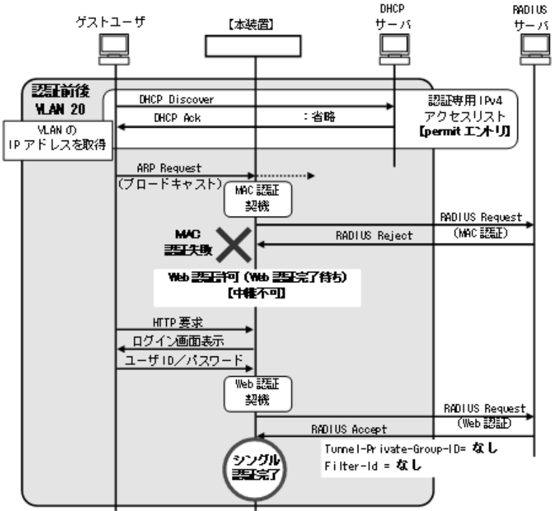
図 12-17 ゲストユーザの認証動作（固定 VLAN モード）
