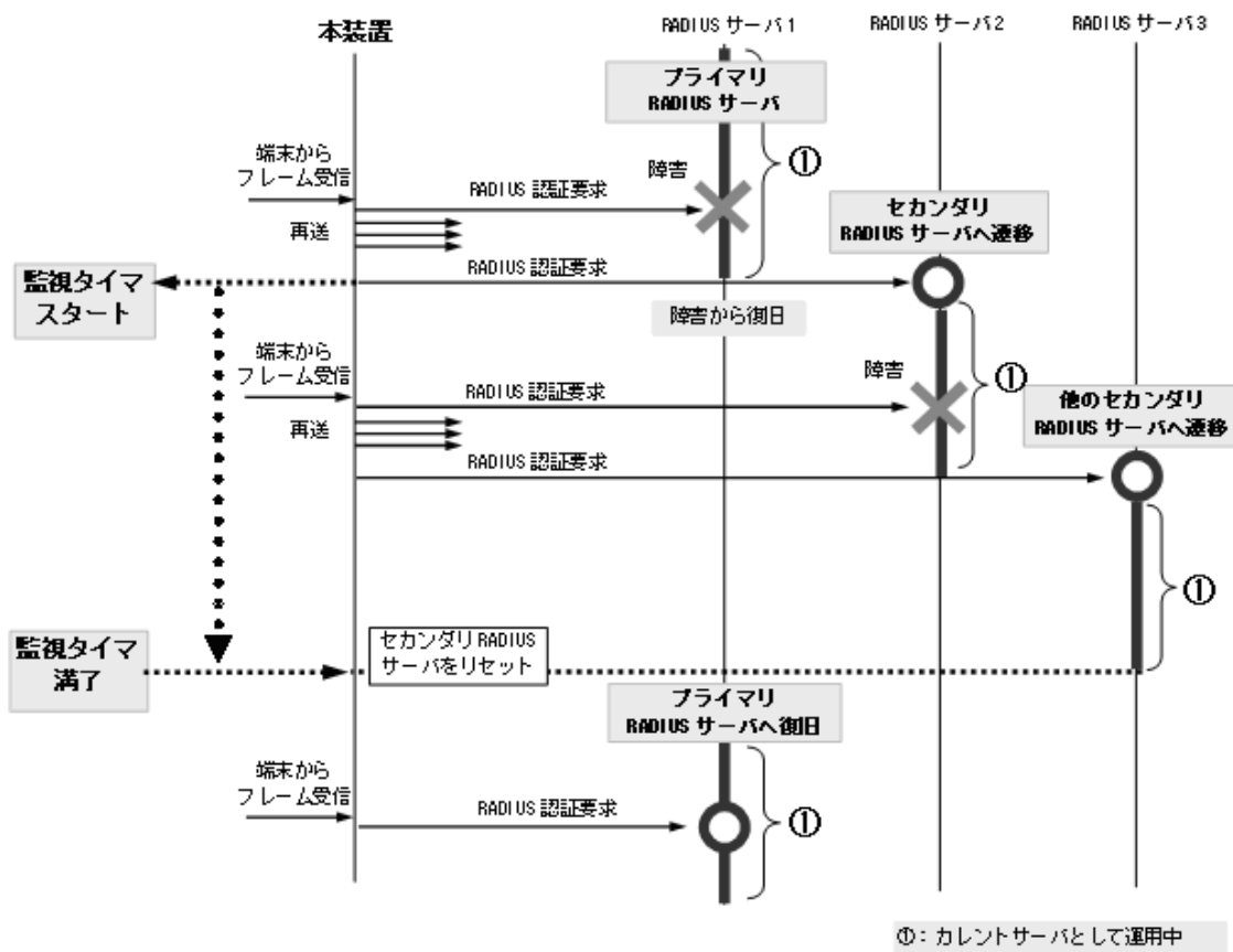
図 5-13 プライマリ RADIUS サーバへの復旧シーケンス (2)
