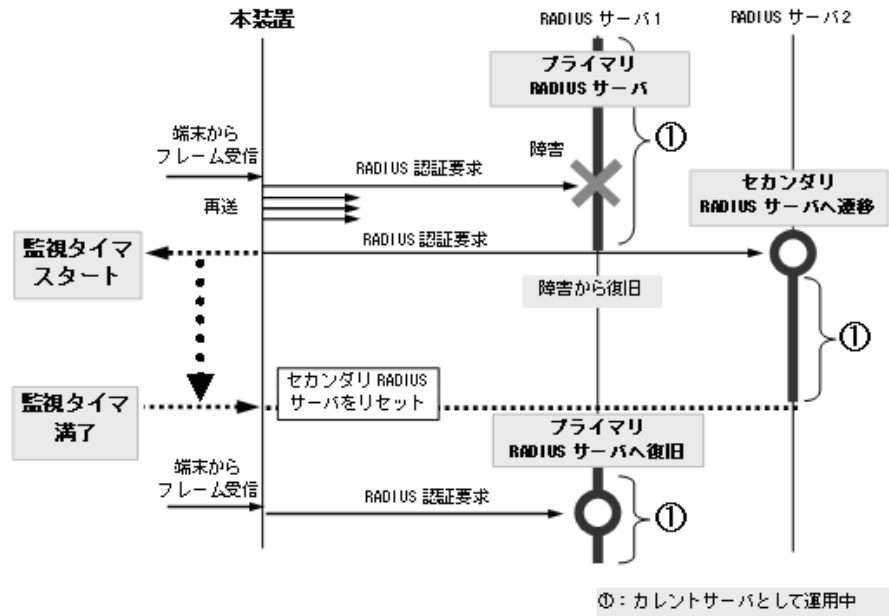
図 5-12 プライマリ RADIUS サーバへの復旧シーケンス (1)
