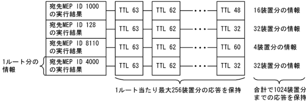
図 21-30 リンクトレースデータベース
