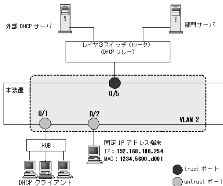
図 13-18 固定 IP アドレス端末を接続した場合の構成例
