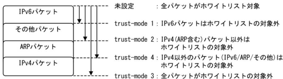
図 14-6 trust モードの対象範囲
