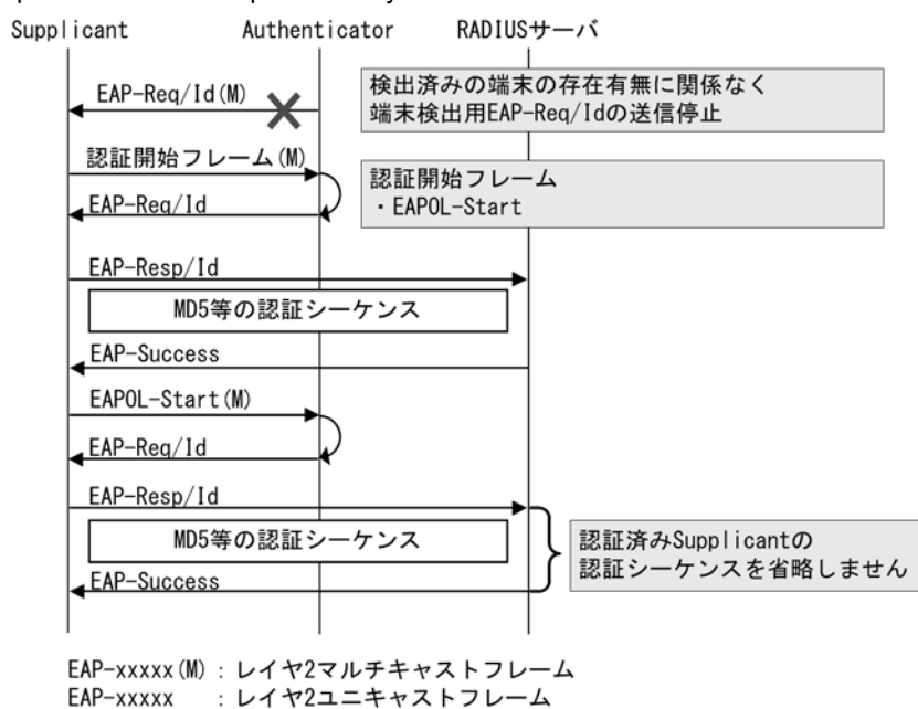
図 6-8 passive の EAP-Request/Identity のシーケンス
