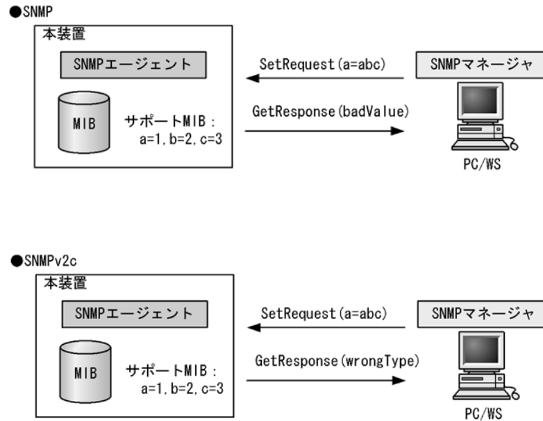
図 22-13 設定値のタイプが正しくない場合の SetRequest オペレーション例
