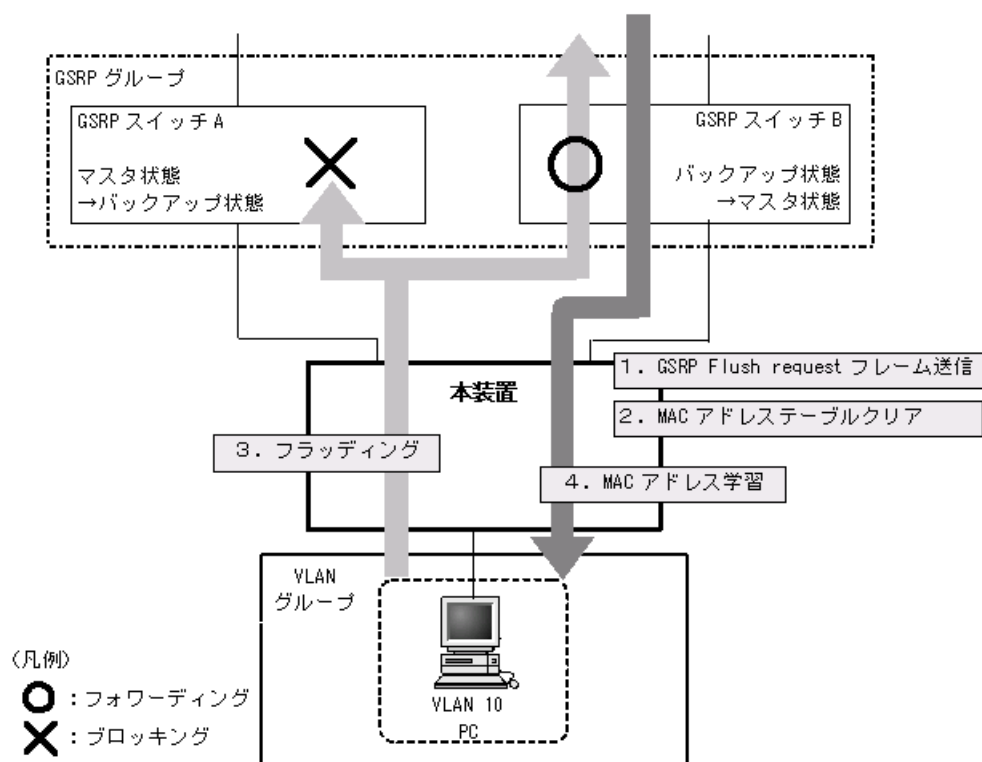
図 16-2 GSRP Flush request フレームによる切り替え制御の概要
