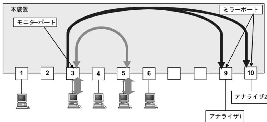
図 26-5 多対 2 のミラーリング
