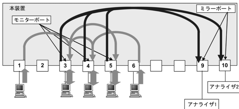
図 26-5 多対 2 のミラーリング
