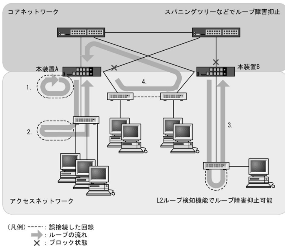
図 20-1 ループ障害の発生例
