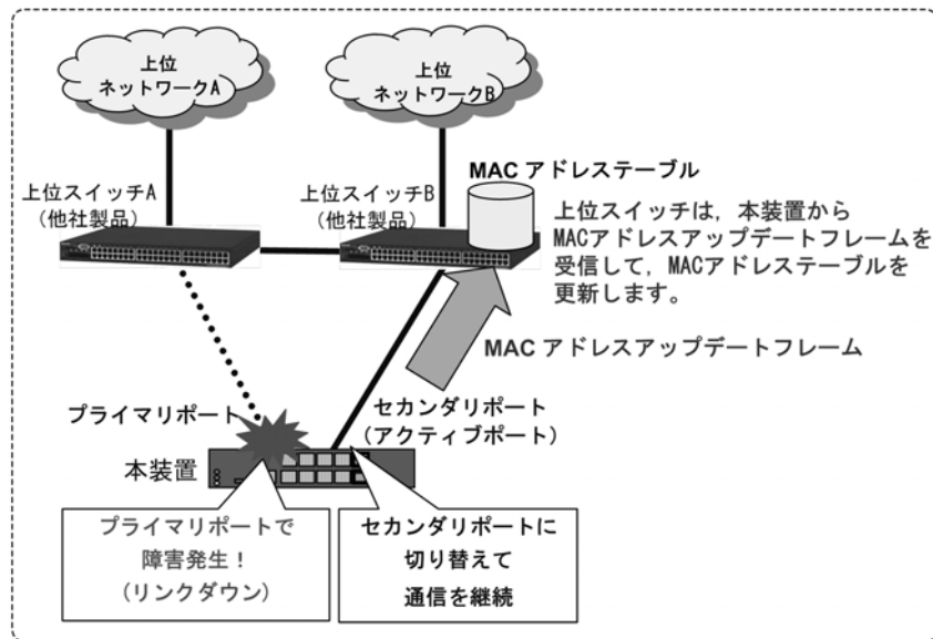
図 17-5 MAC アドレスアップデート機能概要
