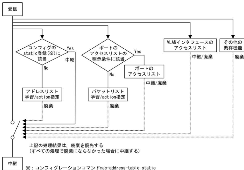
図 14-9 機能併用時の判定イメージと廃棄優先
