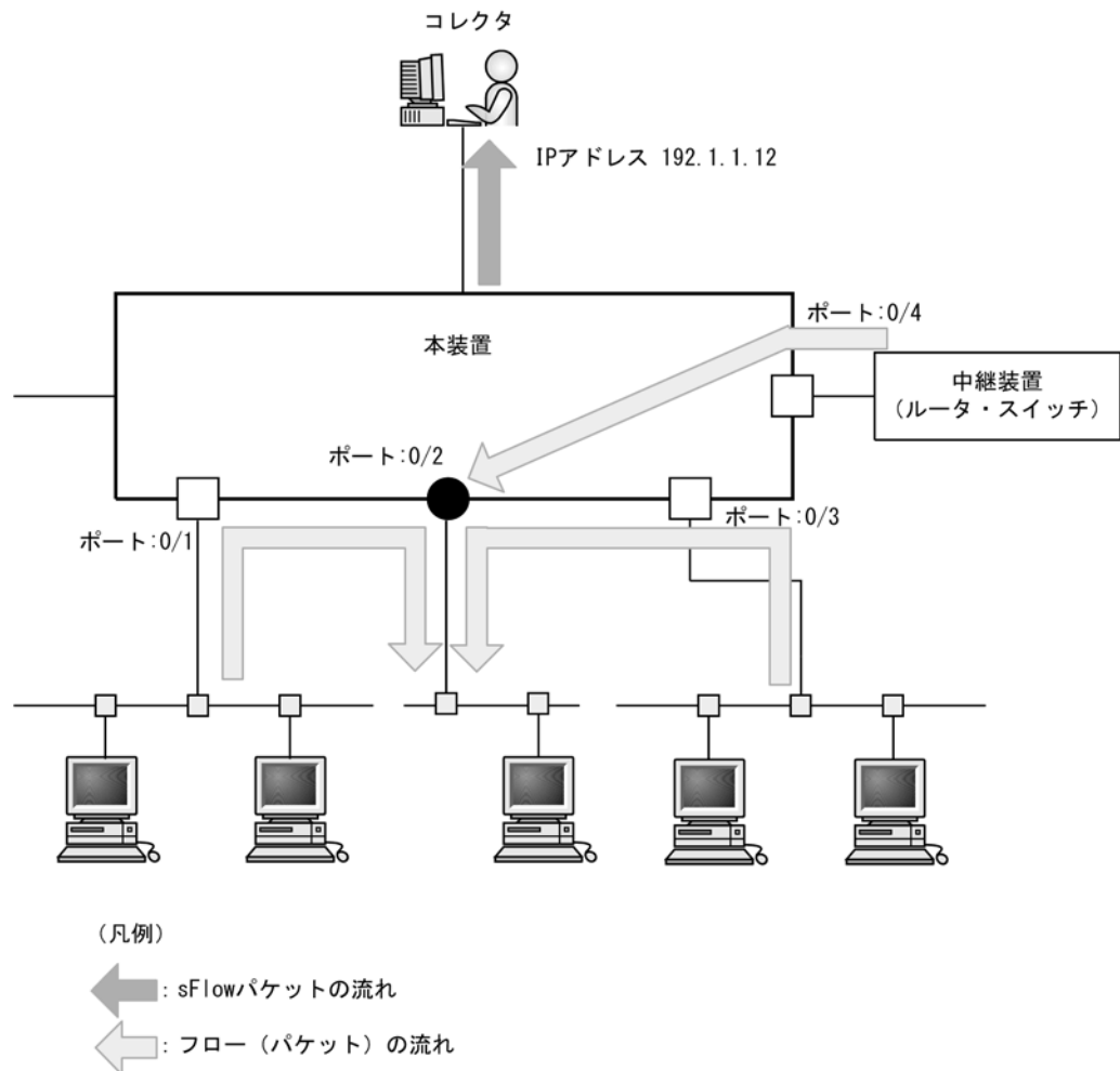
図 24-8 ポート 0/2 の送信パケットをモニタする設定例
