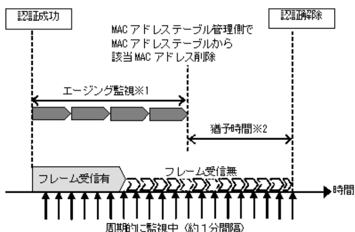
図 6-12 MAC アドレステーブルエイジング監視による解除概要
