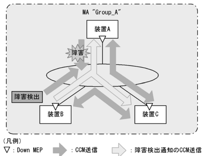
図 21-20 障害を全 MEP に通知
