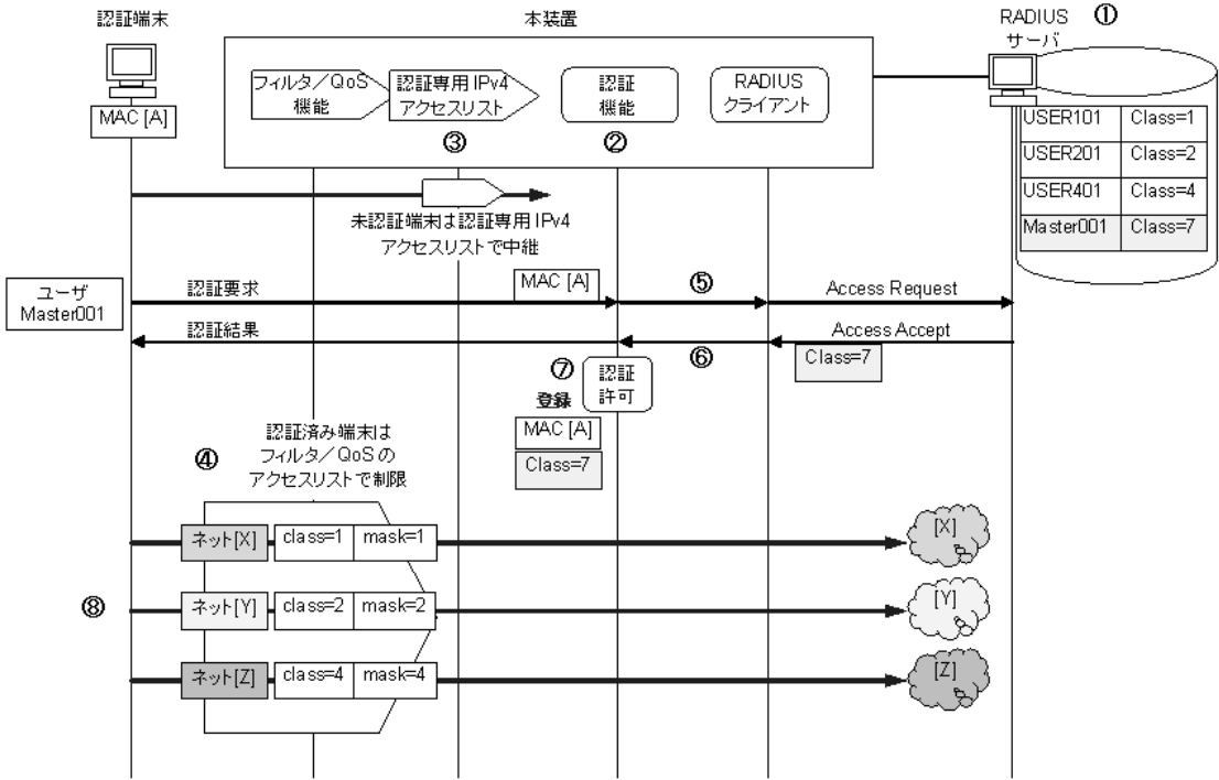
図 5-20 ダイナミック ACL/QoS 機能の動作概要
