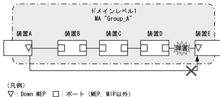
図 21-10 ドメイン内に MIP が設定されていない構成の例
