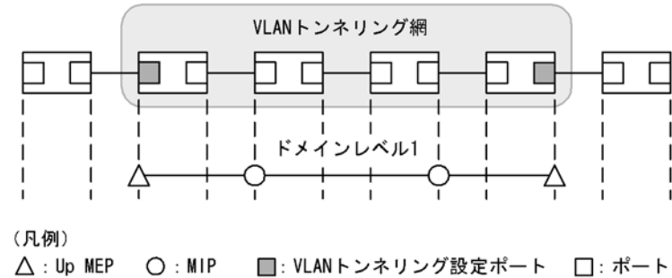
図 21-28 VLAN トンネリング網内だけで CFM を使用する例
