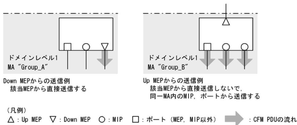
図 21-6 Down MEP, Up MEP からの送信
