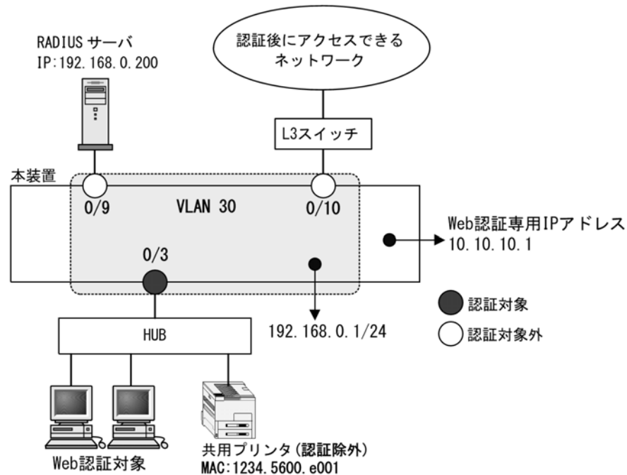
図 9-5 固定 VLAN モードの認証除外の構成例
