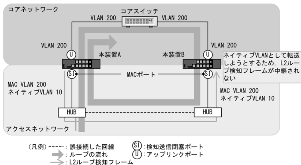
図 20-3 ループ検知の制限となる構成
