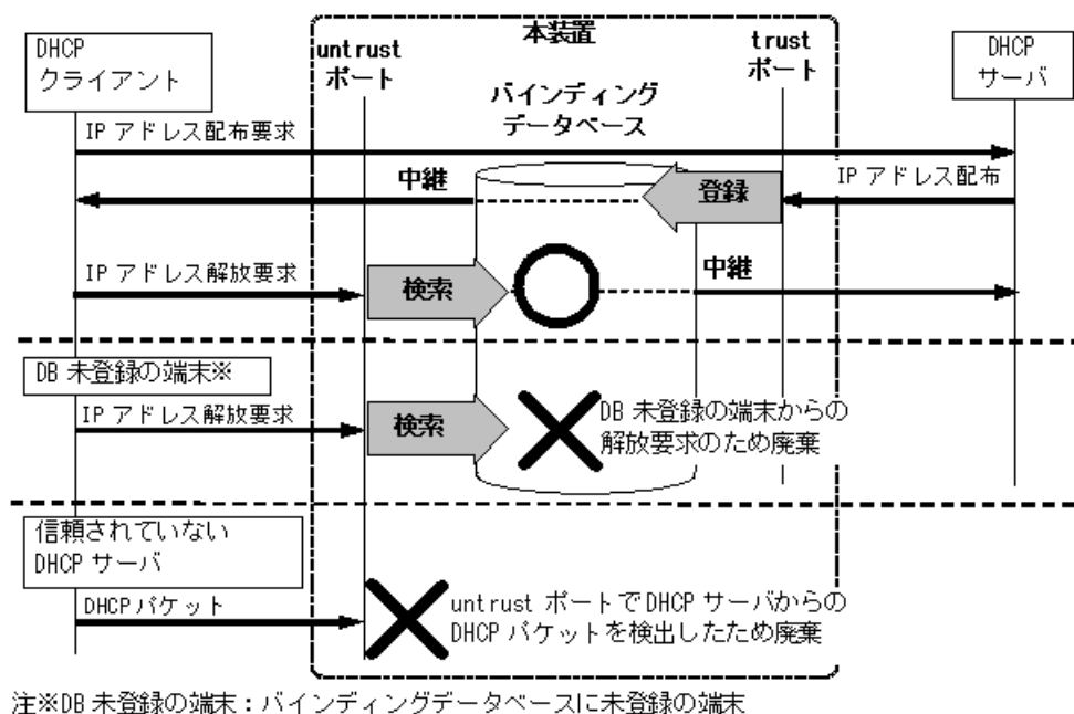
図 13-4 DHCP パケット監視の動作概要
