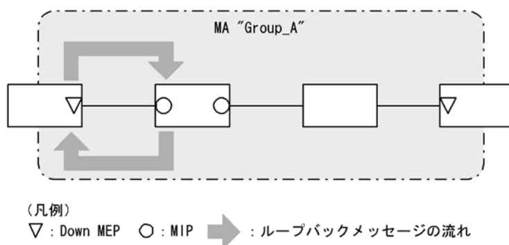
図 21-21 MIP に対して Loopback を実行
