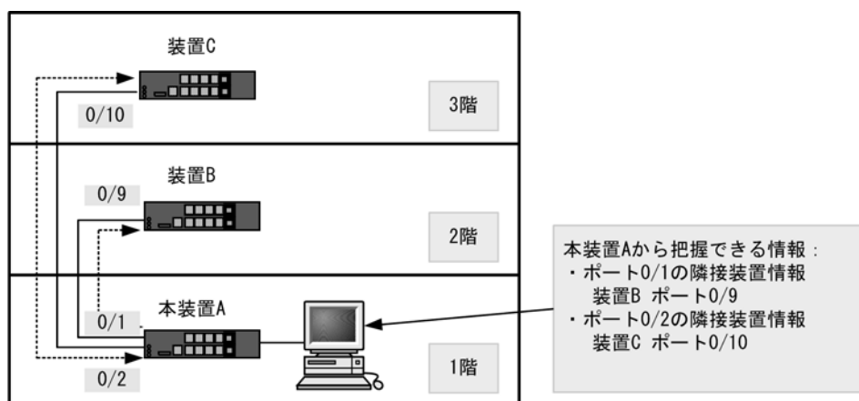
図 25-1 LLDP の適用例
