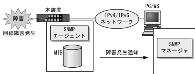
図 22-23 トラップの例
