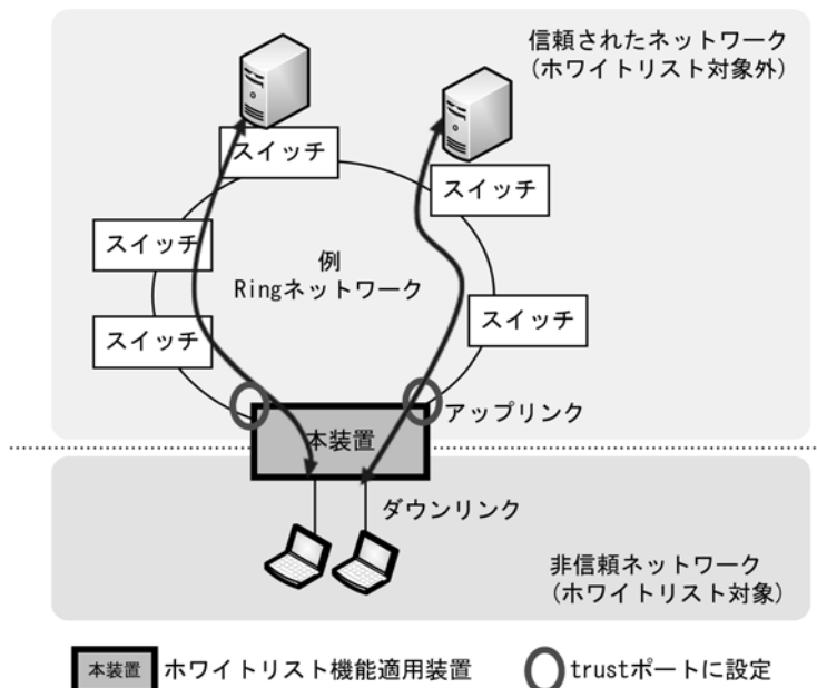
図 14-8 ホワイトリスト機能と Ring ネットワークの併用例
