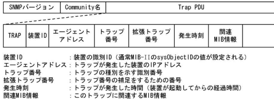
図 22-24 トラップフォーマット
