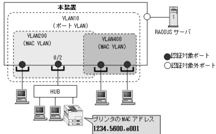
図 7-7 ポート単位認証（動的）の認証除外の構成例
