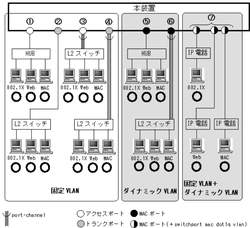
図 5-25 共存使用例と動作可否
