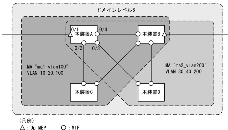
図 21-32 CFM の設定例（同ドメイン、複数 MA）
