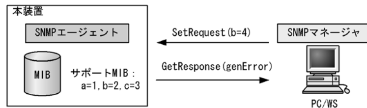
図 22-14 装置の状態によって設定できない場合の SetRequest オペレーション
