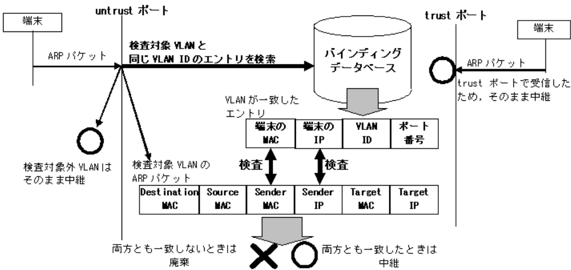
図 13-13 ダイナミック ARP 検査の基本検査概要
