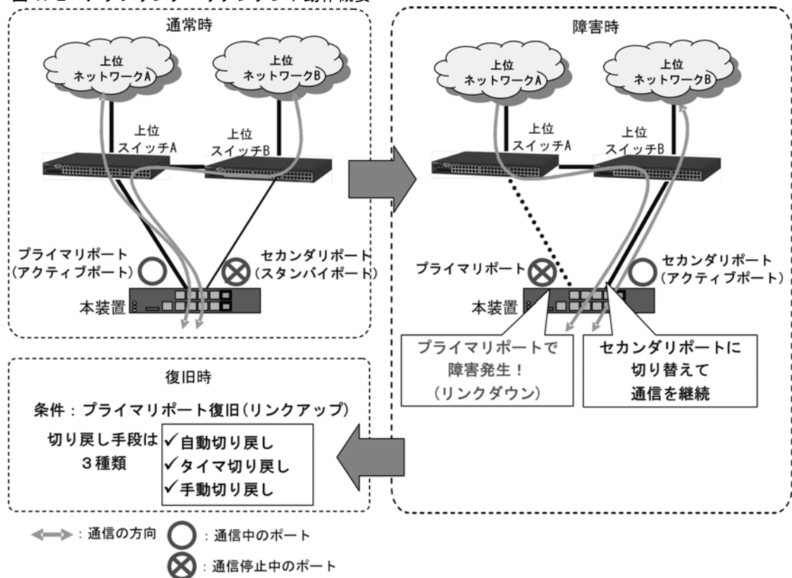
図 17-2 アップリンク・リダンダント動作概要
