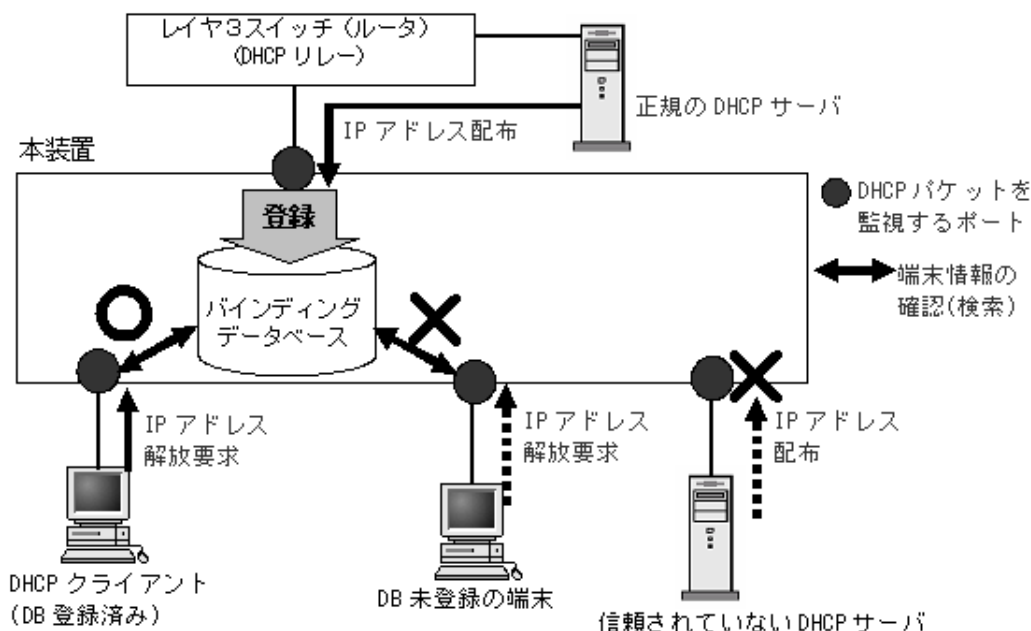
図 13-1 DHCP snooping 概要
