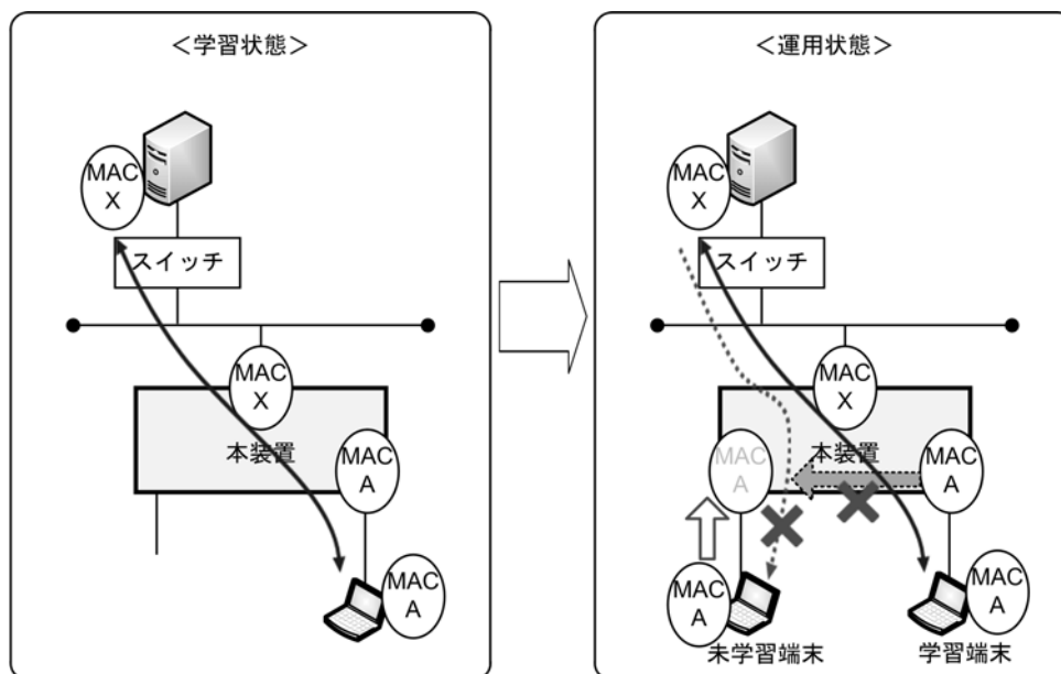
図 14-4 ホワイトアドレスリスト機能の概要
