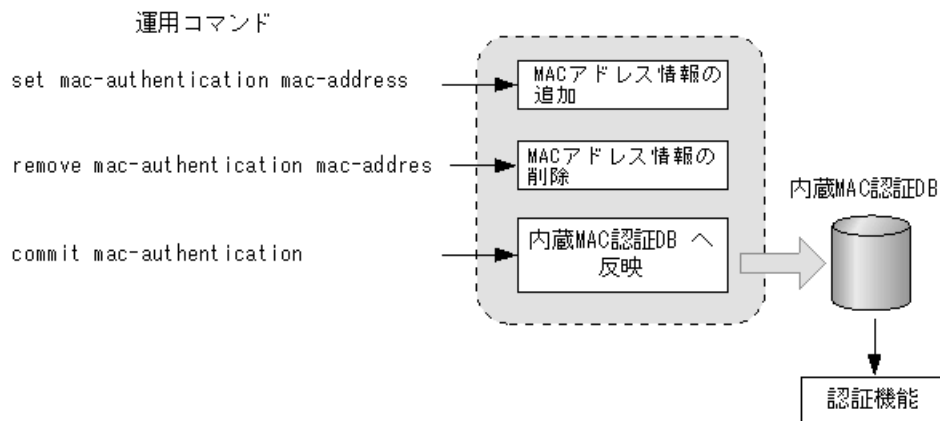
図 10-11 MAC アドレス情報の編集と内蔵 MAC 認証 DB への反映
