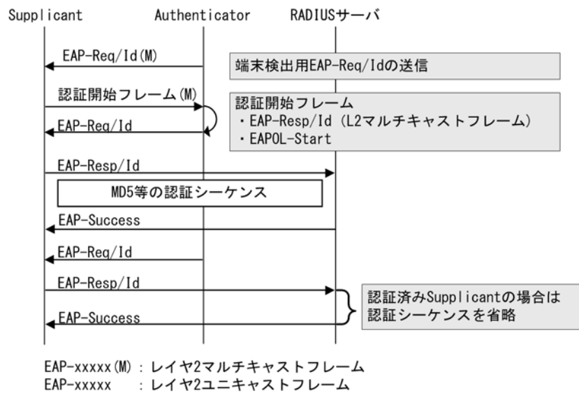
図 6-10 shortcut の EAP-Request/Identity のシーケンス
