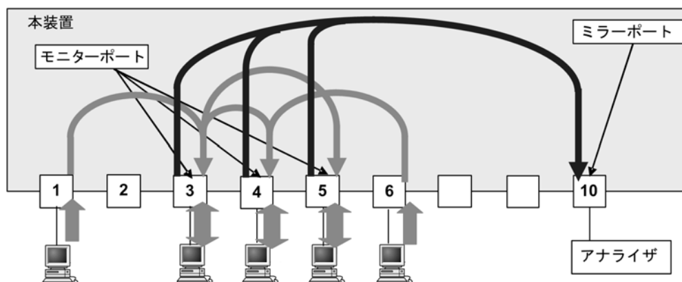
図 26-3 複数ポートのフレームのミラーリング（多対 1）
