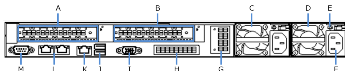
背面図 (標準構成)
