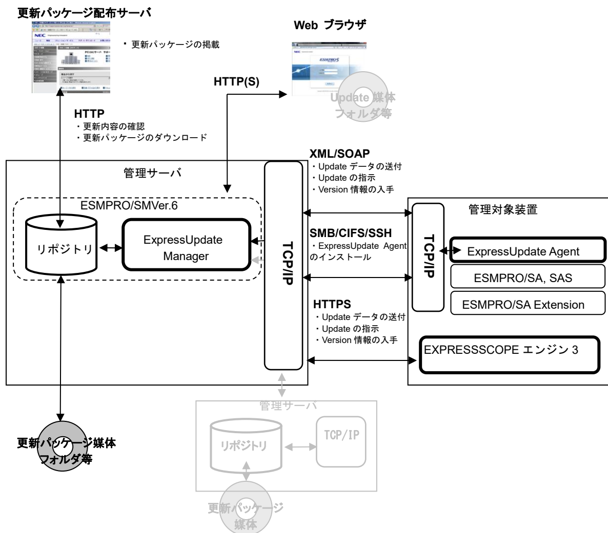
図 76 ExpressUpdate 概念図
