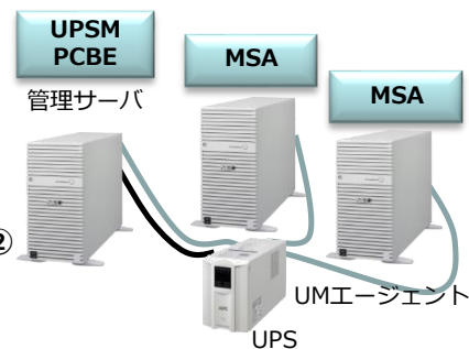
マルチサーバ構成例
