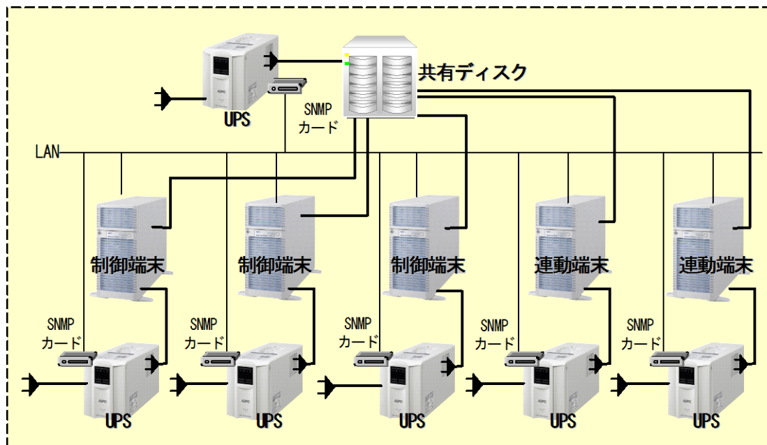
3 ノード以上のクラスタで クラスタ自身を制御端末とする 場合の構成例
