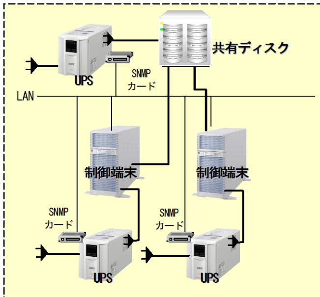
2 ノード構成クラスタ クラスタ自身が制御端末の場合の 構成例
