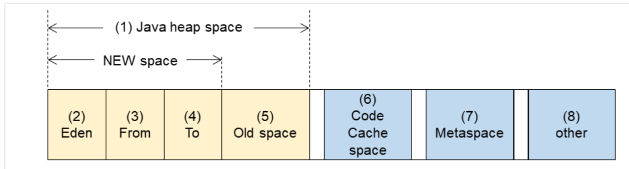
図 5.14 Java VM メモリ空間 (Oracle Java 8/Oracle Java 9/Oracle Java 11)
