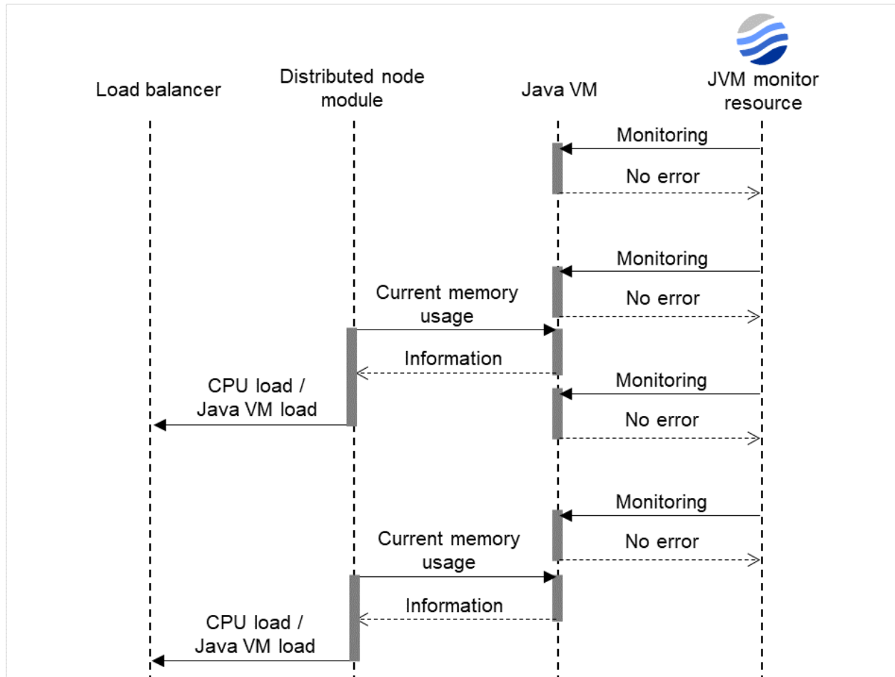
図 5.10 分散ノードモジュールの負荷算出機能
