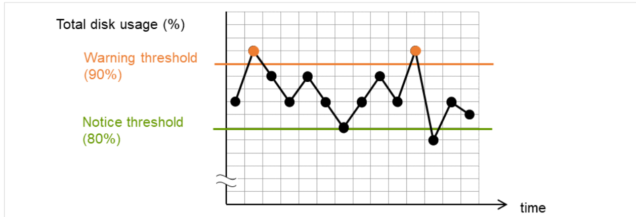
図 5.17 ディスク使用率が警告レベル上限値以上になった場合（異常検出する）
