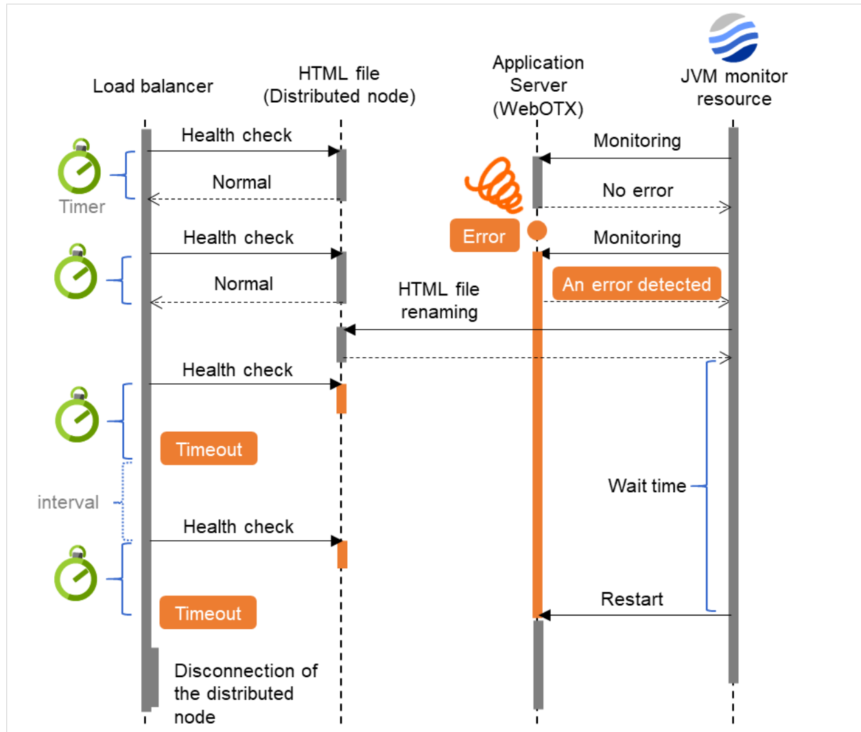
図 5.9 ロードバランサの JVM 監視リソース ヘルスチェック機能
