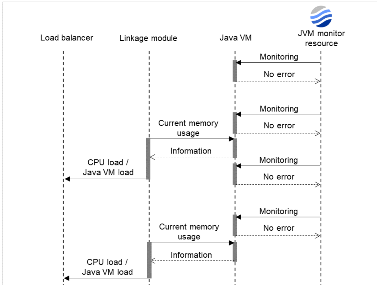
図 5.12 負荷算出機能
