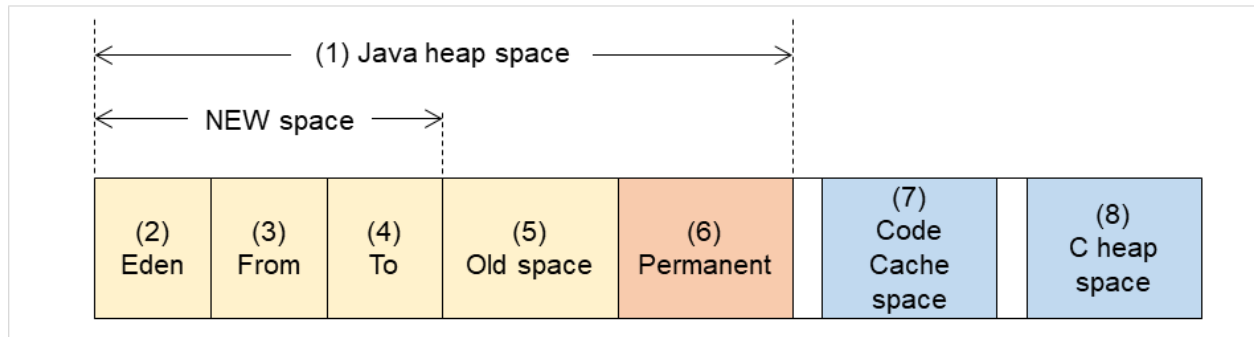
図 5.13 Java VM メモリ空間 (Oracle Java 7)
