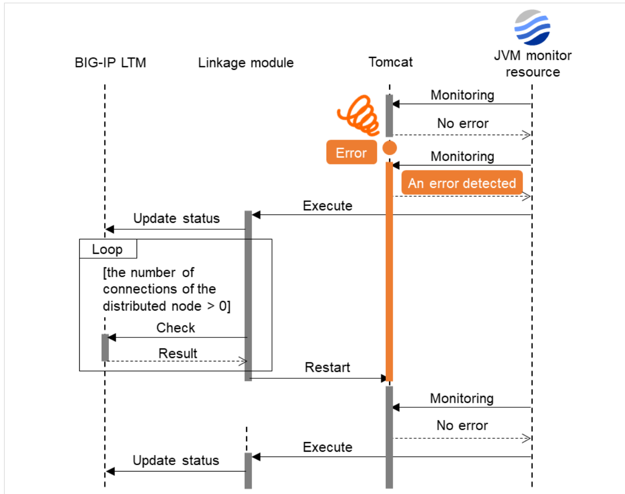
図 5.11 分散ノードの制御機能
