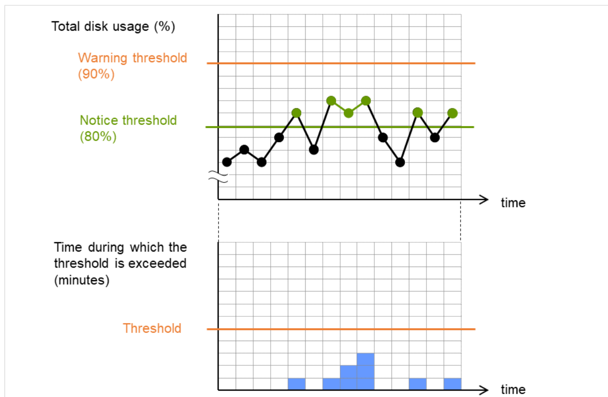
図 5.20 ディスク使用率において、通知レベル上限値以上の状態が一定時間続かない場合（異常検出しない）
