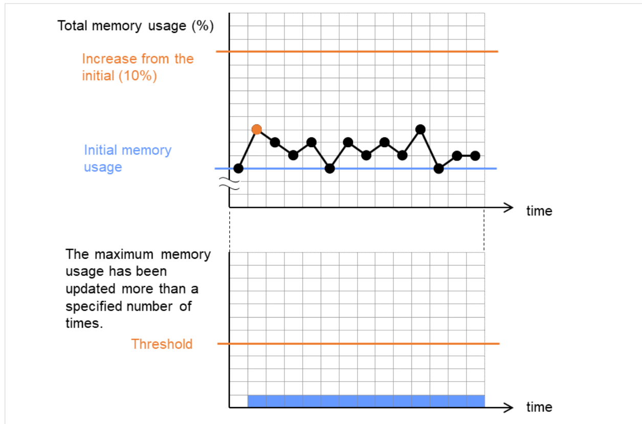
図 5.22 メモリ使用量が一定の範囲内で増減（異常検出しない）
