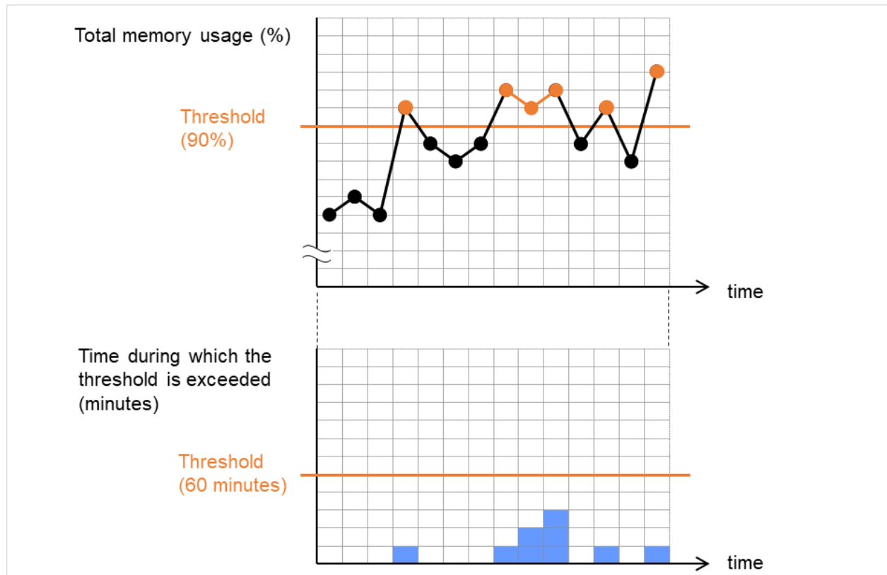
図 5.16 総メモリ使用量のしきい値以上の状態が一定時間続かない場合（異常検出しない）
