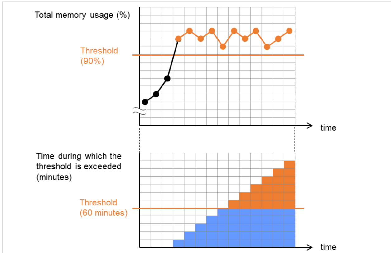
図 5.15 総メモリ使用量のしきい値以上の状態が一定時間続いた場合（異常検出する）
