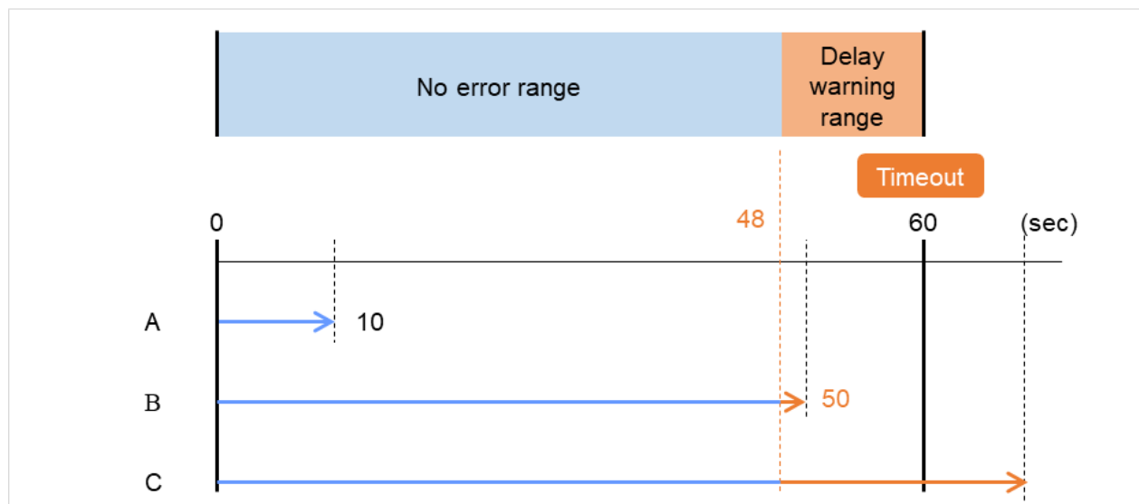
図 7.7 監視ポーリング時間と遅延警告
