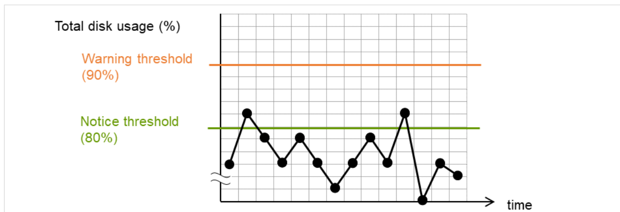
図 5.18 ディスク使用率が警告レベル上限値以上にならない場合（異常検出しない）
