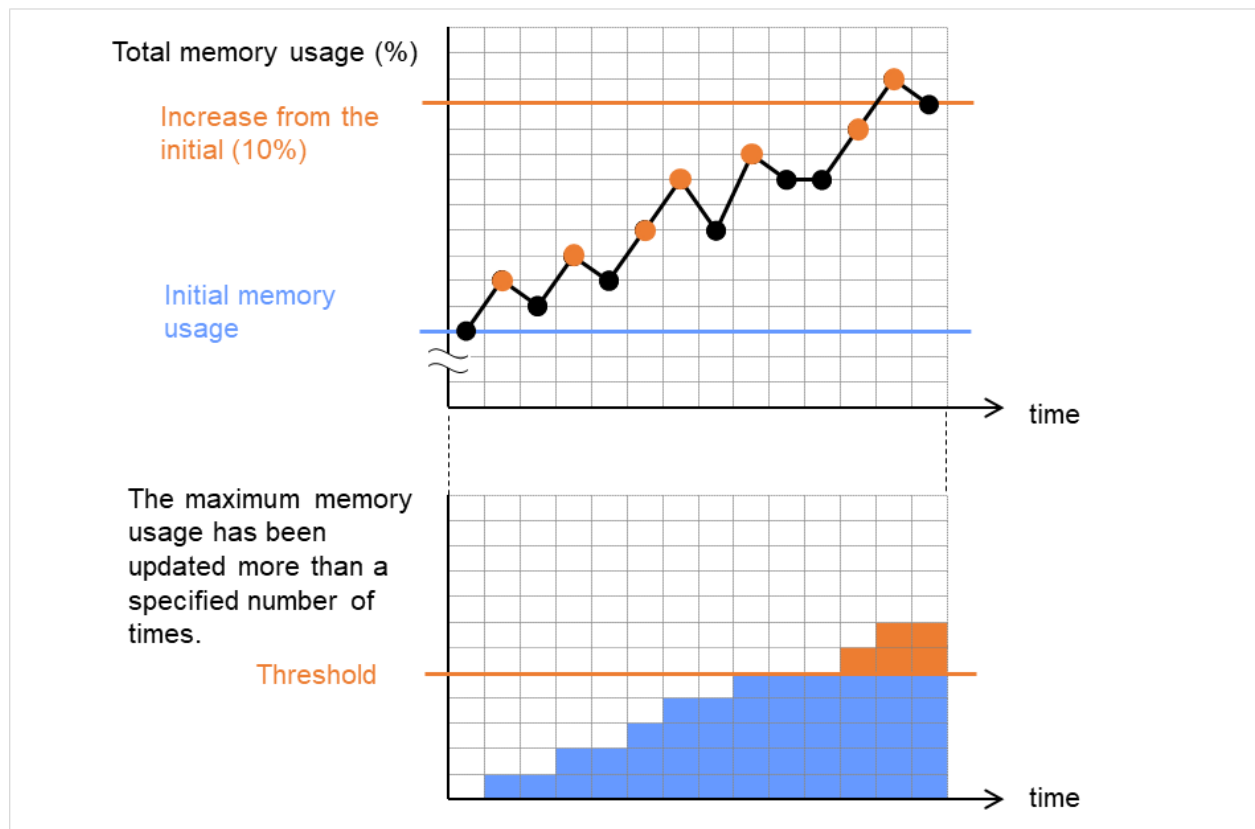
図 5.21 メモリ使用量が規定回数以上最大値を更新し、増加率が初期値の 10% を超過（異常検出する）
