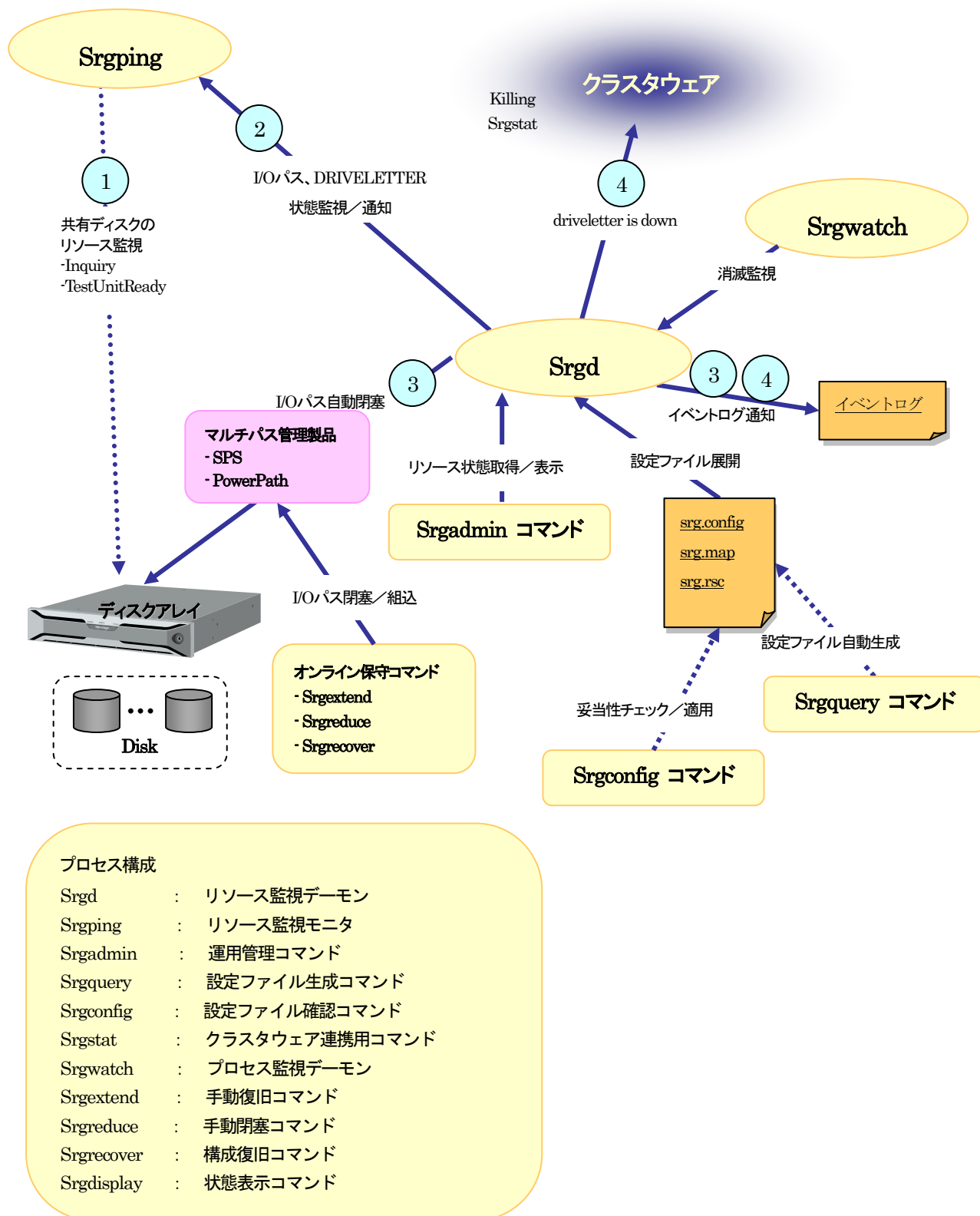
図 3 StorageSaver のプロセスモデル
