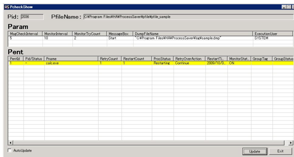
図 19 『Pcheck Show』プロセス消滅検知時画面
