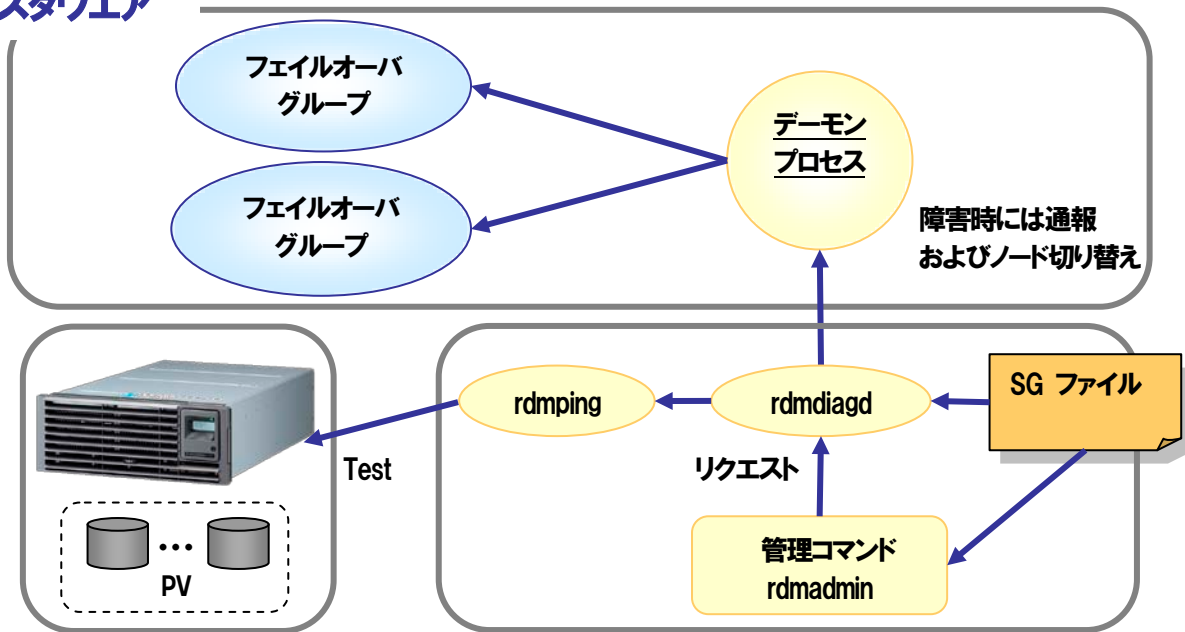
【RootDiskMonitor の構成】
