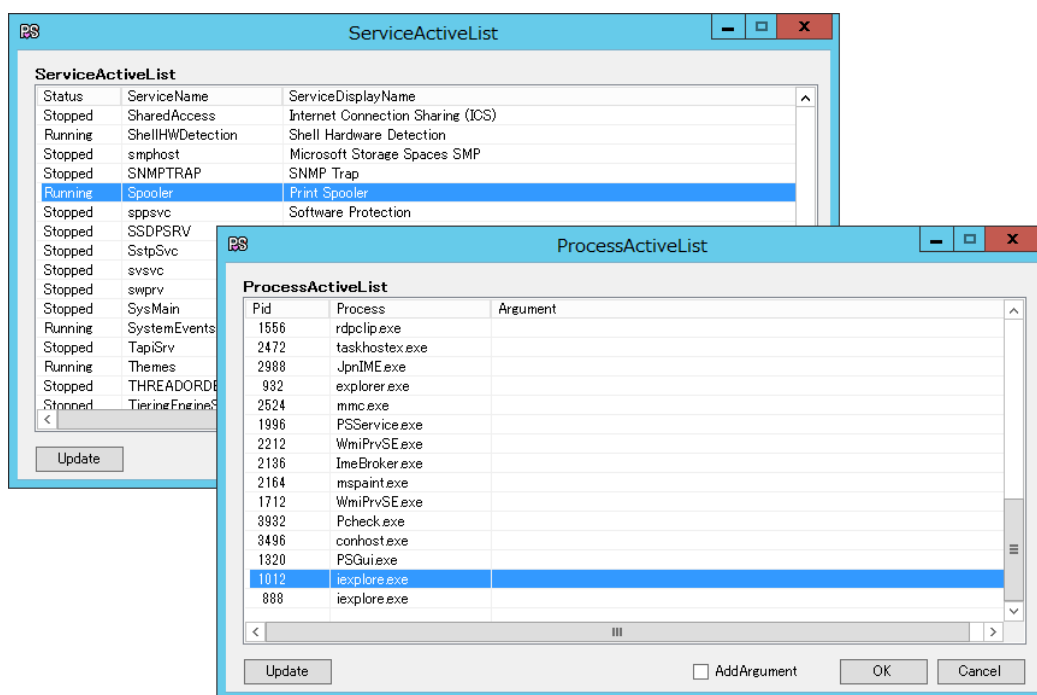
図 9 『ProcessActiveList』/『ServiceActiveList』
