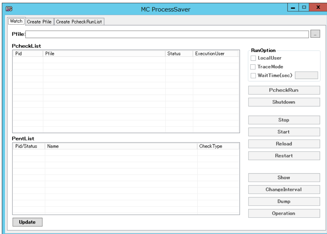
図 1 『Watch』
