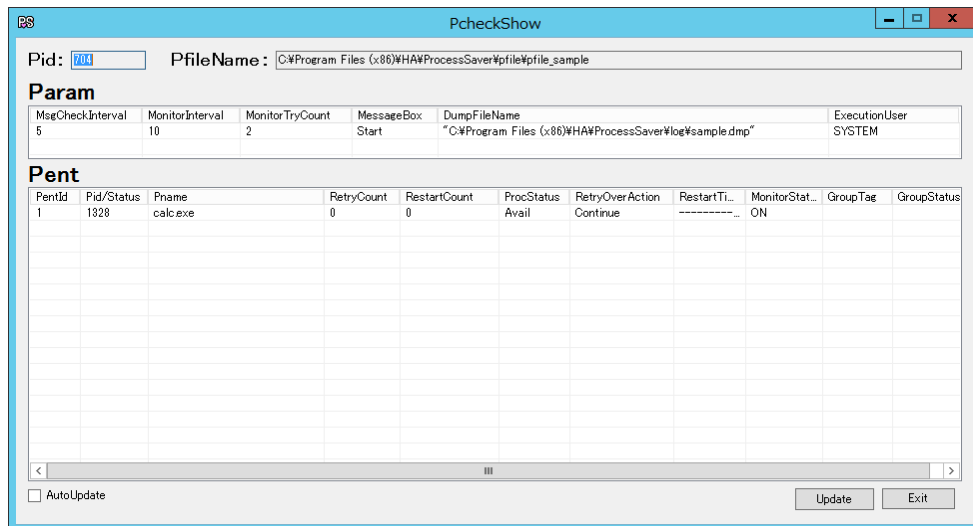
図 18 『Pcheck Show』
