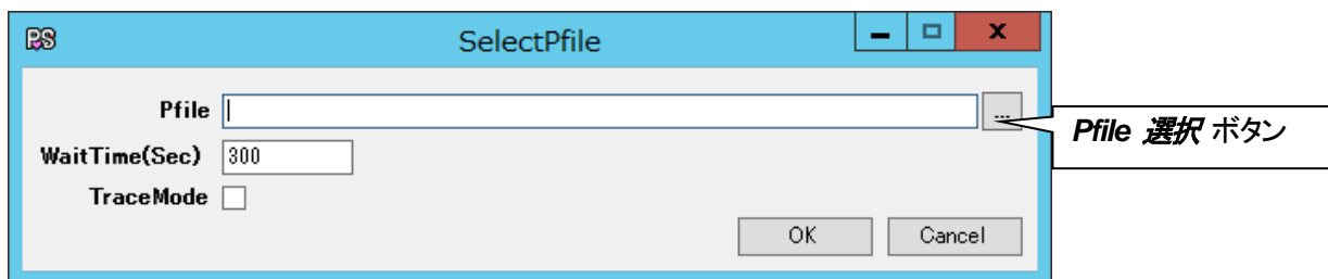
図 25 『SelectPfile』
