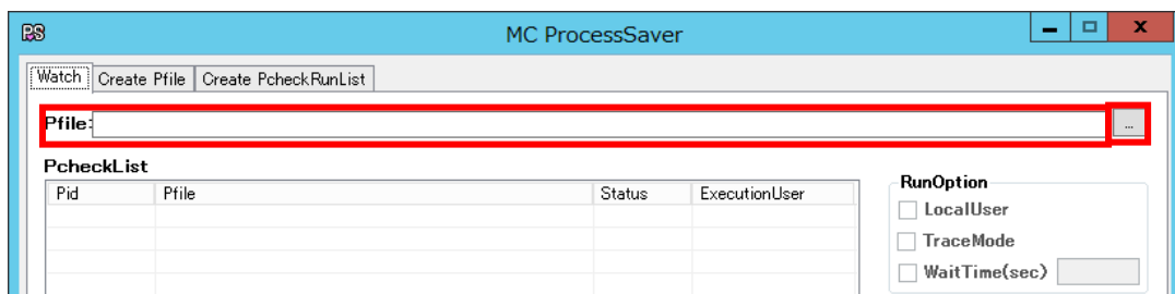
図 14 『Watch』
