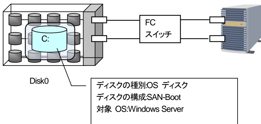
図 2 SAN-Boot 構成
