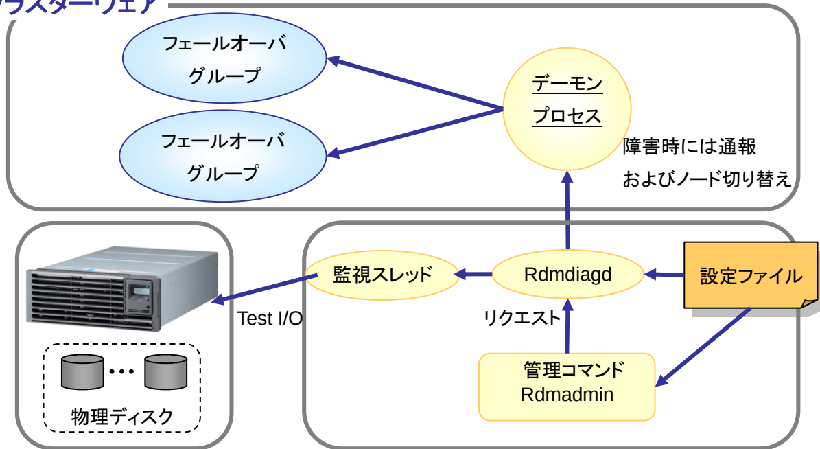
【RootDiskMonitor の構成】
