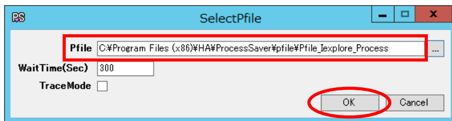
図49 『SelectPfile』
