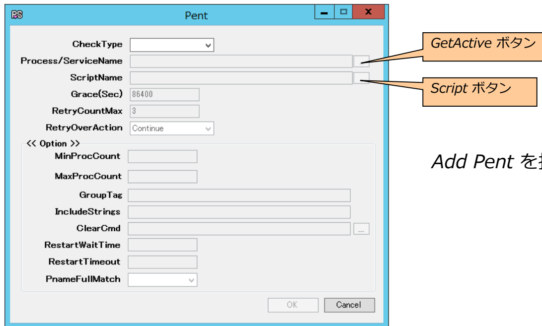
図13 『Pent』
