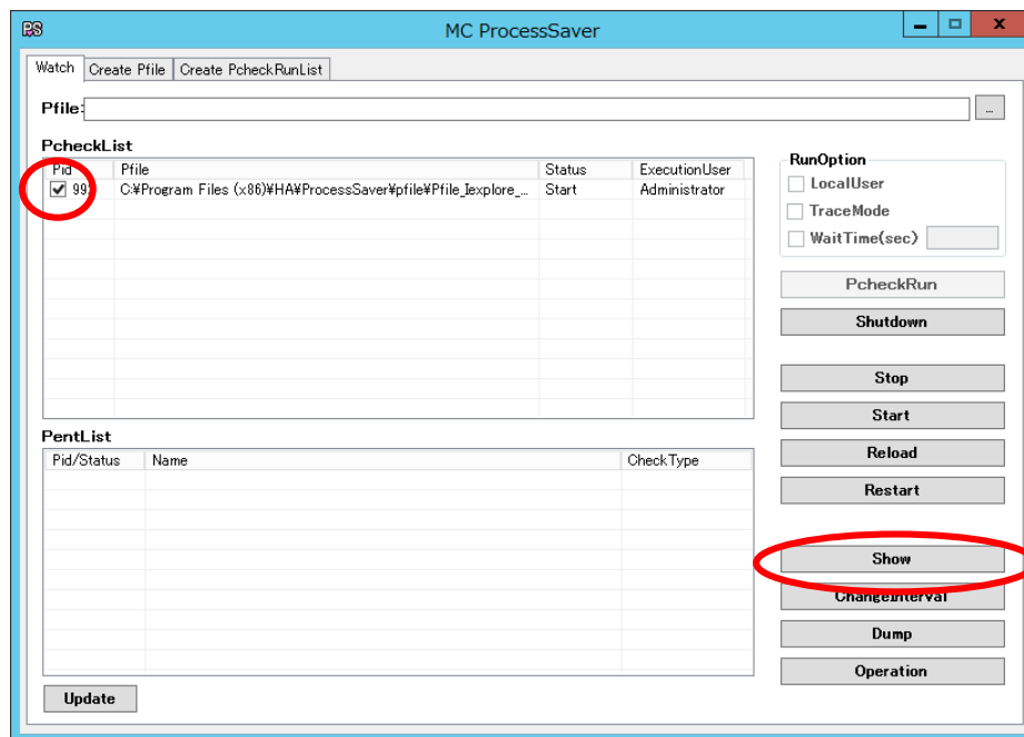
図36 『Watch』
