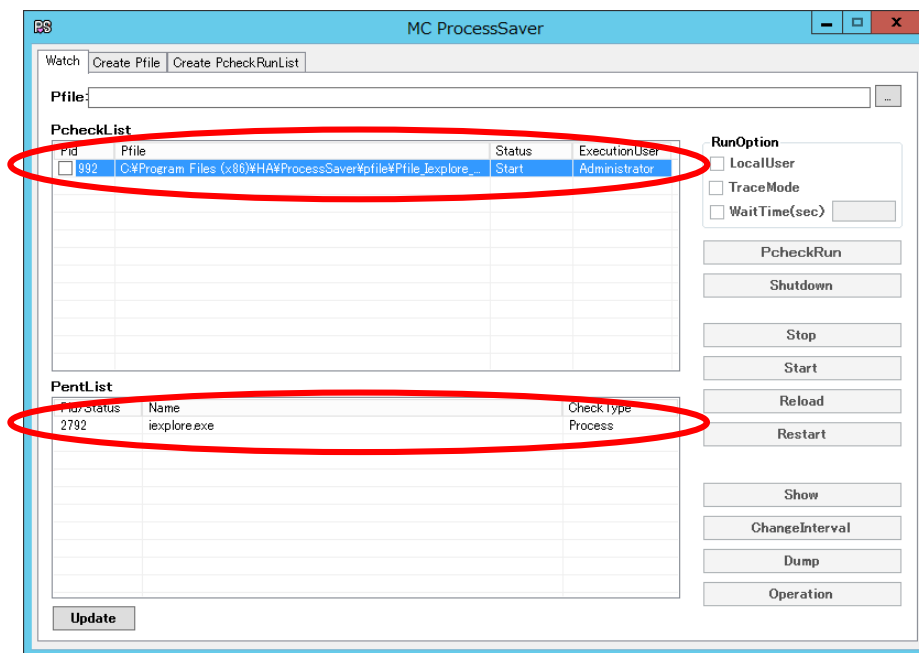
図28 『Watch』
