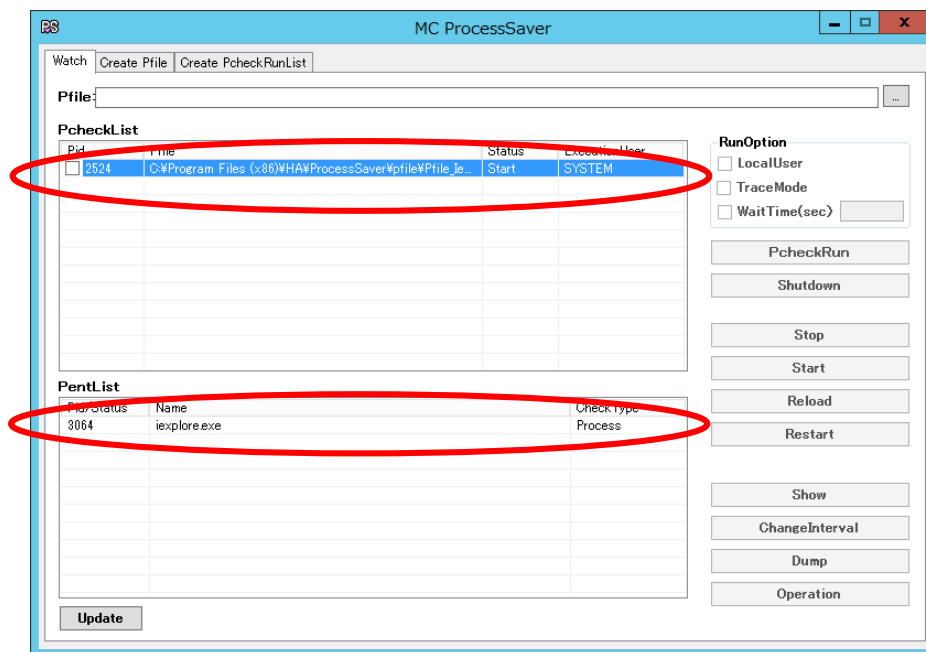
図52 『Watch』
