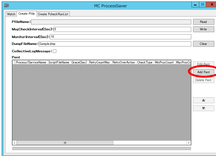
図12 『Create Pfile』
