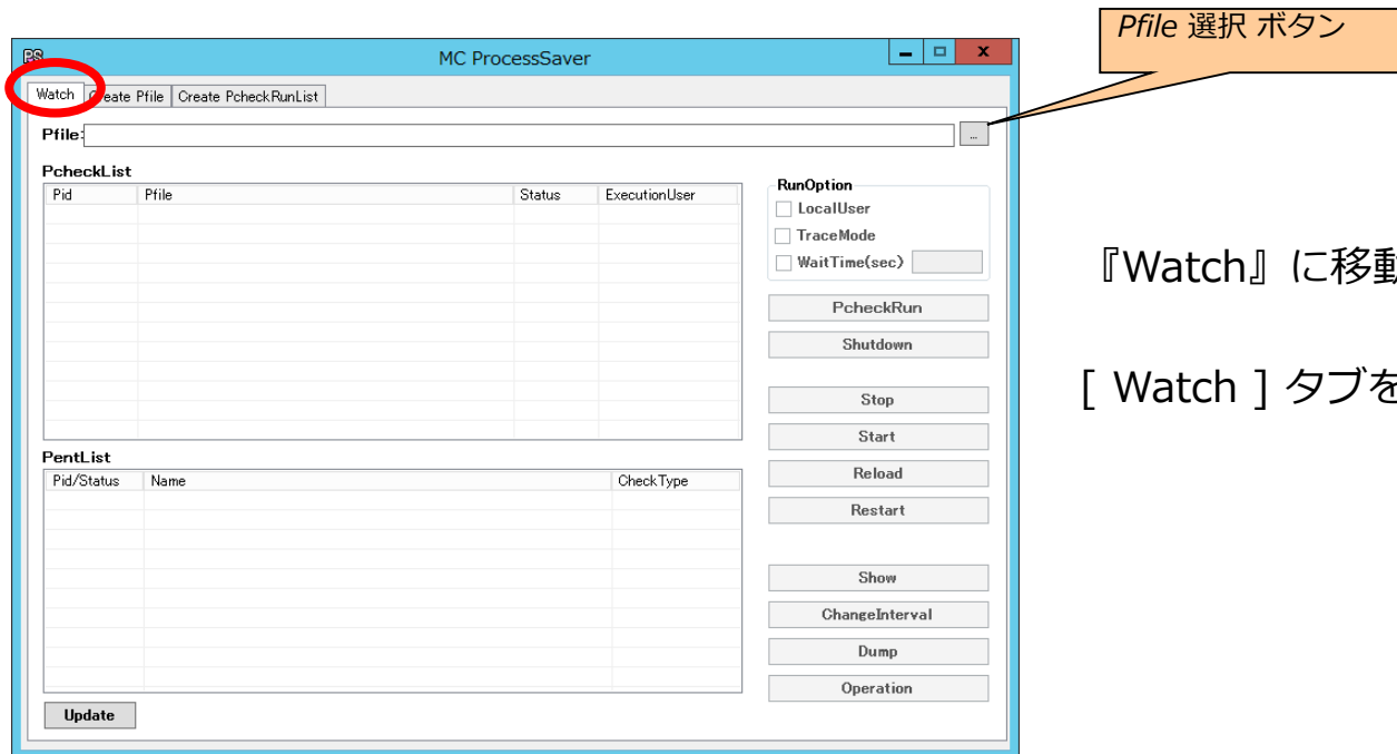
図23 『 Watch 』
