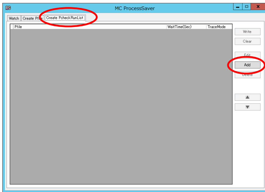
図46 『Create PcheckRunList』
