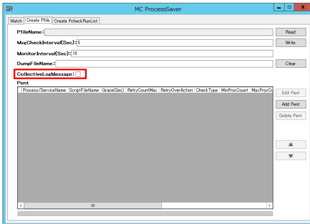
図 9 『Create Pfile』
