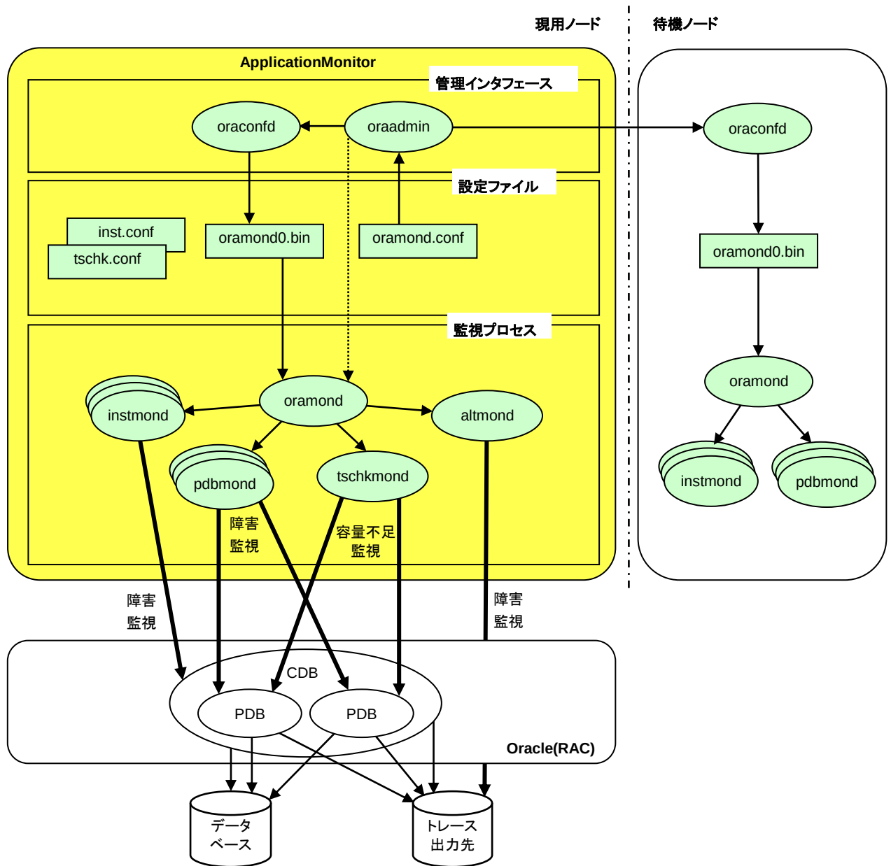
図 2-2 ソフトウェア構成 (マルチテナント構成の PDB 監視)
