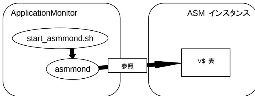
図 4-39 ASM 監視モニタの概要
