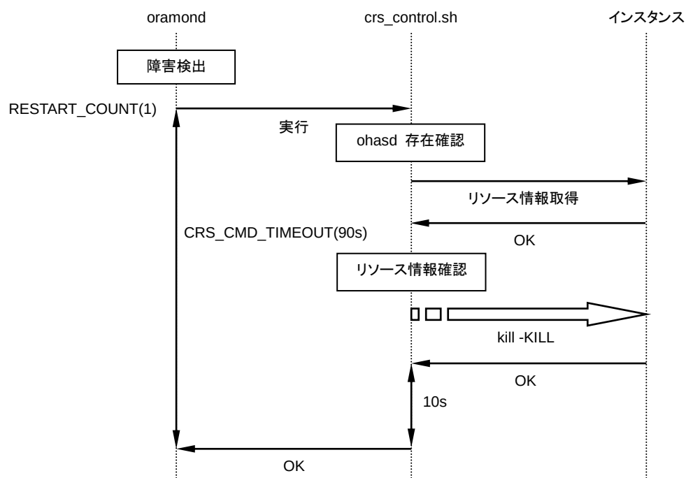
図 4-51 インスタンス監視時の Oracle Clusterware／Oracle Restart リトライ判定シェルスクリプトの動作
