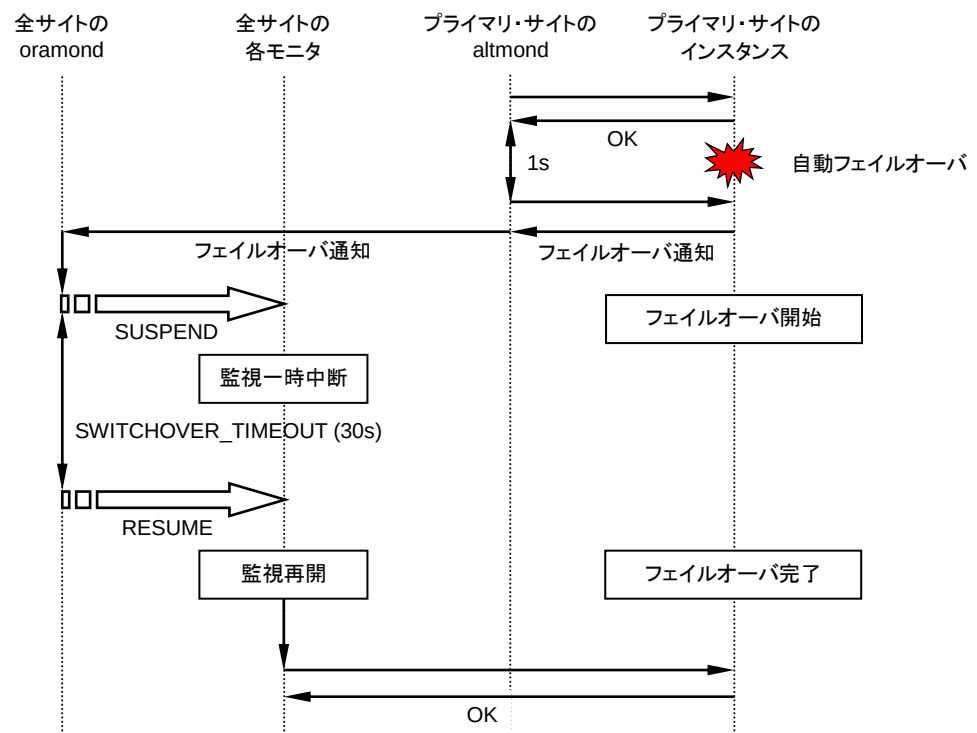
図 4-58 Oracle Data Guard Broker による自動フェイルオーバー時の監視動作
