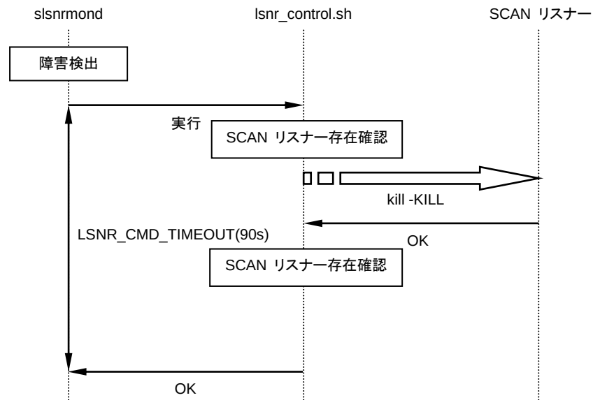
図 4-57 リスナー再起動シェルスクリプトの動作 (Oracle Clusterware による SCAN リスナーの再起動)
