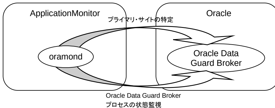
図 4-28 スタンバイ・インスタスの Oracle Data Guard Broker プロセスの状態監視時の概要
