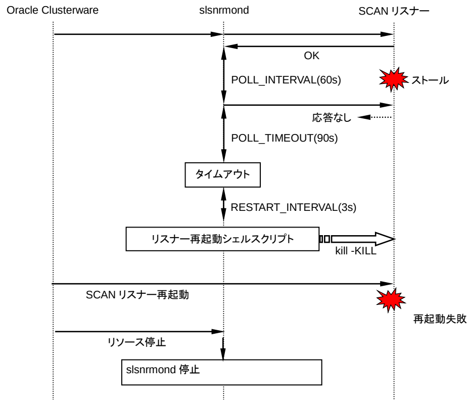
図 4-48 SCAN リスナー監視タイムアウト時の動作（Oracle Clusterware によって SCAN リスナーが再起動されなかった場合）
