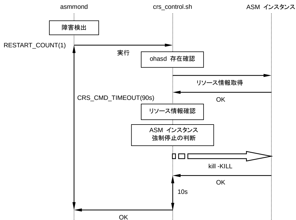
図 4-53 ASM インスタンス監視時の Oracle Clusterware／Oracle Restart リトライ判定シェルスクリプトの動作
