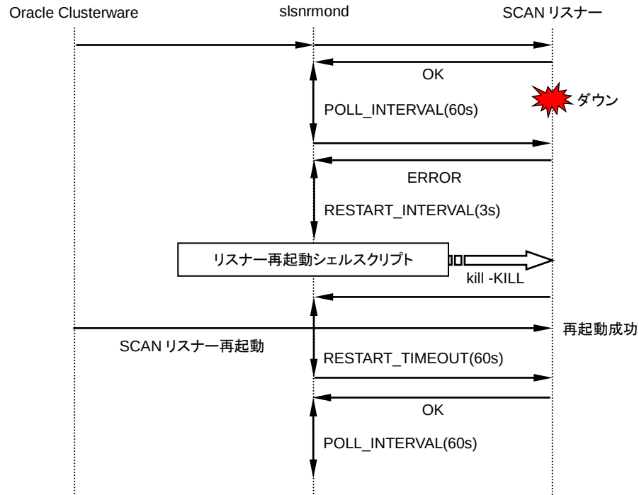
図 4-46 SCAN リスナー監視エラー時の動作（Oracle Clusterware によって SCAN リスナーが再起動された場合）
