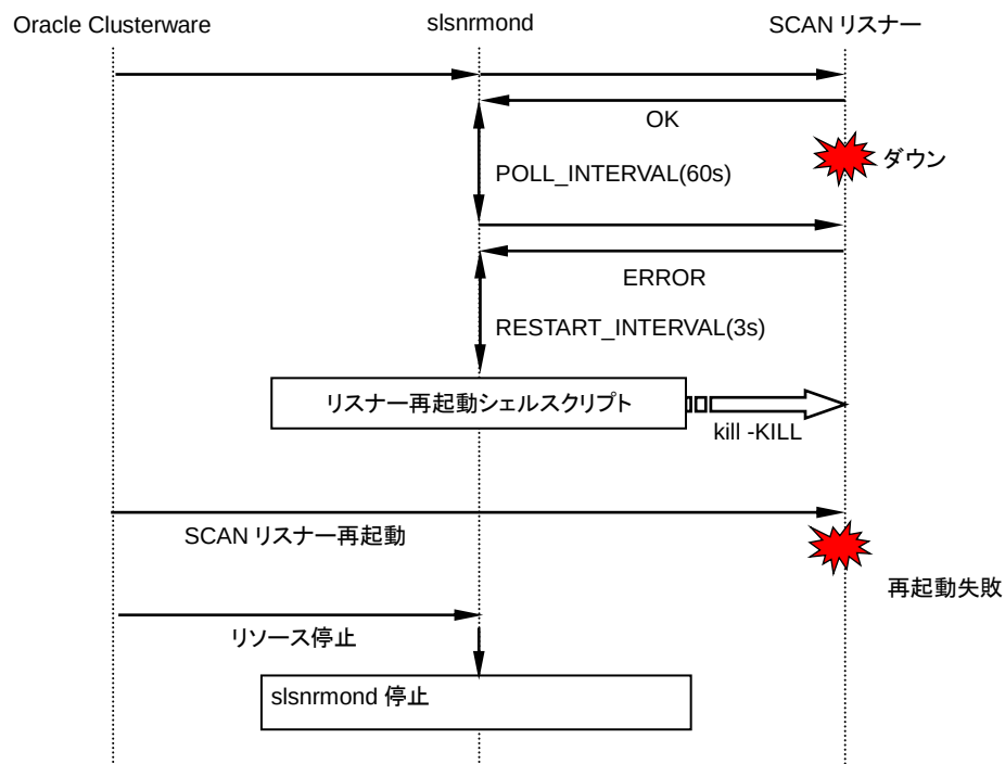
図 4-47 SCAN リスナー監視エラー時の動作（Oracle Clusterware によって SCAN リスナーが再起動されなかった場合）
