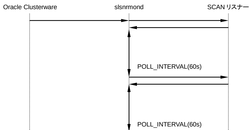
図 4-45 SCAN リスナー監視時の動作
