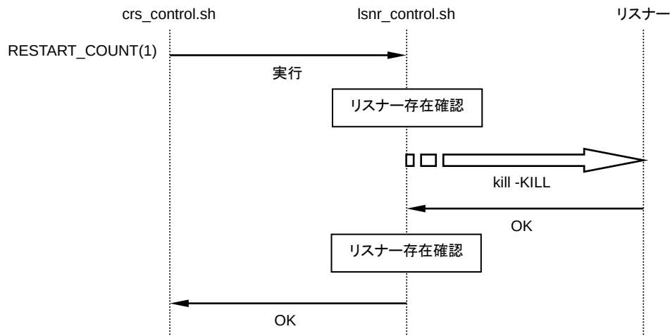
図 4-56 リスナー再起動シェルスクリプトの動作
