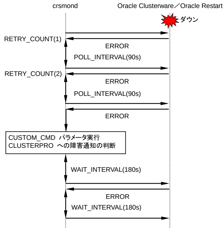
図 4-33 CRS 監視モニタ起動エラー時の動作
