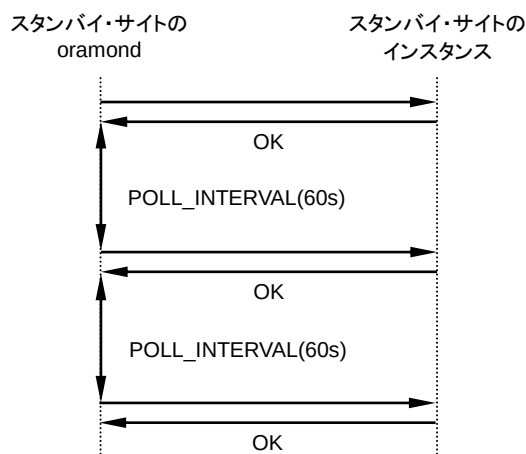
図 4-29 スタンバイ・インスタスの Oracle Data Guard Broker プロセスの状態監視時の動作(一定時間経過による監視)
