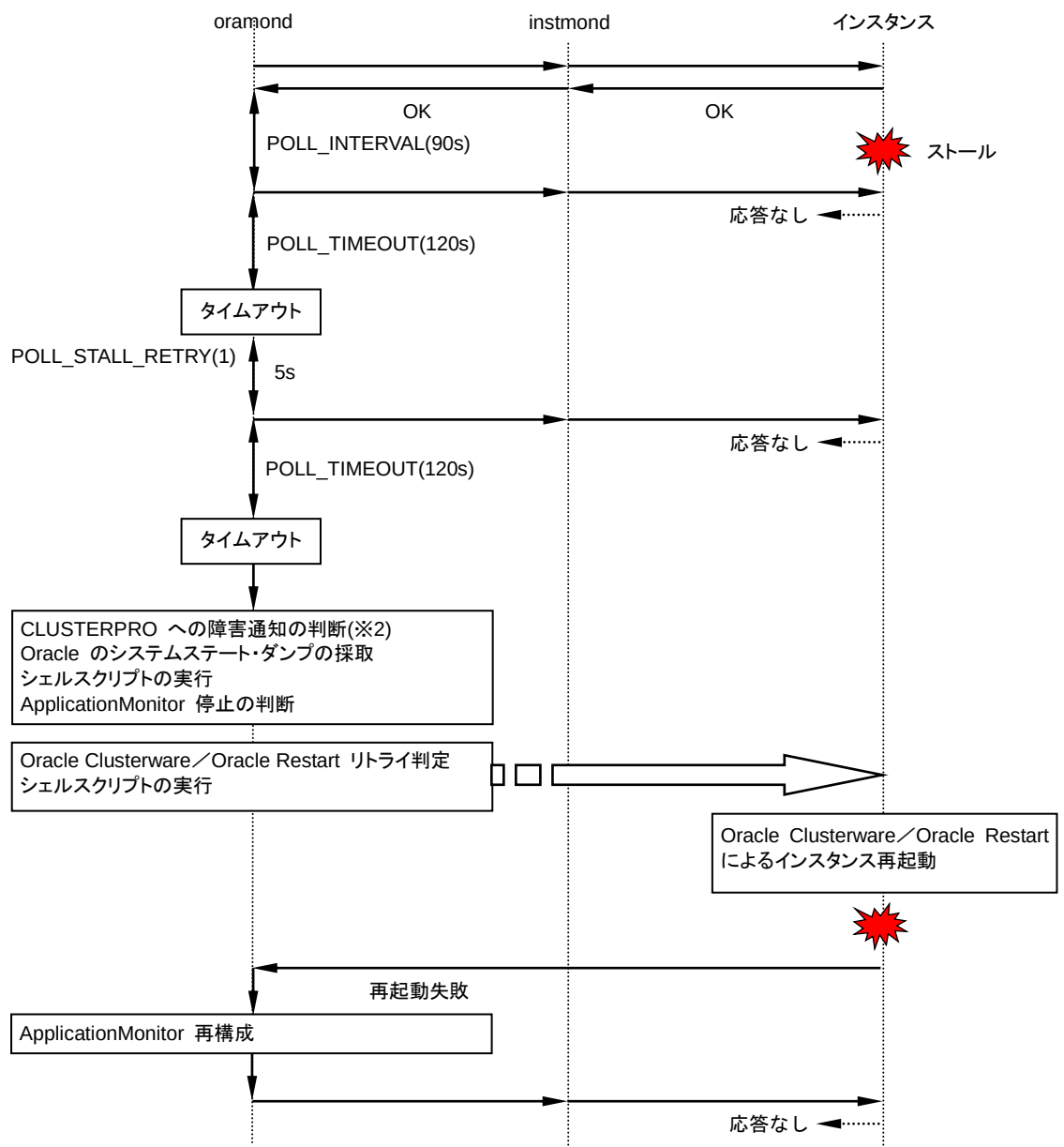
図 4-7 インスタンス監視タイムアウト時の動作
