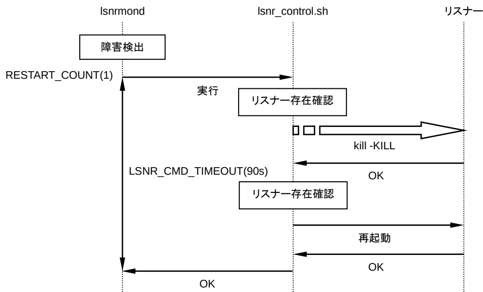
図 4-55 リスナー再起動シェルスクリプトの動作 (ApplicationMonitor によるリスナーの再起動)
