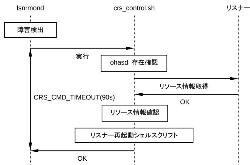
図 4-52 リスナー監視時の Oracle Clusterware／Oracle Restart リトライ判定シェルスクリプトの動作
