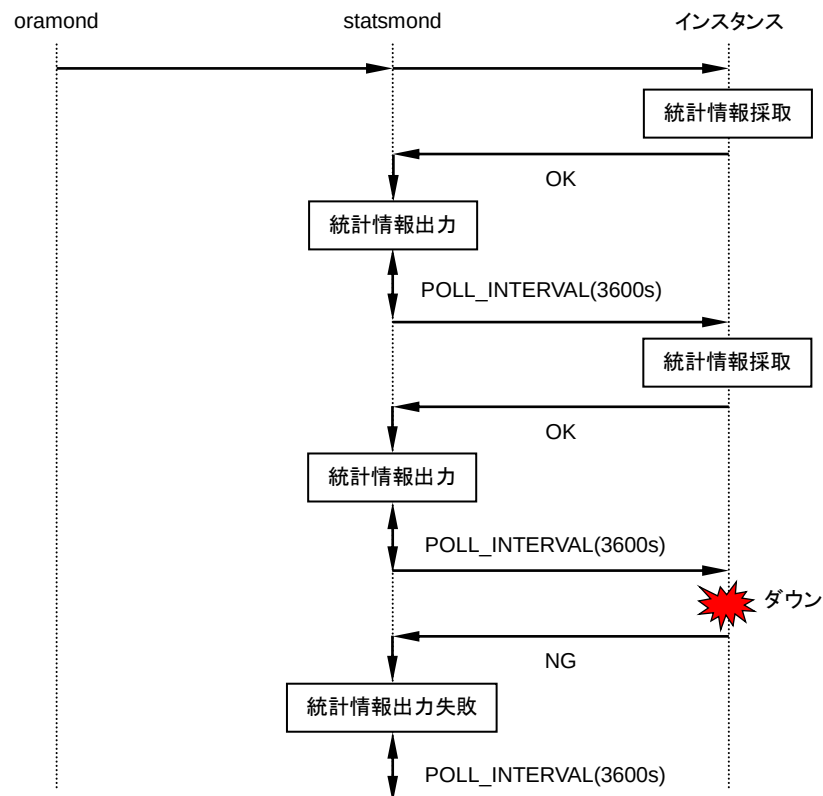
図 4-49 統計情報採取時の動作
