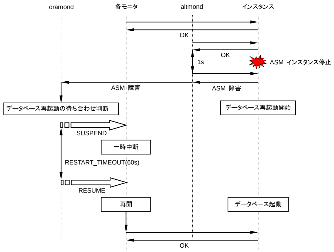
図 4-59 ASM インスタンス停止に伴うデータベースの再起動時の監視動作
