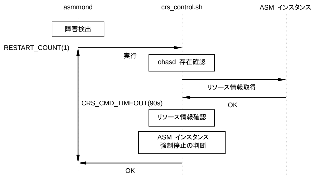
図 4-54 ASM インスタンス監視時の Oracle Clusterware／Oracle Restart リトライ判定シェルスクリプトの動作 (ASM インスタンスの SMON プロセスに対して kill コマンドを実行せず、Oracle Clusterware／Oracle Restart による ASM インスタンス再起動を待ち合わせる場合)
