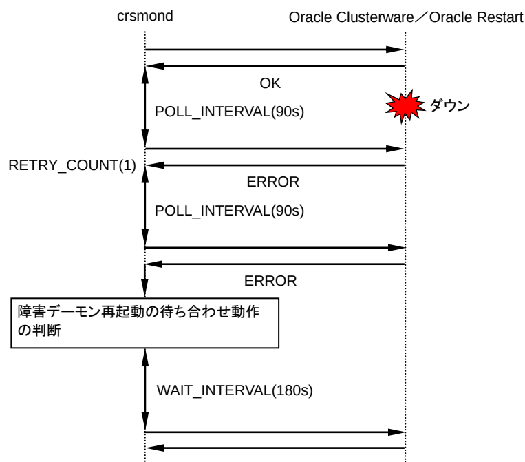
図 4-37 Oracle Clusterware／Oracle Restart 監視エラー時の動作
