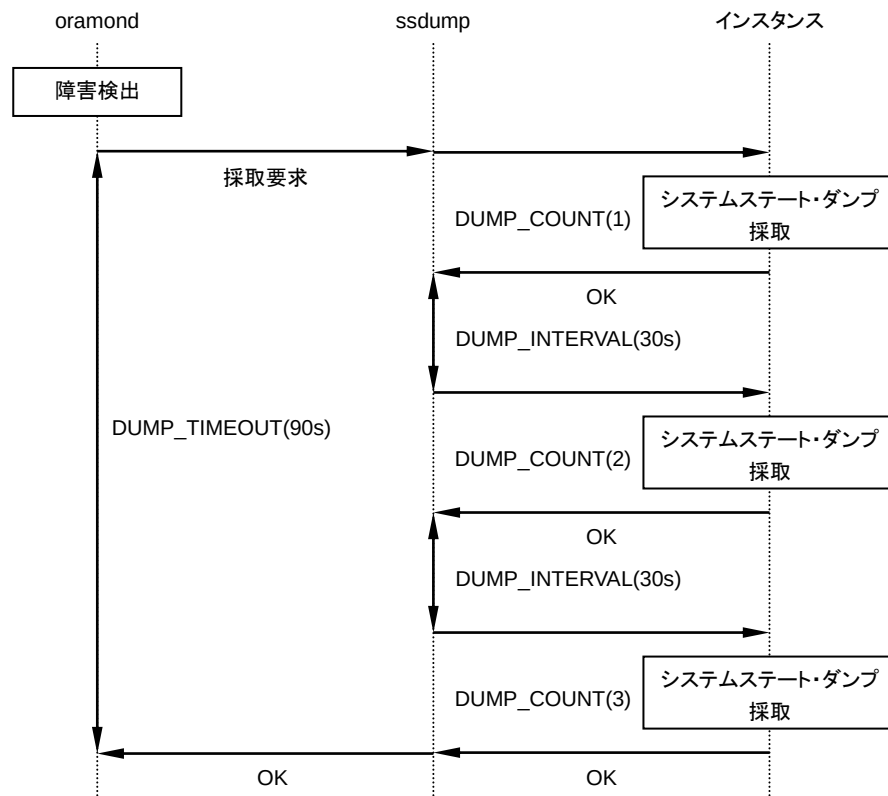
図 4-50 Oracle のシステムステート・ダンプ採取時の動作
