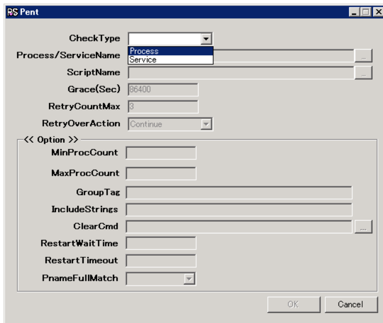
図15 『Pent』
