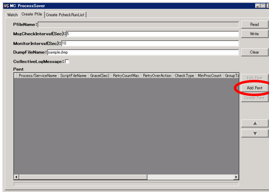
図13 『Create Pfile』
