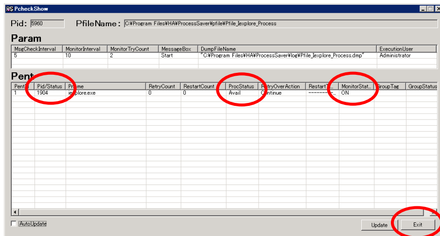
図31 『Pcheck Show』
