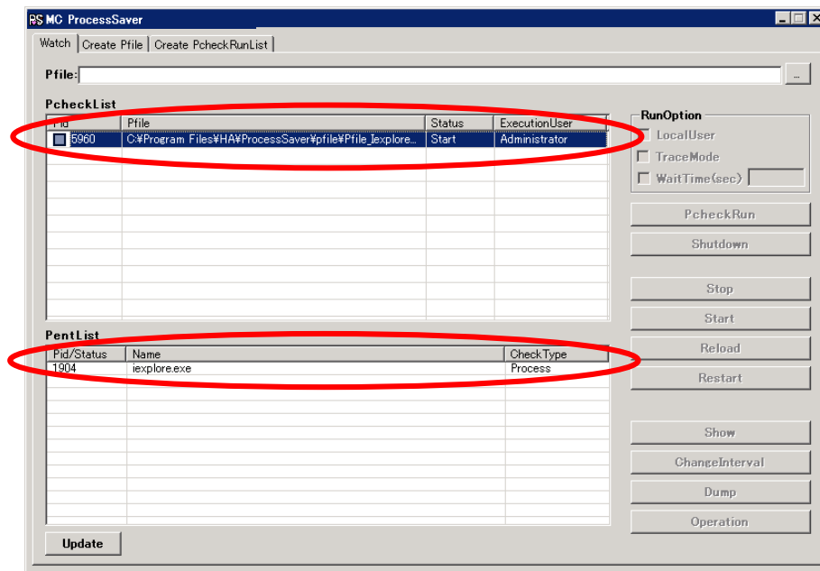
図29 『Watch』
