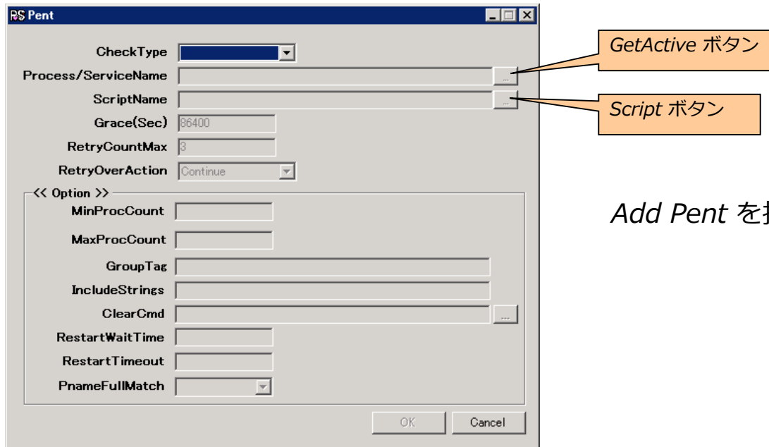
図14 『Pent』
