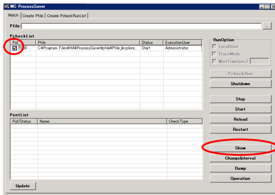
図37 『Watch』
