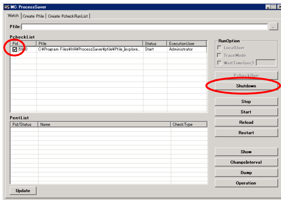
図45 『Watch』
