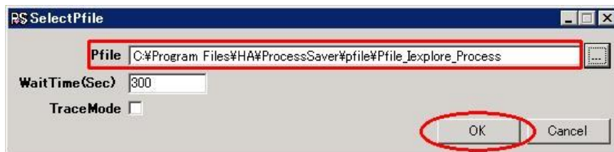
図50 『SelectPfile』
