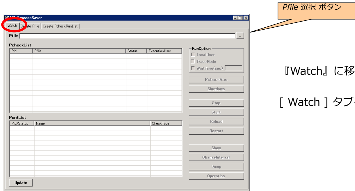
図24 『 Watch 』
