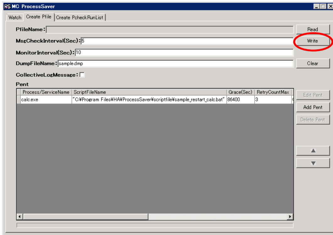
図 12『Create Pfile』
