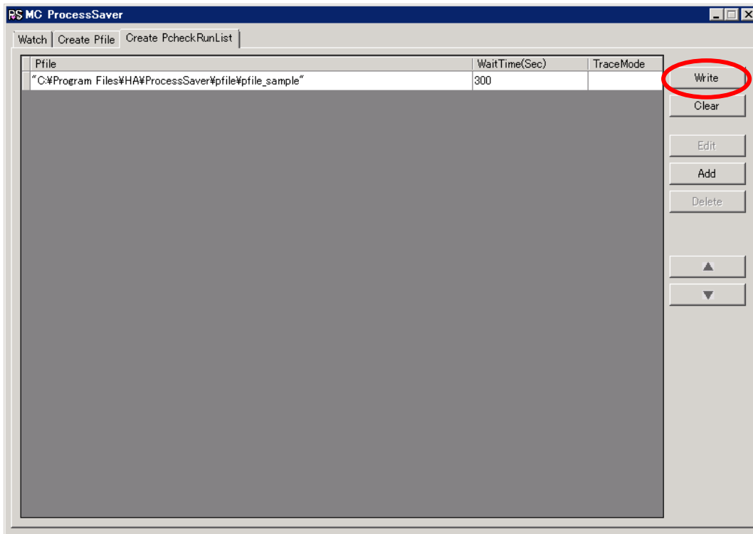
図 28 『Create PcheckRunList』
