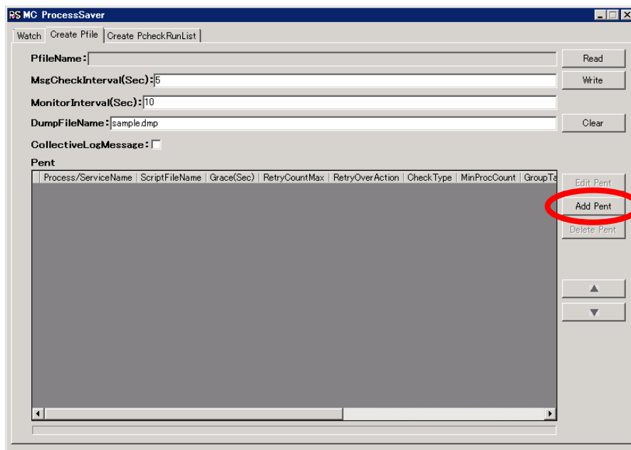
図13 『Create Pfile』
