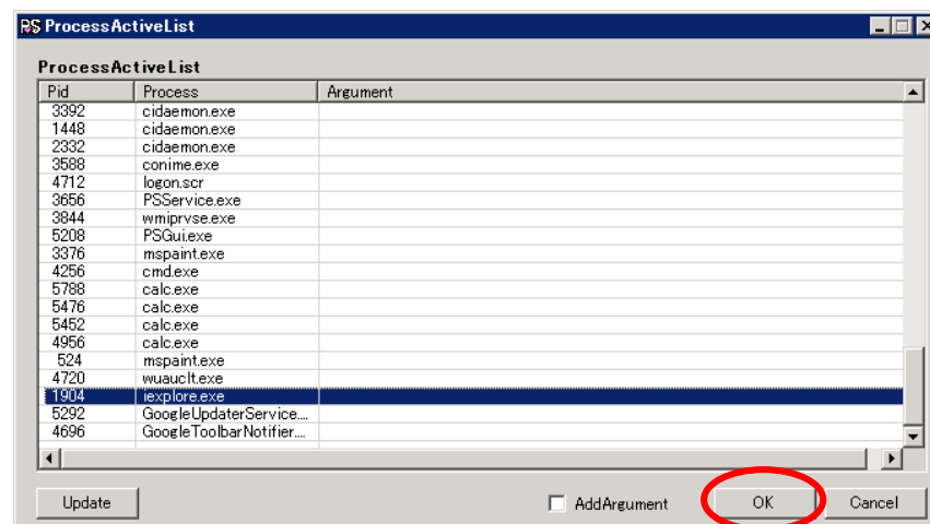
図17 『ProcessActiveList』
