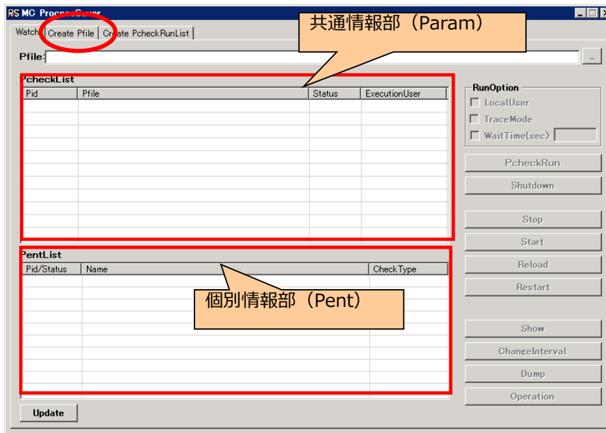
図8 『Create Pfile』
