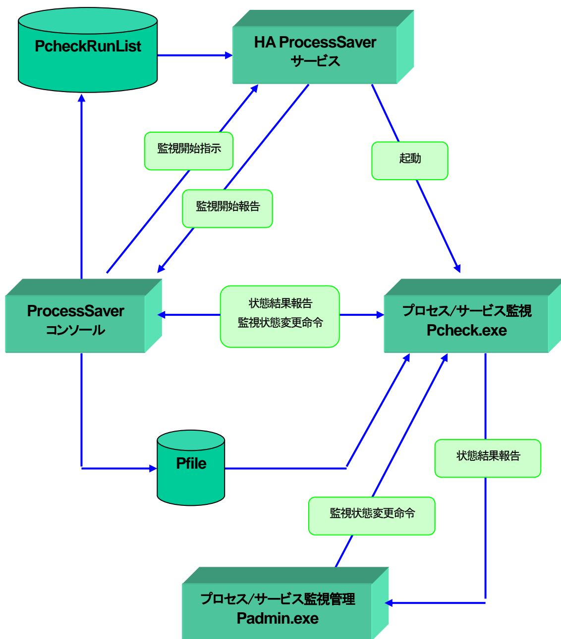
図1 『構成図』
