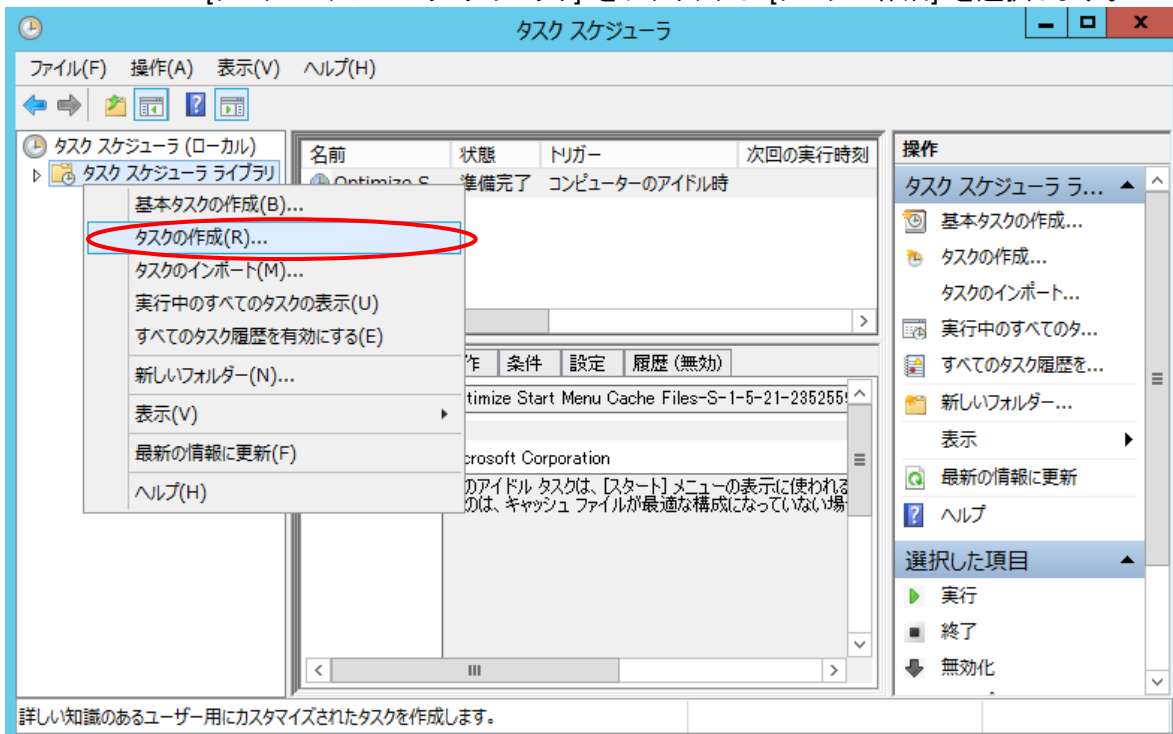
図 6 タスク作成
