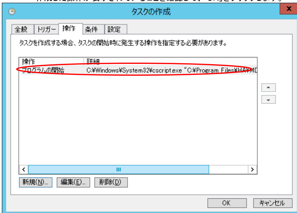
図 37 操作の確認
