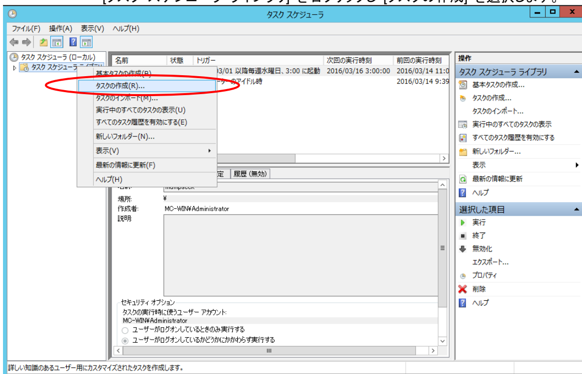
図 21 タスク作成
