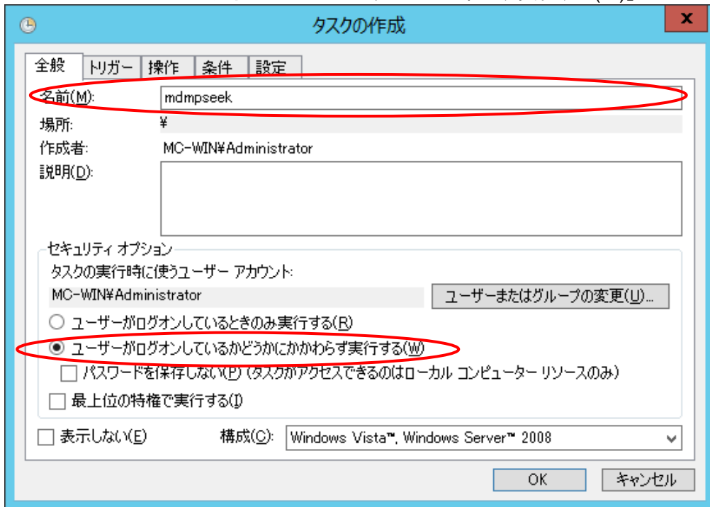
図 7 全般タブ
