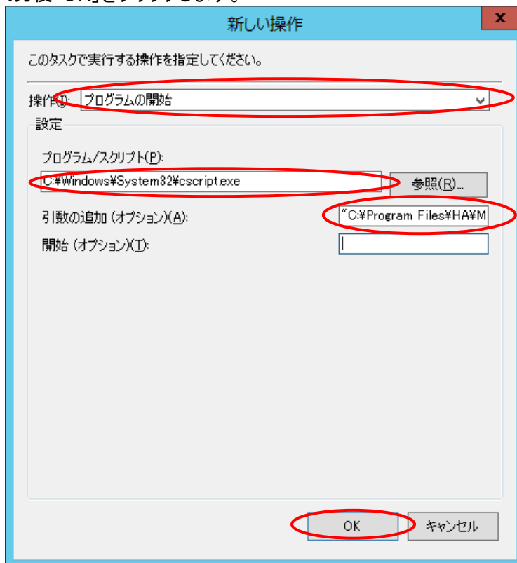
図 27 新しい操作
