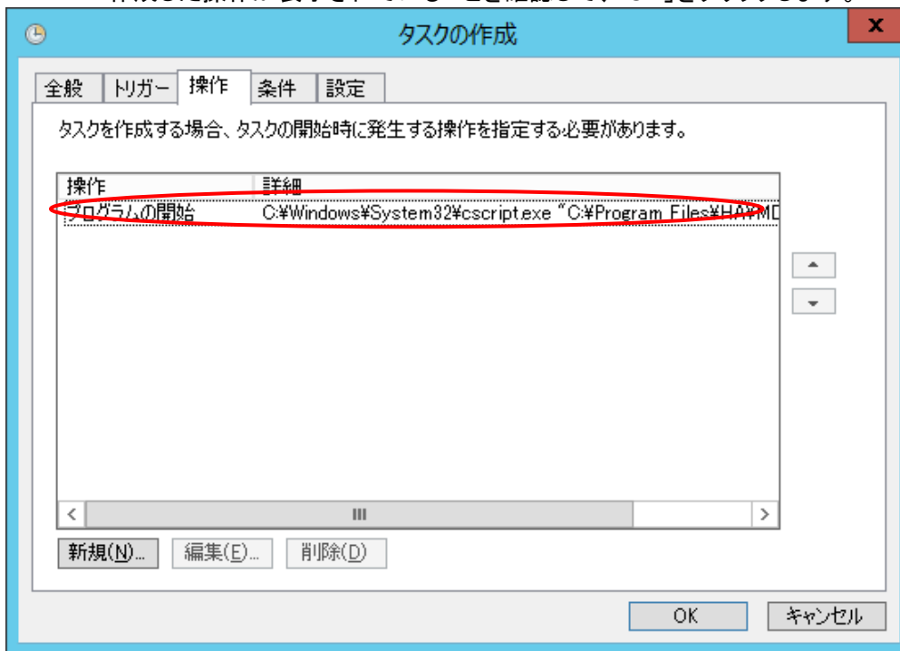
図 28 操作の確認
