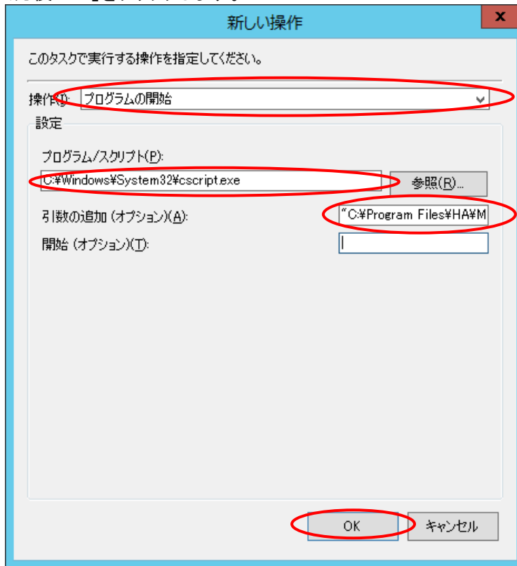
図 36 新しい操作
