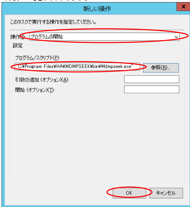
図 12 新しい操作
