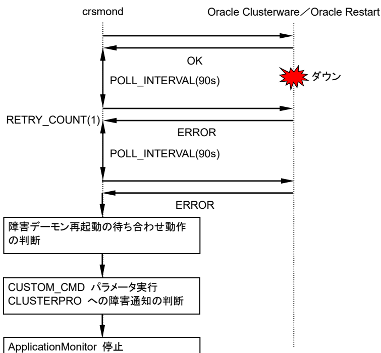
図 4-46 Oracle Clusterware／Oracle Restart 監視エラー時の動作 (障害を検出した Oracle Clusterware／Oracle Restart の デーモンプロセスに対する kill コマンドの実行、 障害デーモンの再起動の待ち合わせを行わない場合)
