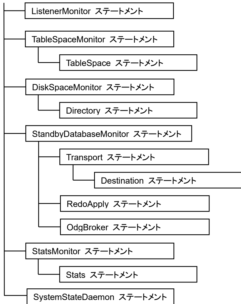
図 3-7 ステートメントの階層
