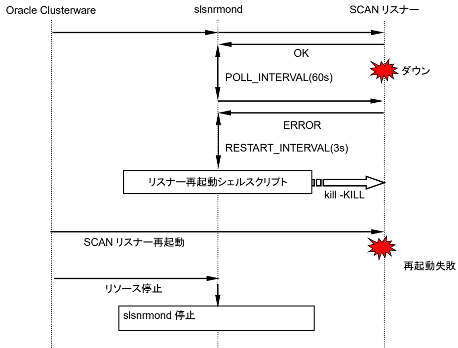
図 4-58 SCAN リスナー監視エラー時の動作 (Oracle Clusterware によって SCAN リスナーが再起動されなかった場合)
