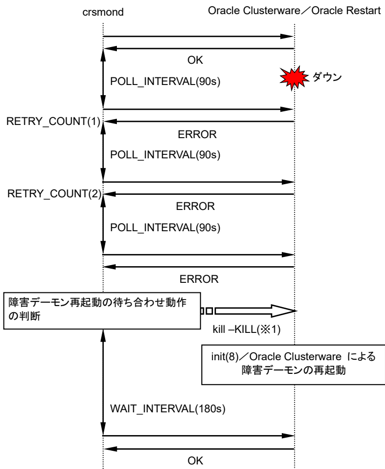
図 4-42 Oracle Clusterware/Oracle Restart 監視エラー時の動作 (init(8)/Oracle Clusterware による 障害デーモンの再起動が行われた場合)
