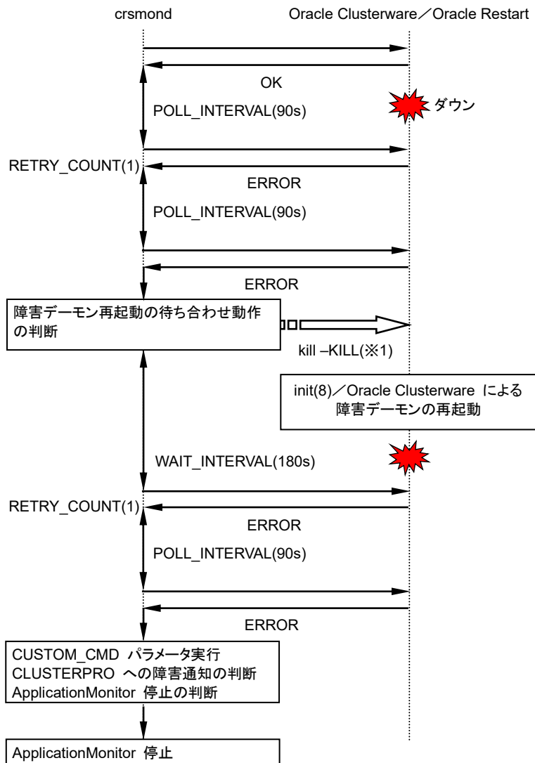
図 4-43 Oracle Clusterware/Oracle Restart 監視エラー時の動作 (init(8)/Oracle Clusterware による 障害デーモンの再起動が行われなかった場合)
