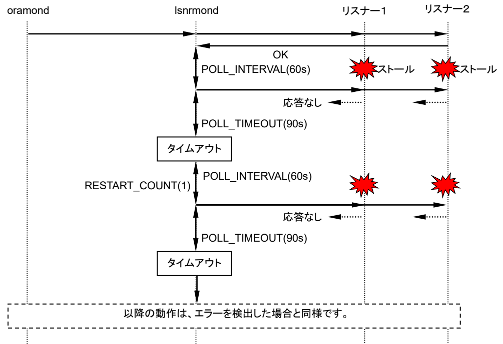
図 4-23 冗長化リスナー接続監視タイムアウト時の動作
