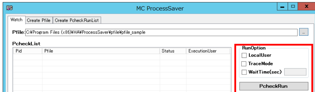
図 15 『Watch』PcheckRun 実行前画面
