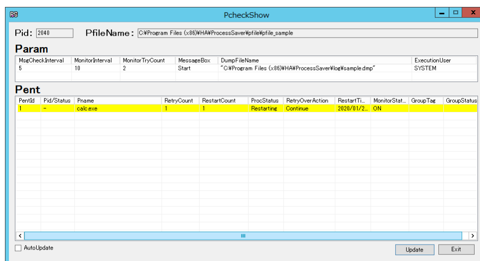
図 19 『Pcheck Show』プロセス消滅検知時画面
