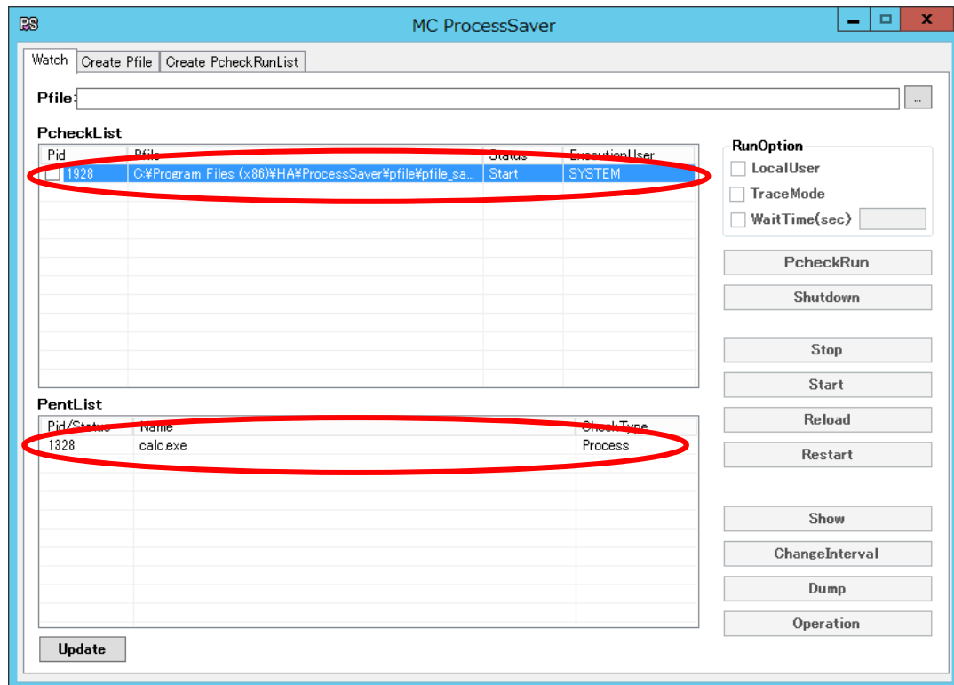
図 16 『Watch』PcheckRun 実行後画面
