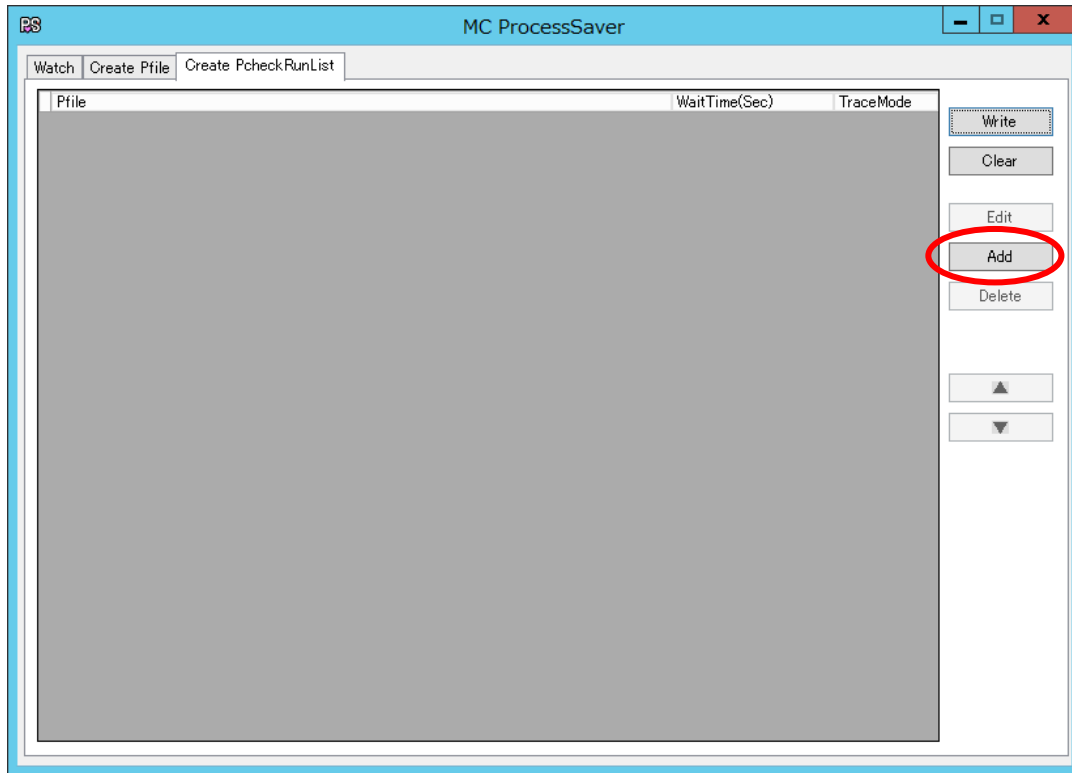
図 24 『Create PcheckRunList』
