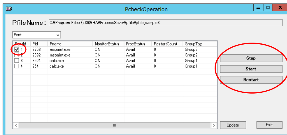
図 21 『PcheckOperation(pent)』
