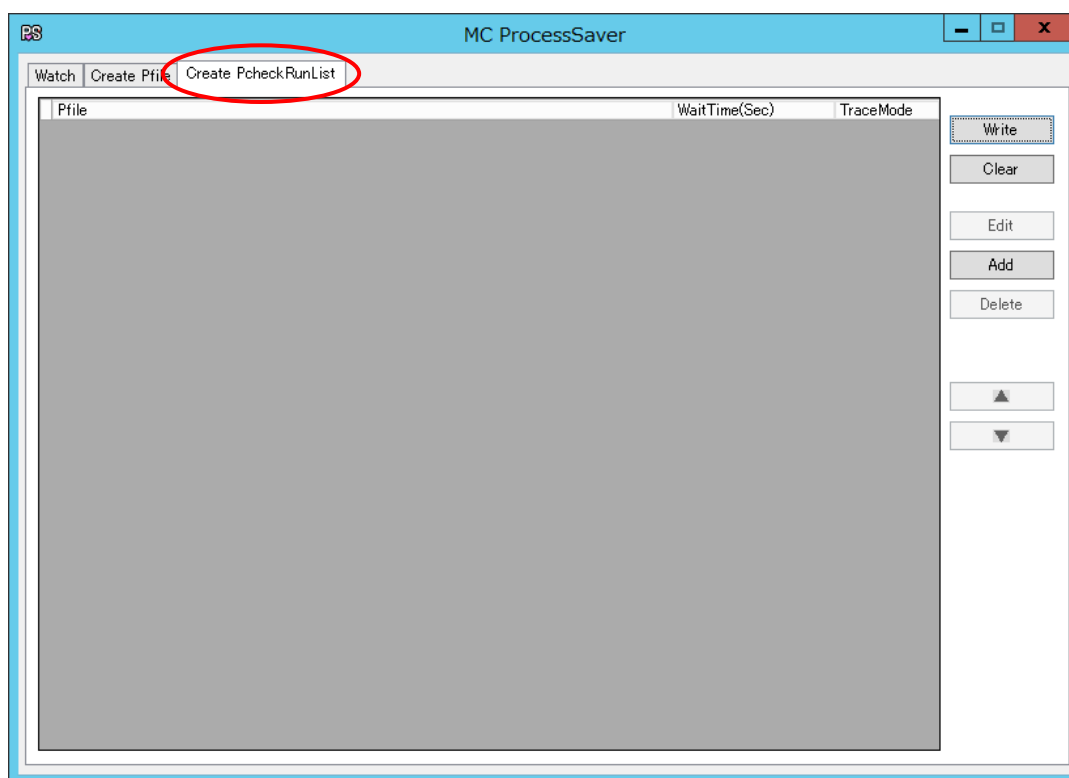
図 23 『Create PcheckRunList』
