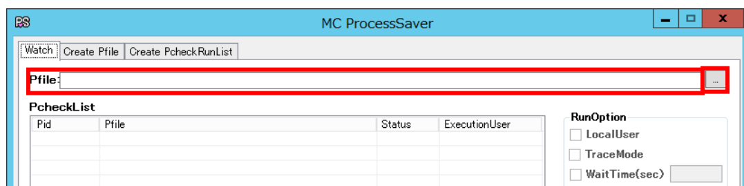
図 14 『Watch』
