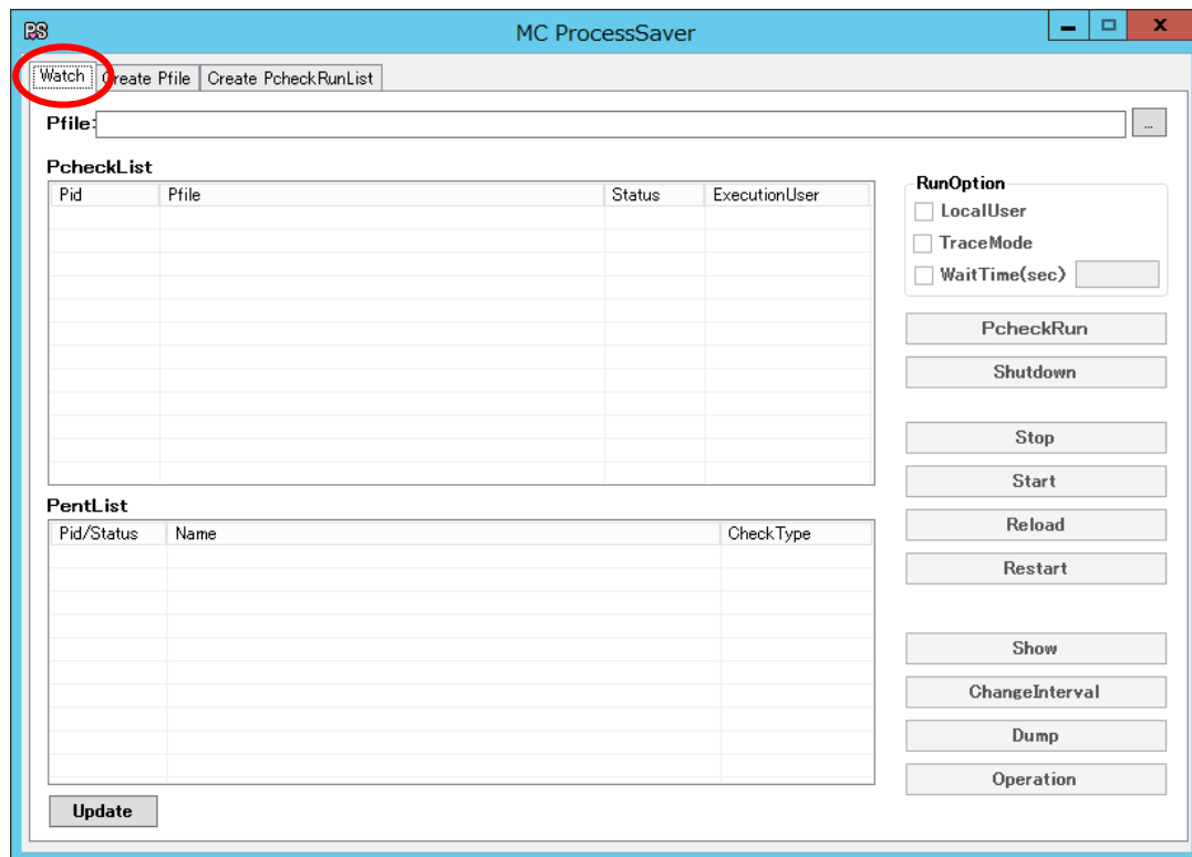
図 13 『Watch』
