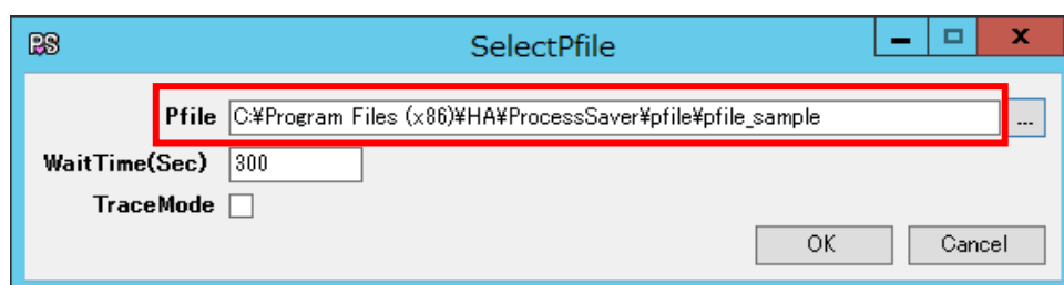
図 26 『SelectPfile』
