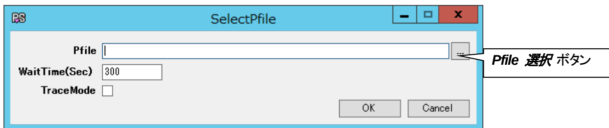
図 25 『SelectPfile』
