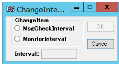
図 17 『ChangeInterval』
