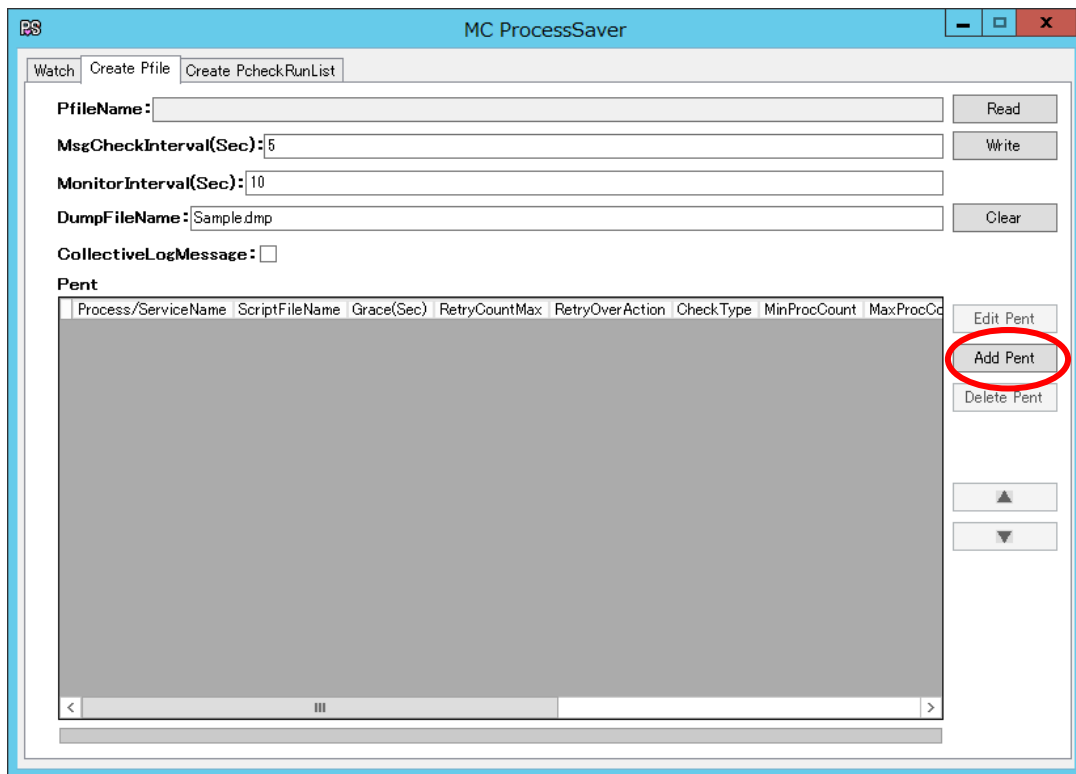
図 7 『Create Pfile』
