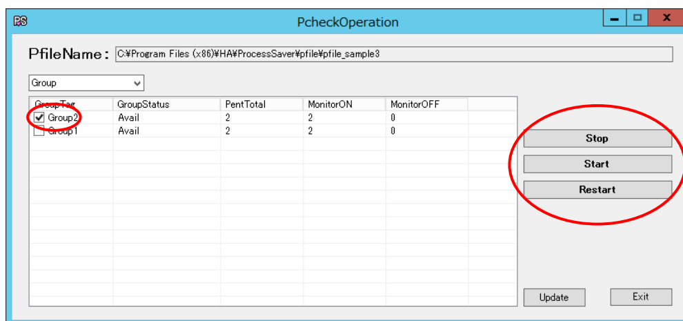
図 22 『PcheckOperation(Group)』
