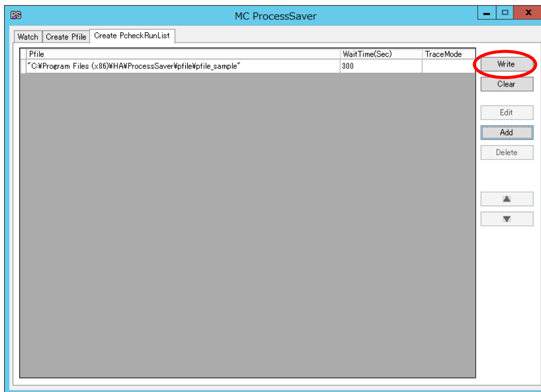
図 27 『Create PcheckRunList』
