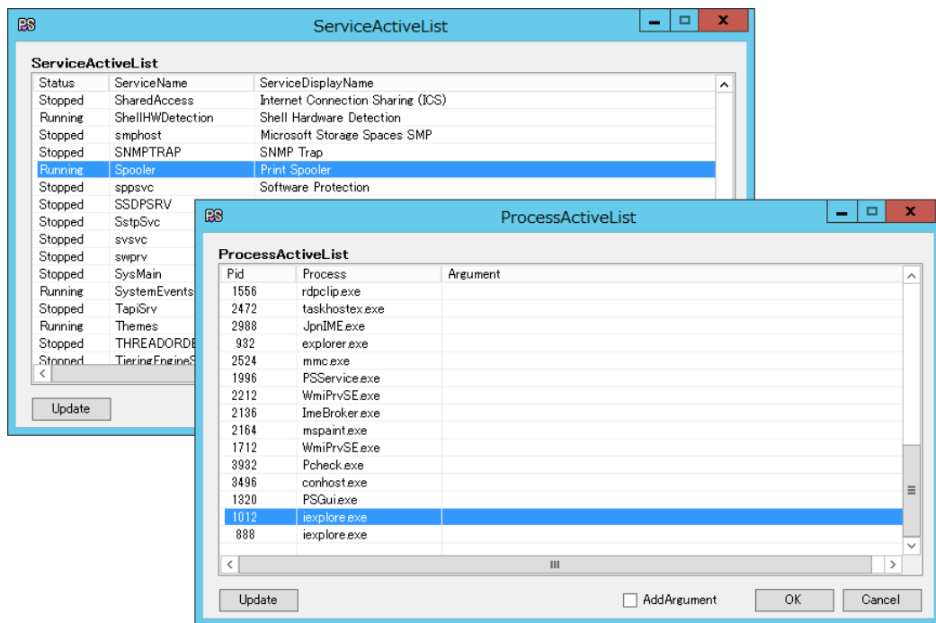
図 9 『ProcessActiveList』/『ServiceActiveList』
