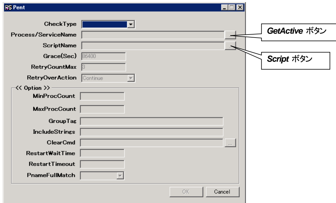
図 10 『Pent』
