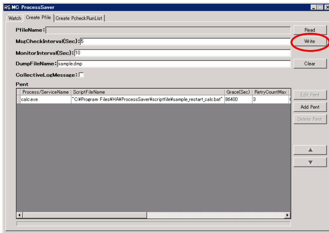
図 12『Create Pfile』
