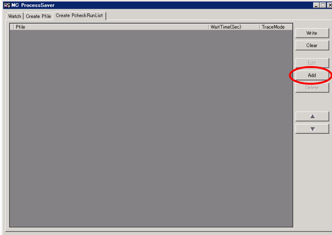
図 25 『Create PcheckRunList』
