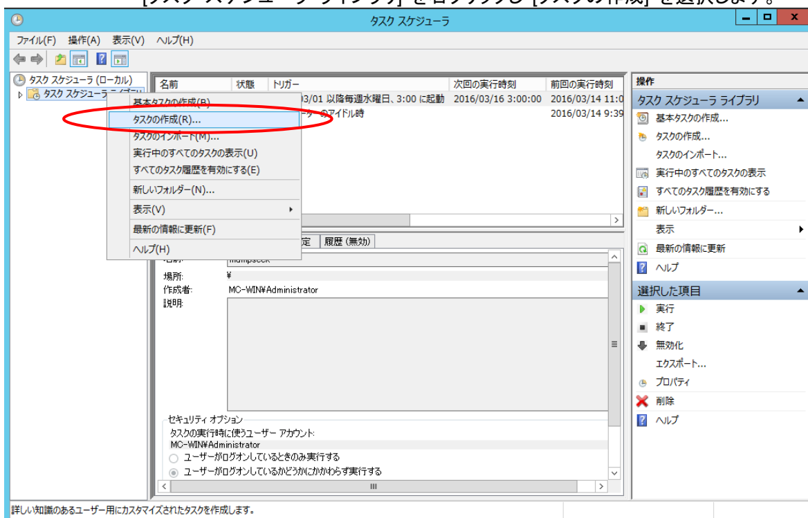
図 21 タスク作成
