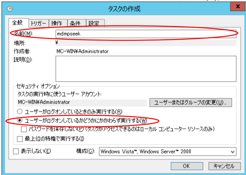
図 7 全般タブ
