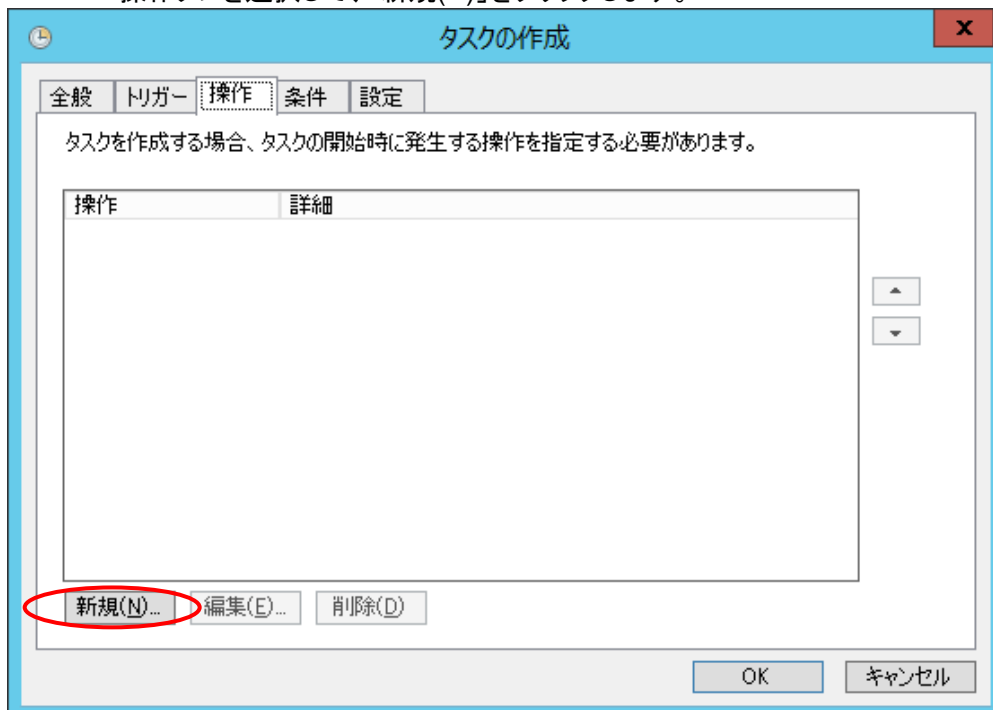
図 35 操作タブ
