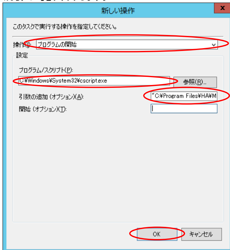
図 27 新しい操作
