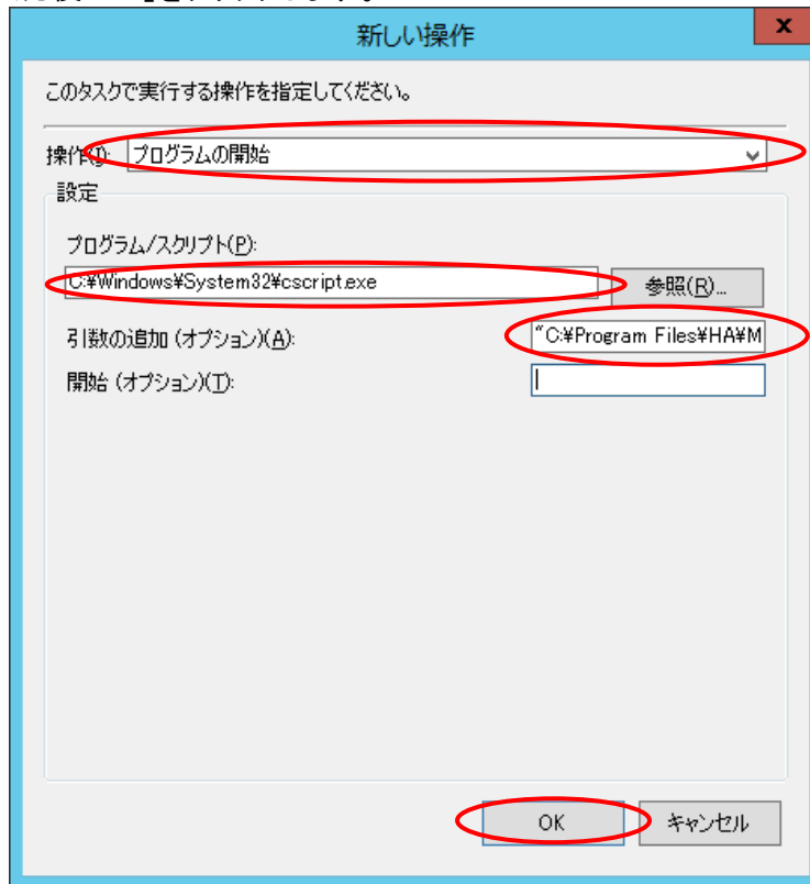
図 36 新しい操作
