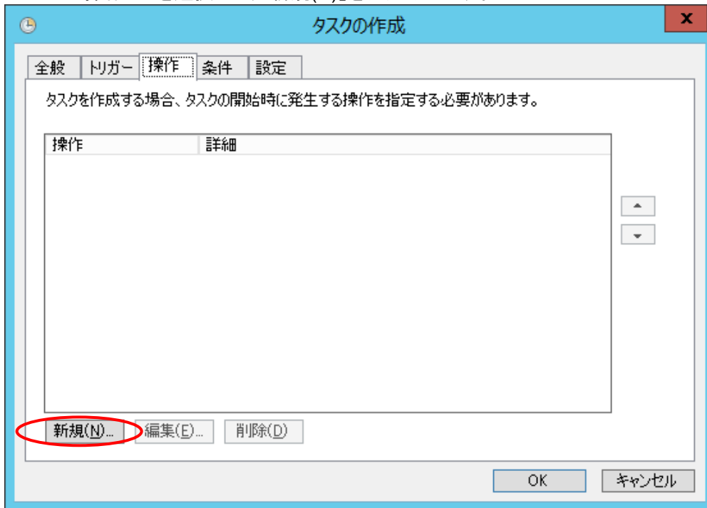
図 26 操作タブ
