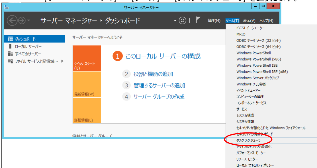
図 40 サーバermanage
