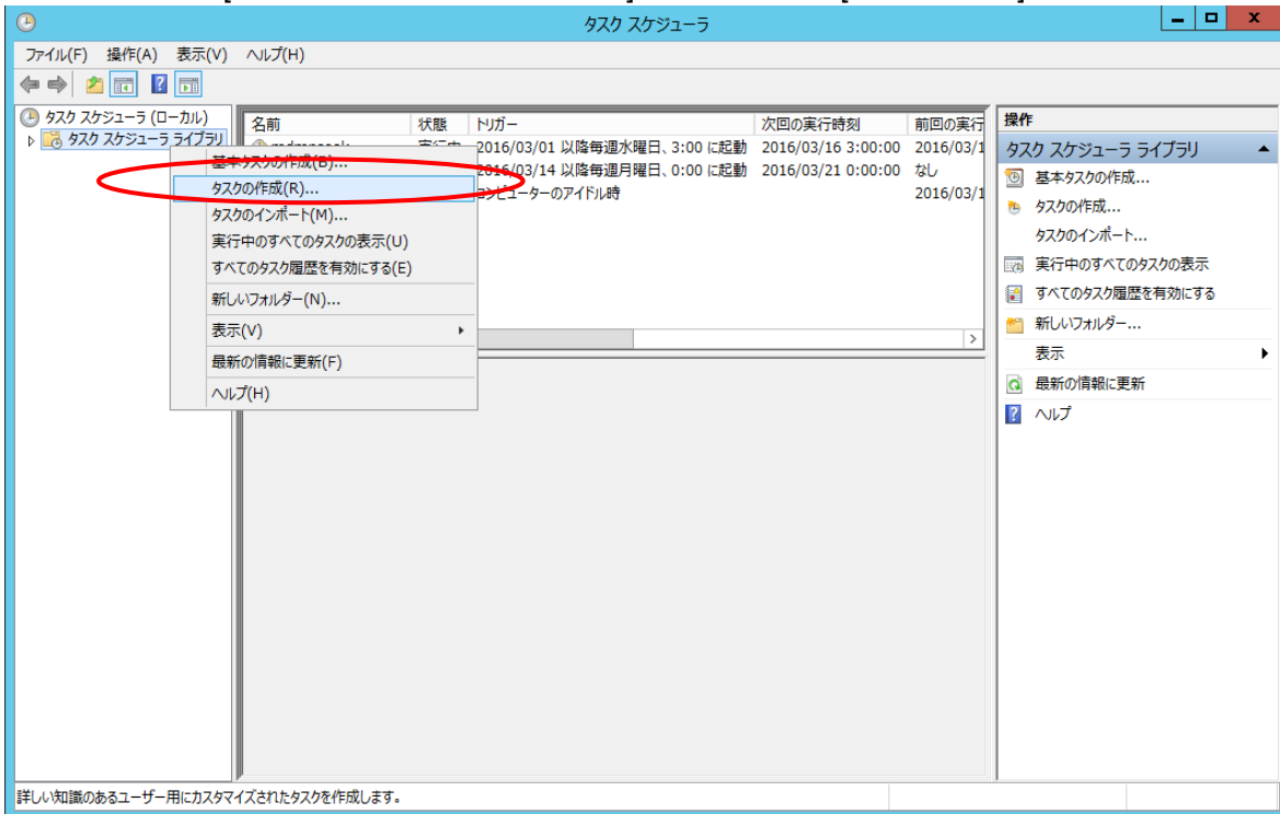
図 30 タスク作成
