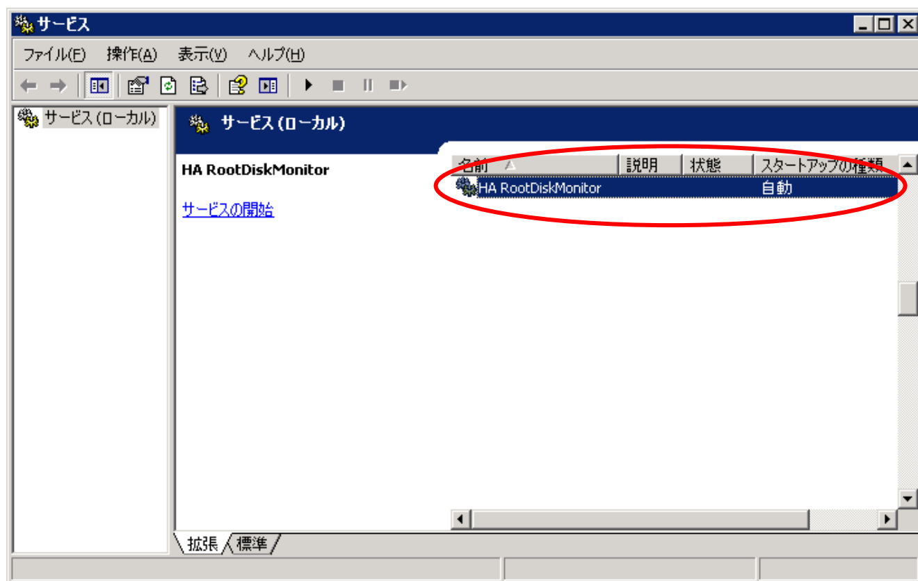
図 12 『サービス』
