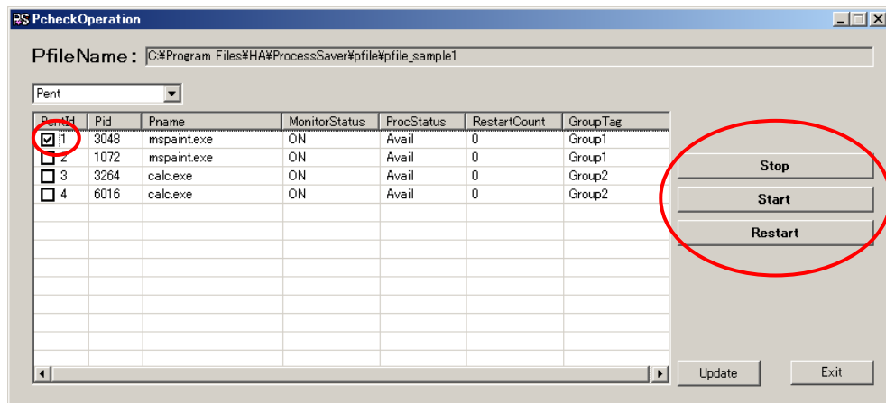
図 22 『PcheckOperation(pent)』
