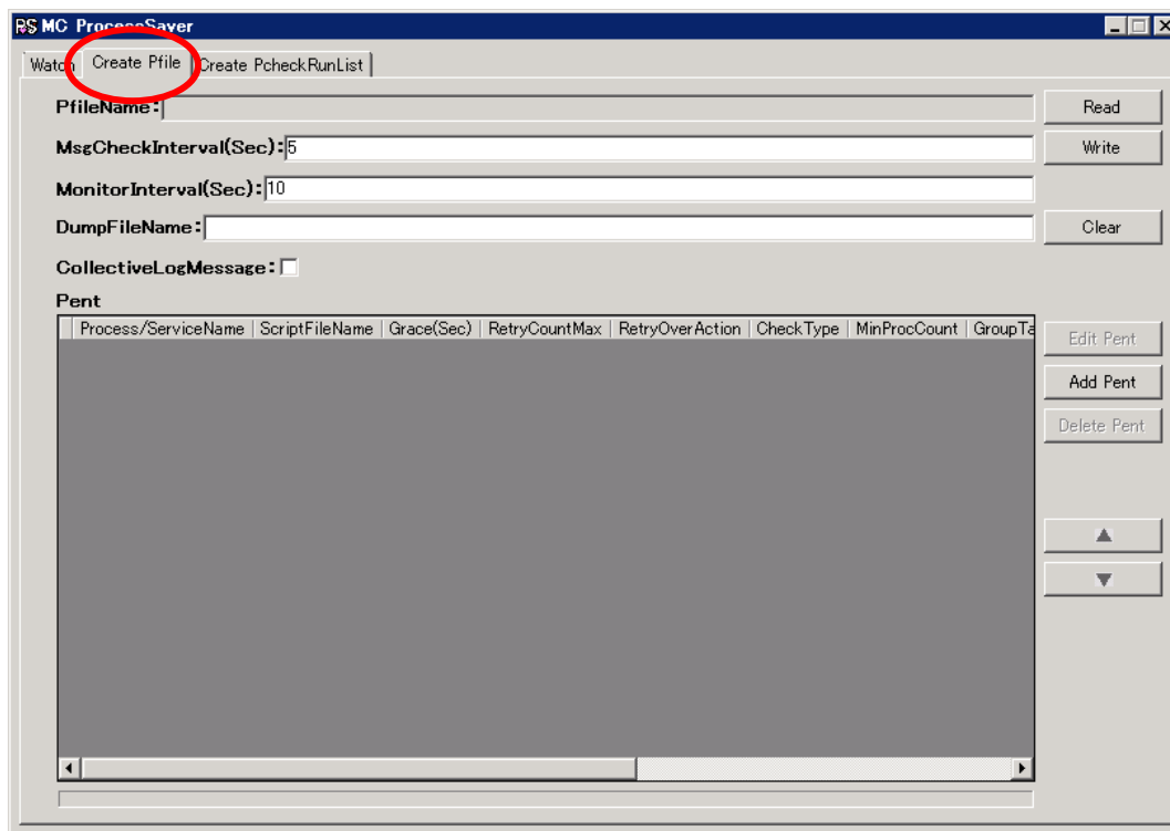
図 4 『Create Pfile』
