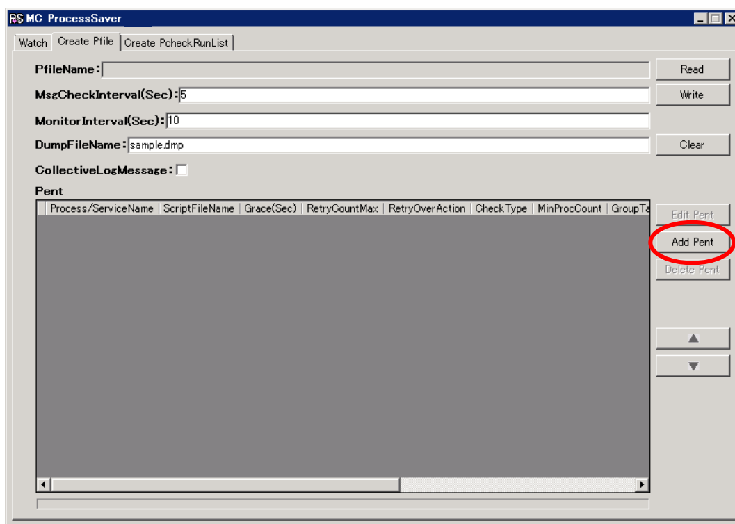
図 9 『Create Pfile』
