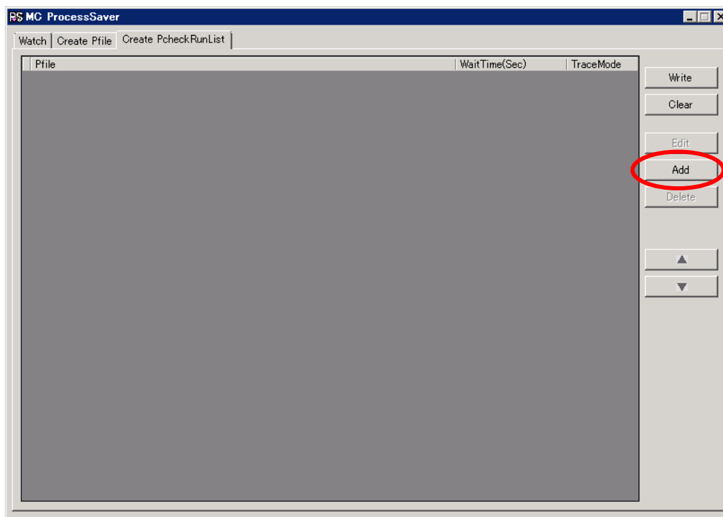
図 25 『Create PcheckRunList』
