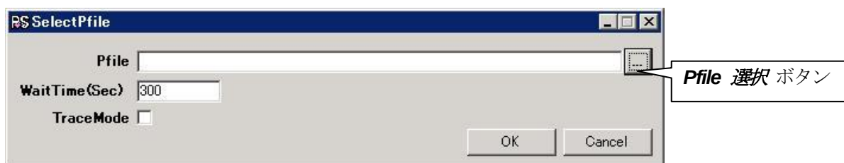
図 26 『SelectPfile』
