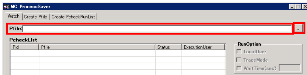
図 15「Watch」
