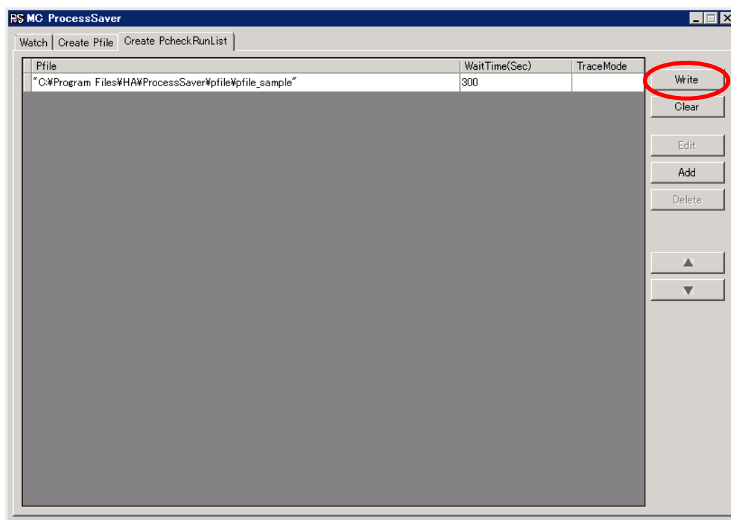
図 28 『Create PcheckRunList』
