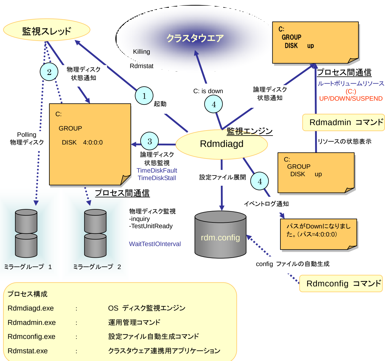
図3 RootDiskMonitor のプロセスモデル
