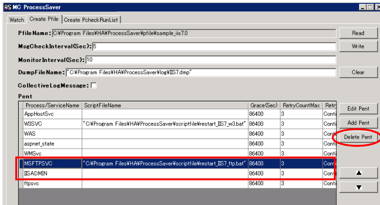
図7 『Create Pfile』
